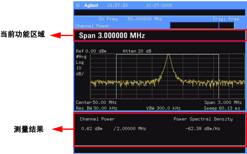
图 21 信道功率测量
