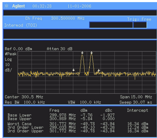
图 24 三阶交调测量
