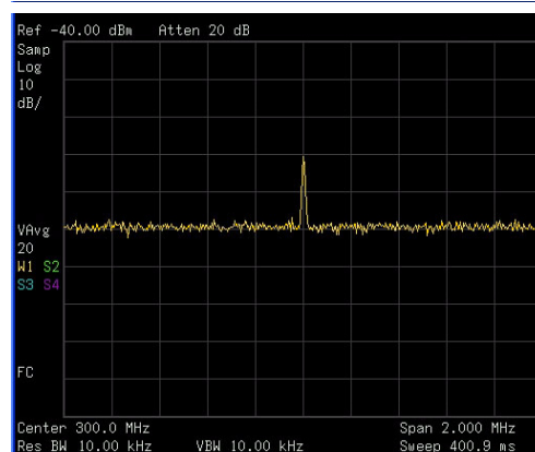
图 13 轨迹平均
