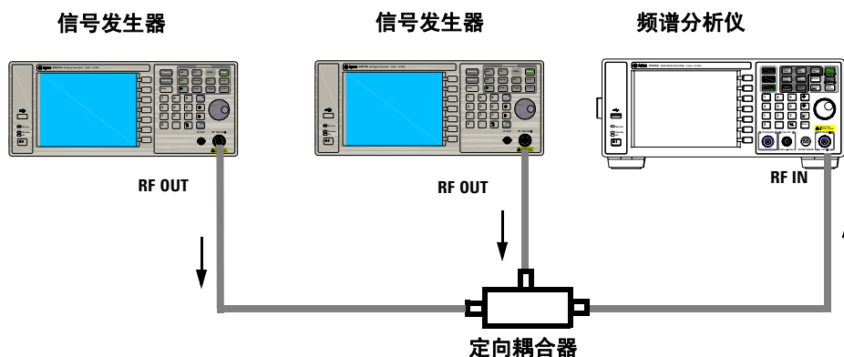
图 4 获取两路信号的仪器设置
