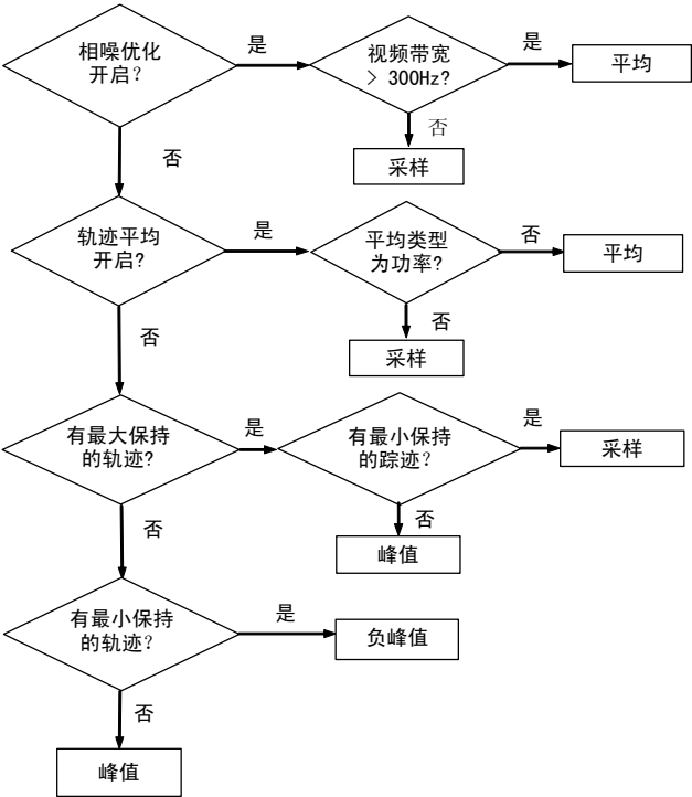
图 20 检波器自动耦合规则
