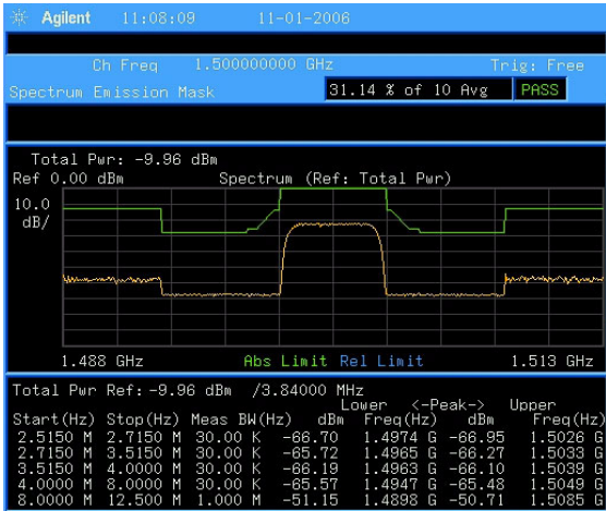
图 25 频谱泄漏模板
