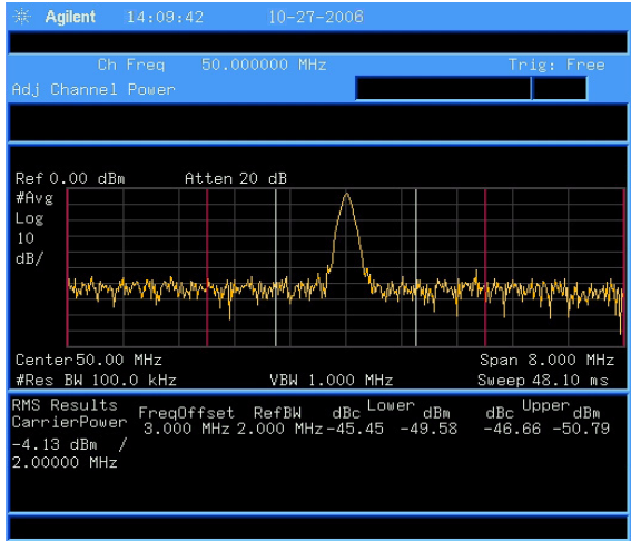
图 23 临信道功率泄漏
