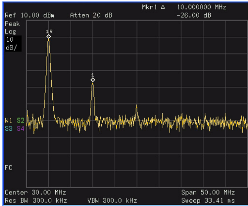
图 2 参考信号在屏幕外的 Delta 标记对
