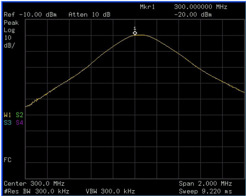
图 5 没有分辨出的两个等幅信号
