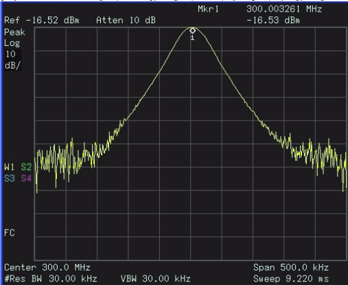
图 7 未从大信号中分辨出的小信号
