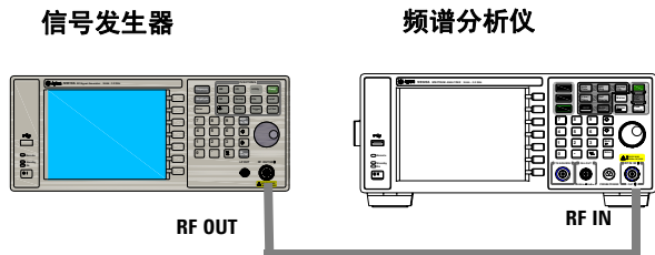
图 9 获取单一信号的仪器设置
