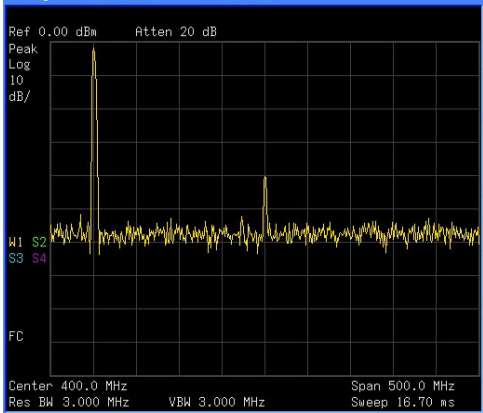
图 16 谐波失真
