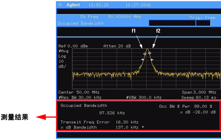
图 22 占用带宽测量
