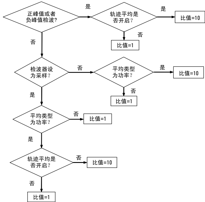
图 18 视分带宽比自动耦合规则
