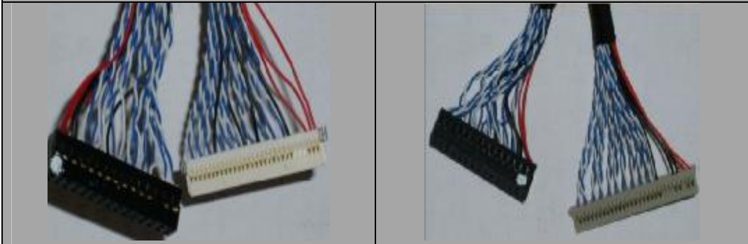
FIX-S8/30-30 (有两种不同线序, 常用) DF14-S8/30-30
