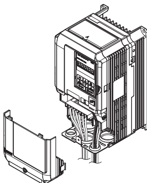
图 82 变频器的更换（端子外罩的拆卸）
