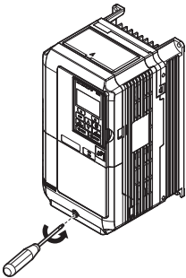
图 13 端子外罩的拆卸方法 (封闭壁挂型)
