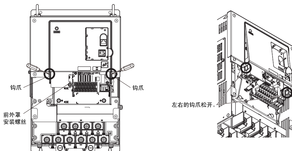
图 22 前外罩的拆卸 (2A0085 ~ 2A0415, 4A0045 ~ 4A0605)
