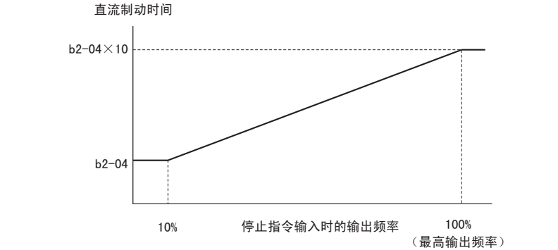
图 58 直流制动时间与输出频率的关系
