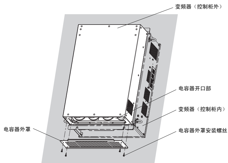
图 95 电容器外罩的安装
