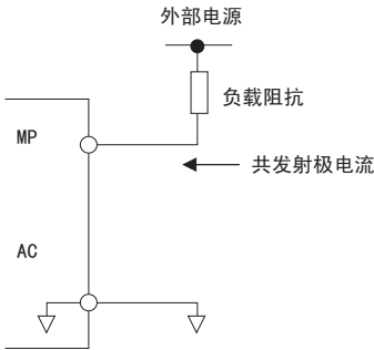
图 42 使用了外部电源的脉冲输出连接
