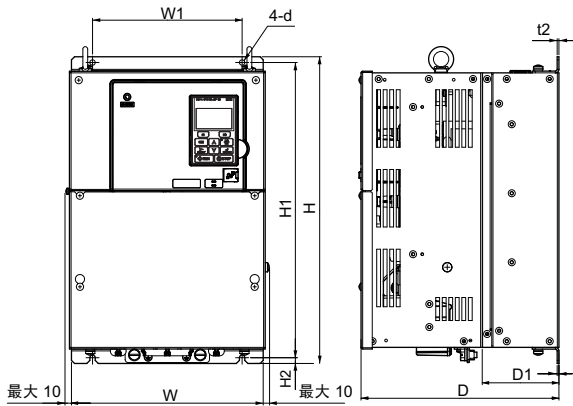
外形图 1
