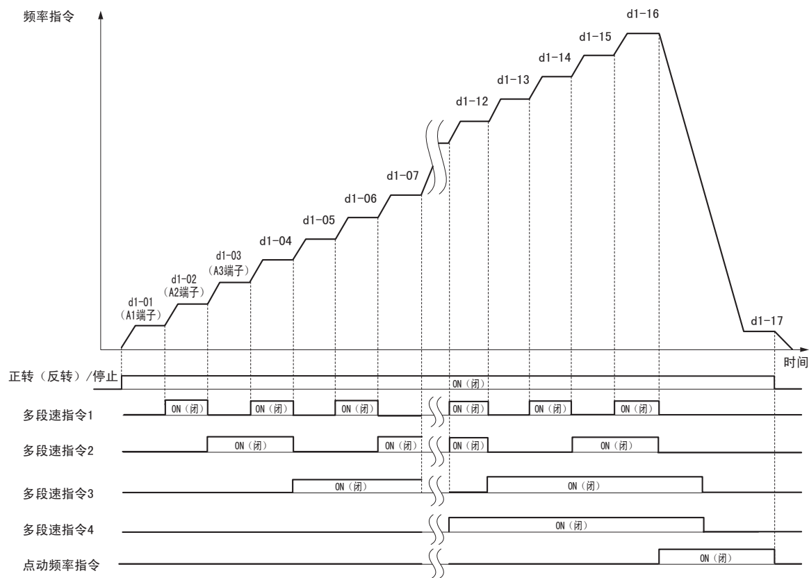
图 66 多段速指令 / 点动频率选择的时序图
