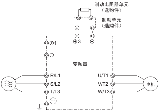
图 12 主回路端子的连接
