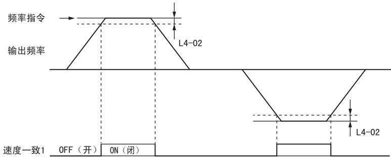
图 70 速度一致 1 的时序图
