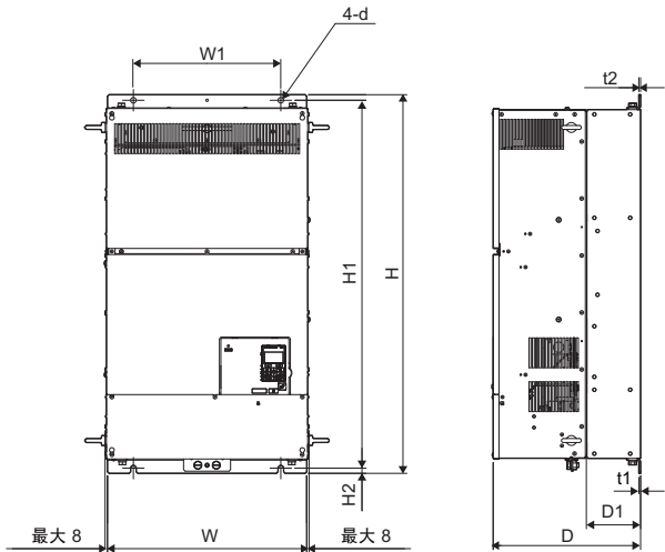
外形图 2
