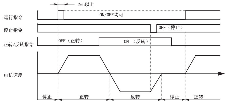
图 69 3 线制顺控的时序图
