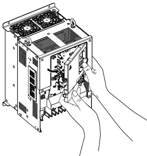
图 23 前外罩的拆卸 (2A0085 ~ 2A0415, 4A0045 ~ 4A0605)
