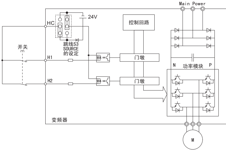
图 99 安全输入的接线示例（SOURCE 模式）
