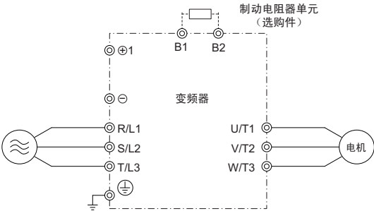
图 11 主回路端子的连接
