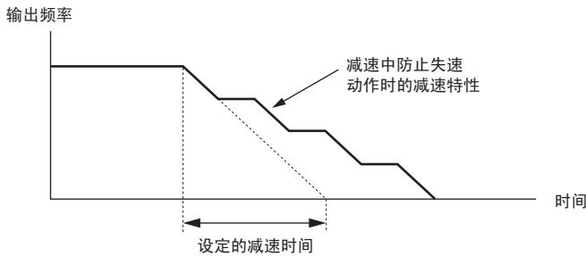
图 78 减速中防止失速的动作示例
