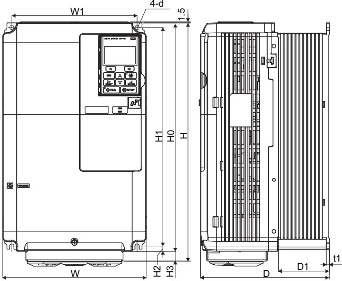
外形图 2
