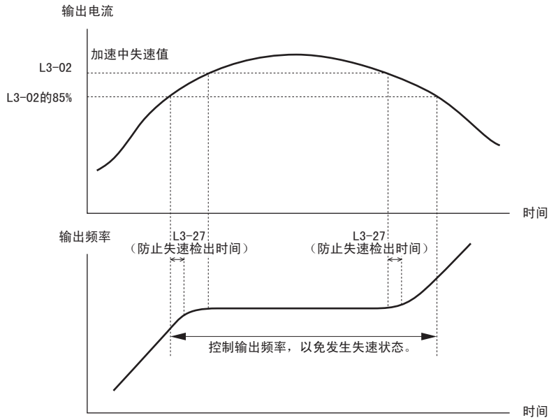
图 75 使用 IM 电机时的加速中防止失速功能
