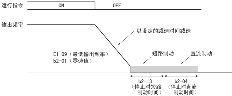
图 54 减速停止（PM 用无 PG 矢量控制、PM 用无 PG 高级矢量控制模式时）
