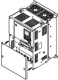
图 17 端子外罩的拆卸方法（柜内安装型）
