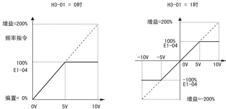
图 72 调整了模拟量输入的增益设定时的频率指令
