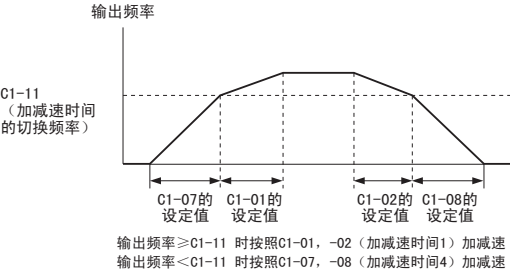
图 65 加减速时间的切换频率
