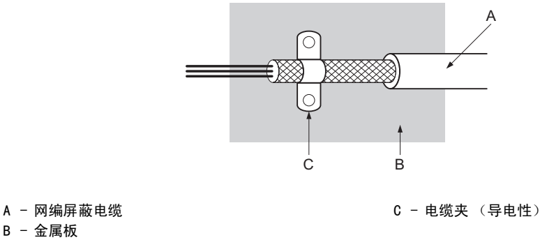
图 90 电缆的接地方法
