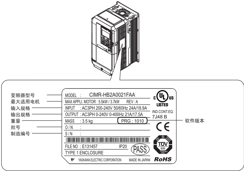
图 3 变频器的铭牌
