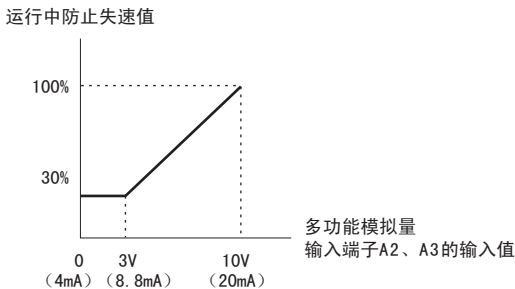
图 79 通过模拟量输入设定运行时防止失速值
