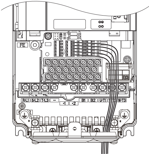
图 35 控制回路的接线（TB4、TB5、TB6）
