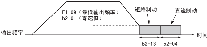
图 62 停止时短路制动（无 PG：PM 电机）
