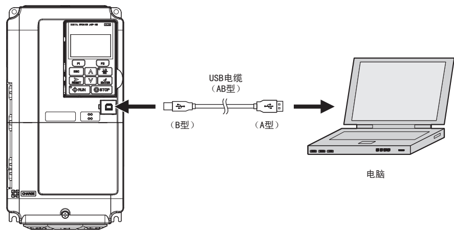
图 44 与电脑的连接（USB）
