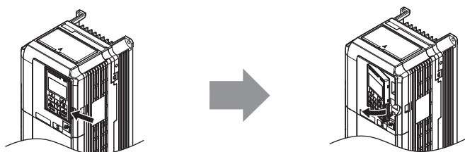
图 19 操作器的拆卸
