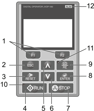
图 45 操作器各部分的名称与功能
