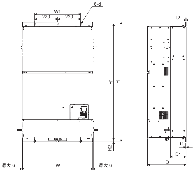
外形图 3
