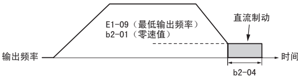
图 61 无 PG V/f 控制、带 PG V/f 控制、无 PG 矢量控制时的停止时直流制动动作
