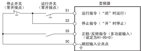
图 68 3 线制顺控的接线示例
