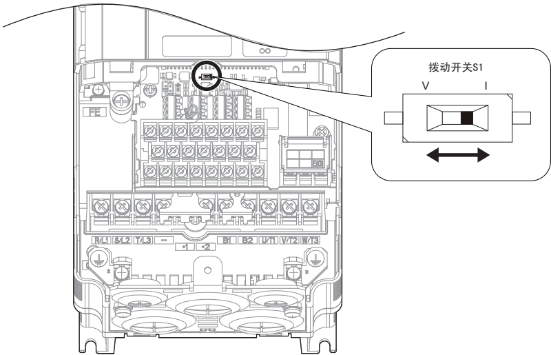
图 43 拨动开关 S1
