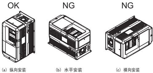
图 4 安装方向
