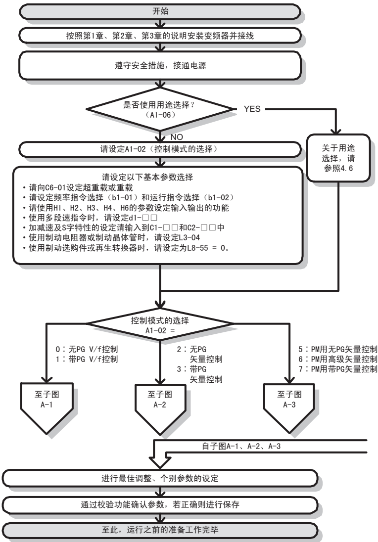
图 47 运行前的基本步骤
