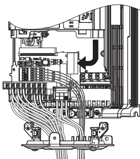
图 84 变频器的更换（端子排的拆卸）
