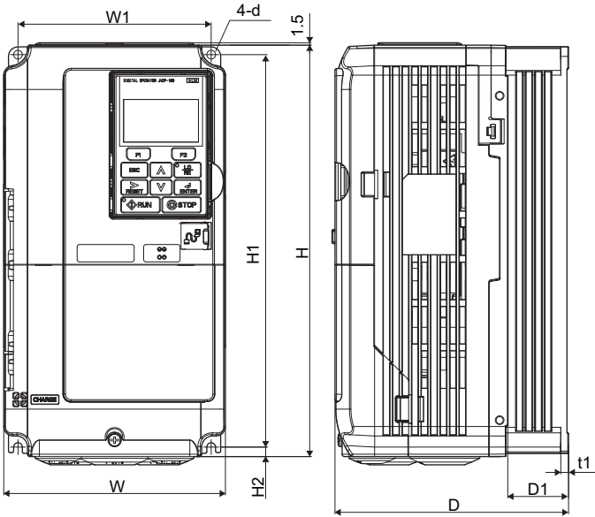
外形图 1
