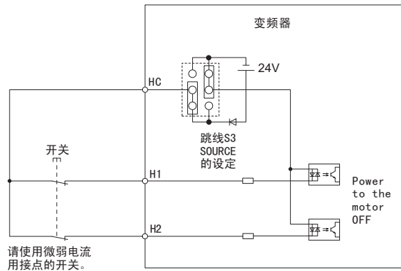
图 104 安全输入的连接示例（双工化）
