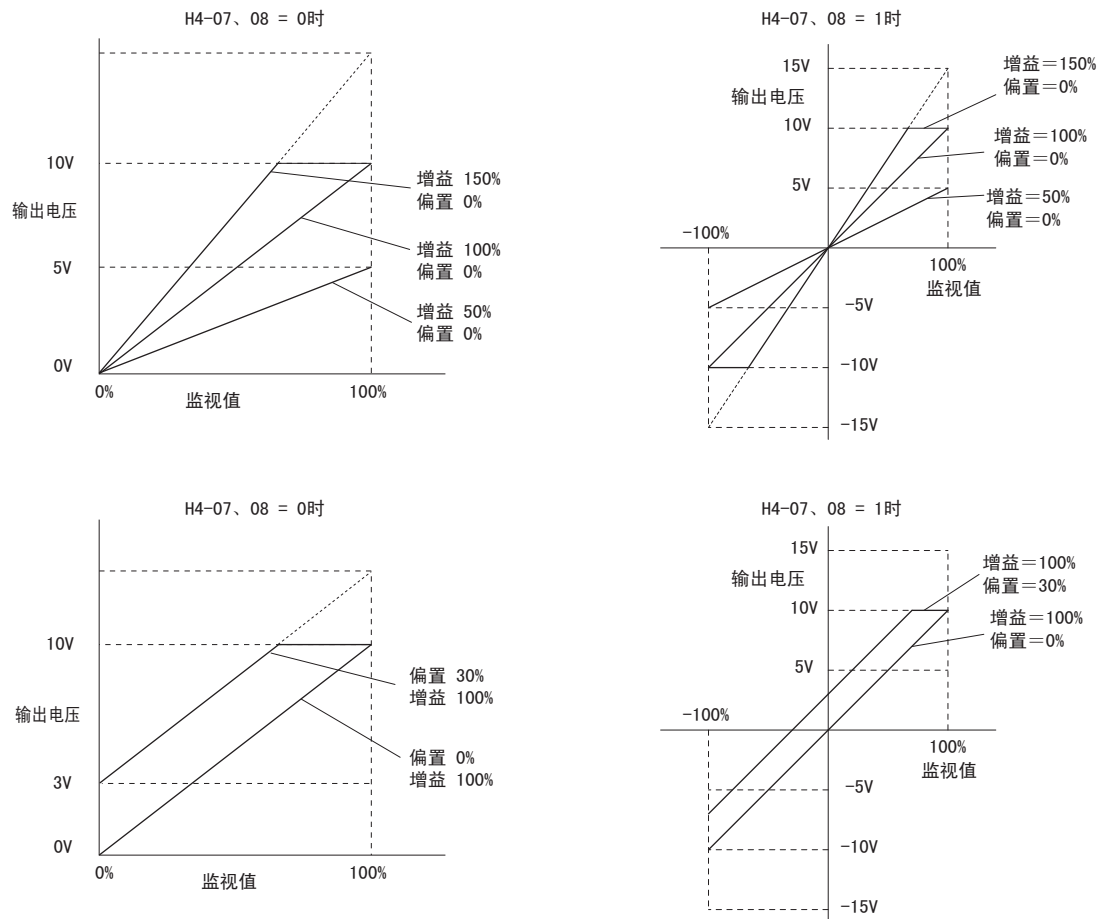
图 74 模拟量输出的增益 / 偏置设定
