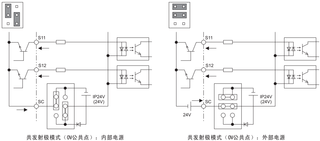
图 38 共发射极模式（0V 公共点）
