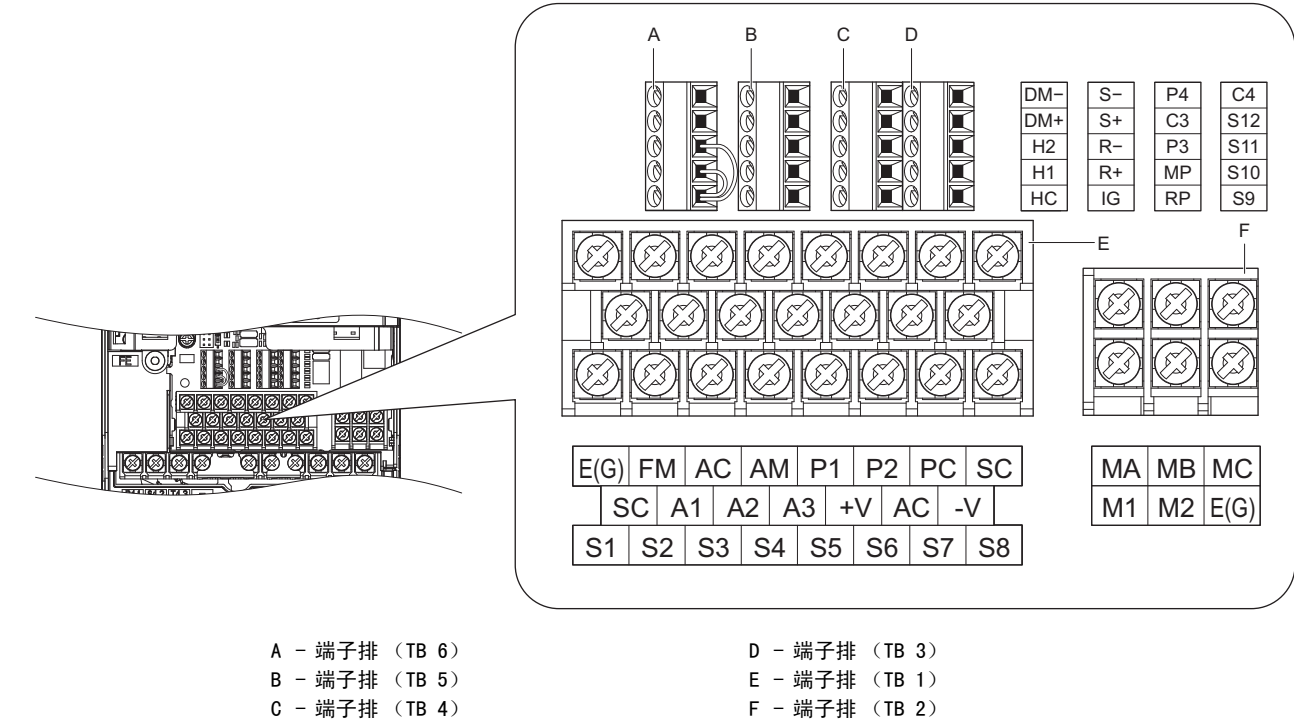
图 31 带参数备份功能的拆装式端子排的排列 (CIMR-HB□□□□□□□□)
