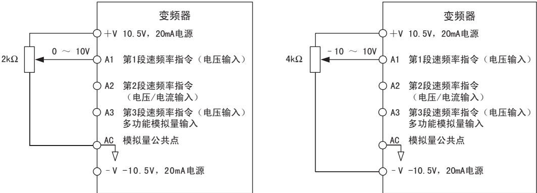
图 51 端子 A1 的电压输入设定示例
