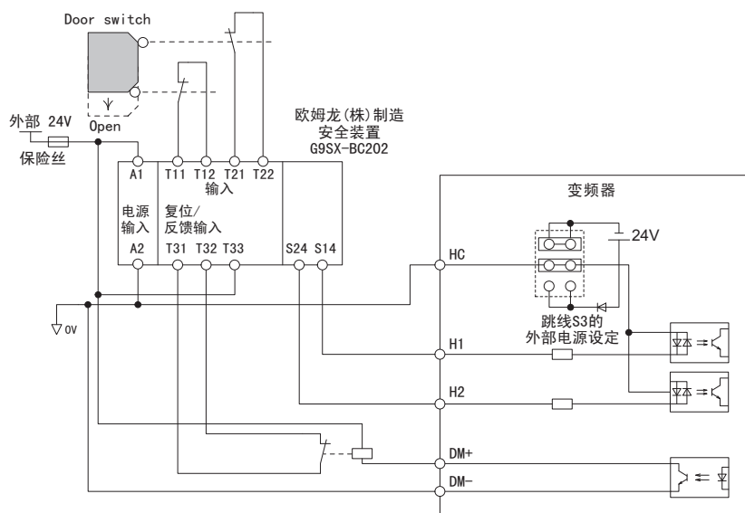
图 106 安全功能的连接示例
