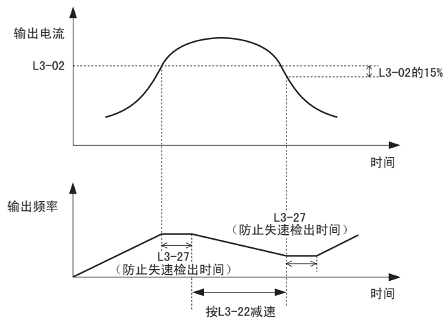
图 76 PM 用无 PG 矢量控制时的加速中防止失速功能
