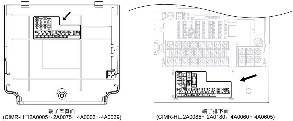
图 32 端子排的排列标示
