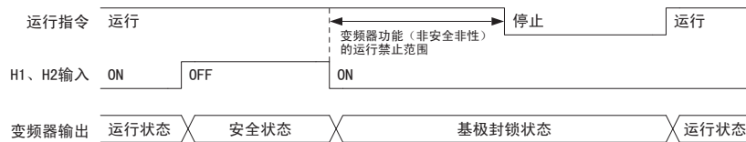
图 103 从安全状态（STO 状态）返回 （在运行过程中 H1、H2 输入变为 OFF 而进入安全状态时）
