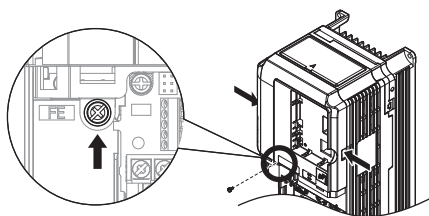
图 21 前外罩的拆卸 (2A0005 ~ 2A0075, 4A0003 ~ 4A0039)
