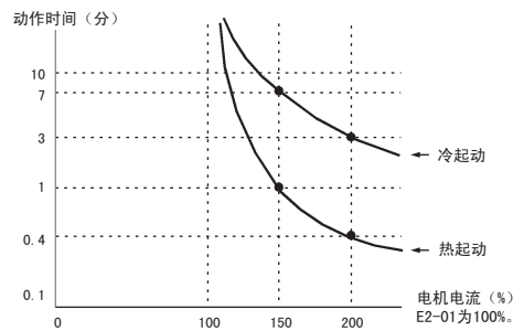
图 94 由输出频率和负载决定的电机过载保护时间
