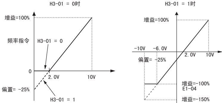
图 73 设定了负值偏置时的频率指令
