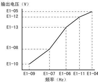
图 67 V/f 曲线图
