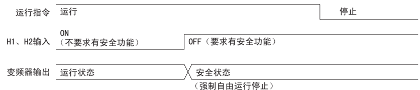
图 101 如果在运行中将安全输入置为 OFF，电机将自由运行停止
