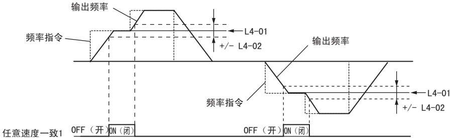
图 71 任意速度一致 1 的时序图
