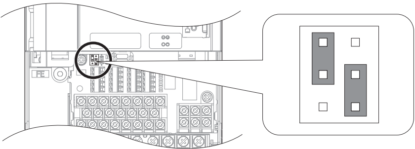
图 37 跳线 S3
