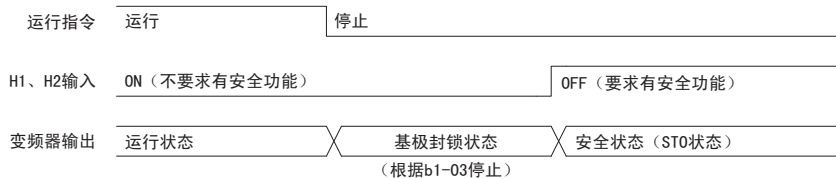
图 100 安全功能动作时的变频器状态
