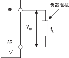
图 41 使用了内部电源的脉冲输出连接
