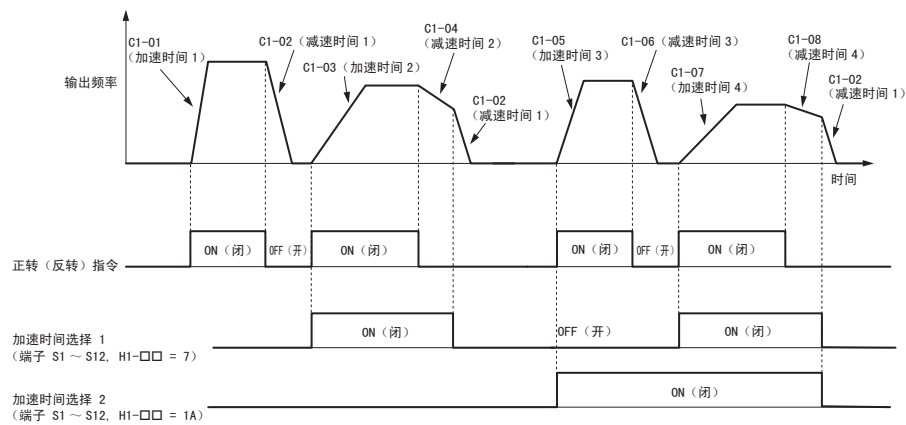
图 64 加减速时间的时序图
