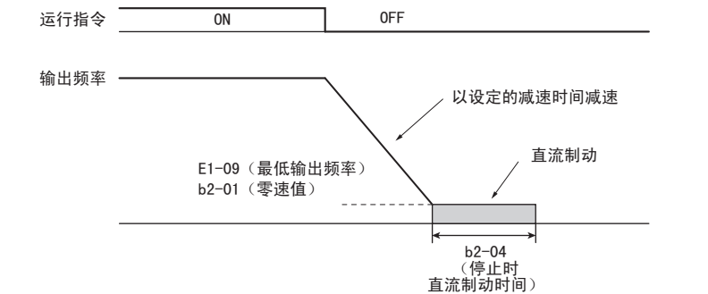
图 53 减速停止（无 PG V/f 控制、带 PG V/f 控制、无 PG 矢量控制模式）
