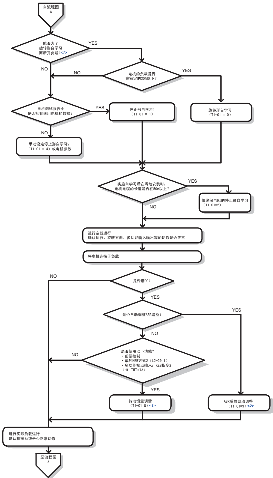
图 49 无 PG / 带 PG 矢量控制下的高精度运行
