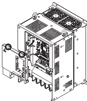
图 24 前外罩的安装（2A0085 ~ 2A0415, 4A0045 ~ 4A0605）
