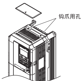
图 26 上部保护罩的安装
