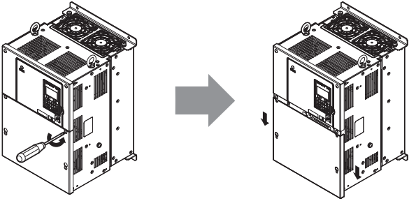
图 16 端子外罩的拆卸方法（柜内安装型）
