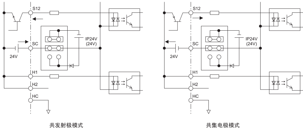
图 40 不使用安全输入时的接线示例
