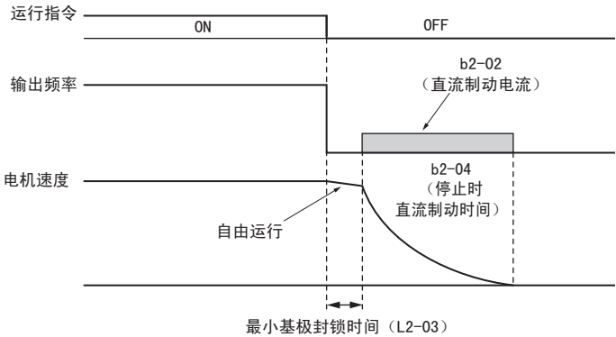
图 57 全域直流制动（DB）停止
