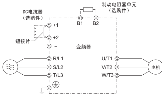
图 10 主回路端子的连接
