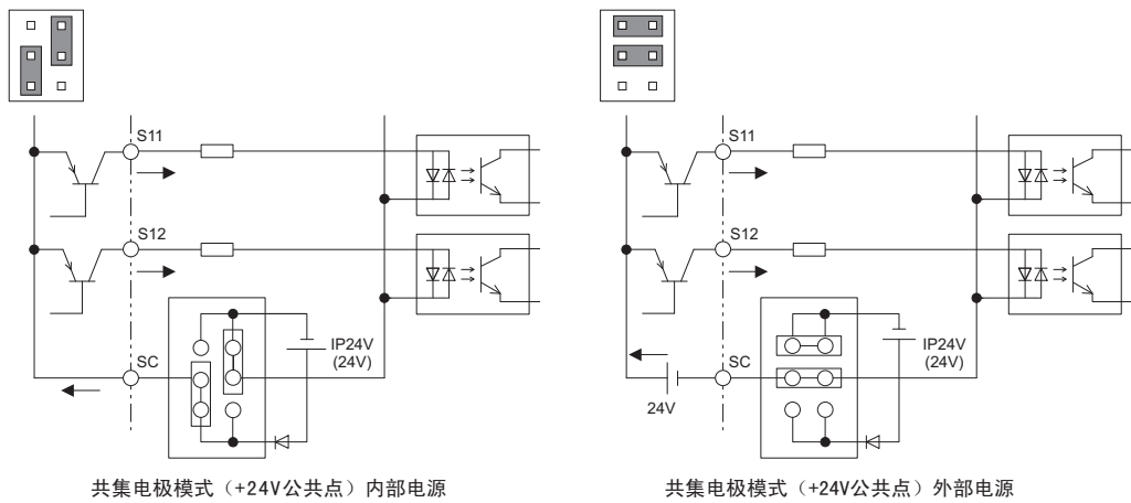
图 39 共集电极模式（+24V 公共点）
