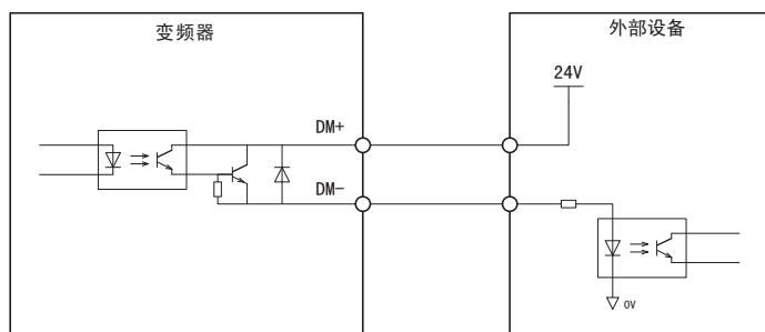
图 105 安全监视输出的连接示例
