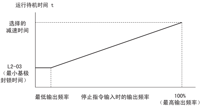
图 60 运行等待时间与输出频率的关系
