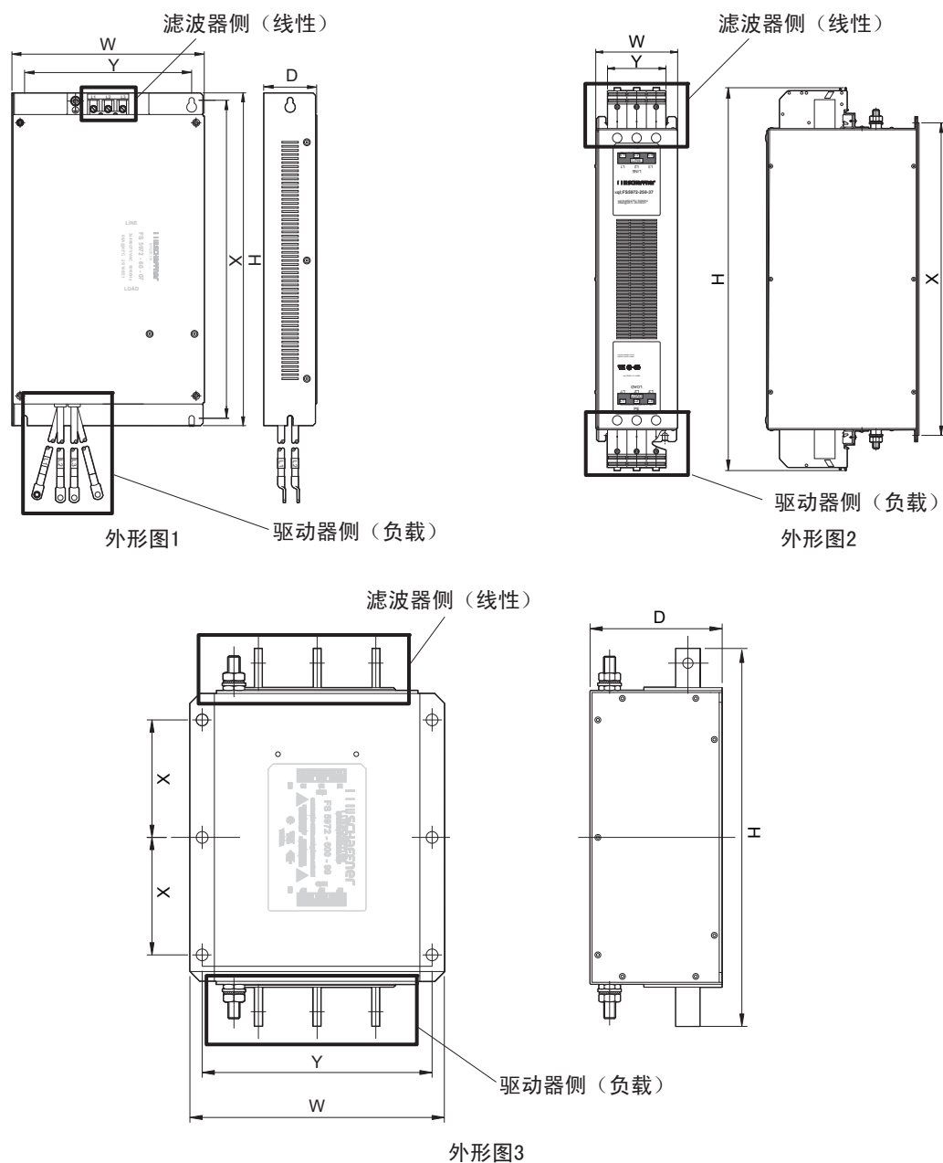
图 92 EMC 噪声滤波器的外形尺寸
