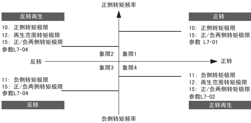
图 80 模拟量输入的转矩极限
