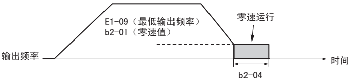
图 63 停止时零速运行
