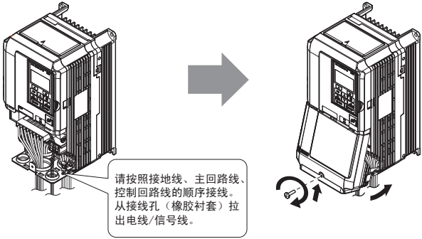
图 15 端子外罩的安装方法（封闭壁挂型）
