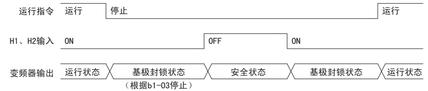
图 102 从安全状态（ST0 状态）返回
