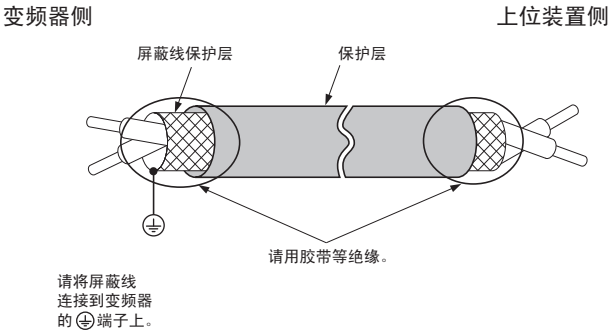
图 36 屏蔽线的线头处理
