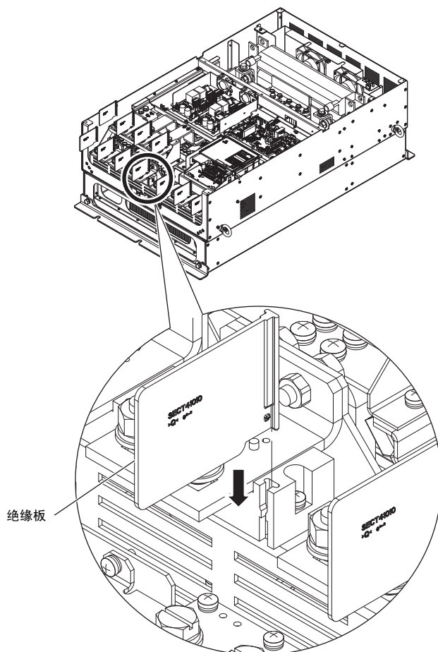
图 27 绝缘板的安装
