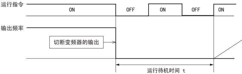
图 59 带定时的自由运行停止
