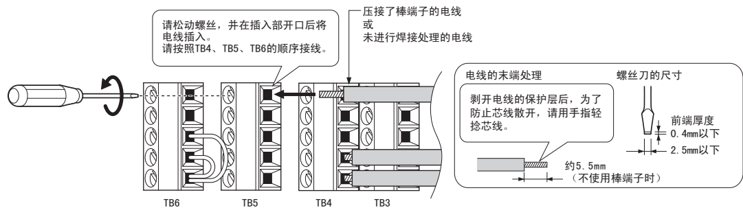
图 34 控制回路的接线步骤
