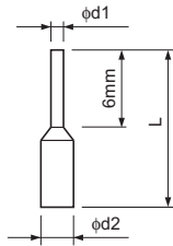
图 33 棒端子的外形尺寸图
