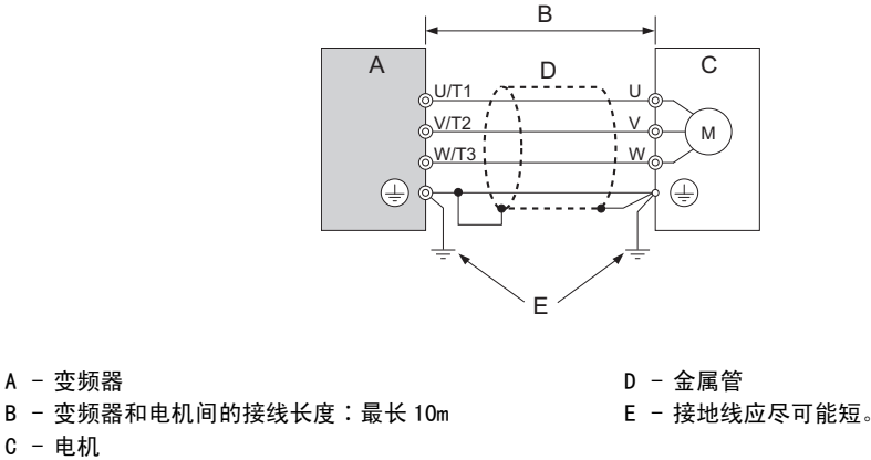
图 89 安装方法
