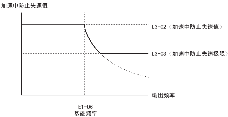
图 77 加速中防止失速值 / 极限
