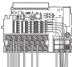
图 85 变频器的更换 （已拆下的拆装式端子排）
