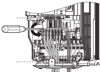
图 83 变频器的更换（拧松固定螺丝）
