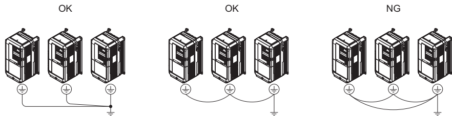
图 28 多台变频器的接线
