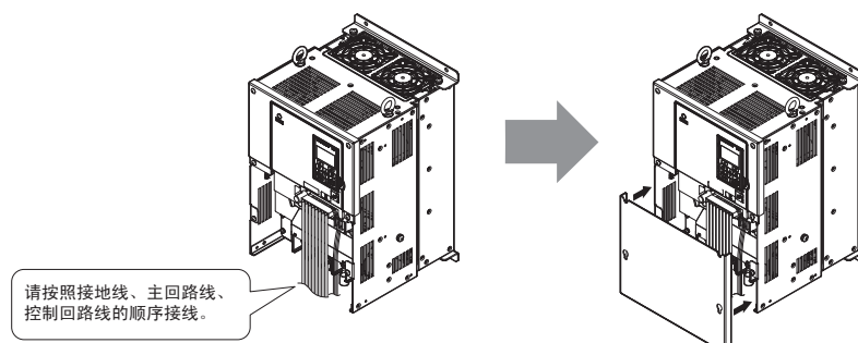
图 18 端子外罩的安装方法（柜内安装型）
