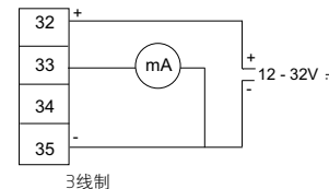
3线制
