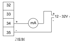
2线制
