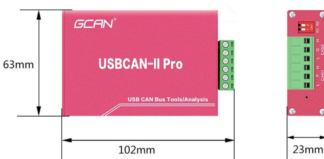
图 2.1 USBCAN-II Pro 外形尺寸
