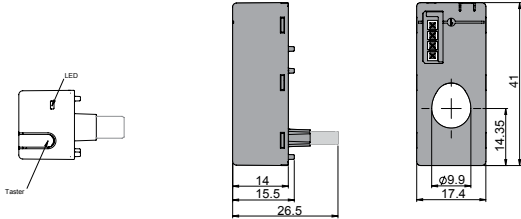
互感器 (CMS-100PS)
