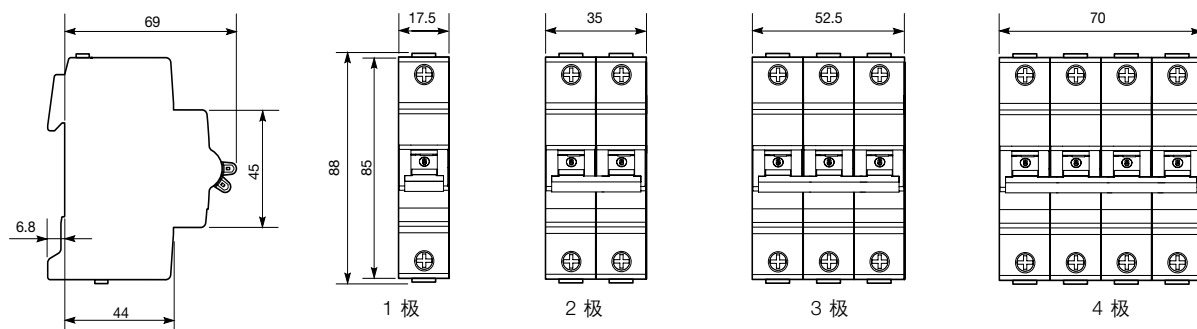
M200M 外形尺寸 (与S200系列一致)
