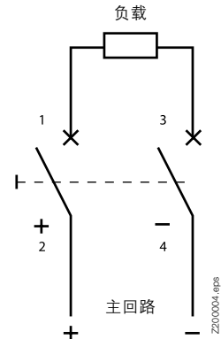
接线图
