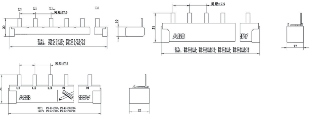
尺寸图
