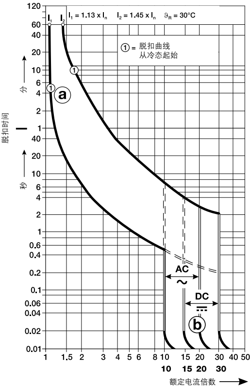
脱扣特性 D
