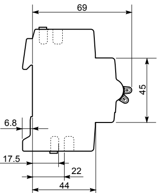
外形尺寸图（mm）
