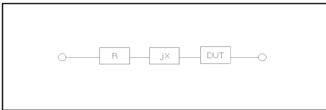
图 3-2 寄生阻抗
