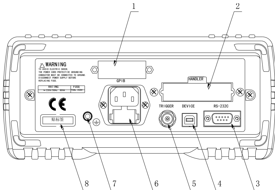
图 2-2. 后面板说明
