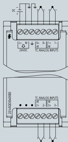
6ES7 231-5QD30-0XB0
