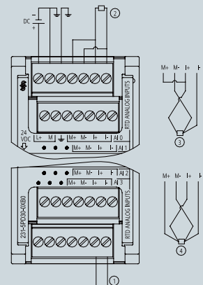
6ES7 231-5PD30-0XB0
