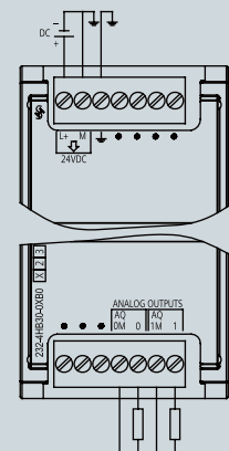
6ES7 232-4HB30-0XB0
