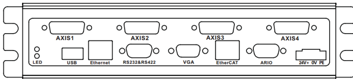
图表 4.2-1 控制器接口定义图 ( 1 )
