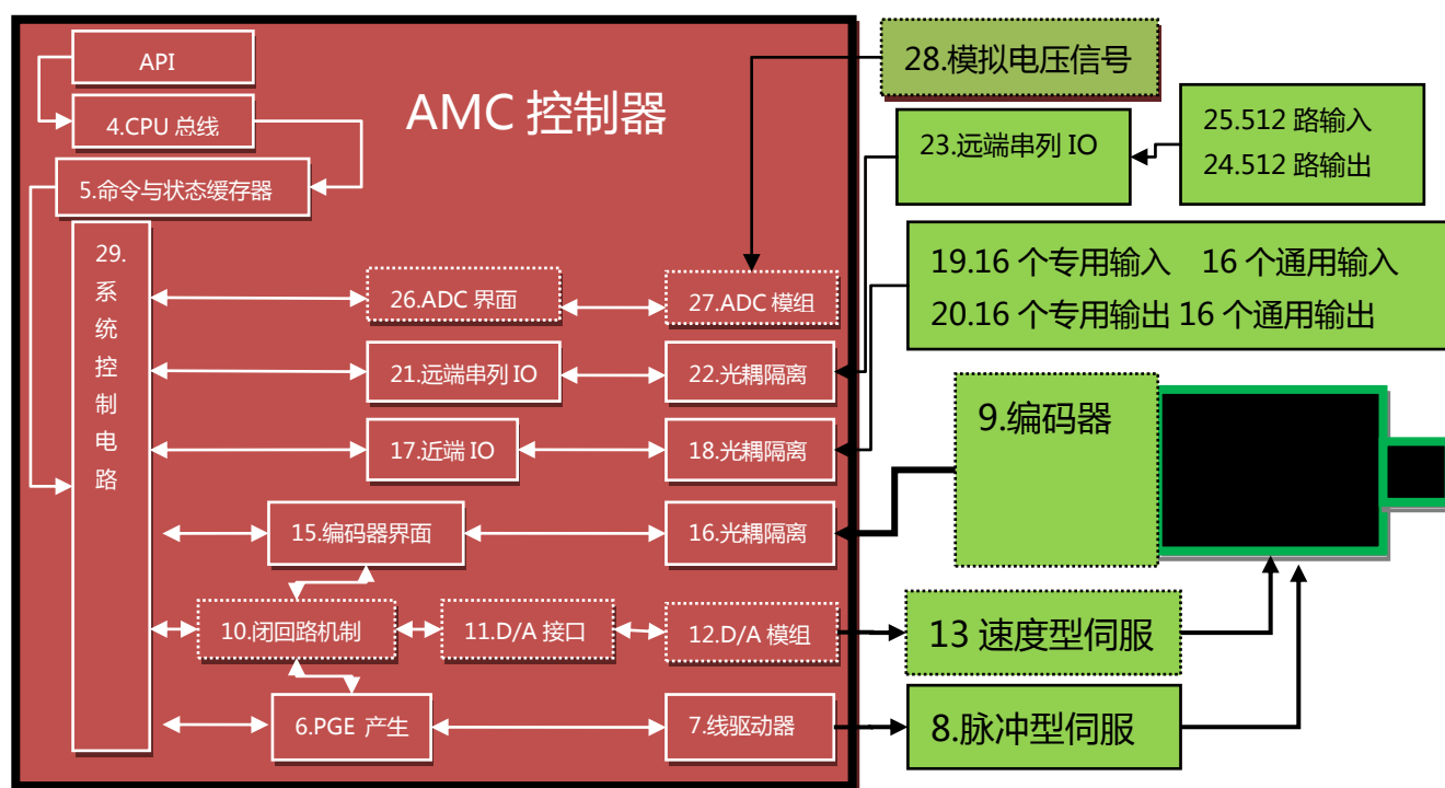
图表 2.2-2 控制框图
