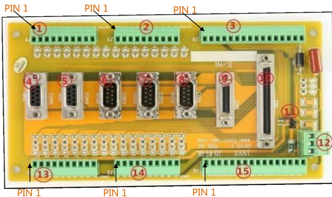
图表 4.4-1 扩展板接口分布图
