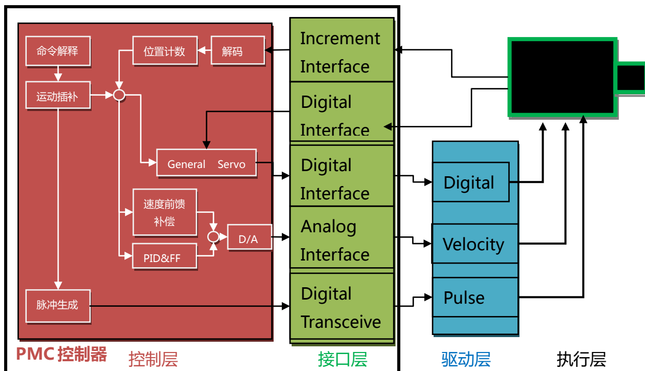
图表 2.2-2 控制模块图
