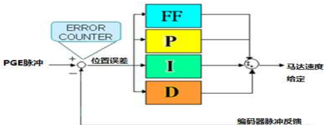
图表 2.2-4 闭合路控制为 PID 和 FF 控制法
