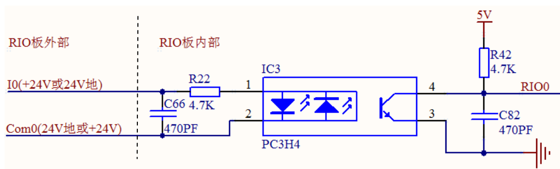
图表 4.5-1 ARIO 输入电路
