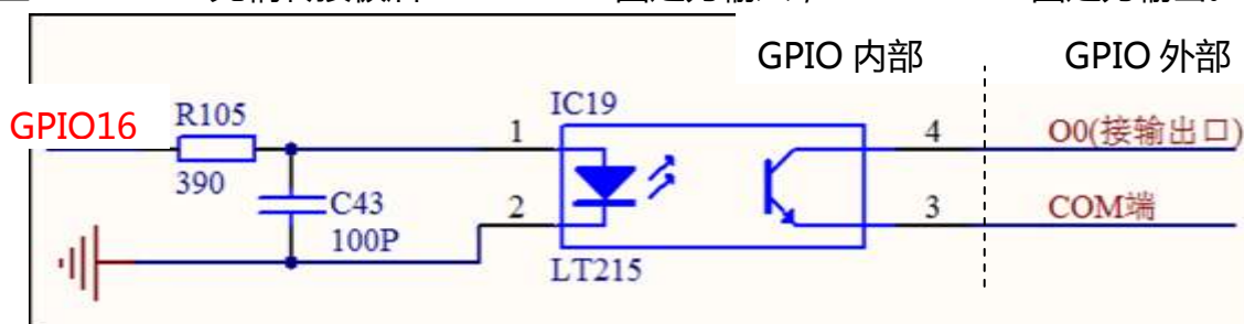
图表 4.4-2 GPIO 输出电路
