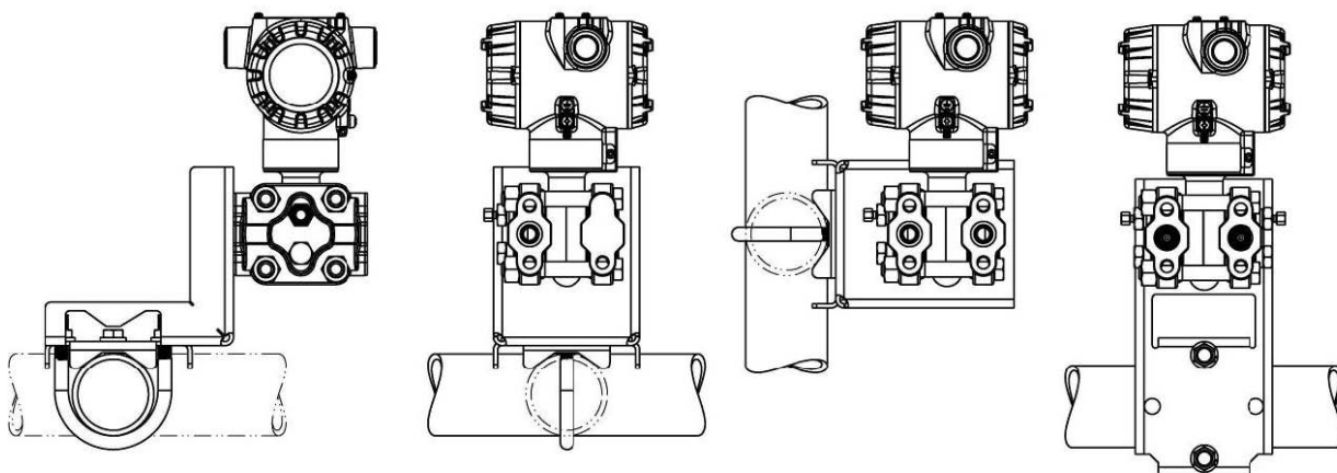
图4 - 安装配置
