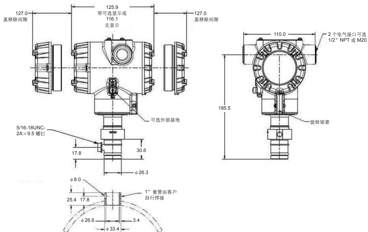
图 3 STG73P / STG73SP 典型安装尺寸图
