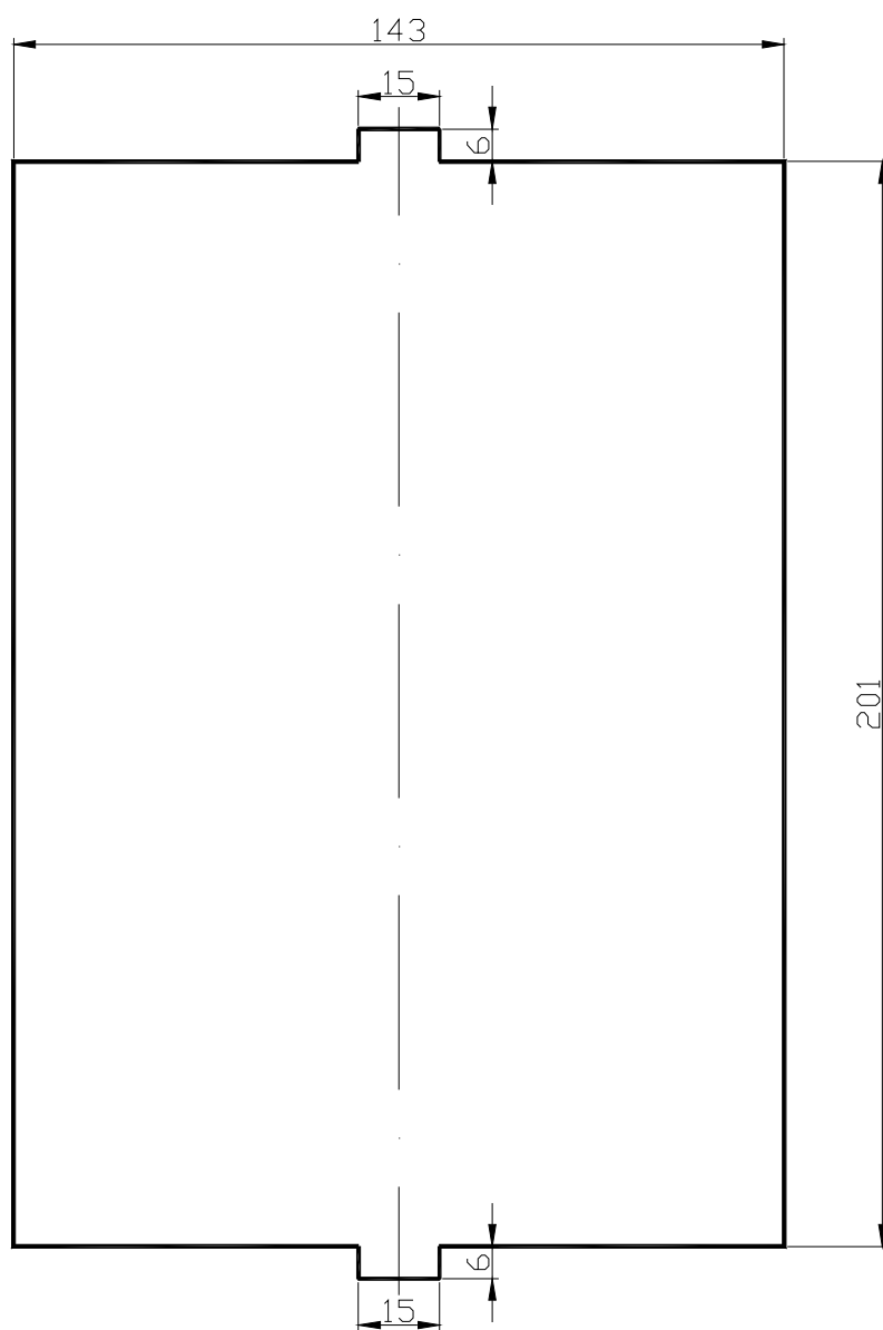
PS690U系列保护装置机箱开孔尺寸图 (单位mm)
