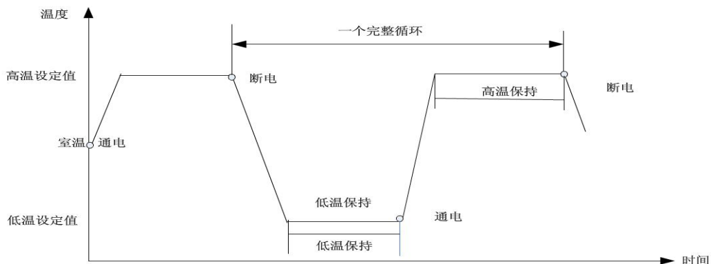
循环测试流程图
