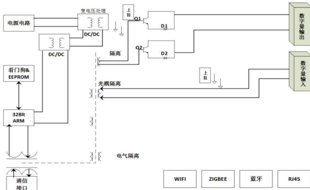
原理框图
