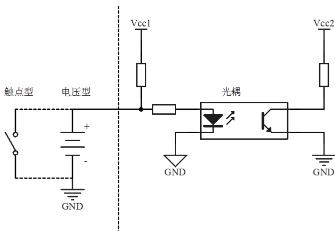
数字量输入原理示意图
