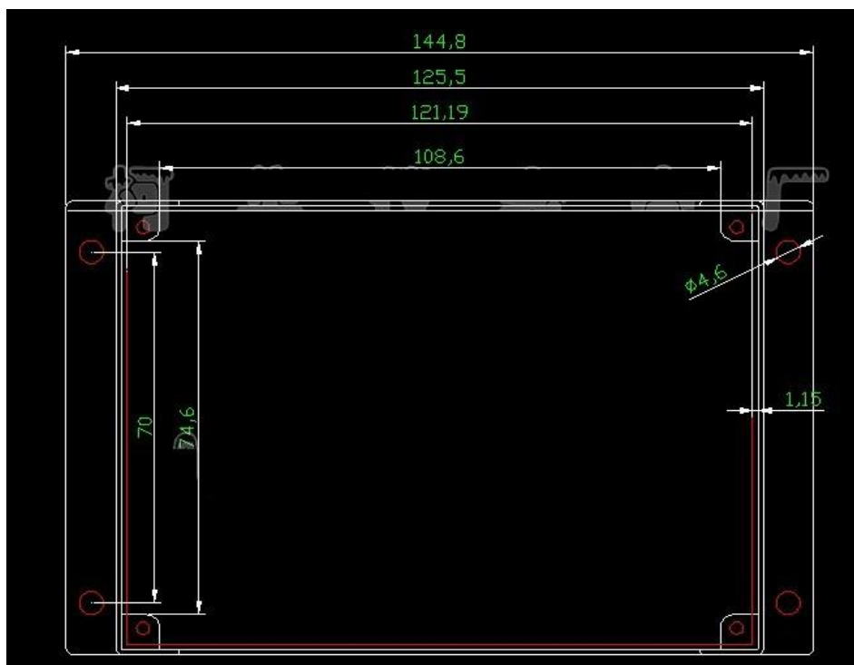
外壳机械尺寸示意图
