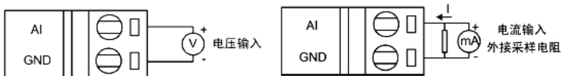
模拟量单端输入接线方式图
