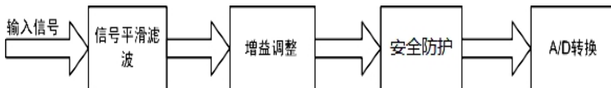
模拟量输入采样前端调理电路图
