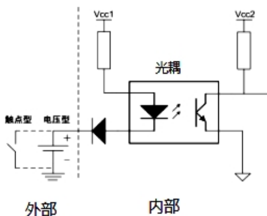
数字量输入原理示意图
