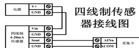
电流传感器接线图
