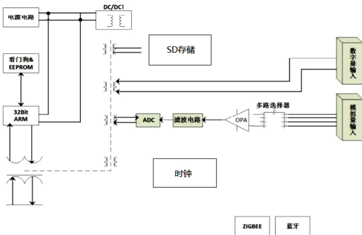
原理框图
