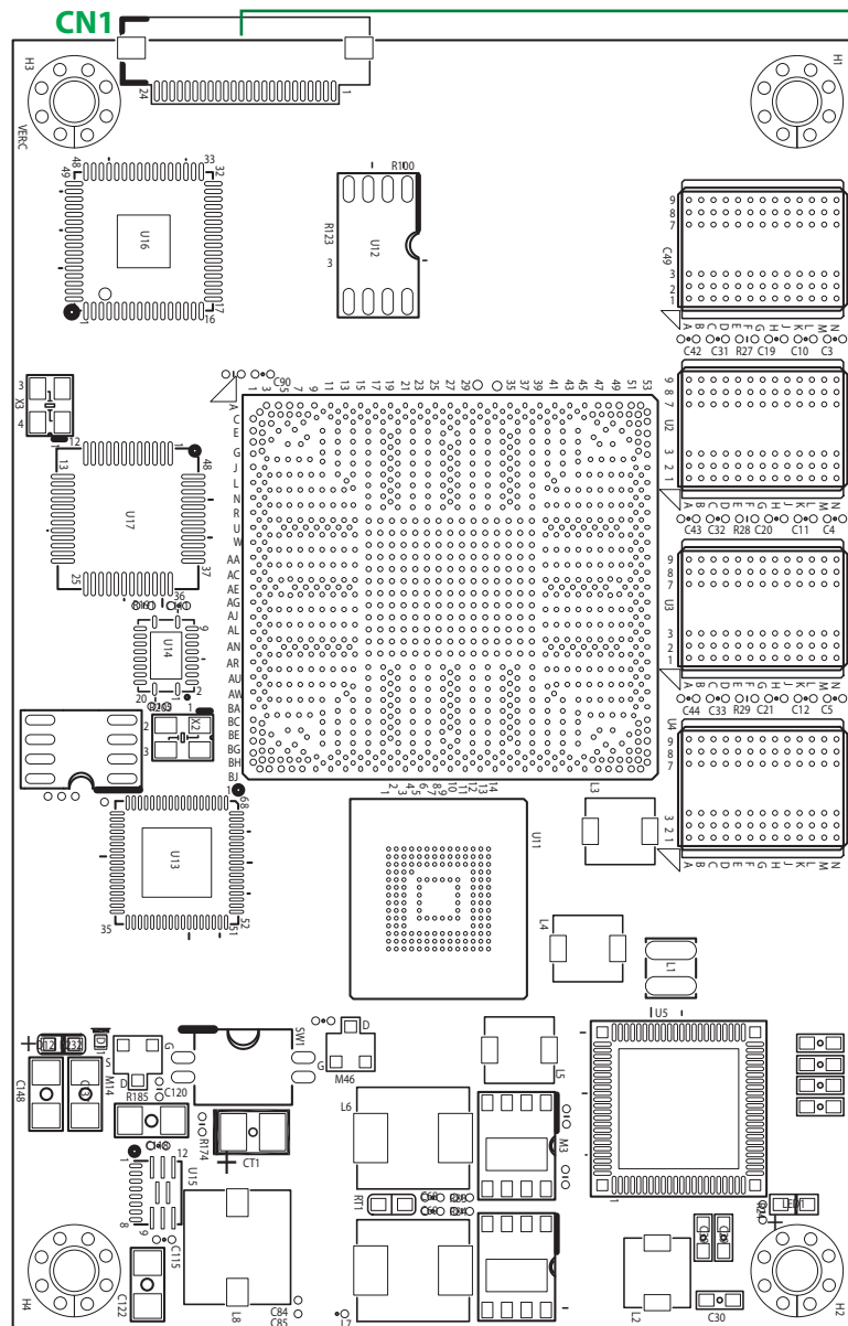
• CN1: EC JTAG
