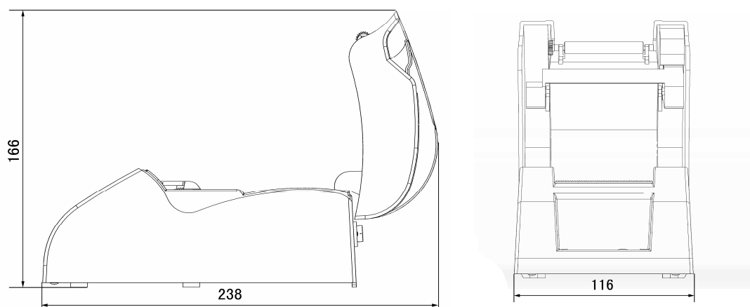
图 4.2-1 结构空间图
