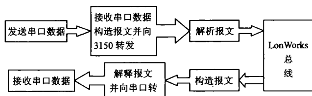
图3 适配器工作原理
