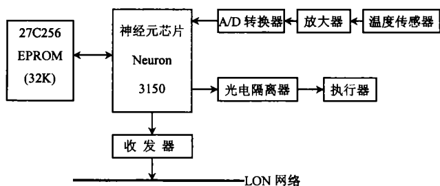
图 2 硬件框图
