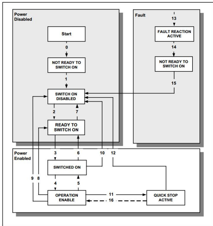
驱动器状态机
