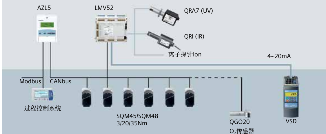
LMV5...电子空/燃比例控制系统
