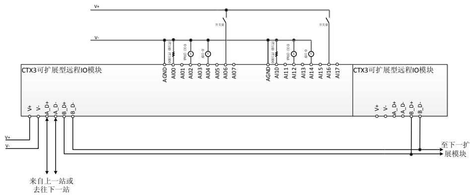
端子定义
