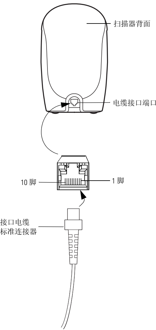
图 3-1 扫描器电缆引线
