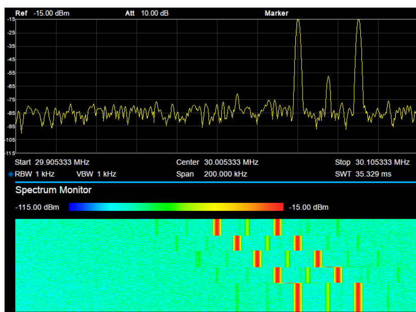
图 2-19 频谱监测
