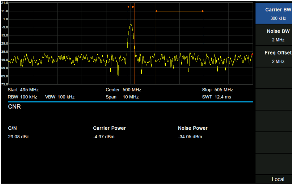
图 2-20 载噪比
