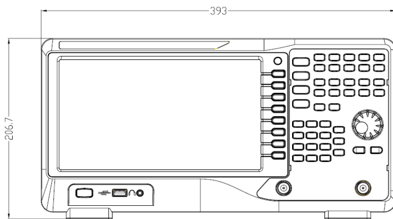
图 1-1 正视图
