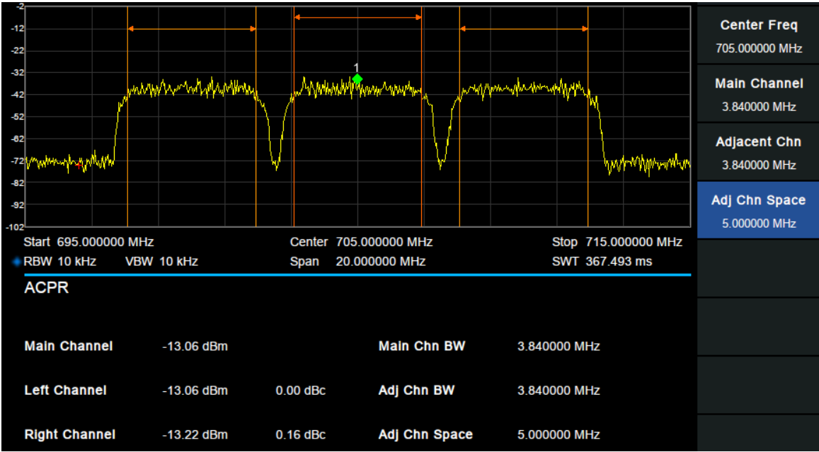
图 2-15 邻道功率比
