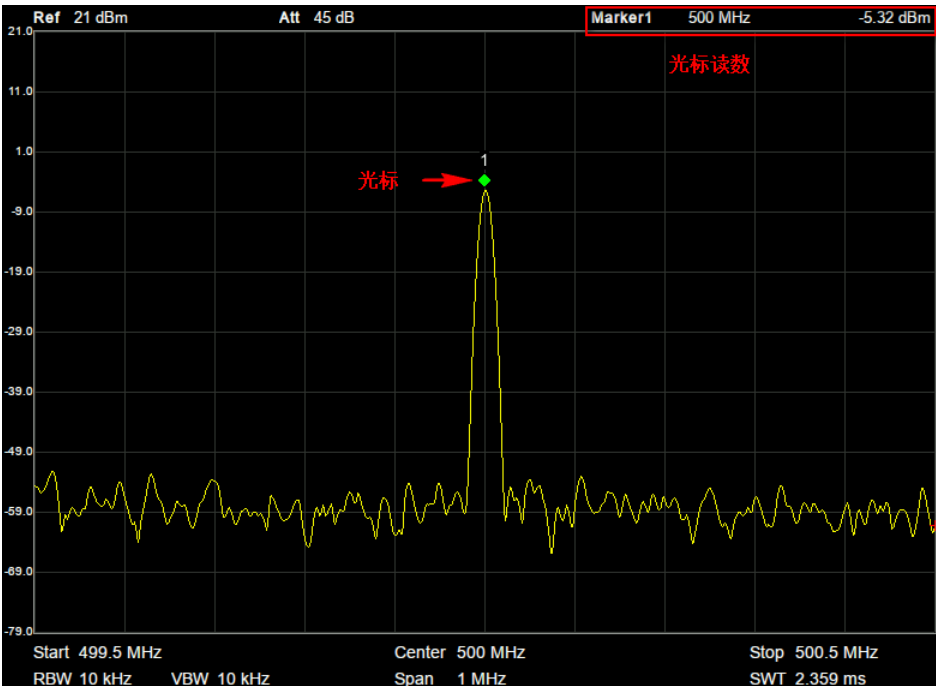
图 2-10 光标示意图
