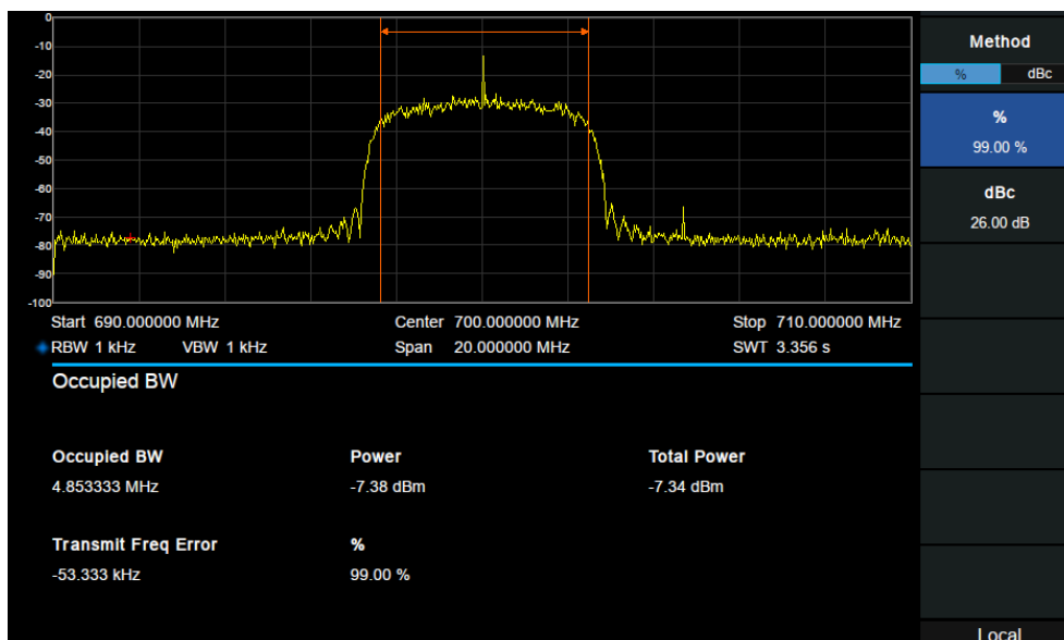
图 2-16 占用带宽
