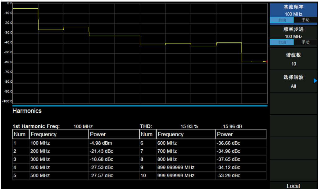
图 2-21 谐波分析
