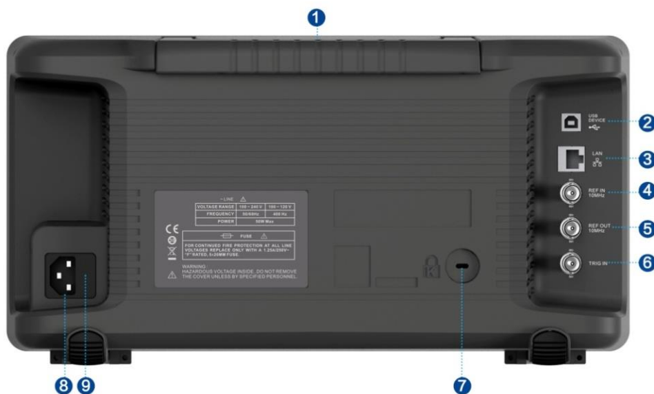
图 1-11 后面板
