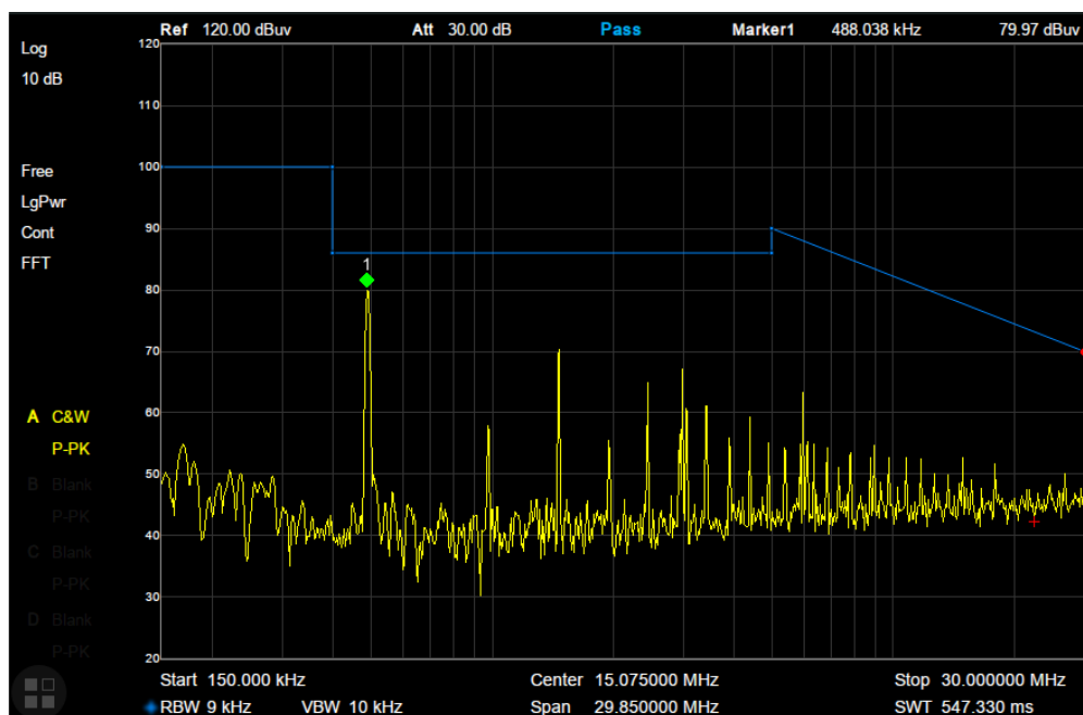
图 2-4 对数轴
