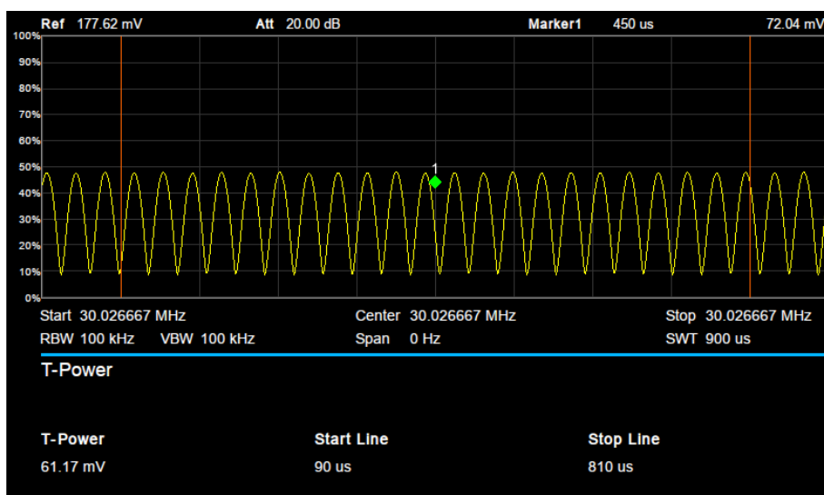
图 2-17 时域功率
