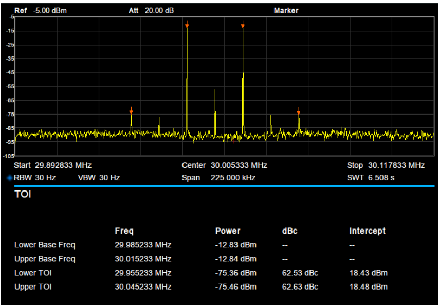
图 2-18 三阶交调
