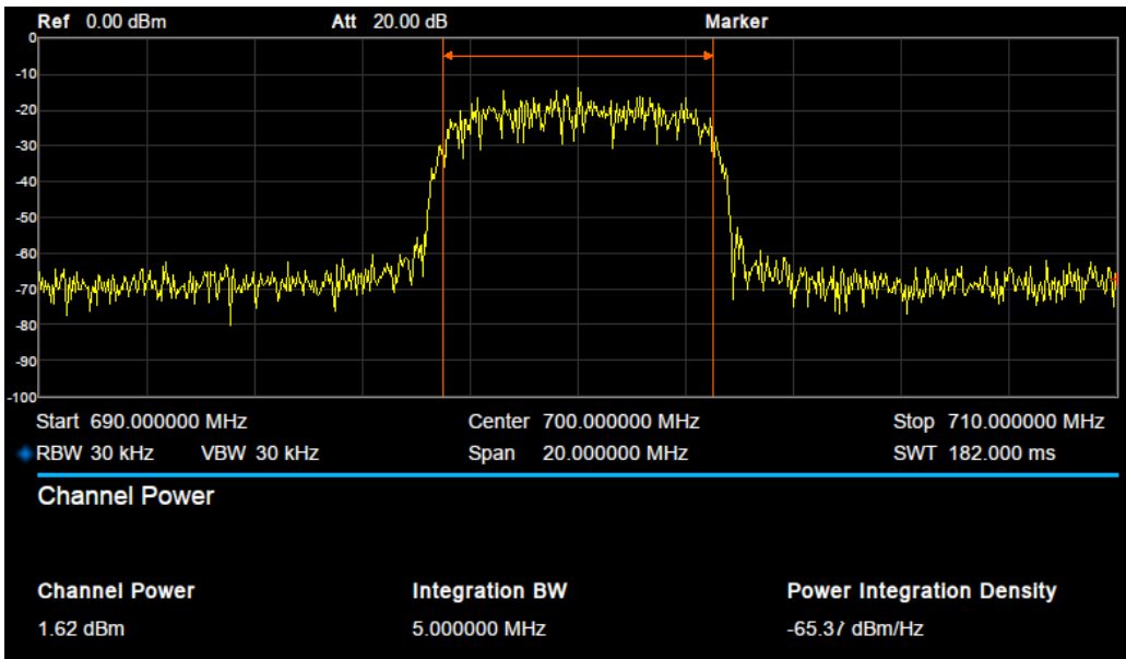
图 2-14 信道功率
