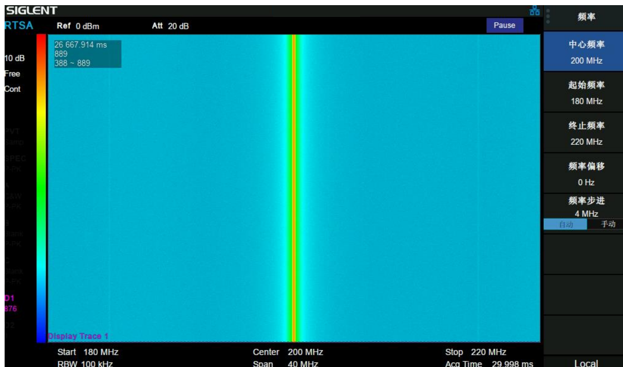
图 6-3 波谱图
