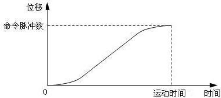
图2-6位移曲线
