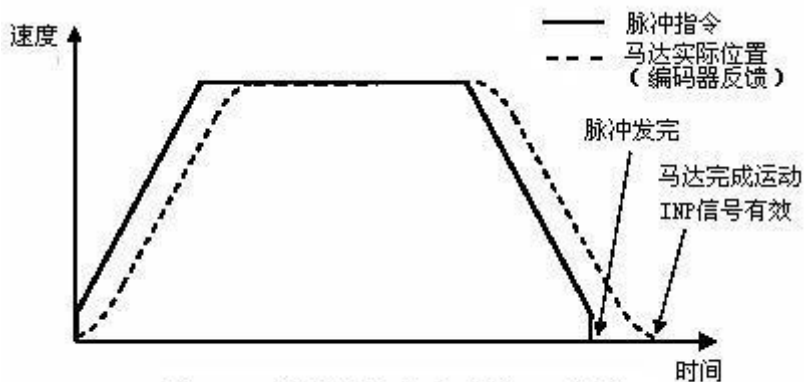
图2-21 伺服定位完成时的INP信号
