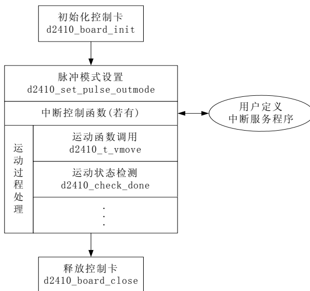
图 7-2 控制软件的典型流程
