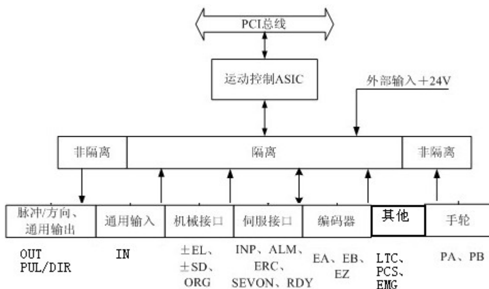
图2-2 DMC-2410B运动控制卡系统框图
