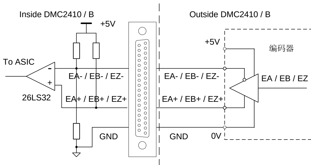
图2-25 差分输出编码器接线原理图
