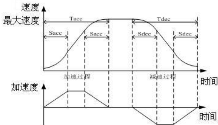
图2-9 S形速度曲线及其加速度曲线
