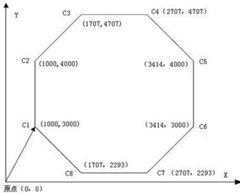
图4-21 DMC2410 两轴连续插补示例
