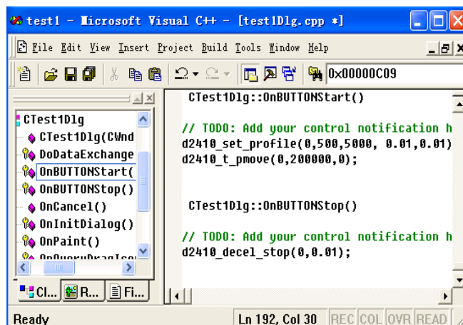
图 7-12 程序中调用运动控制卡库函数
