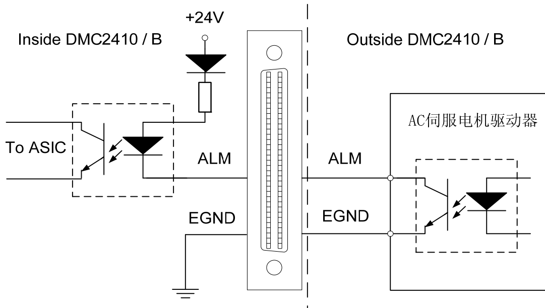
图2-22 ALM信号接线原理图
