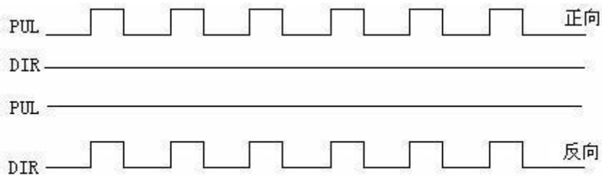
图2-14 双脉冲模式
