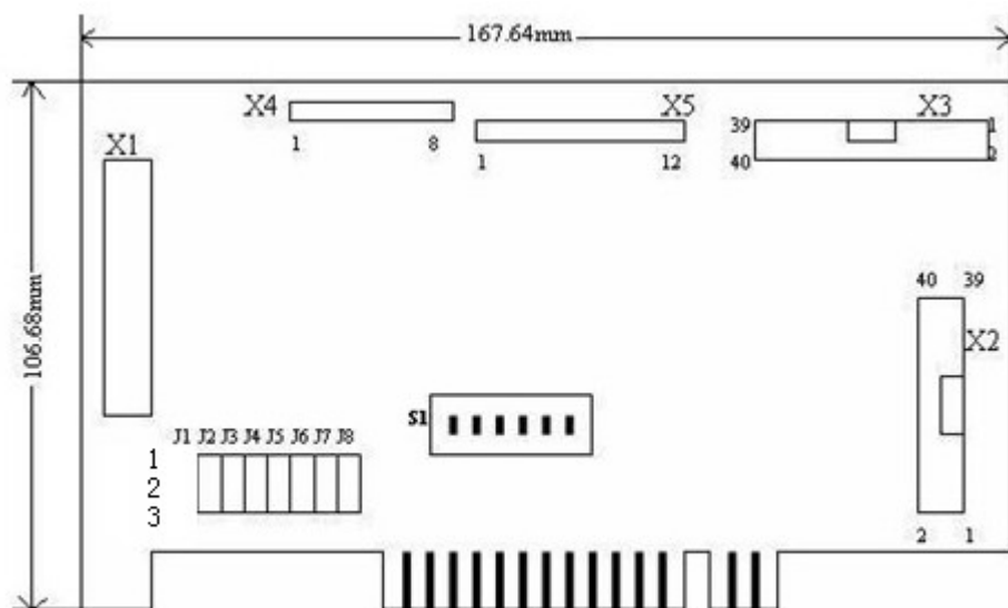
图2-3 DMC2410 运动控制卡结构尺寸图
