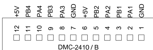
图 8-5 接口 X5 示例
