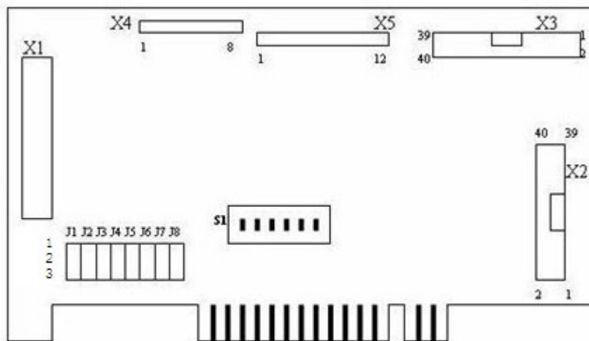
图3-1 DMC2410 板卡跳线、开关布局
