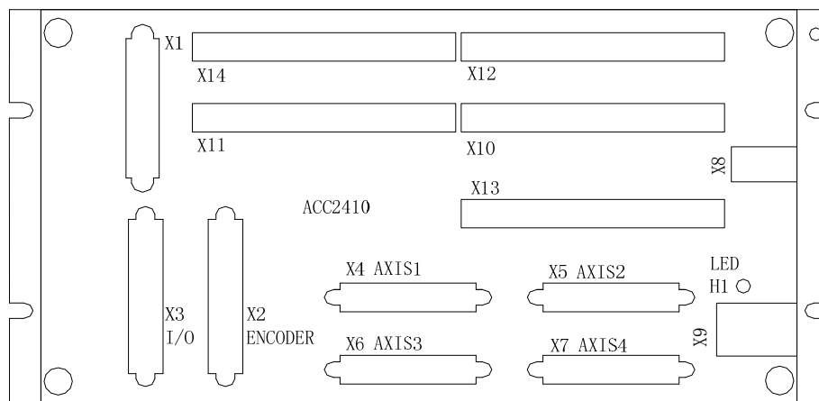
图 8-6 ACC2410 接线板示意图
