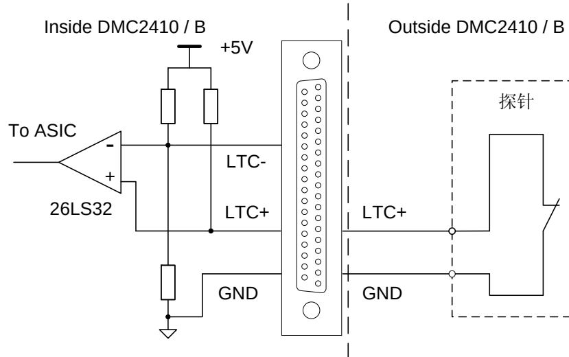
图2-27 位置锁存输入信号接口原理图
