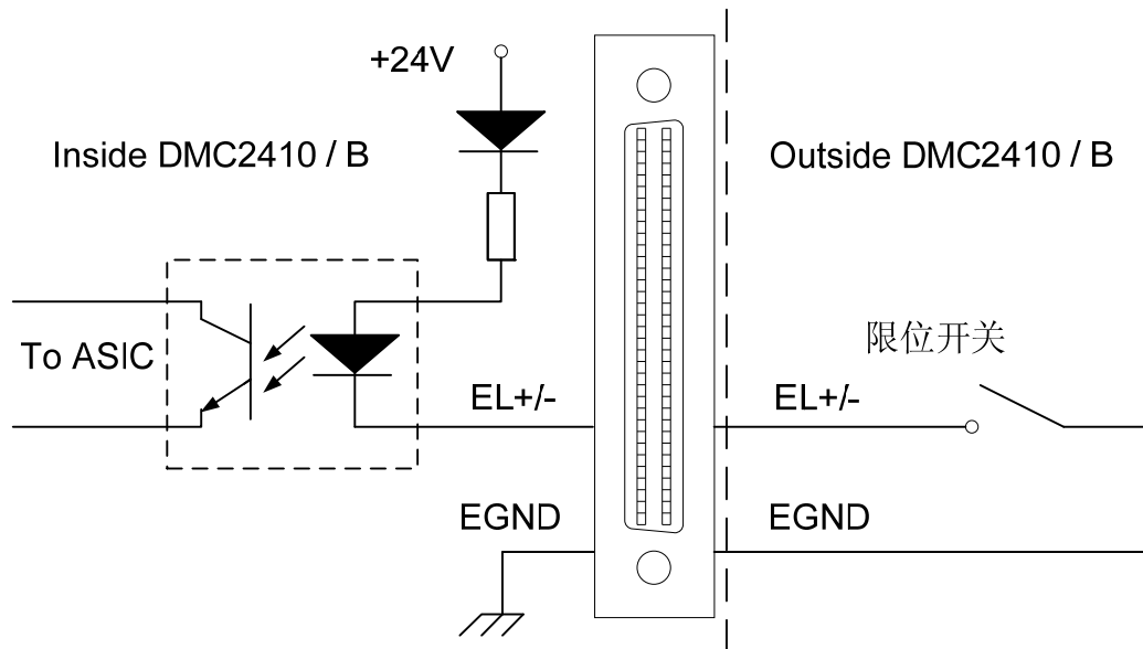
图2-17 限位信号接口原理图
