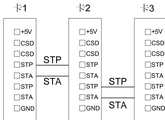
图2-34 多卡同时启停的连接方式
