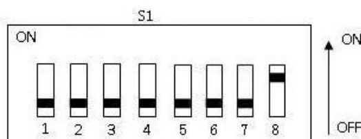
图3-6 DMC-2410的拨码开关设置示意图
