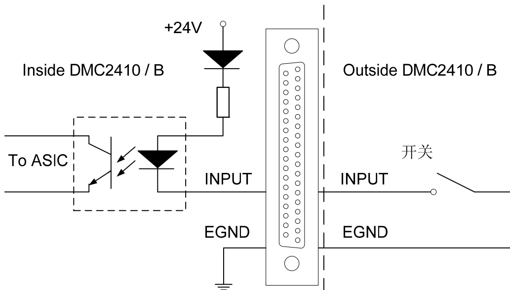
图2-30 INPUT 信号输入原理图
