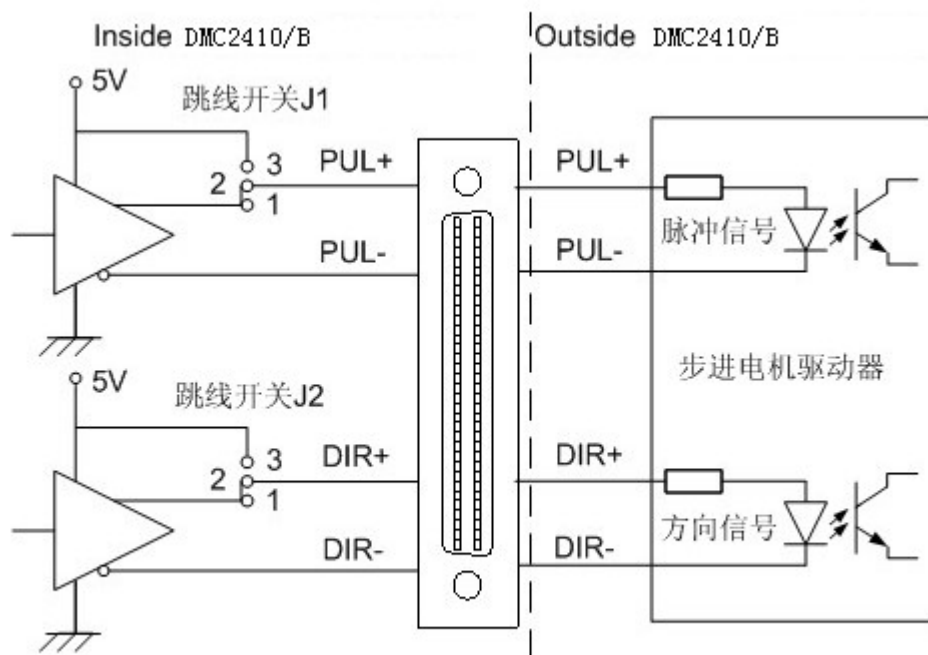
图 2-11 差分方式接线图
