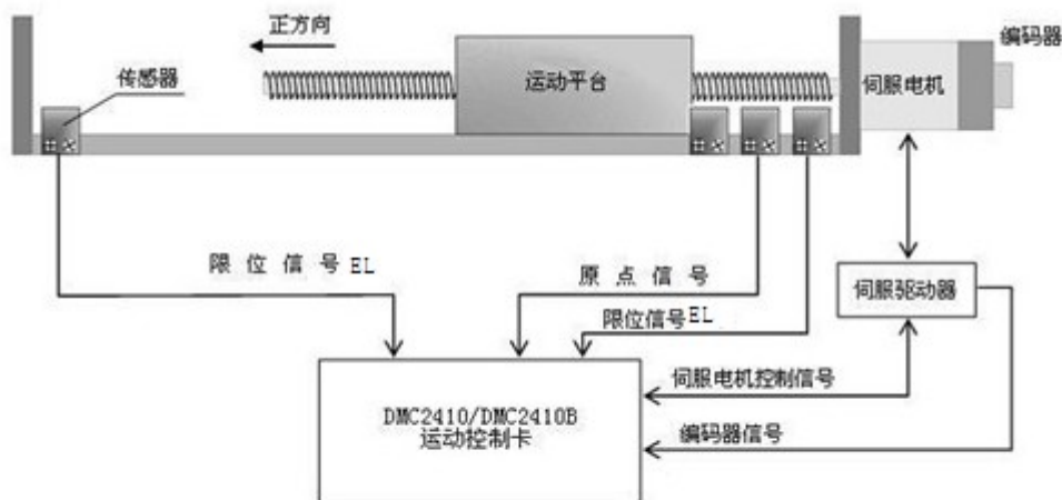
图 2-35 运动平台位置传感器及控制信号的布置图
