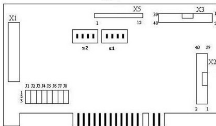
图3-2 DMC2410B 板卡跳线、开关布局
