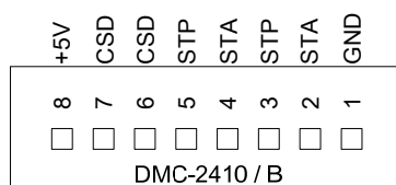
图 8-4 接口 X4 示例
