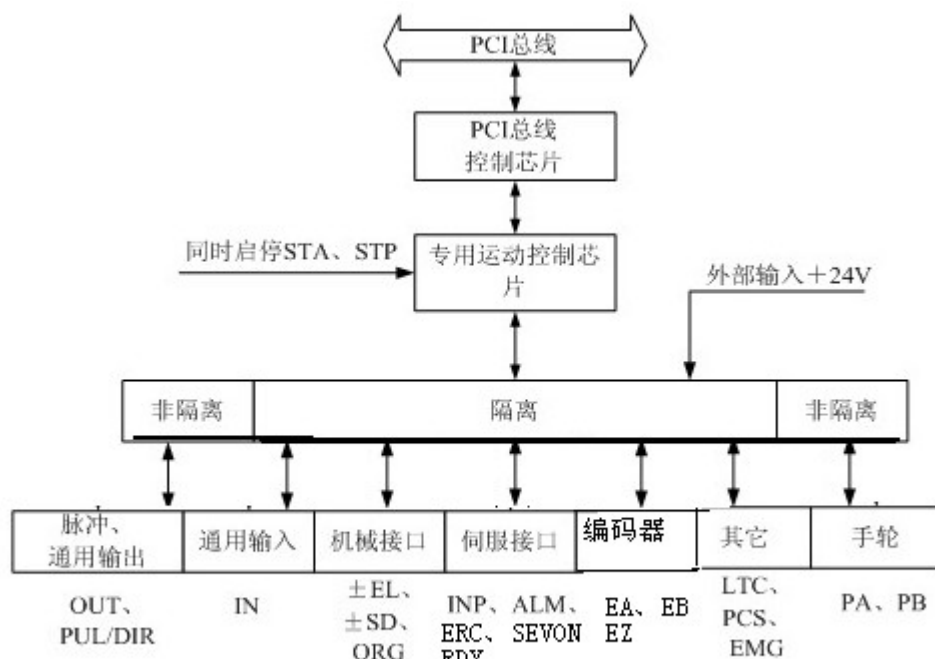
图2-1 DMC-2410运动控制卡系统框图
