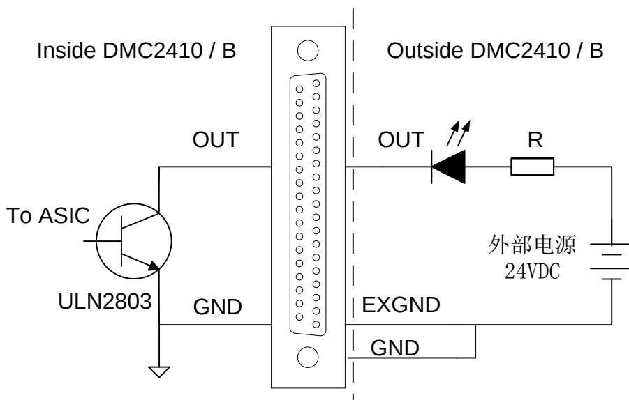
图2-31 输出口接发光二极管原理图
