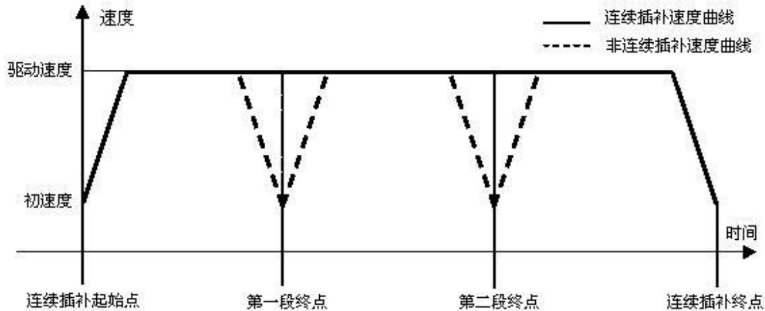
图4-19 连续插补运动
