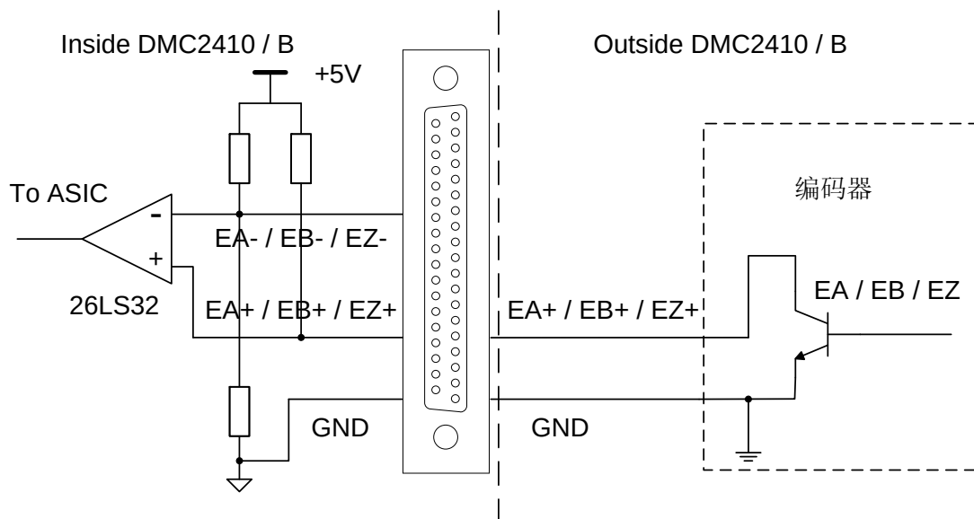
图2-26 集电极开路输出的编码器接线原理图
