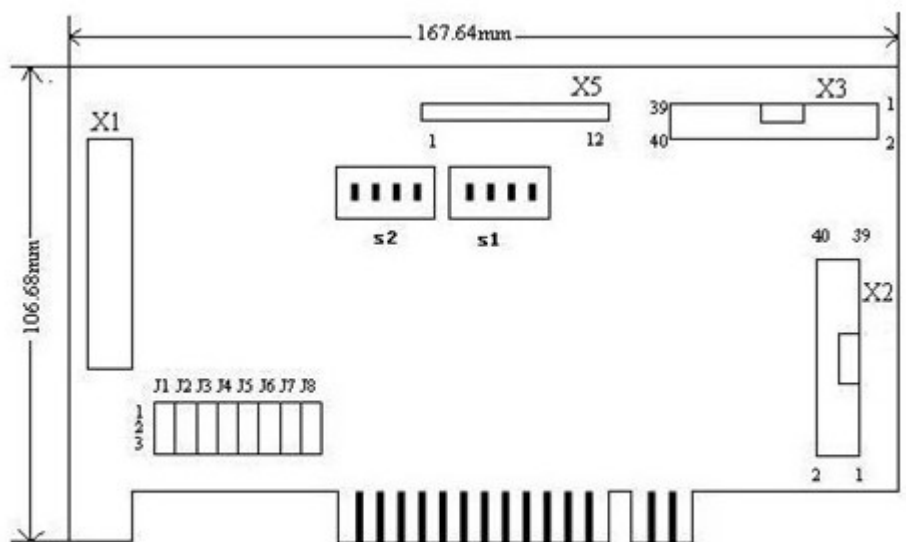
图2-4 DMC2410B 运动控制卡结构尺寸图
