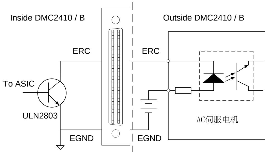
图2-23 ERC信号接线原理图
