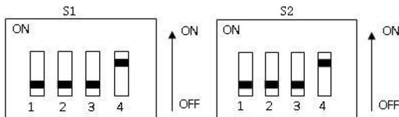
图3-5 DMC-2410B的拨码开关设置示意图
