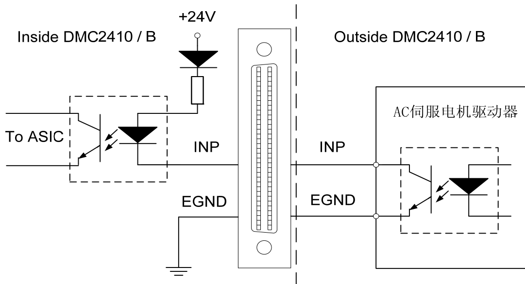
图2-20 INP信号接线原理图
