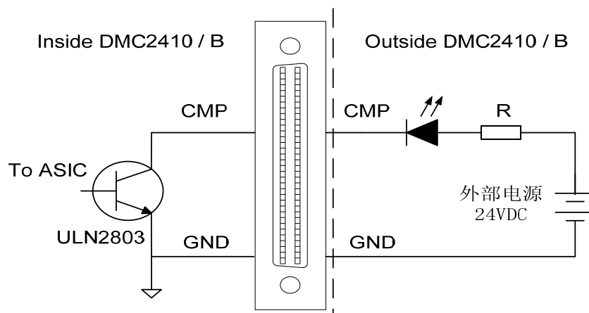
图2-28 位置比较输出信号原理图
