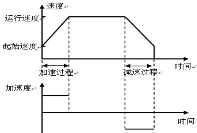
图 2-8 梯形速度曲线及加速度曲线
