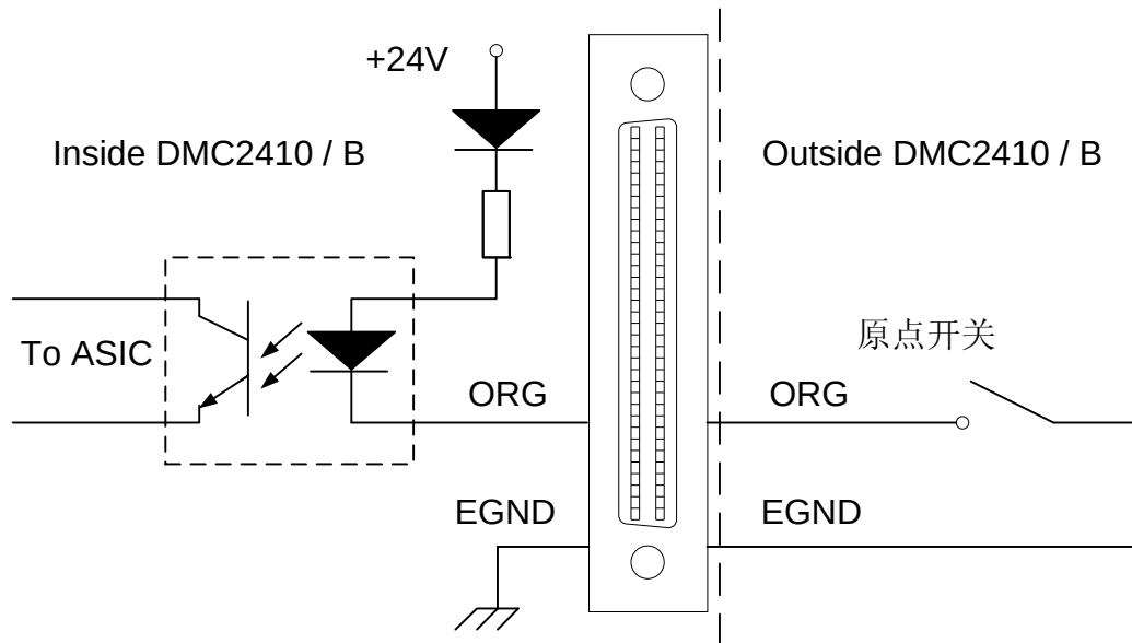
图2-15 原点信号接口原理图
