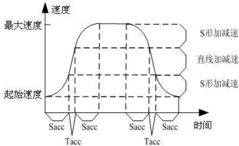
图2-10 S形速度曲线
