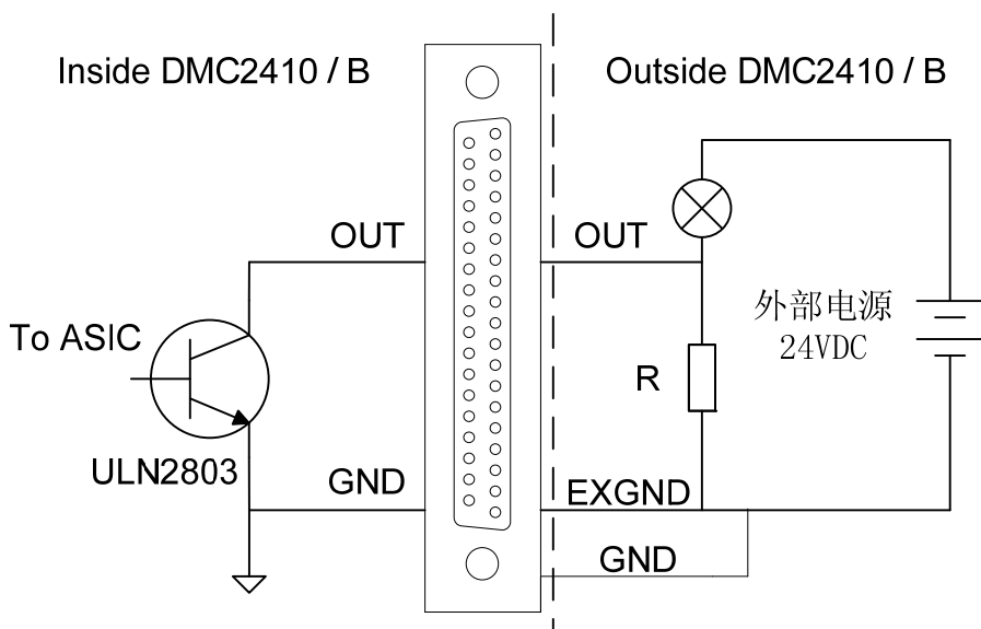
图2-32 输出口接指示灯原理图
