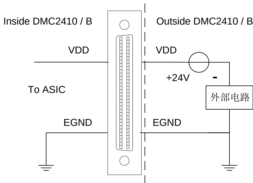
图2-5 板卡供电
