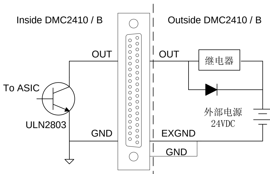
图2-33 接小型继电器原理图
