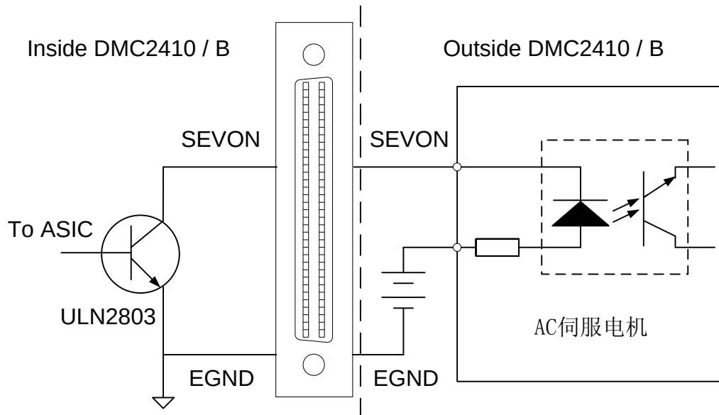
图2-18 SEVON信号接线原理图
