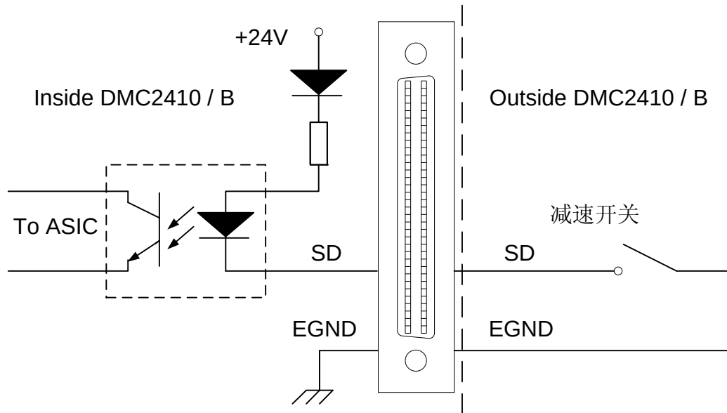
图2-16 减速信号接口原理图
