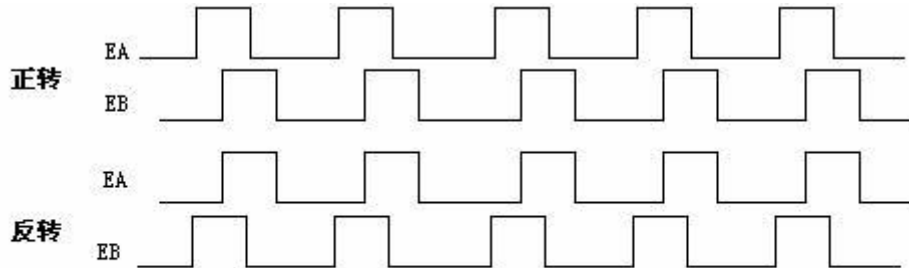
图2-24 正反转A/B相正交信号
