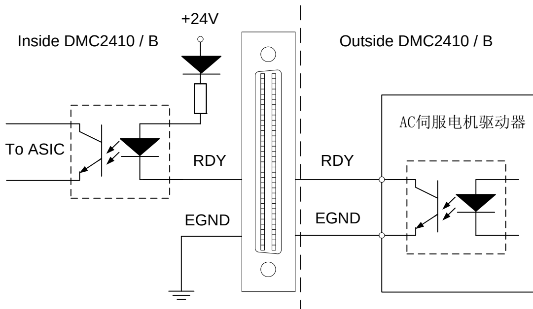
图2-19 RDY信号接线原理图
