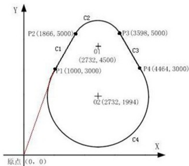
图4-22 DMC2410B 两轴连续插补示例
