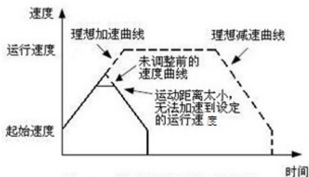
图4-10 运动距离小于加速距离
