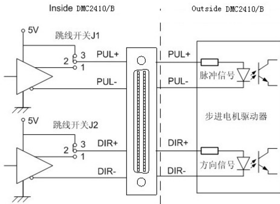
图 2-12 单端输出方式接线图
