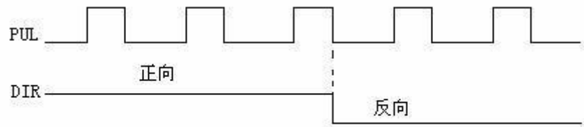
图2-13 单脉冲模式
