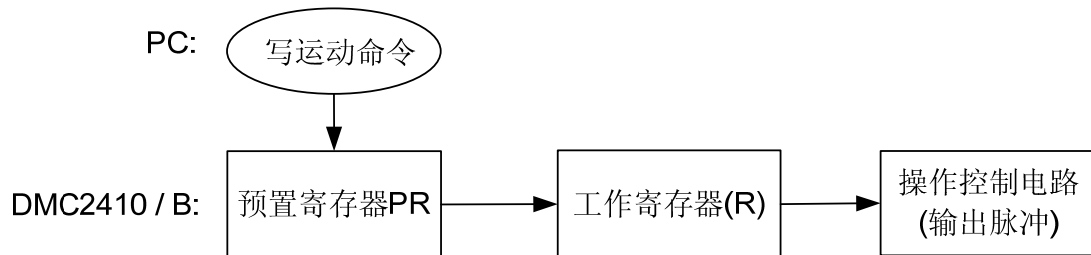
图4-20 DMC-2410双缓冲寄存器连续插补的工作原理
