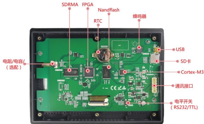
图 1-3 硬件配置图
