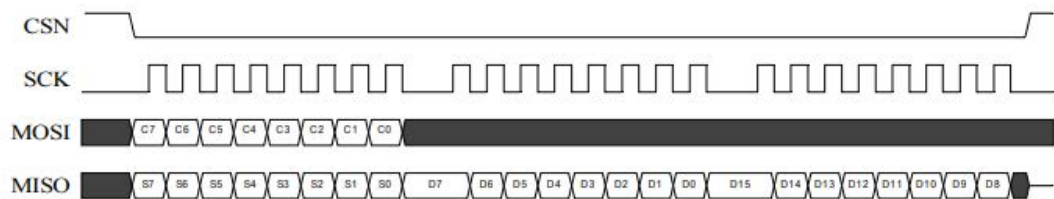
图 5-5 SPI 写操作
