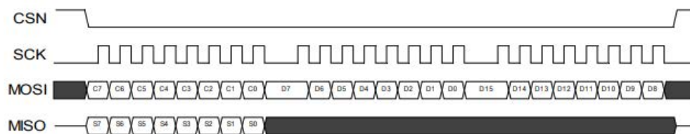
图 5-6 SPI 读操作
