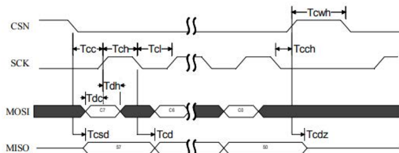
图 5-7 SPI 典型时序
