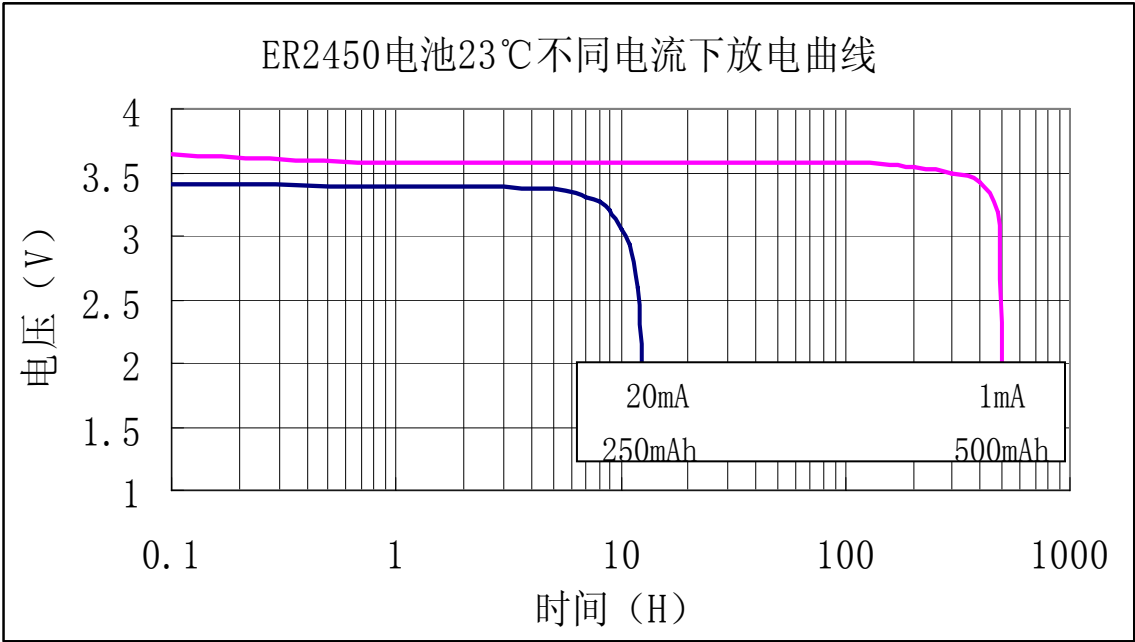
附图 1. 电池放电曲线
