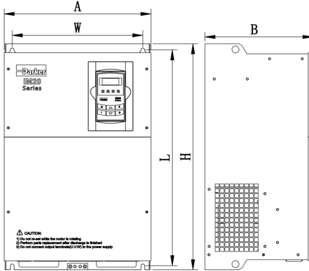
图 3-1 驱动器安装尺寸图
