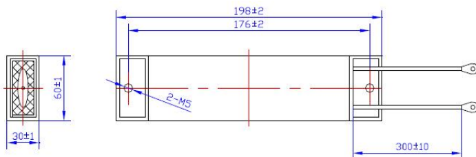
图 3-4 制动电阻尺寸图(铝合金电阻)
