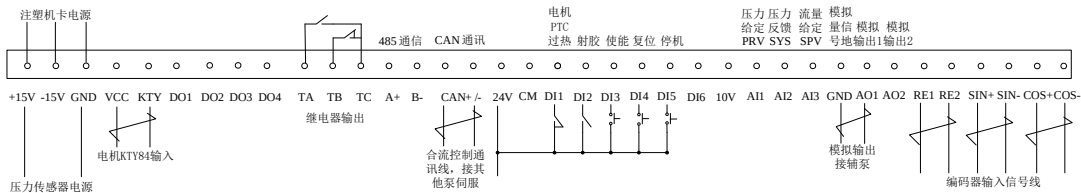
主泵伺服接线示意图
