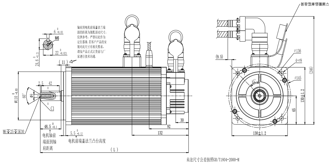
附图 2 7(130 法兰)机座伺服电机结构尺寸图
