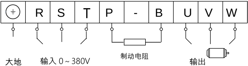
图 4-3 主电路接线示意图
