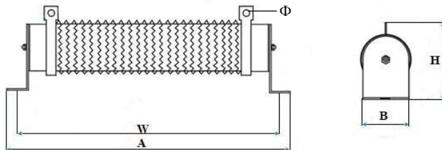
图 3-5 制动电阻尺寸图(无感波纹瓷管电阻)
