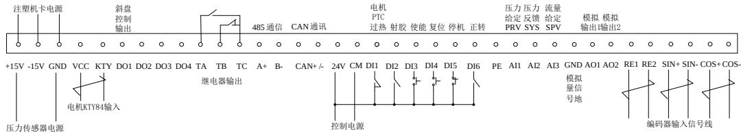
图 4-4 驱动器单泵控制示意图
