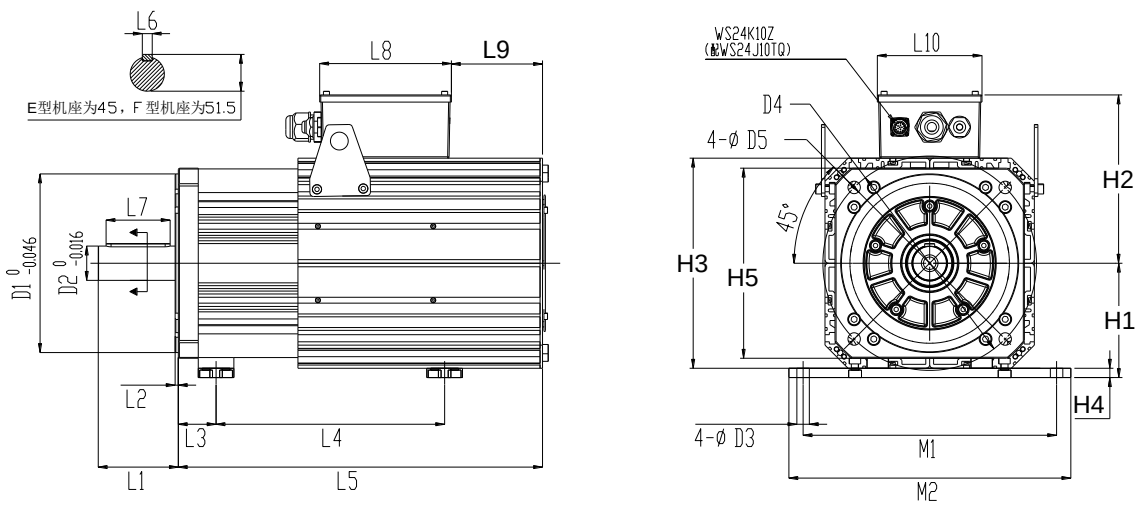
附图 4 E、F 机座伺服电机结构尺寸图(mm) (设计代码 L)
