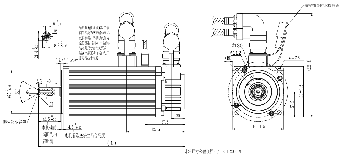
附图1 5(110 法兰)机座伺服电机结构尺寸
