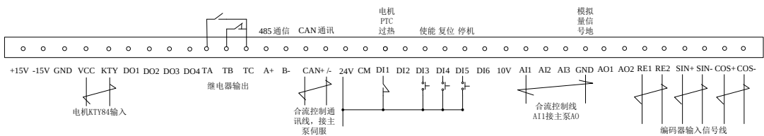
辅泵伺服接线示意图
