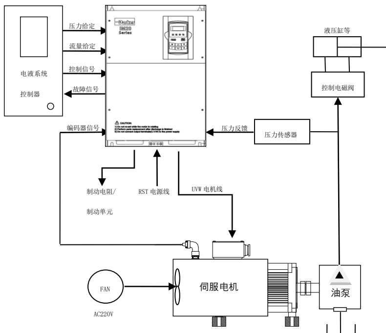
图 4-1 电液系统构成示意图
