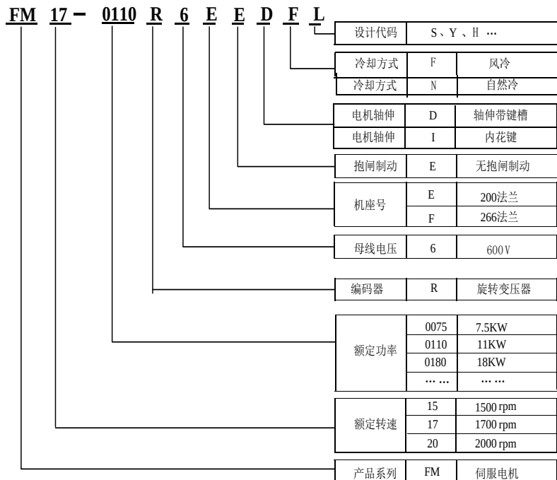
图 1.5.2 伺服电机的命名规则（7.5KW 及以上电机）
