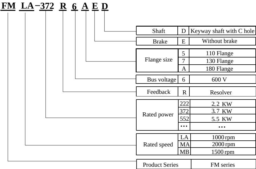
图 1.5.1 伺服电机的命名规则（5.5KW 及以下电机）
