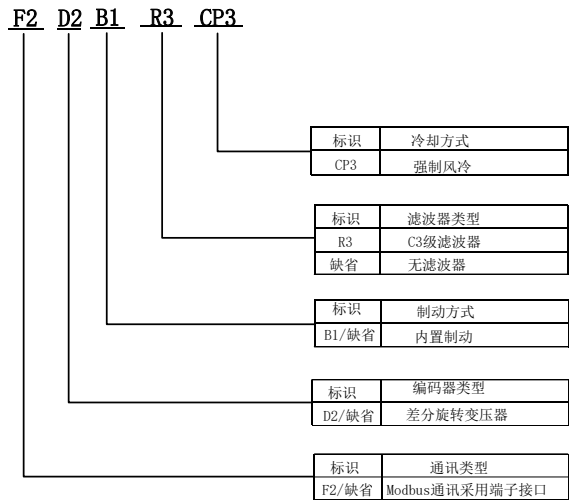
图 1.4.2 伺服驱动器功能部分命名规则
