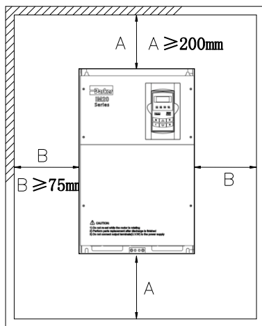
图 3-2 驱动器安装示意
