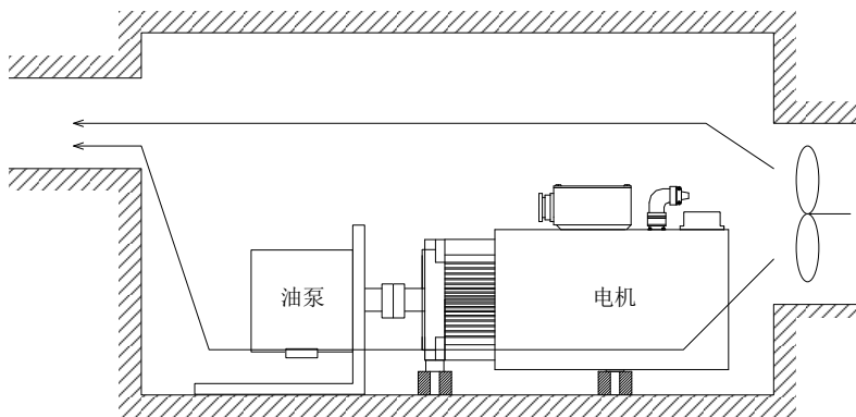
图 3-3 正确的安装方式
