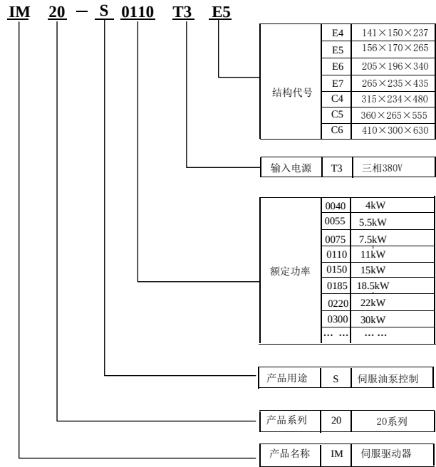
图 1.4.1 伺服驱动器命名规则
