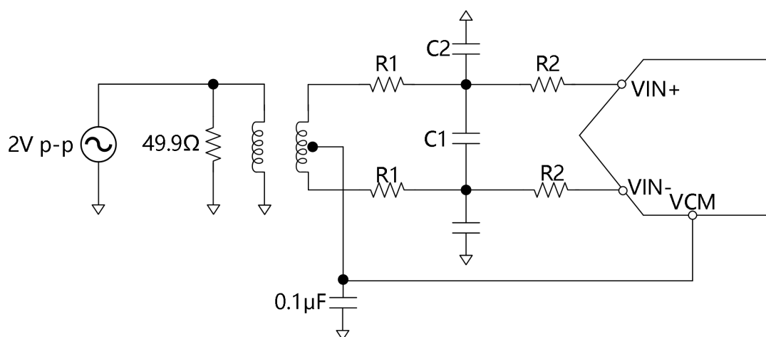
图 14 差分变压器耦合输入配置
