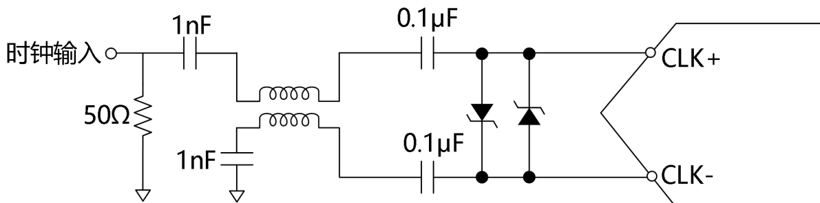
图 19 巴伦配置的时钟
