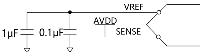
图 17 SENSE 引脚接 AVDD 模式 (VREF 需外)
