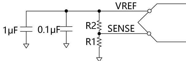
图 16 外接电阻串模式 (VREF 外部配置模式)
