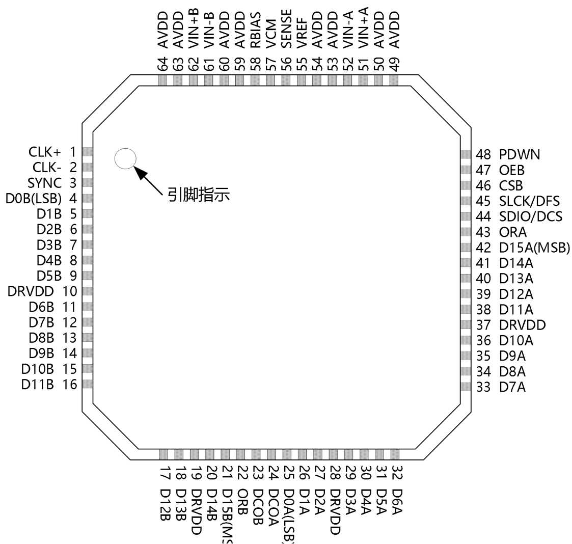
图 3. 并行 CMOS 引脚配置（顶视图）
