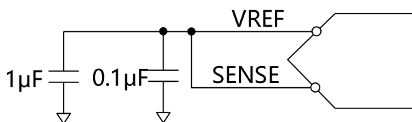
图 15 SENSE 引脚接地模式 (VREF 内部配置模式)
