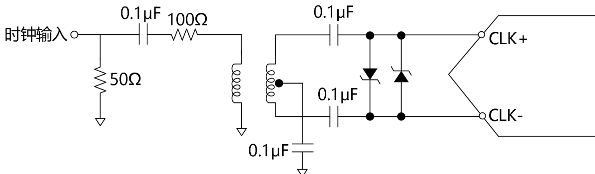
图 18 变压器配置的时钟输入
