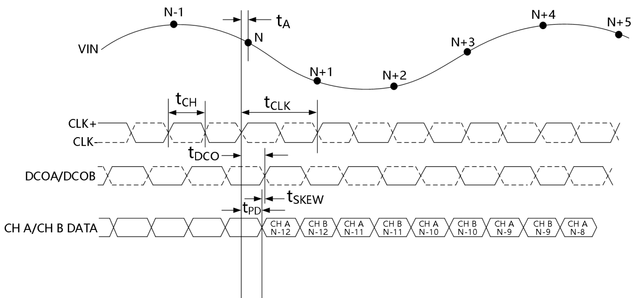
图 2 CMOS 默认输出模式数据输出时序
