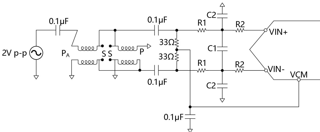
图 15 差分双巴伦耦合输入配置
