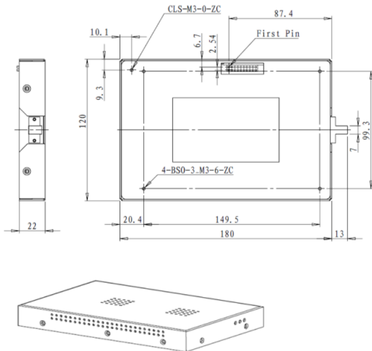
图 2.1 模块尺寸图
