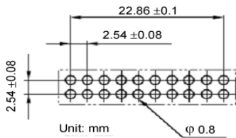
图 2.2 电接口
