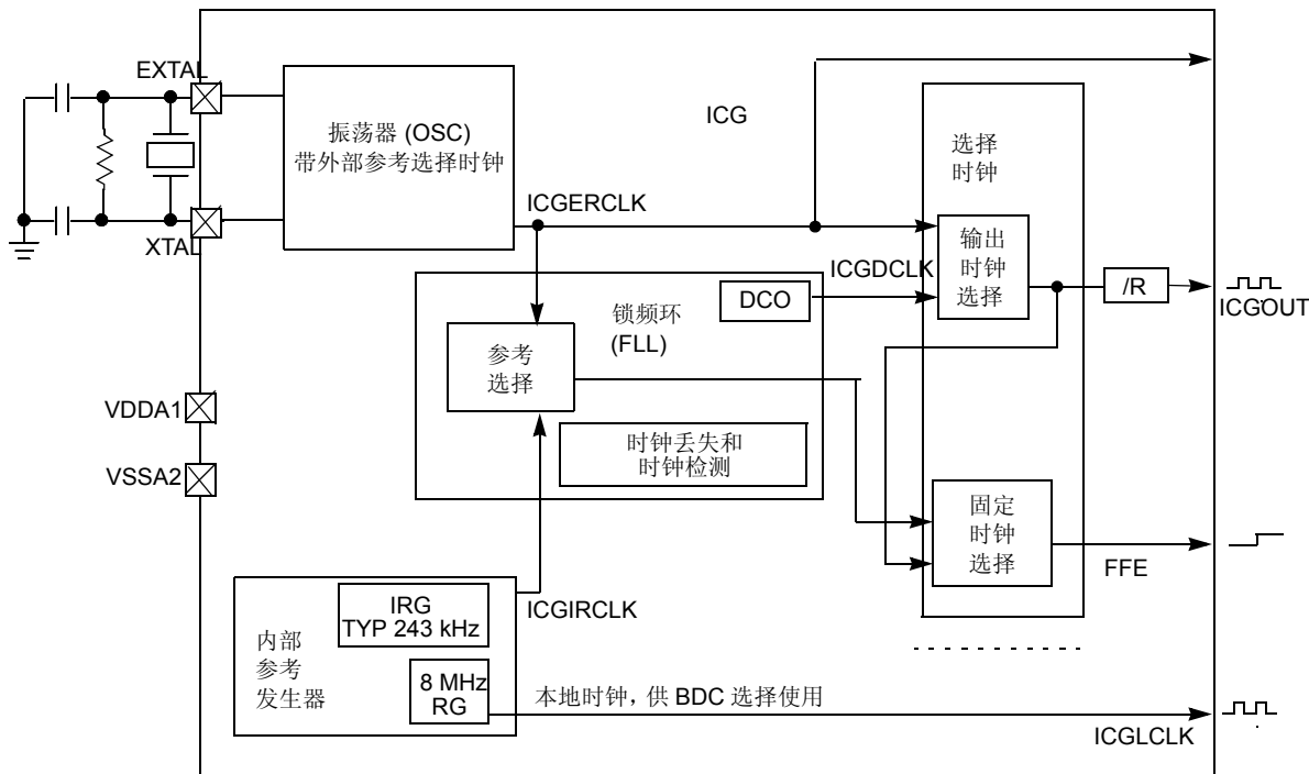
图 8-3. ICG 框图
