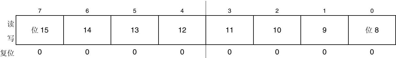
图 12-10. TPM 计数器模寄存器高位 (TPMxMODH)
