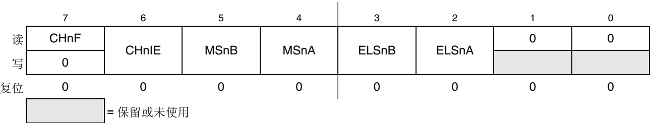
图 12-12. TPM 通道 n 状态和控制寄存器 (TPMxCnSC)
