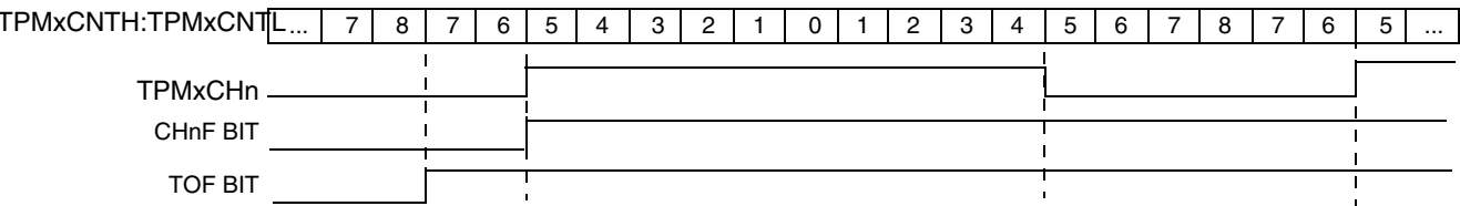
图 12-5. 中心对齐 PWM 模式的高真脉冲
