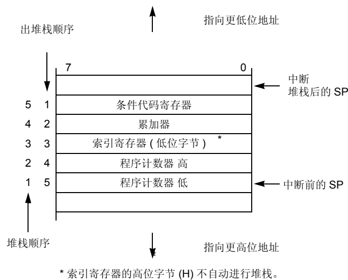
图 5-1. 中断堆栈帧
