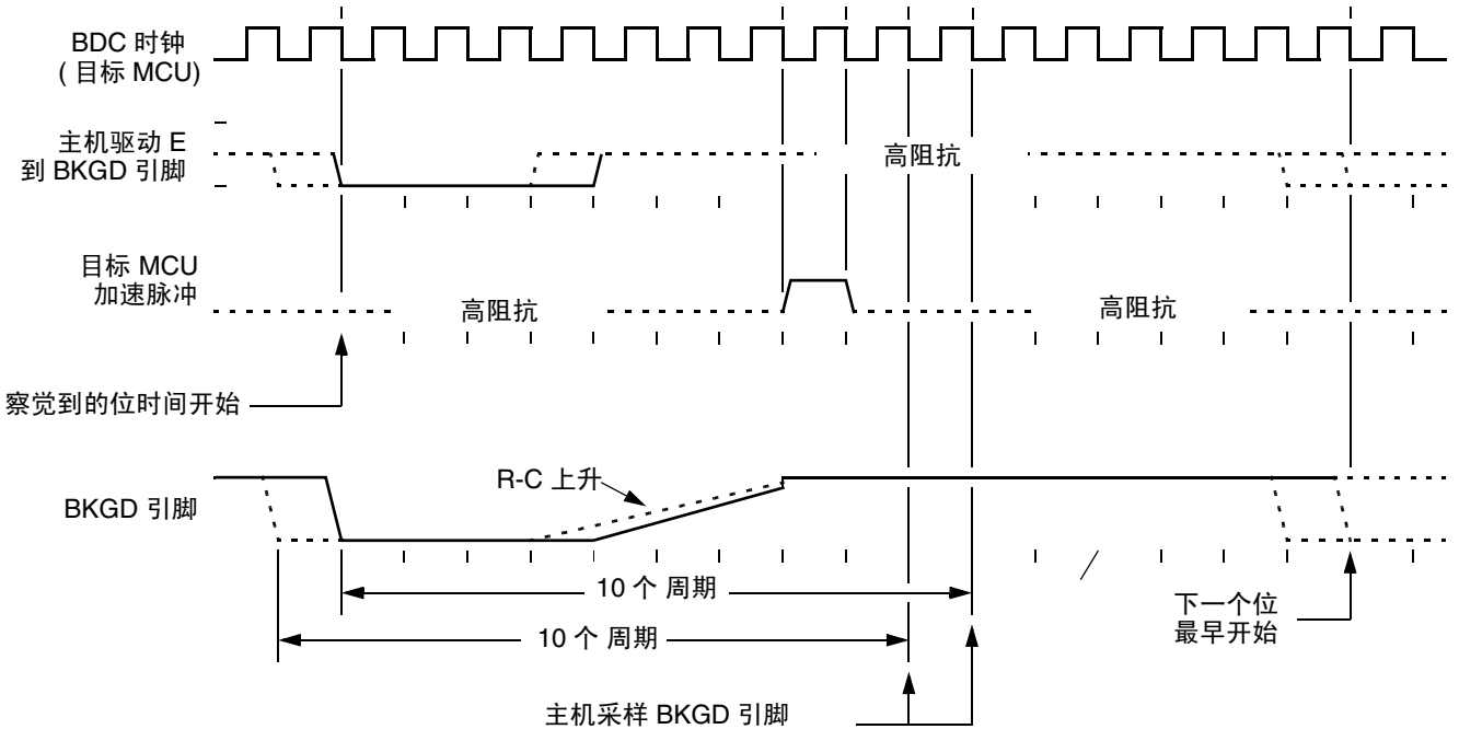
图 13-3. BDC 目标 - 到 - 主机串行位时序 (逻辑 1)
