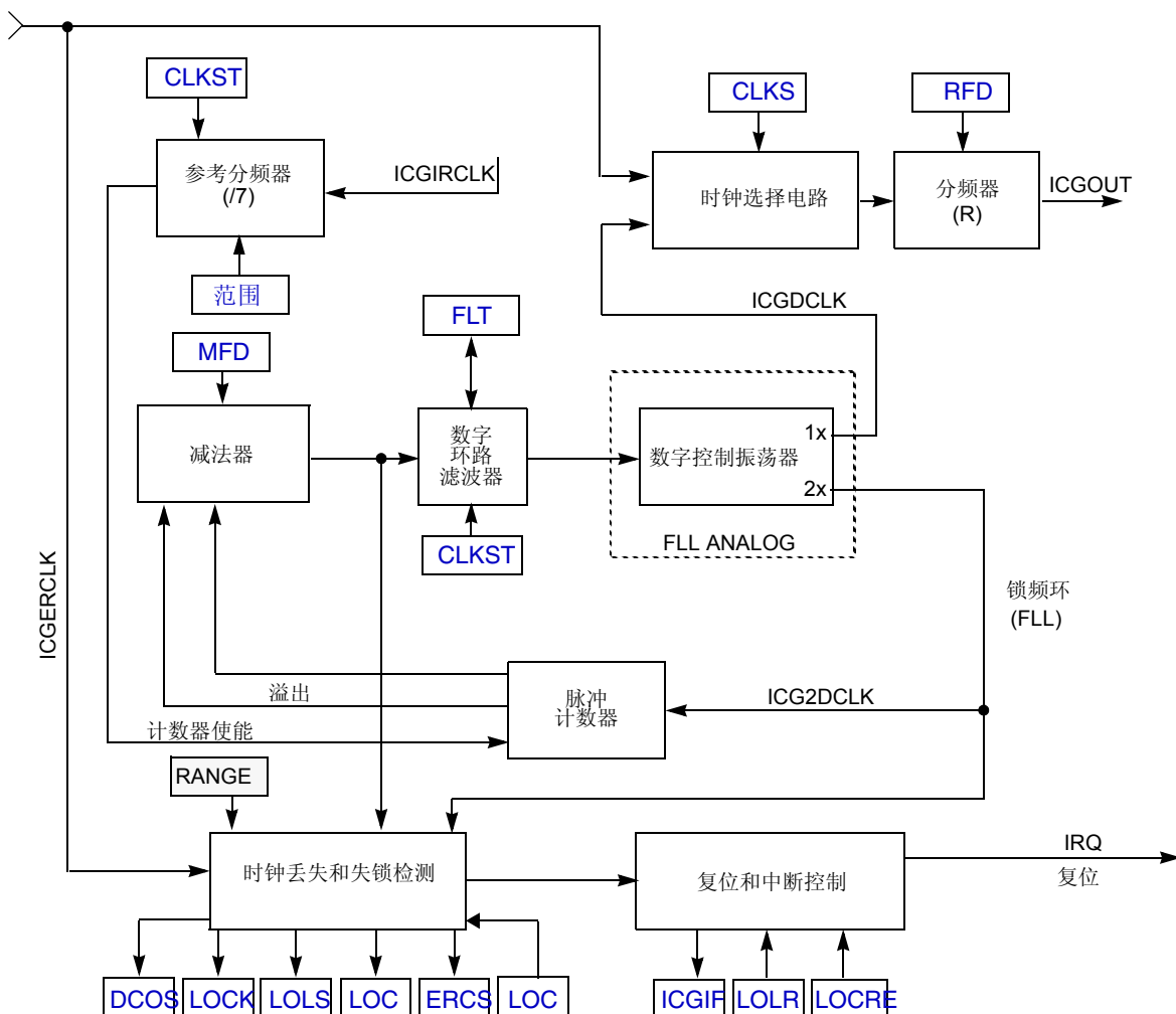
图 8-13. 详细的锁频环框图
