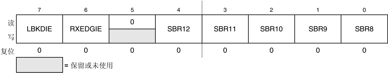
图 10-4. SCI 波特率寄存器（SCIxBDH）
