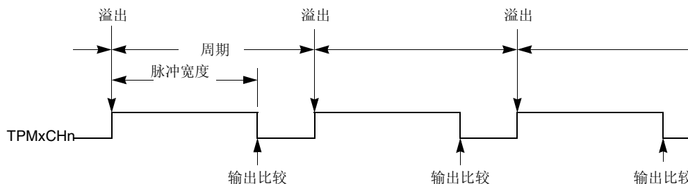
图 12-15. PWM 周期和脉冲宽度 (ELSnA= 0)
