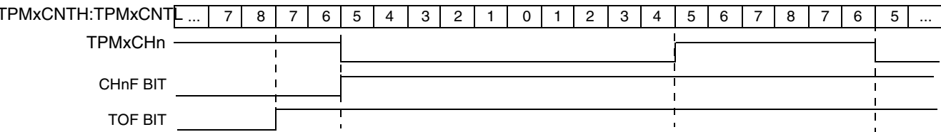
图 12-6. 中心对齐 PWM 模式的低真脉冲
