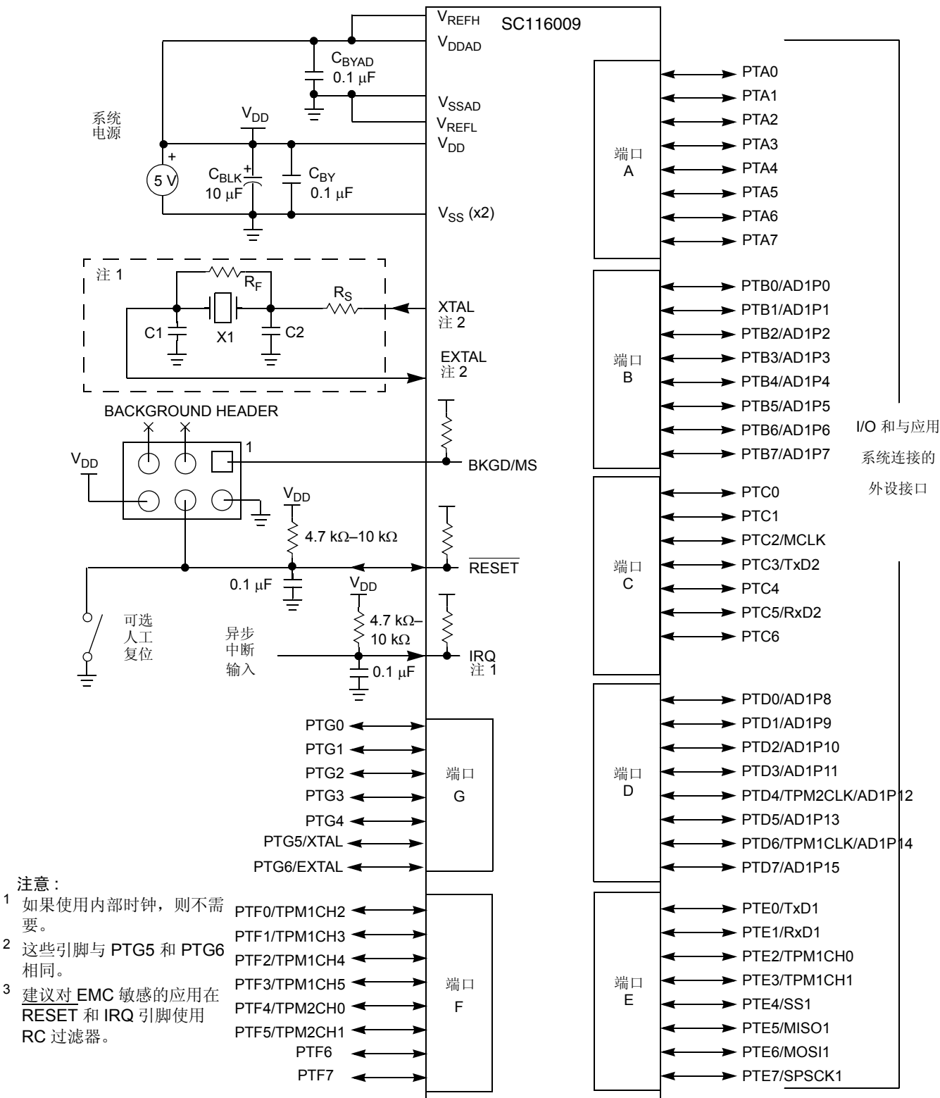
图 2-3. 基本系统连接
