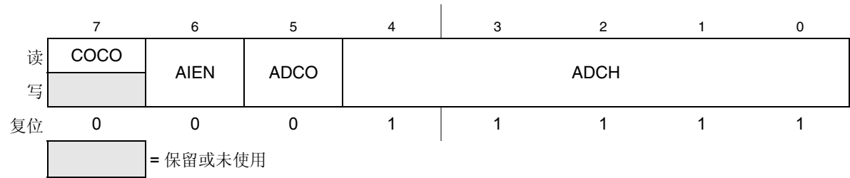
图 9-3. 状态和控制寄存器 (ADCSC1)
