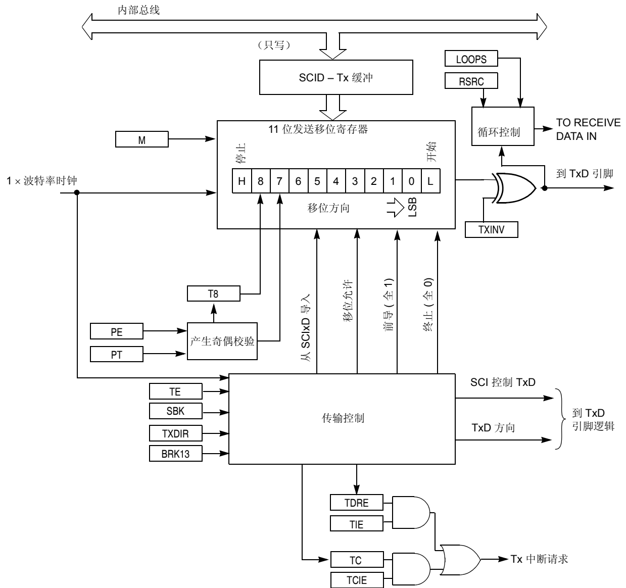
图 10-2. SCI 发送器原理结构图
