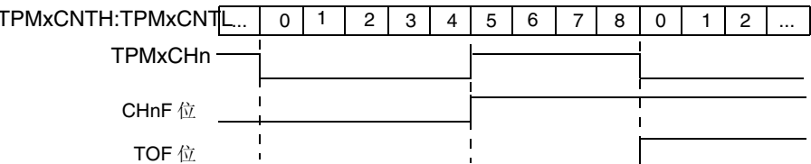
图 12-4. 边缘对齐 PWM 模式的低真脉冲
