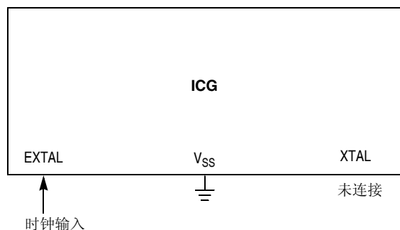
图 8-4. 外部时钟连接
