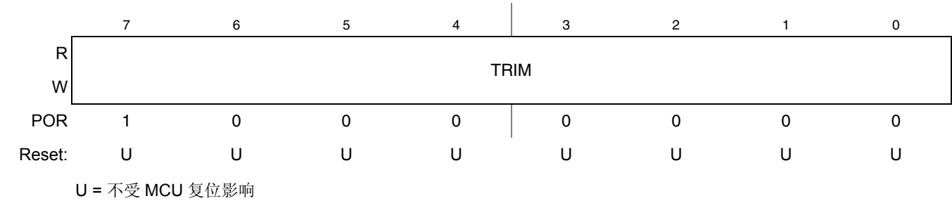
图 8-12. ICG 调整寄存器 (ICGTRM)
