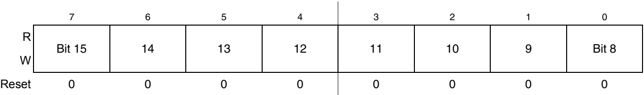
图 12-13. TPM 通道值寄存器高位 (TPMxCnVH)
