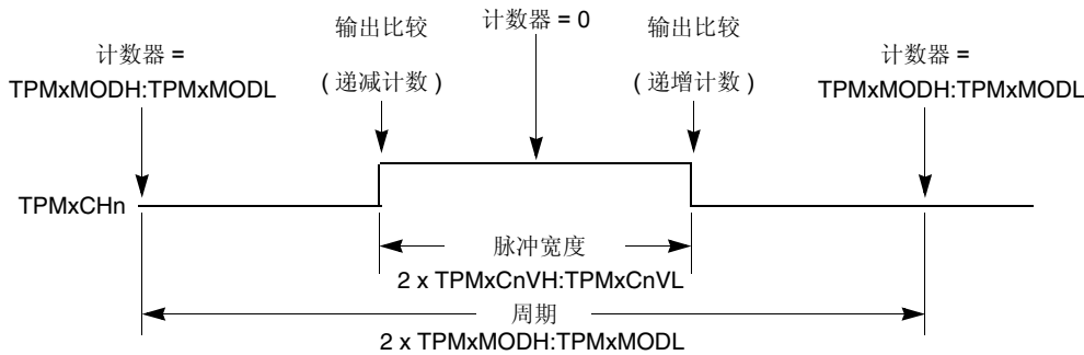
图 12-16. 16CPWM 周期和脉冲宽度（ELSnA=0）
