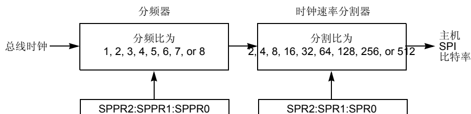
图 11-4. SPI 波特率发生器
