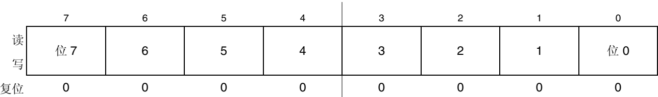
图 12-11. TPM 计数器模寄存器低位 (TPMxMODL)
