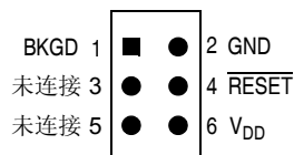
图 13-1. BDM 工具连接器
