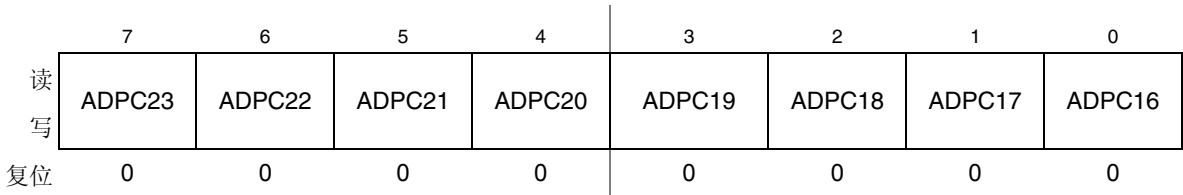
图 9-12. 引脚控制 3 寄存器 (APCTL3)
