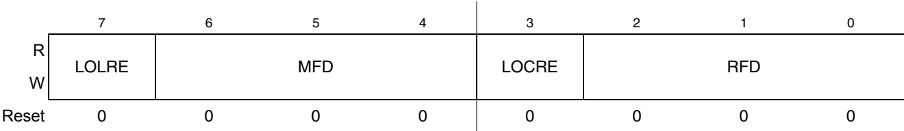
图 8-7. ICG 控制寄存器 2 (ICGC2)
