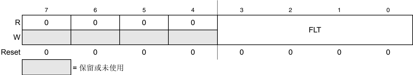
图 8-10. ICG 滤波寄存器高八位 (ICGFLTU)
