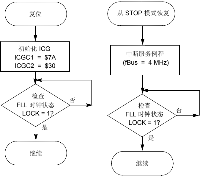
图 8-15. 用于例 2 情况下的 ICG 初始化和从 stop 模式复位
