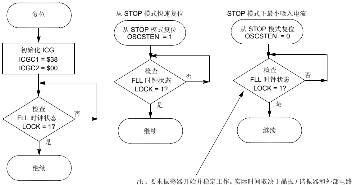
图 8-14. ICG 初始化用于 FEE 在例 1 情况下
