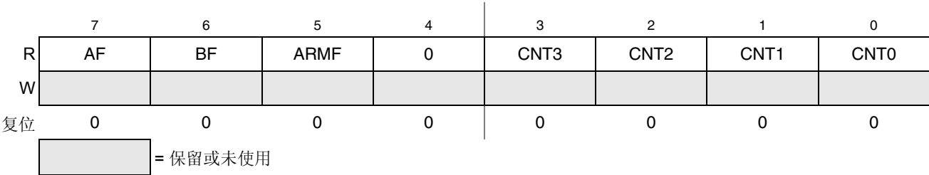
图 13-9. 调试状态寄存器 (DBGS)
