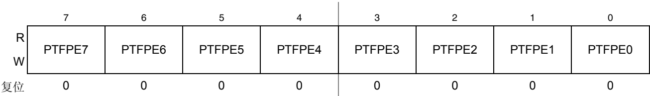
图 6-29. F 端口内部上拉使能寄存器 (PTFPE)
