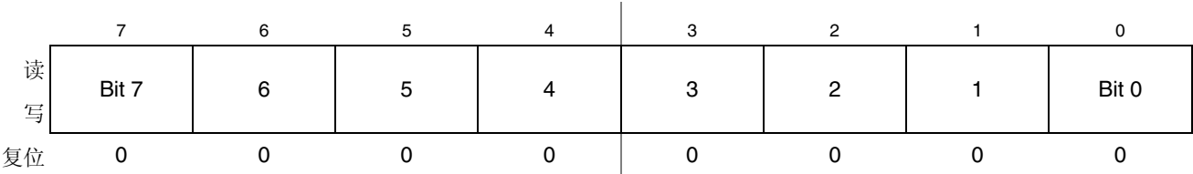
图 11-9. SPI 数据寄存器（SPID）
