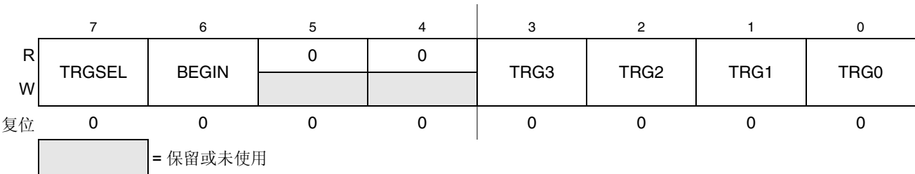
图 13-8. 调试触发寄存器 (DBGT)
