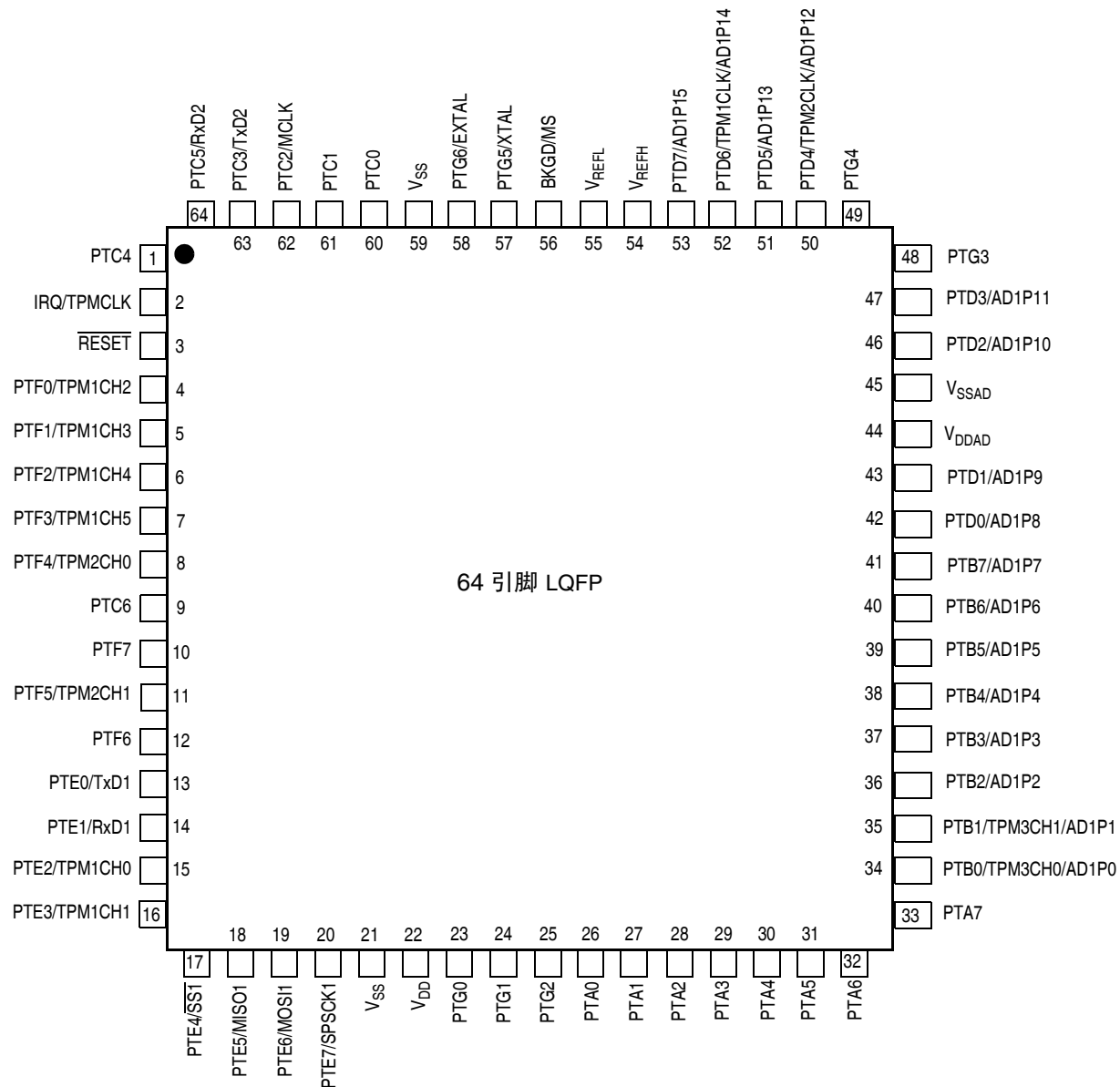
图 2-1. SC116009 系列 64 引脚 LQFP 封装
