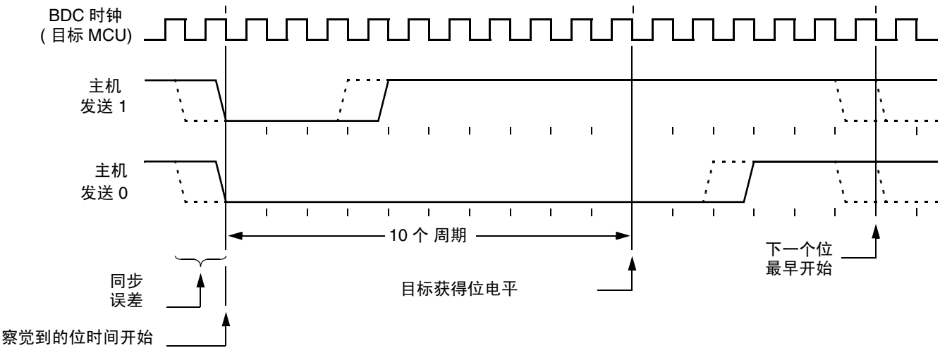
图 13-2. BDC 主机到目标方向串行位时序
