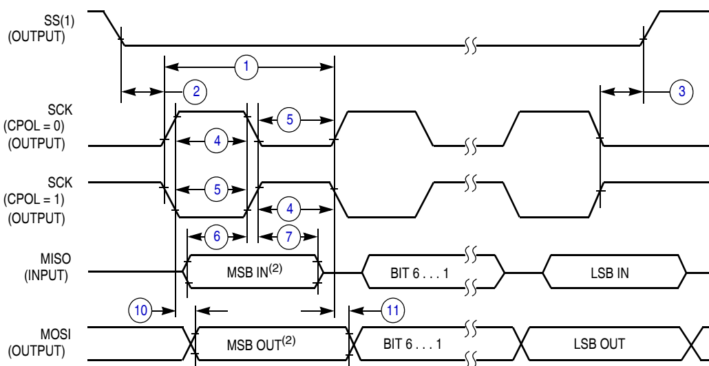
图 A-15. SPI 主时序 (CPHA = 0)
