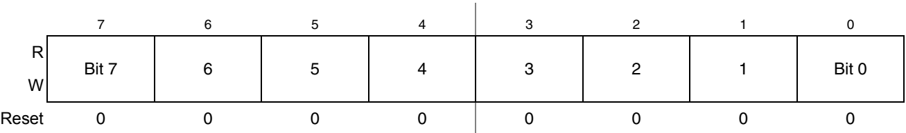
图 12-14. TPM 通道值寄存器低位 (TPMxCnVL)
