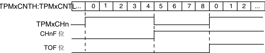
图 12-3. 边缘对齐 PWM 模式的高真脉冲
