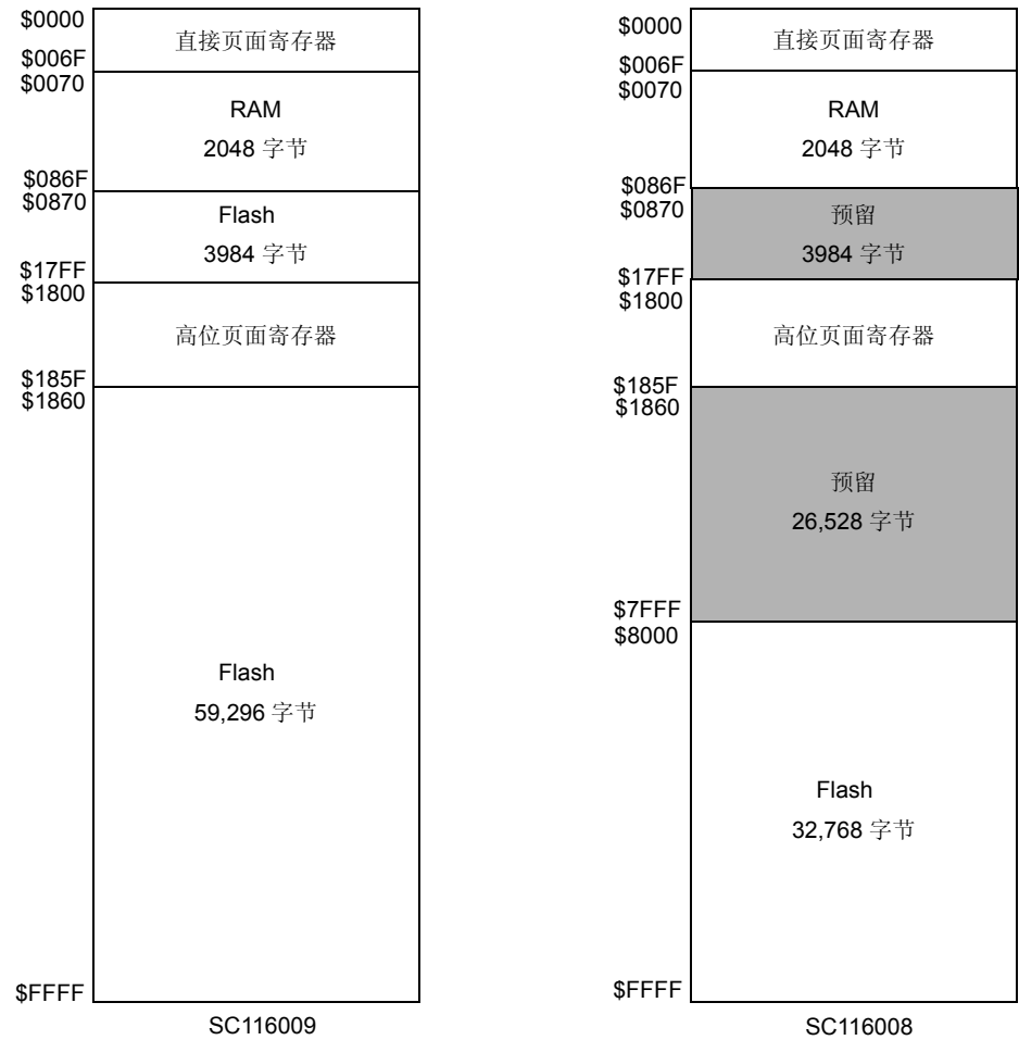
图 4-1. SC116009 系列存储器映射
