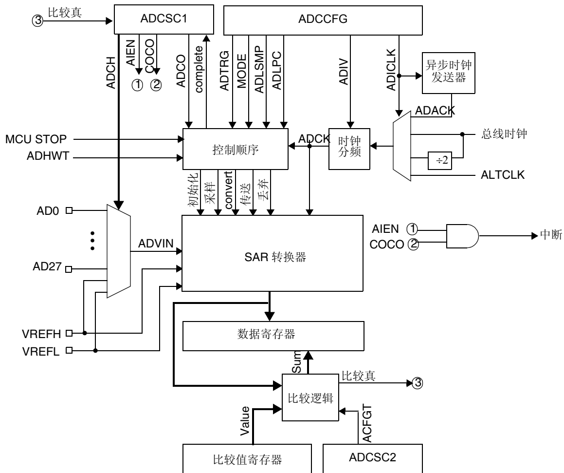
图 9-2. ADC 框图
