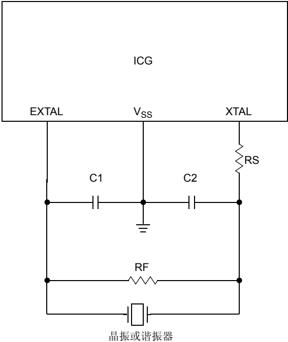
图 8-5. 使用外部参考频率的连接
