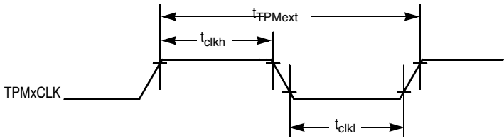
图 A-13. 定时器外部时钟
