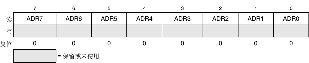
图 9-6. 数据低结果寄存器 (ADCRL)
