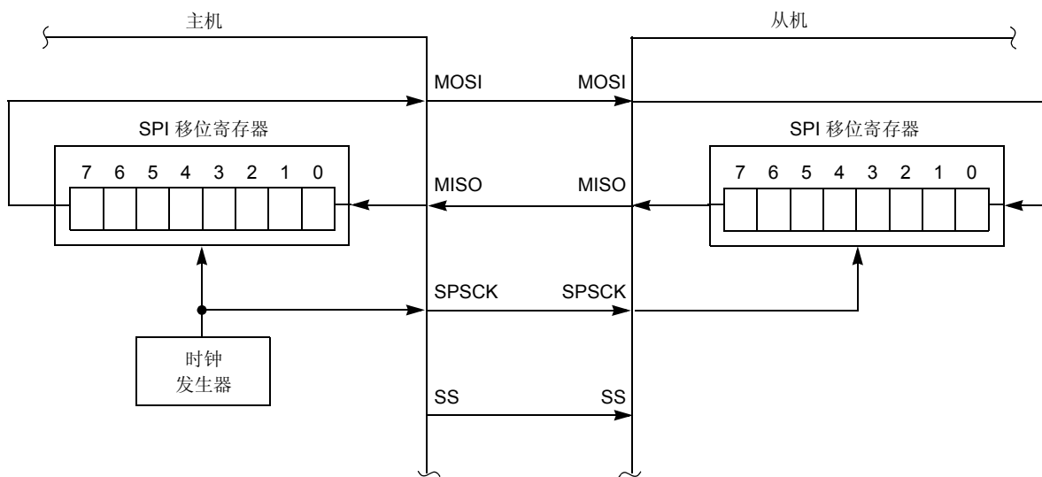
图 11-2. SPI 系统连接
