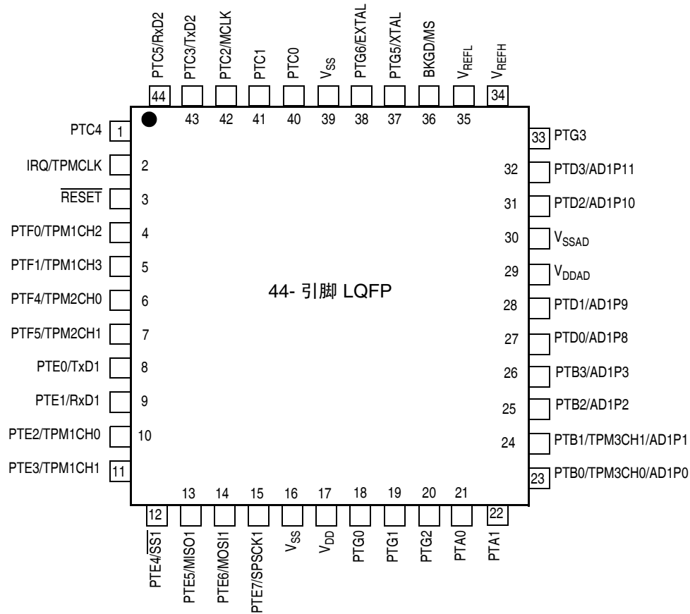
图 2-2. SC116009 系列 44 引脚 LQFP 封装
