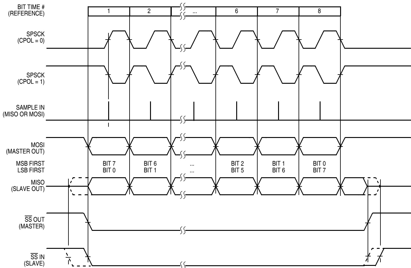
图 11-11. SPI 时钟格式 (CPHA=0)
