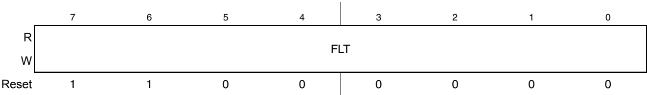
图 8-11. ICG 滤波寄存器低八位 (ICGFLTL)
