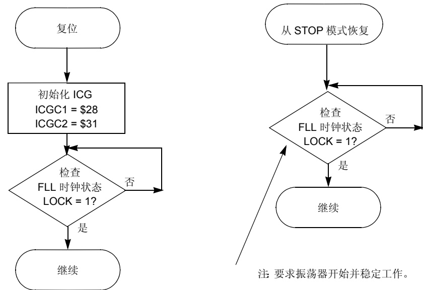
图 8-16. 用于例 3 情况下的 ICG 初始化和从 stop 模式复位
