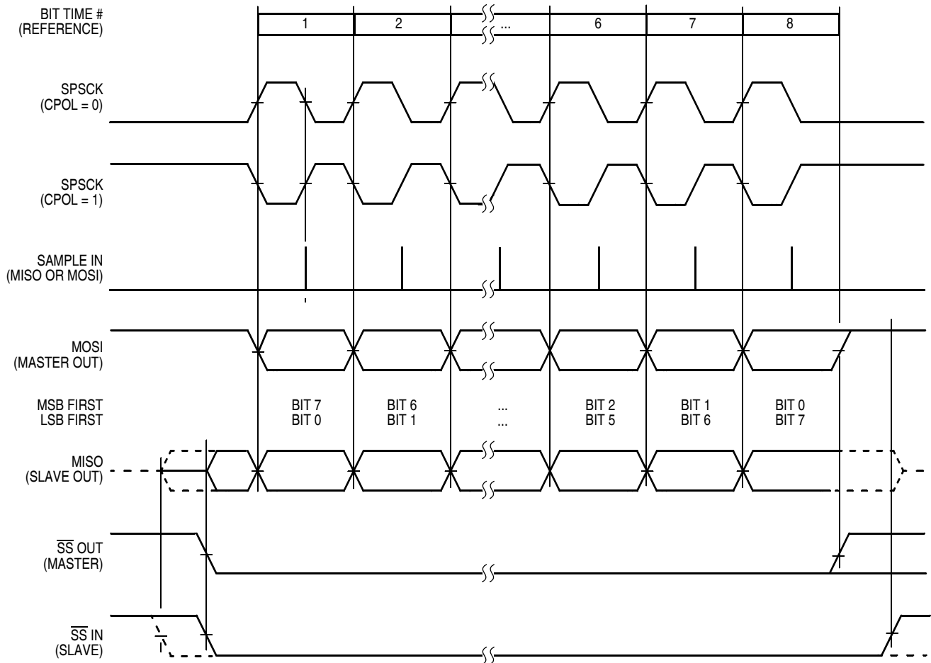
图 11-10. SPI 时钟格式 (CPHA=1)
