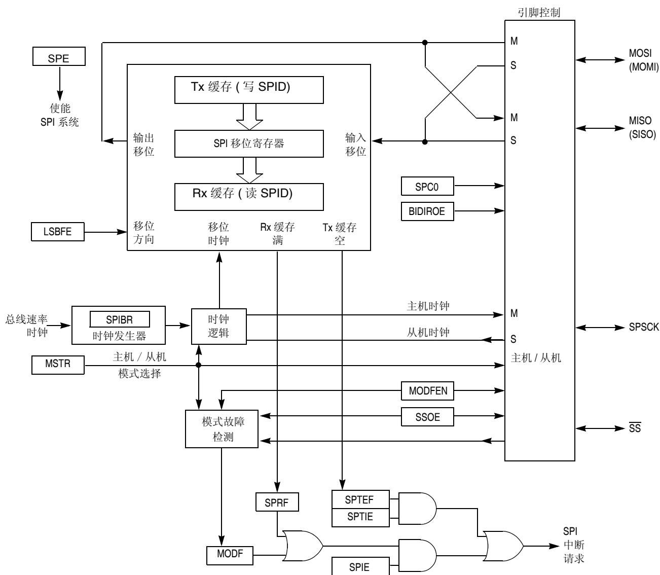
图 11-3. SPI 模块结构图
