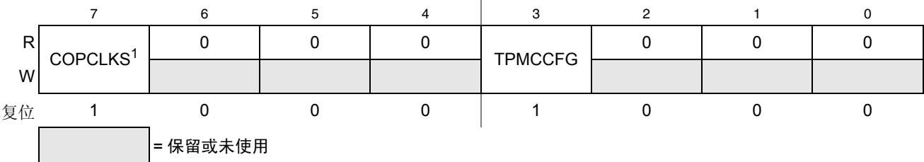
图 5-11. 系统选项寄存器 2 (SOPT2)
