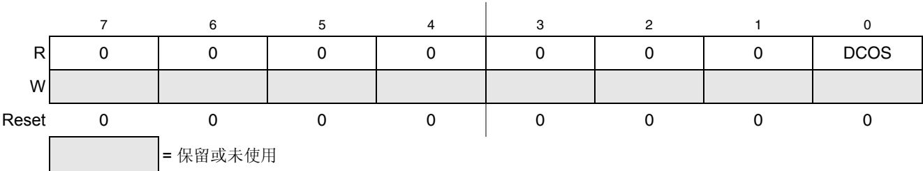
图 8-9. ICG 状态寄存器 2（ICGS2）
