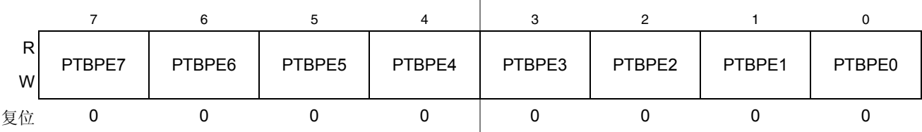
图 6-9. B 端口内部上拉使能寄存器 (PTBPE)
