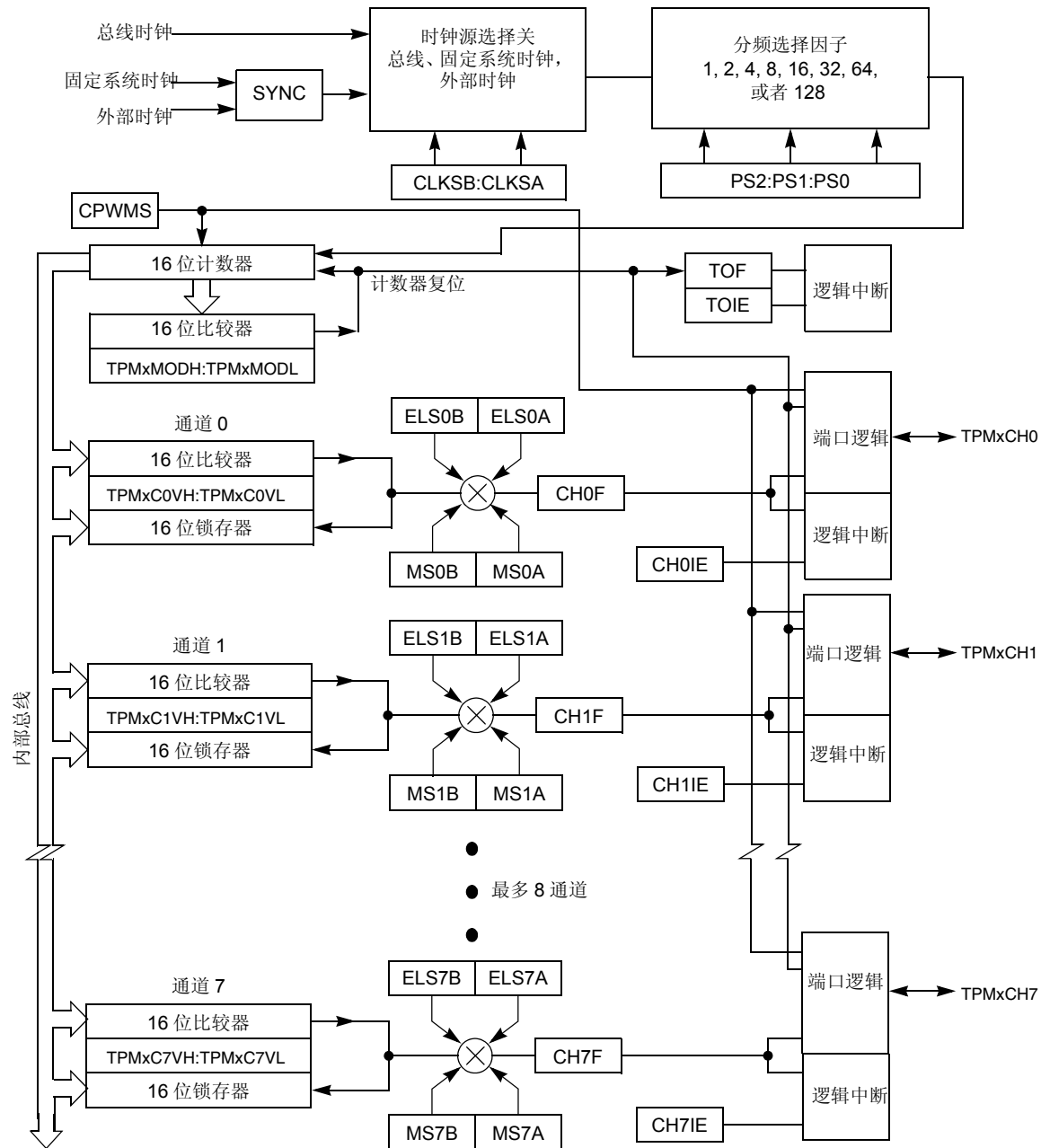
图 12-2. TPM 结构图
