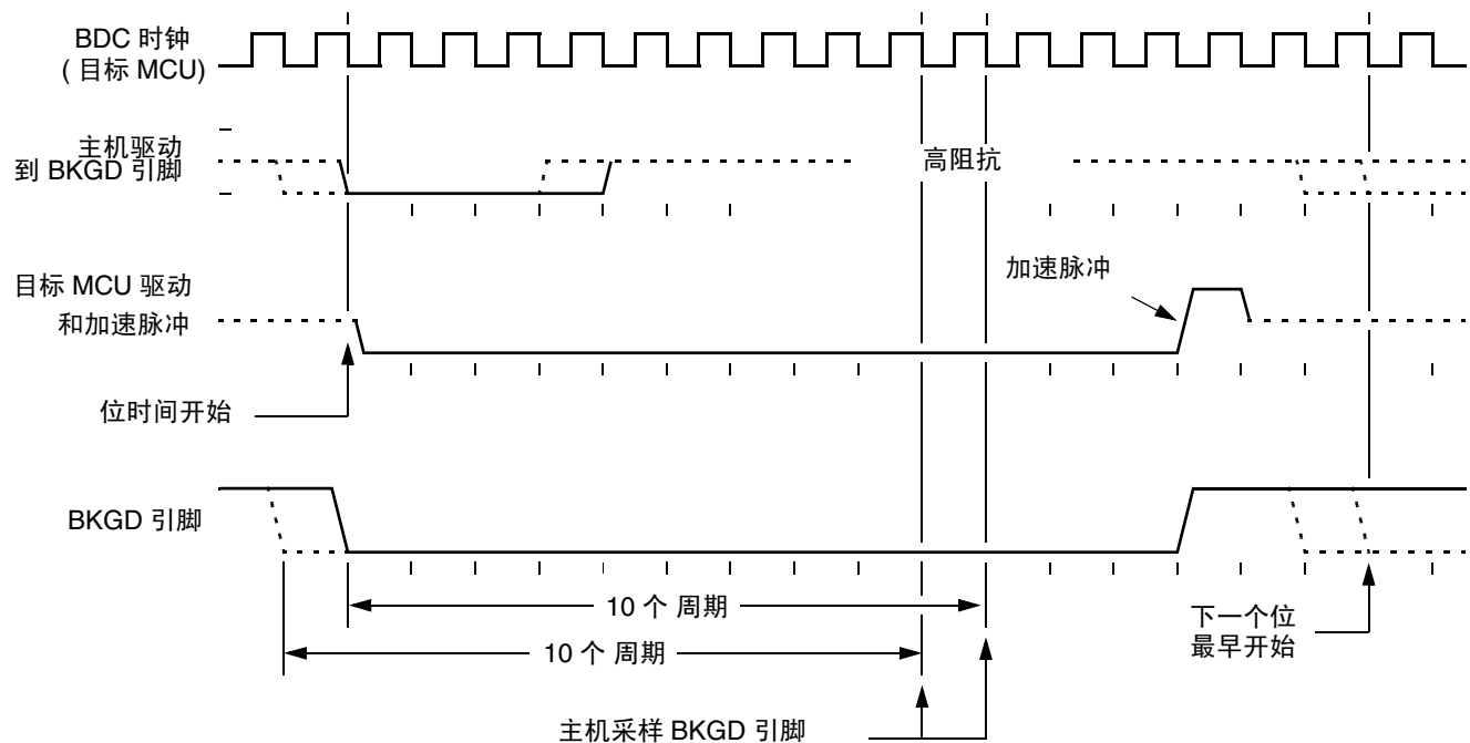
图 13-4. BDM 目标 - 到 - 主机串行位时序 (逻辑 0)
