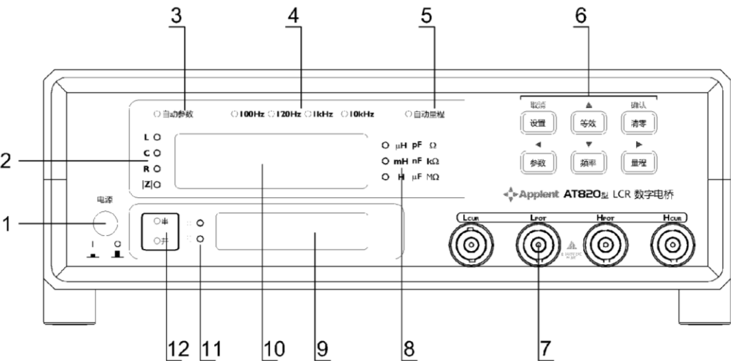
图 3-1 前面板
