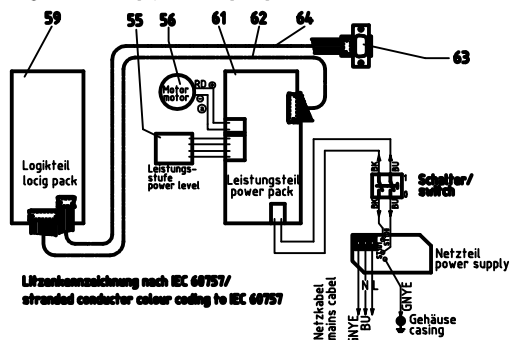
© Verdrahtungsplan/wiring diagram
