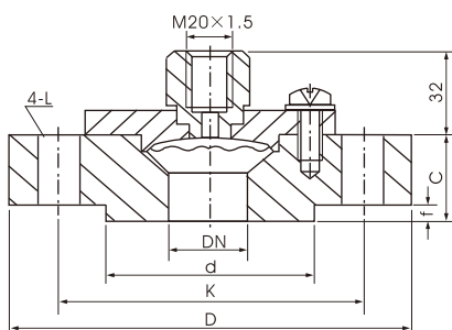
图一：MF1型 ( P \leq 4\text{MPa} ) Drawing 1, MF1 Type
