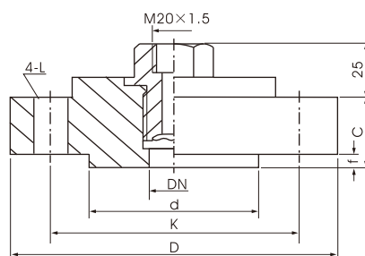
图二：MF1型 ( 6\text{MPa} \leq P \leq 25\text{MPa} ) Drawing 2, MF1 Type
