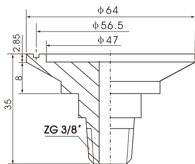
夹子式下座 1Cr18Ni9
