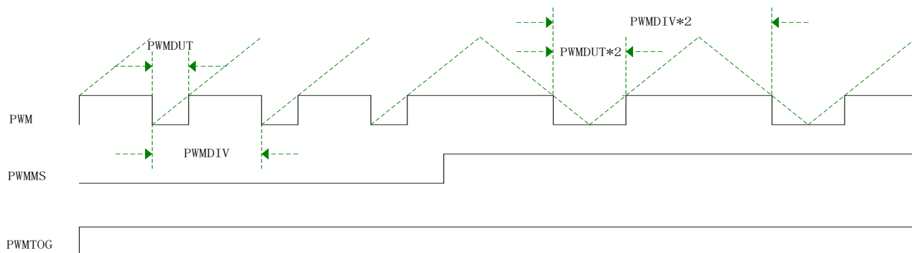
图 18-1-2 PWMTOG=1 时 PWM 输出波形
