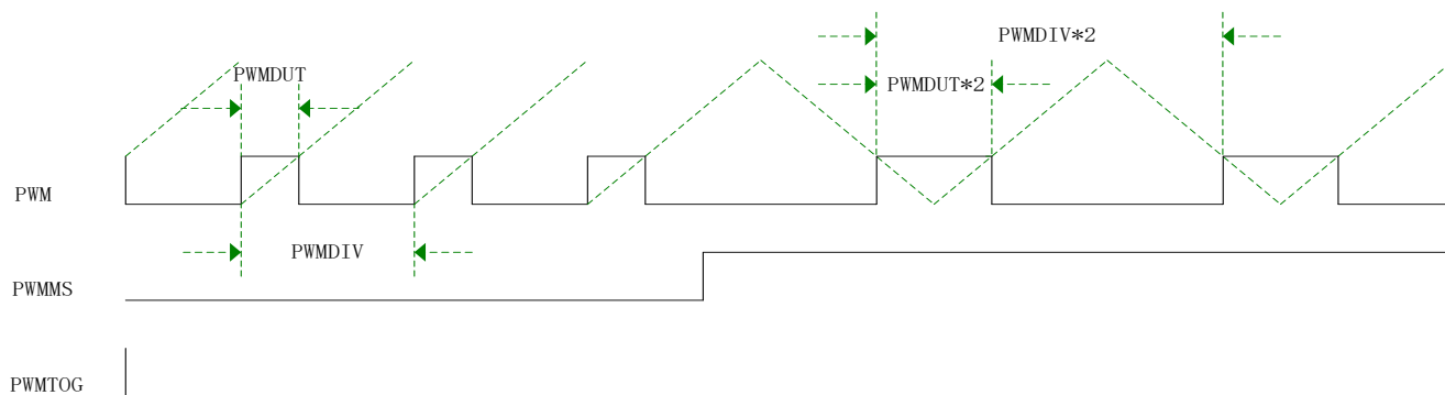
图 18-2-1 PWMTOG=0 时 PWM 输出波形
