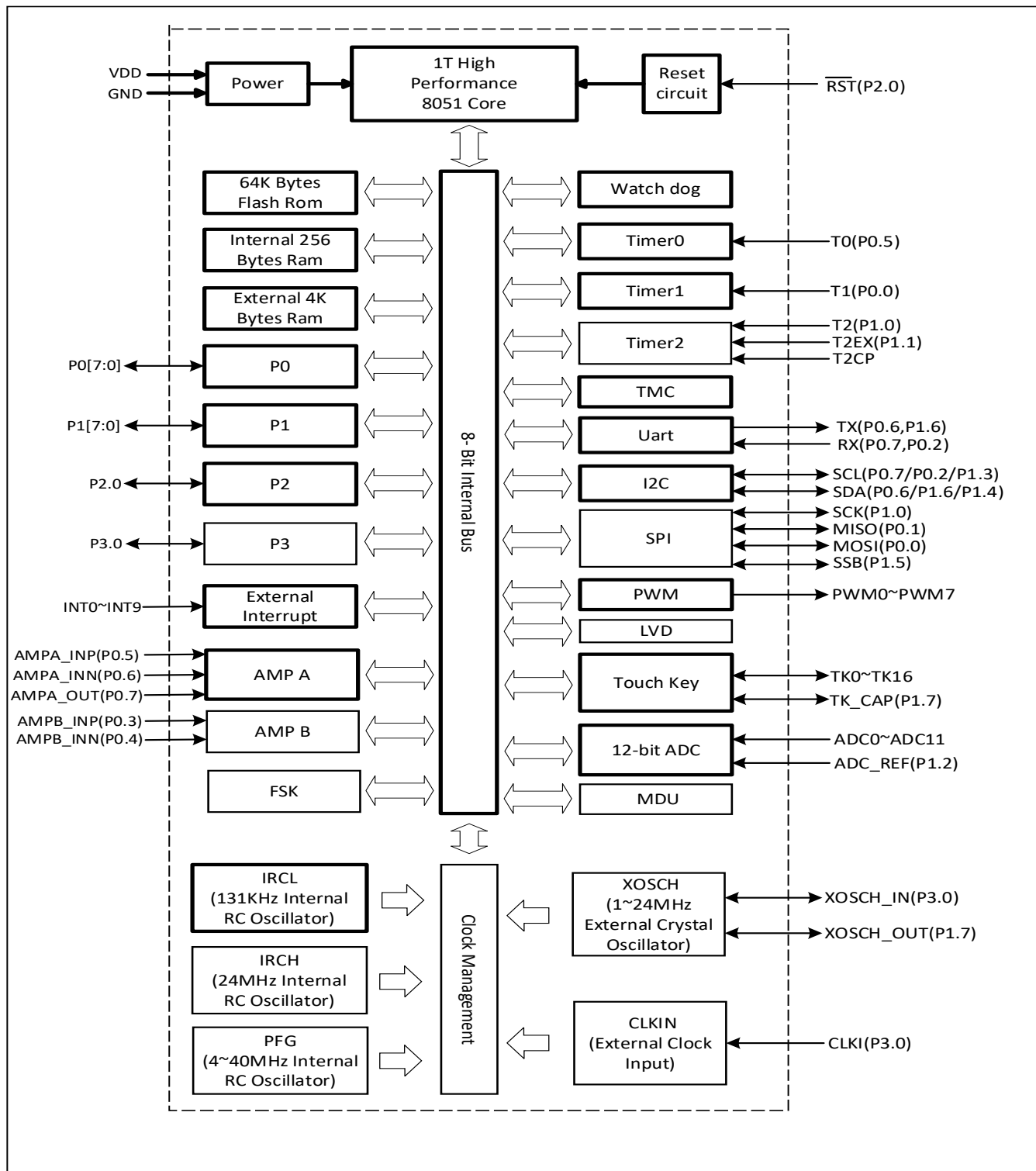
图 4-1-1 芯片框图
