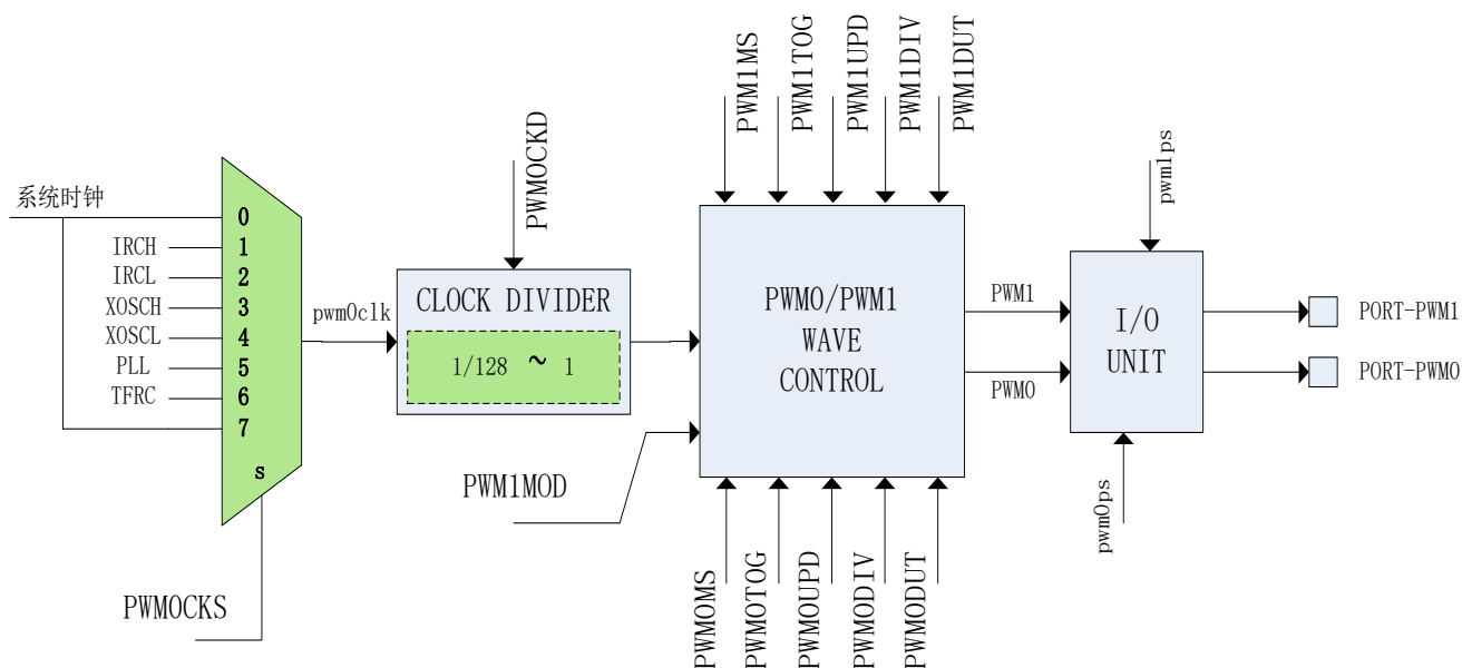
图 18-1-3 PWM0、PWM1 原理示意图
