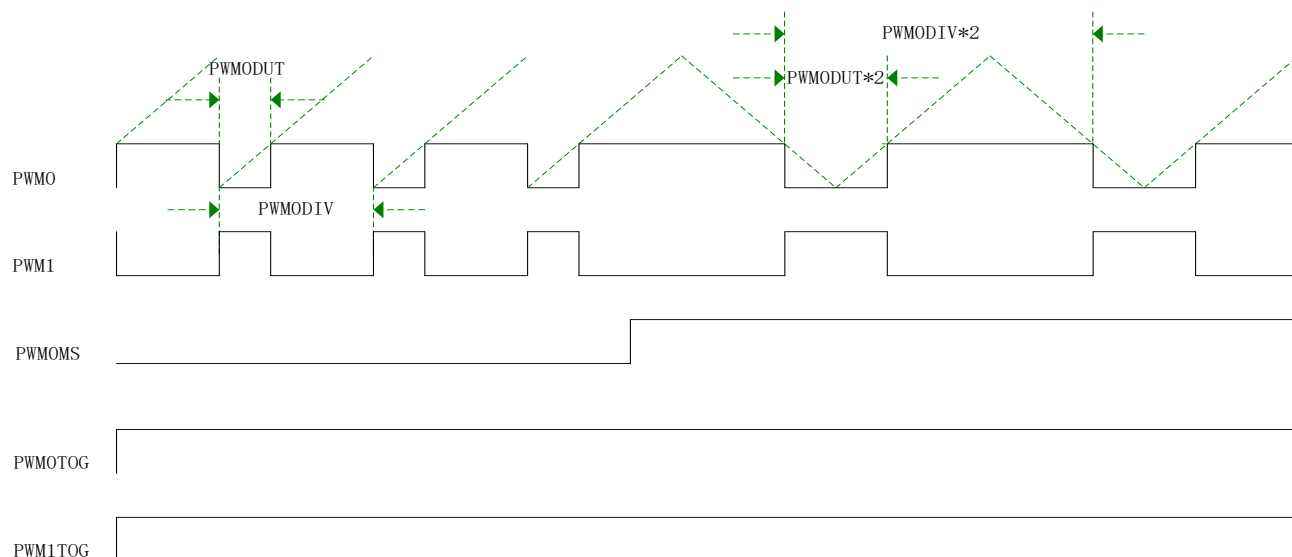
图 18-1-5 PWMTOG=1 时 PWM0、PWM1 输出互补波形
