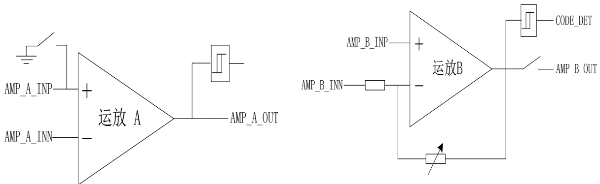
图 20-3-1 运放结构图
