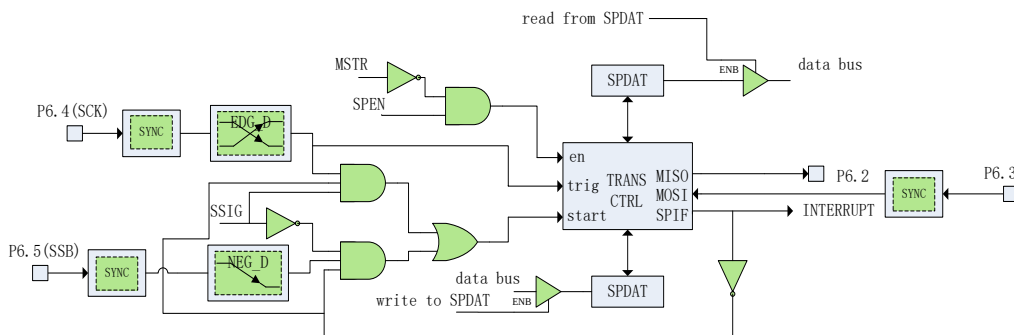
图 25-1-2 SPI 从机模式示意图
