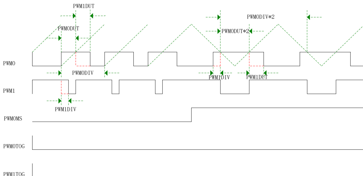
图 18-1-6 PWMTOG=0 时 PWM0、PWM1 死区控制波形
