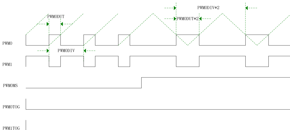
图 18-1-4 PWMTOG=0 时 PWM0、PWM1 输出互补波形
