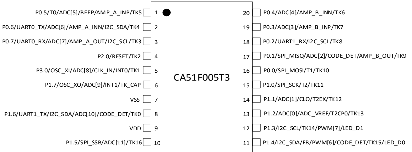
图 5-1-1 TSSOP20 封装图
