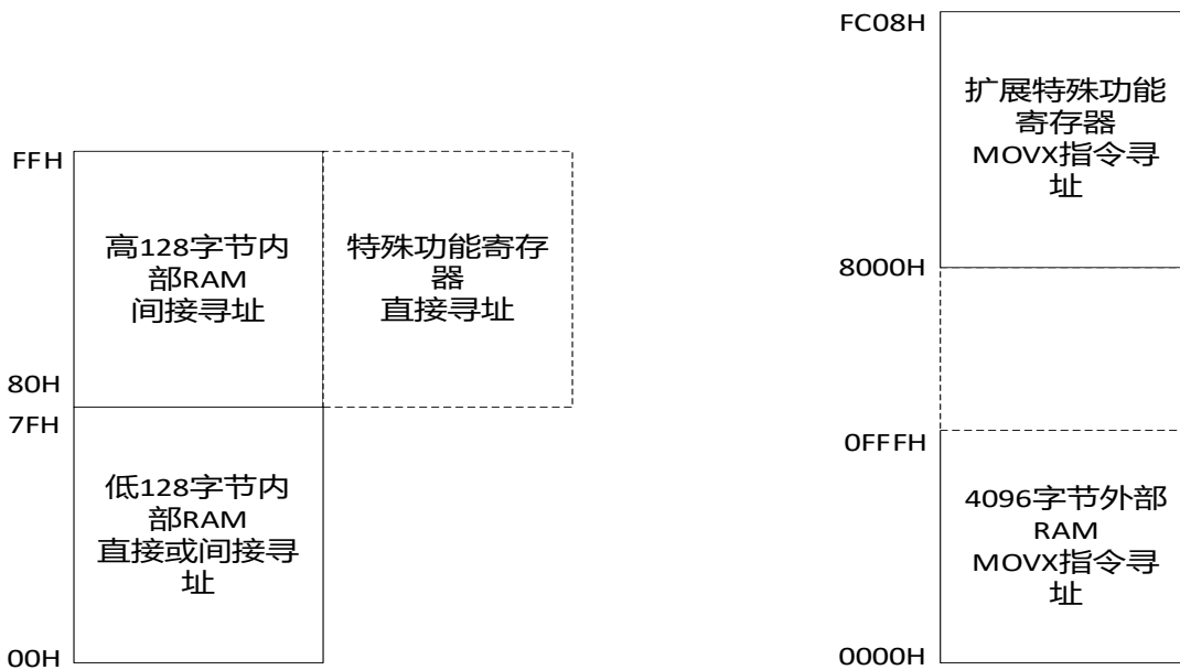
图 7-1-1 RAM 组织结构图
