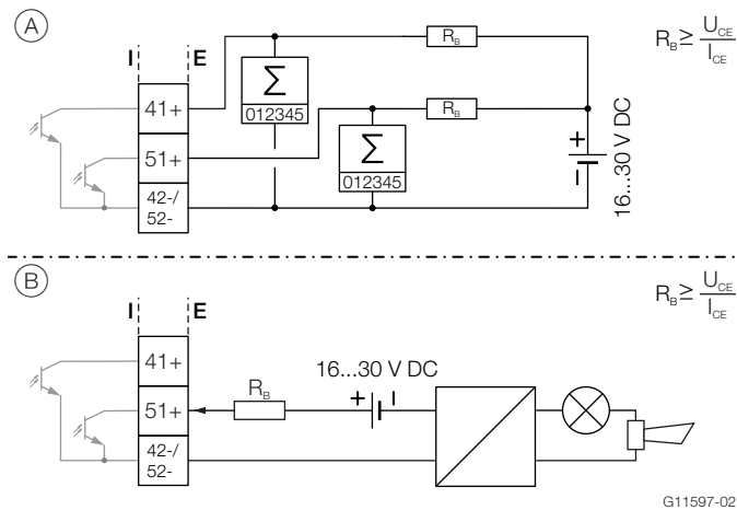
Fig. 34: (I = internal, E = external, R_B = load)
