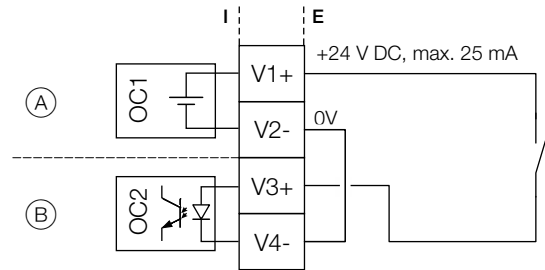
Fig. 43: Active digital input V3 / V4 (example)
