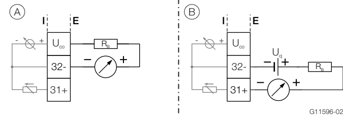
Fig. 32: (I = internal, E = external, R_B = load)
