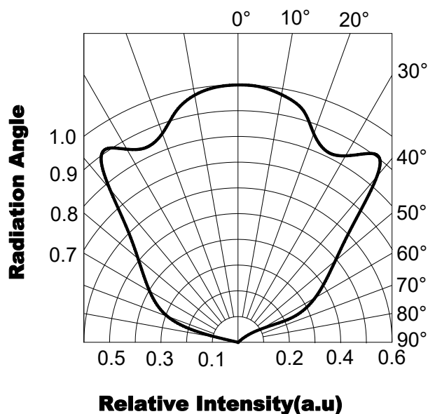
角度与相对发光强度 (Ta=25°C)
