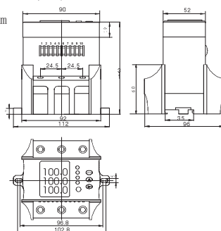
MS2320-T 外形图 Outline demension
