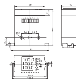
MS2320 外形图 Outline demension
