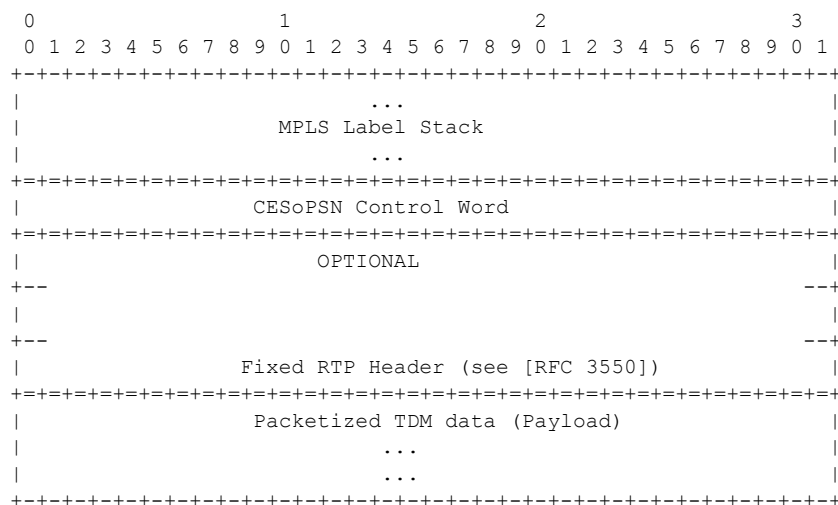
Figure 10: CESoPSN MPLS Encapsulation
