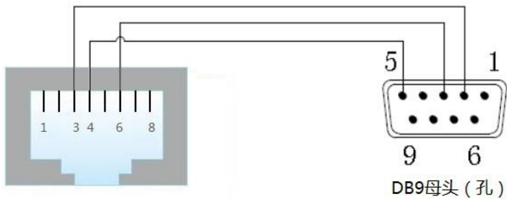
图 2.7 GCAN-PLC-400 可编程序控制器 RS-232 接口
