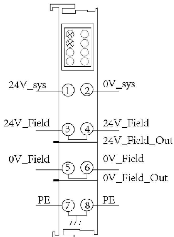
图 2.5 GCAN-PLC-400 可编程序控制器电源接线端子排
