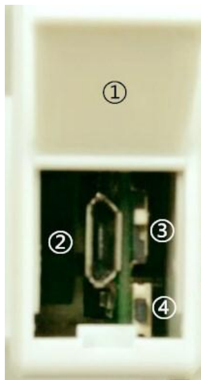
图 4.1 编程下载接口实物图
