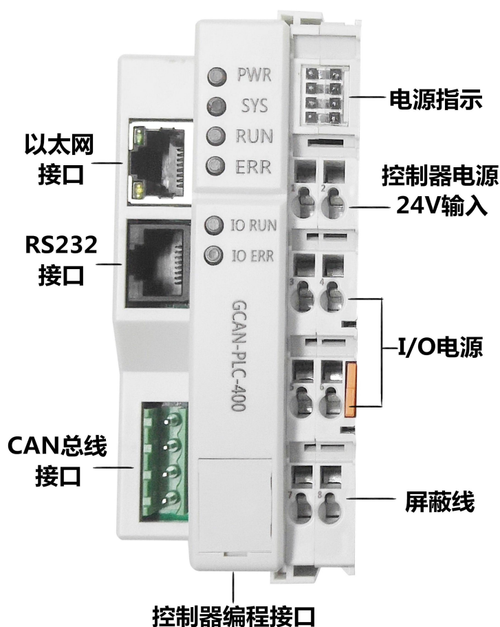
图 2.1 GCAN-PLC-400 可编程序控制器外观图
