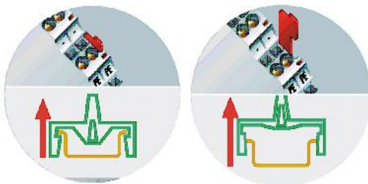
图 2.3 GCAN-PLC-400 可编程序控制器自锁机制
