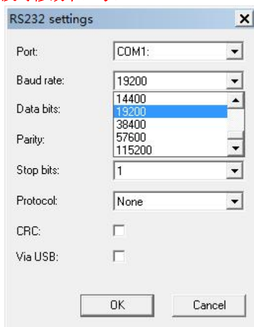
图 5.9 RS232 波特率设置
