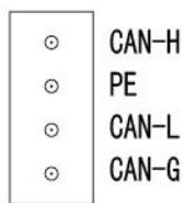
图2.6 GCAN-PLC-400 可编程序控制器CAN总线端子排
