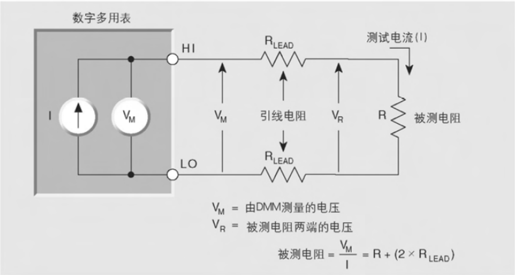
上图为两线制测量原理图
