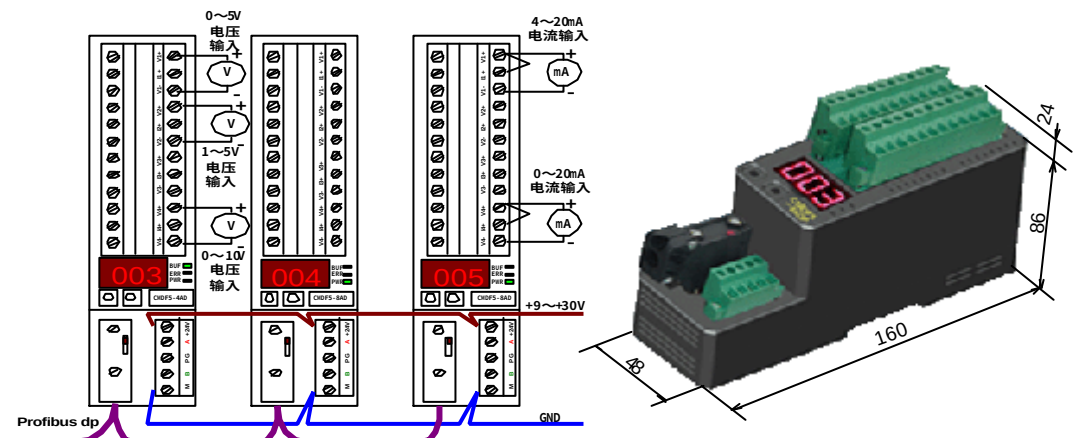
CMD5-4AD 连接示意图
