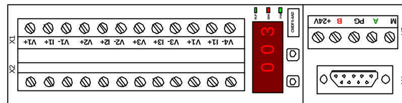
（图 1）CMDF5-4AD 端子示意图
