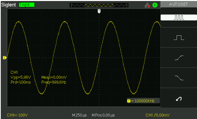
图 2-3 自动设置
