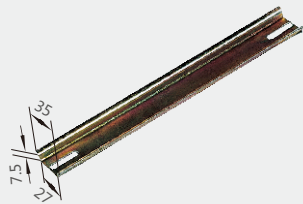
图3 TH35-7.5型安装导轨尺寸
