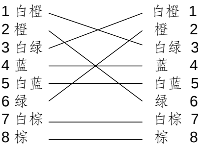
交叉线两端对应关系
