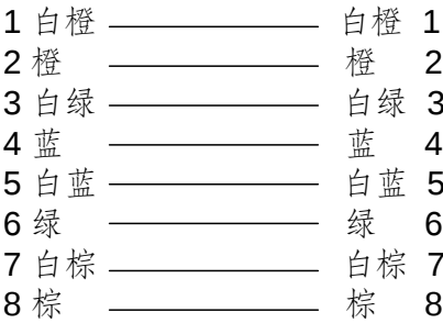
直通线两端对应关系
