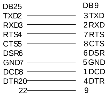
DB25 与 DB9 连线图
