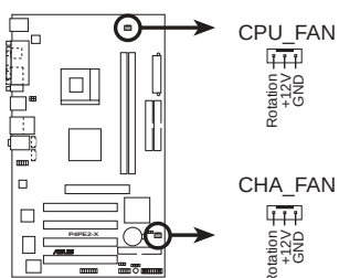
P4PE2-X 12-Volt Fan Connectors
