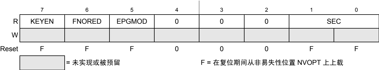
Figure 0-12. Flash 和 EEPROM 选项寄存器 (FOPT)
