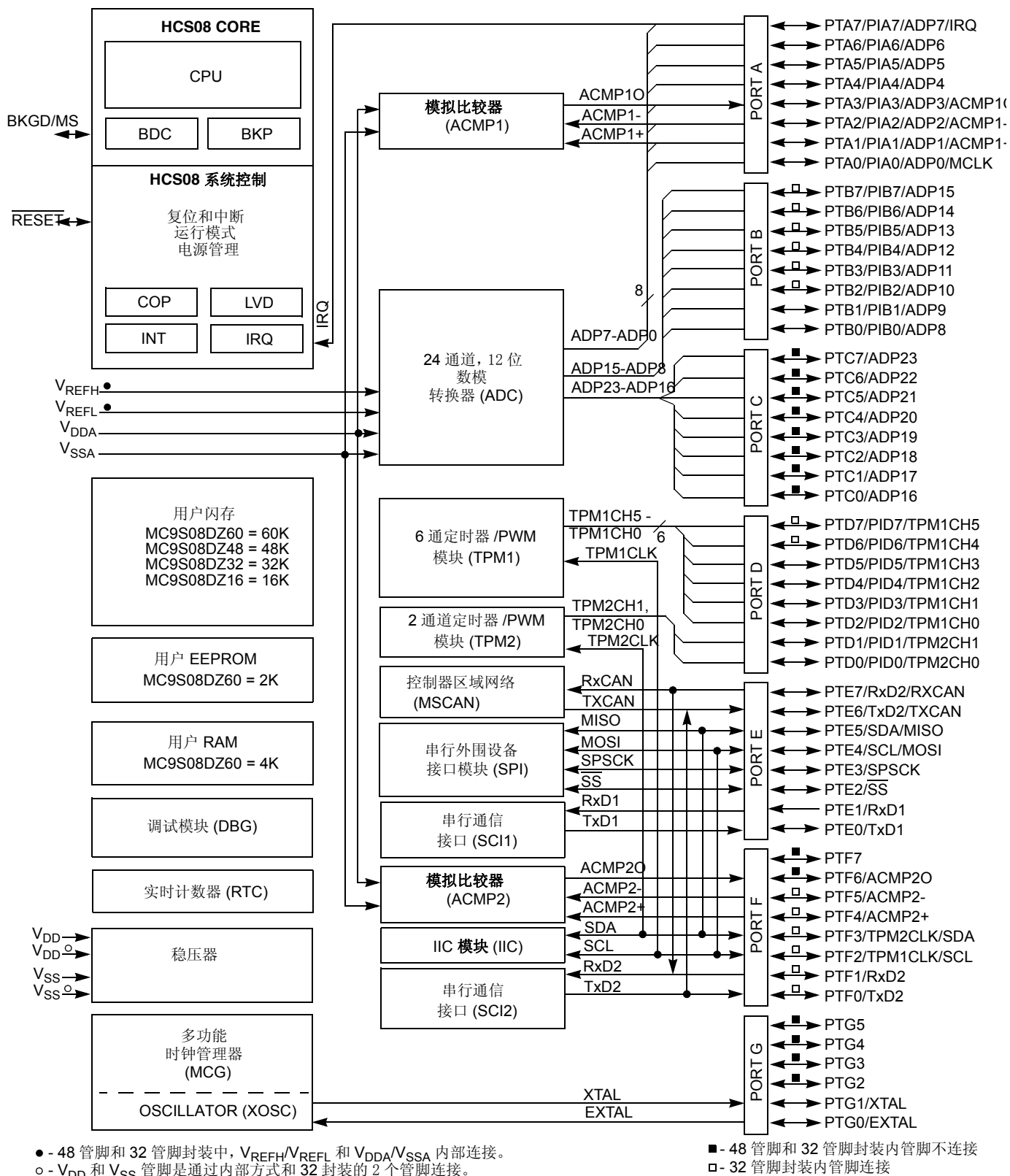
Figure 0-1. MC9S08DZ60 结构图
