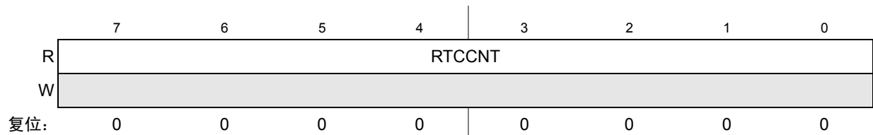
Figure 16-4. RTC 计数器寄存器 (RTCCNT)
