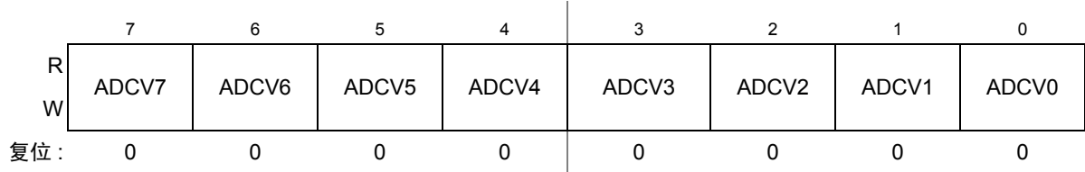
Figure 11-8. 比较值低地址寄存器（ADCCVL）
