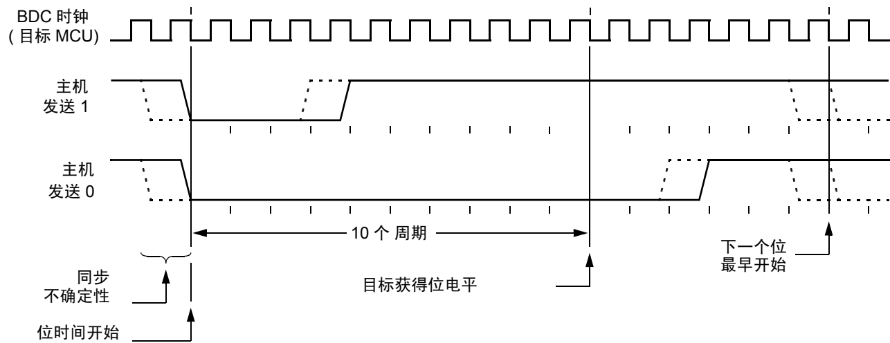
Figure 18-2. BDC 主机到目标方向串行位时序
