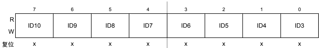
Figure 13-32. 标识符寄存器 0 — 标准映射
