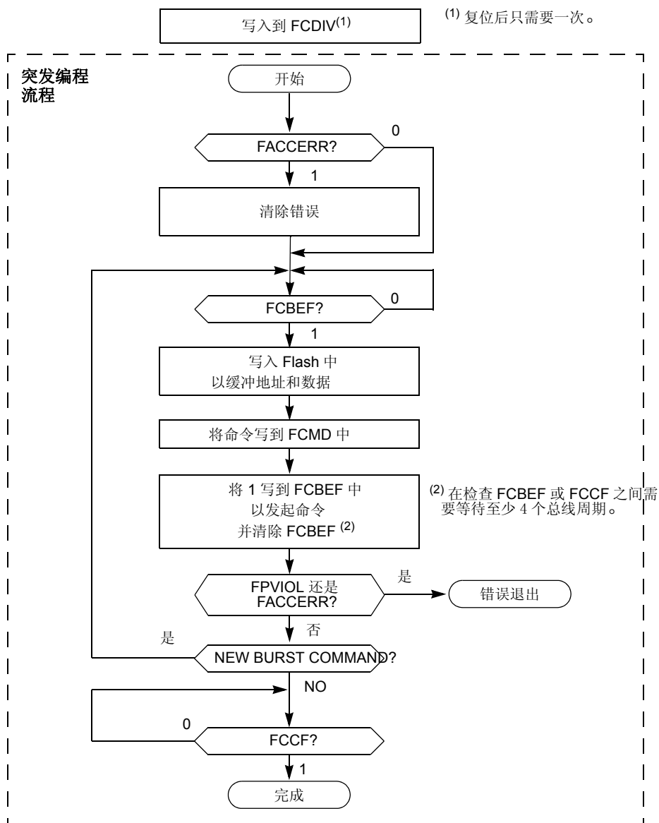
Figure 0-9. 突发编程流程图
