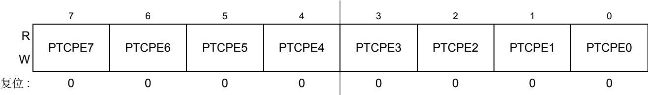
Figure 0-47. C 端口寄存器内部上拉使能 (PTCPE)
