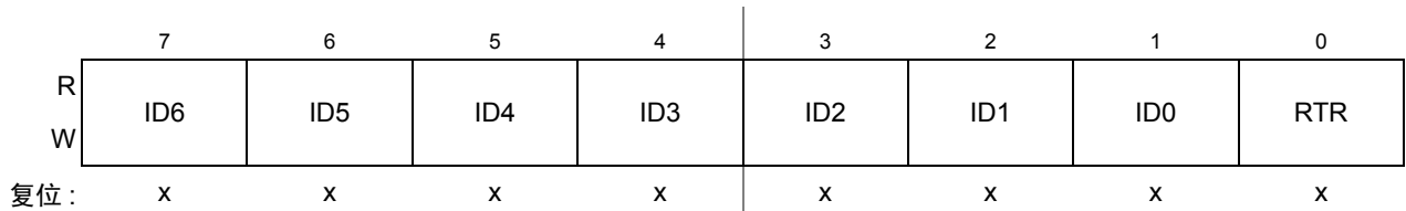
Figure 13-31. 标识符寄存器 3 (IDR3) — 扩展标识符映射
