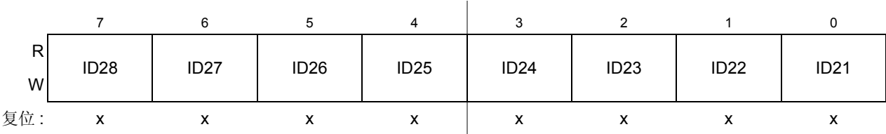
Figure 13-26. 标识符寄存器 1（IDR1）— 扩展标识符映射
