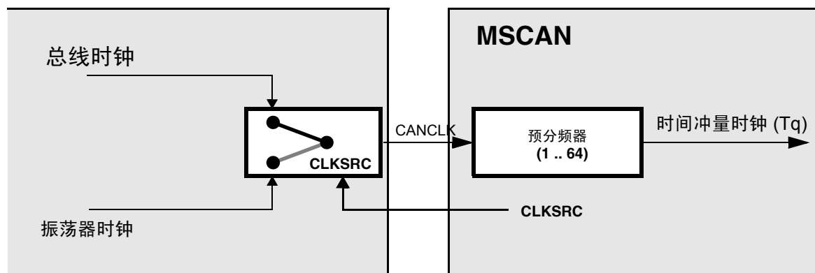
Figure 13-45. MSCAN 时钟机制
