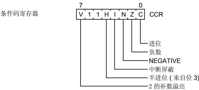
Figure 8-2. 条件码寄存器
