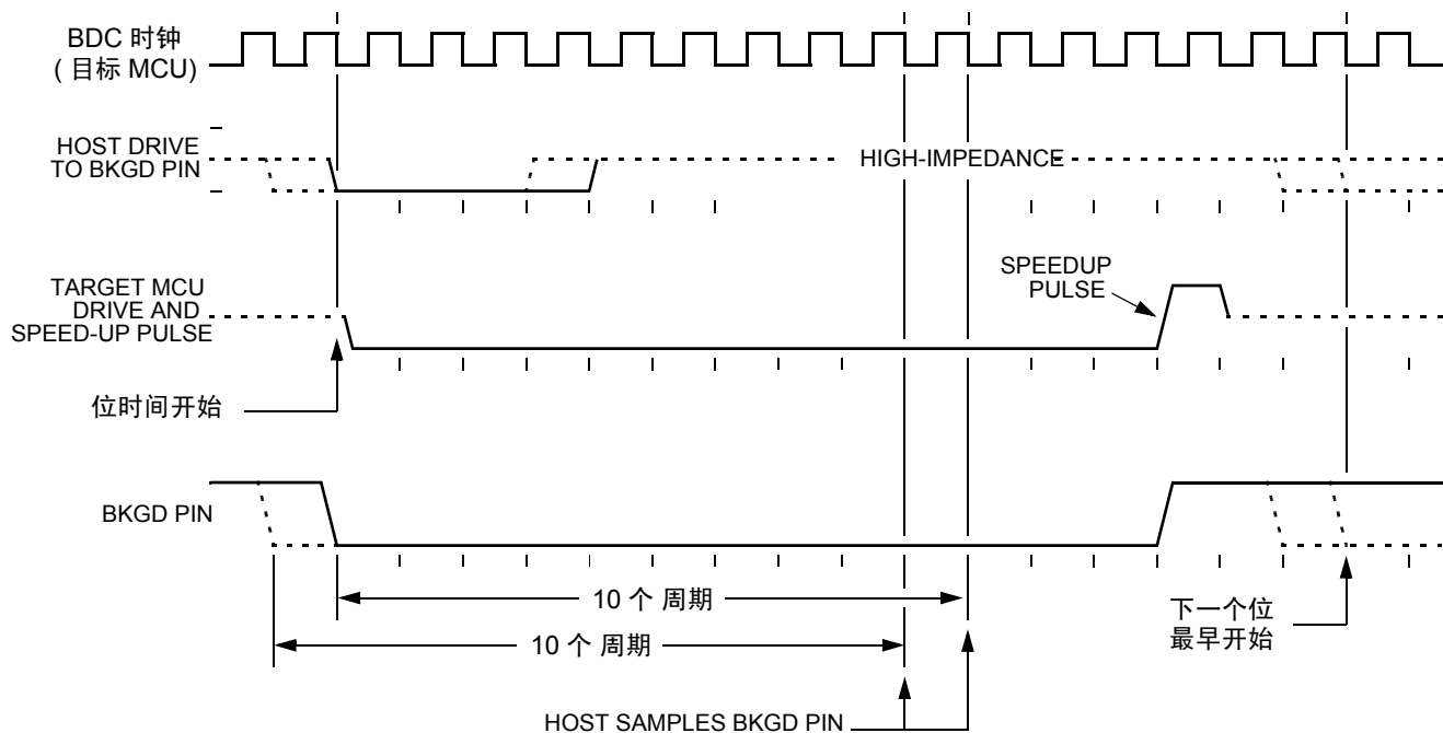
Figure 18-4. BDM 目标 - 到 - 主机串行位时序 (逻辑 0)
