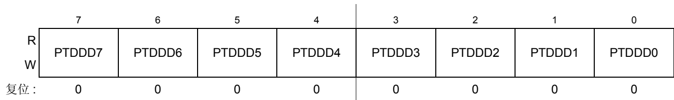
Figure 0-51. D 端口数据方向寄存器 (PTDDD)
