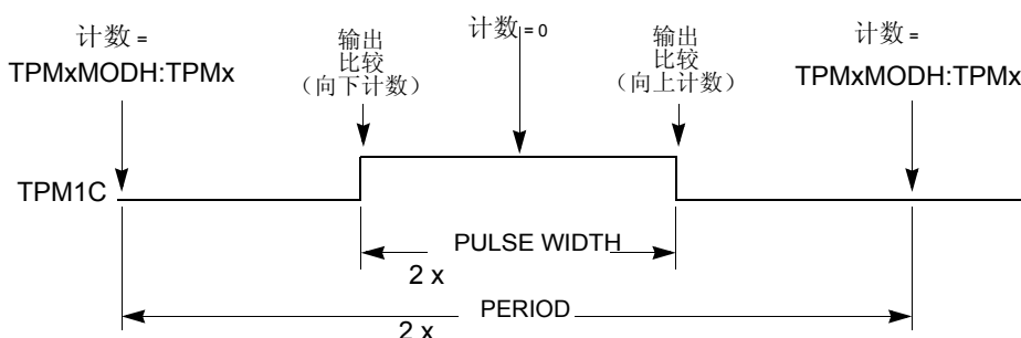
Figure 18-20. CPWM 周期和脉冲宽度 (ELSnA = 0)
