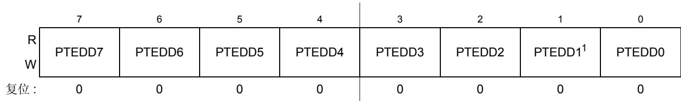
Figure 0-59. E 端口数据方向寄存器 (PTEDD)
