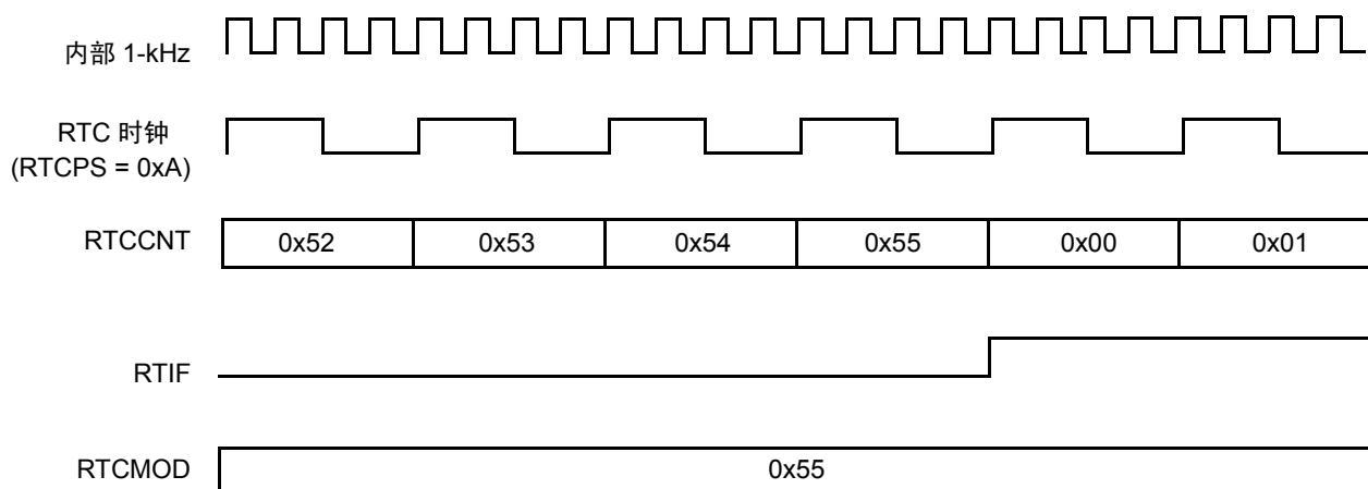
Figure 16-6. RTC 计数器溢出实例
