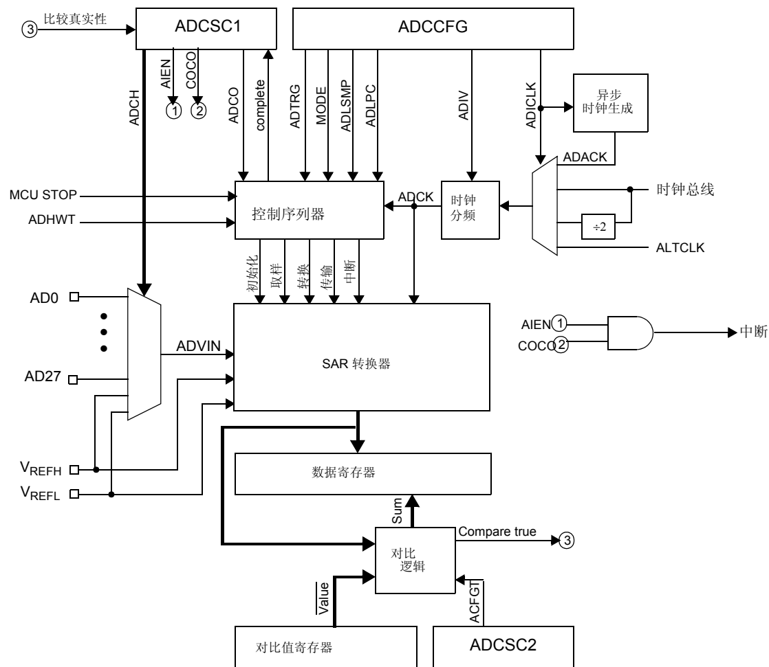
Figure 11-2. ADC 结构图
