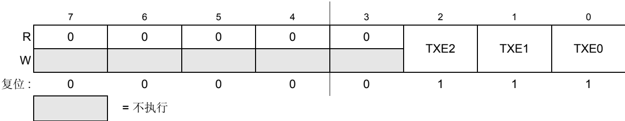
Figure 13-10. MSCAN 发送器标志寄存器 (CANTFLG)
