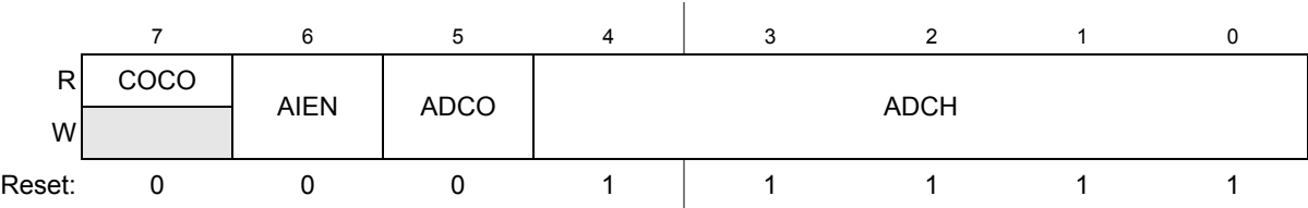
Figure 11-3. 状态和控制寄存器（ADCSC1）
