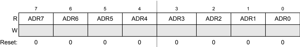
Figure 11-6. 数据结果低态寄存器（ADCRL）
