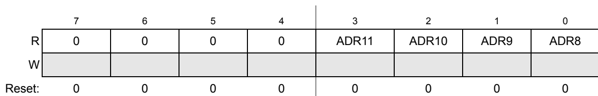
Figure 11-5. 数据结果高地址寄存器 (ADCRH)
