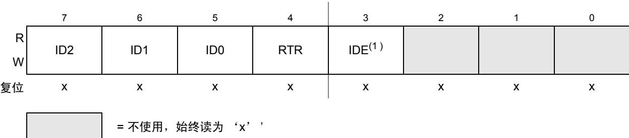
Figure 13-33. 标识符寄存器 1 —标准映射
