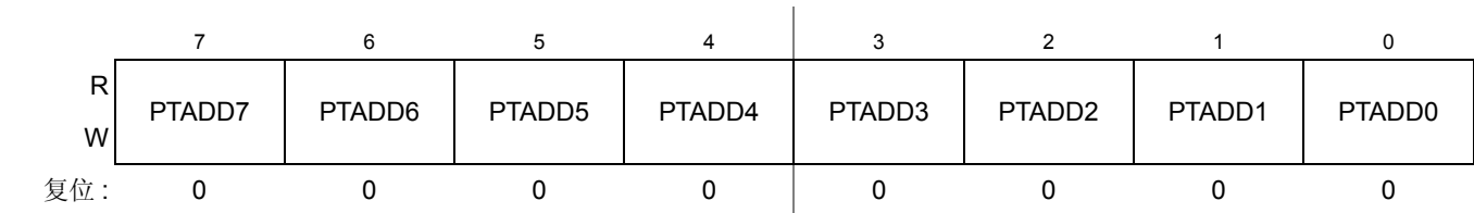
Figure 0-30. 端口数据方向寄存器 (PTADD)
