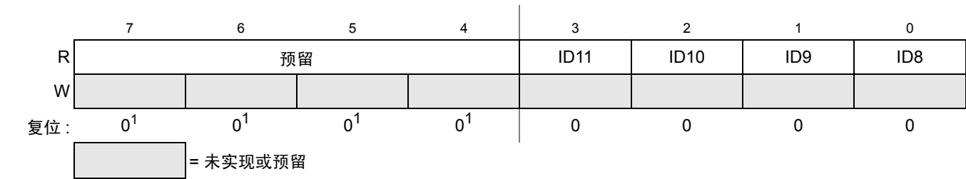
Figure 0-23. 系统器件识别寄存器 — 高 (SDIDH)
