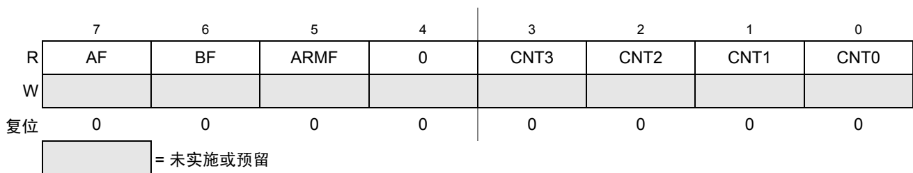
Figure 18-9. 调试状态寄存器 (DBGS)
