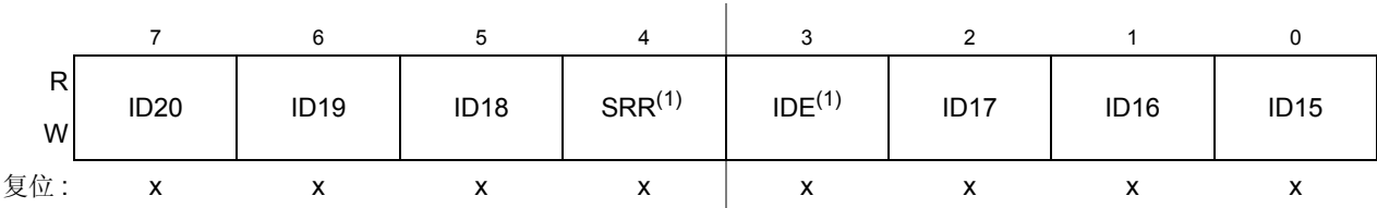
Figure 13-28. I 标识符寄存器 3（IDR3）— 扩展标识符映射
