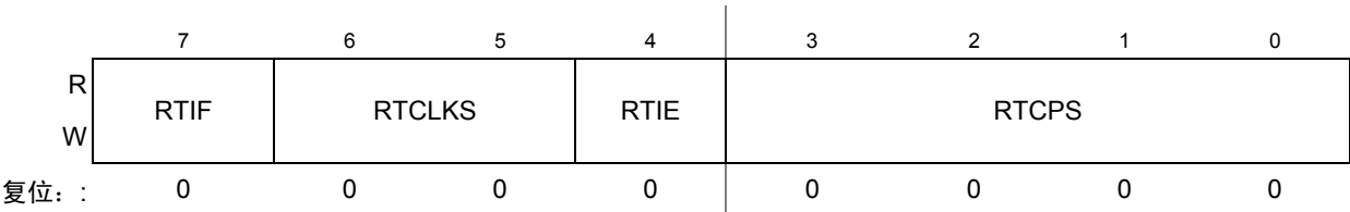
Figure 16-3. RTC 状态和控制寄存器（RTCSC）
