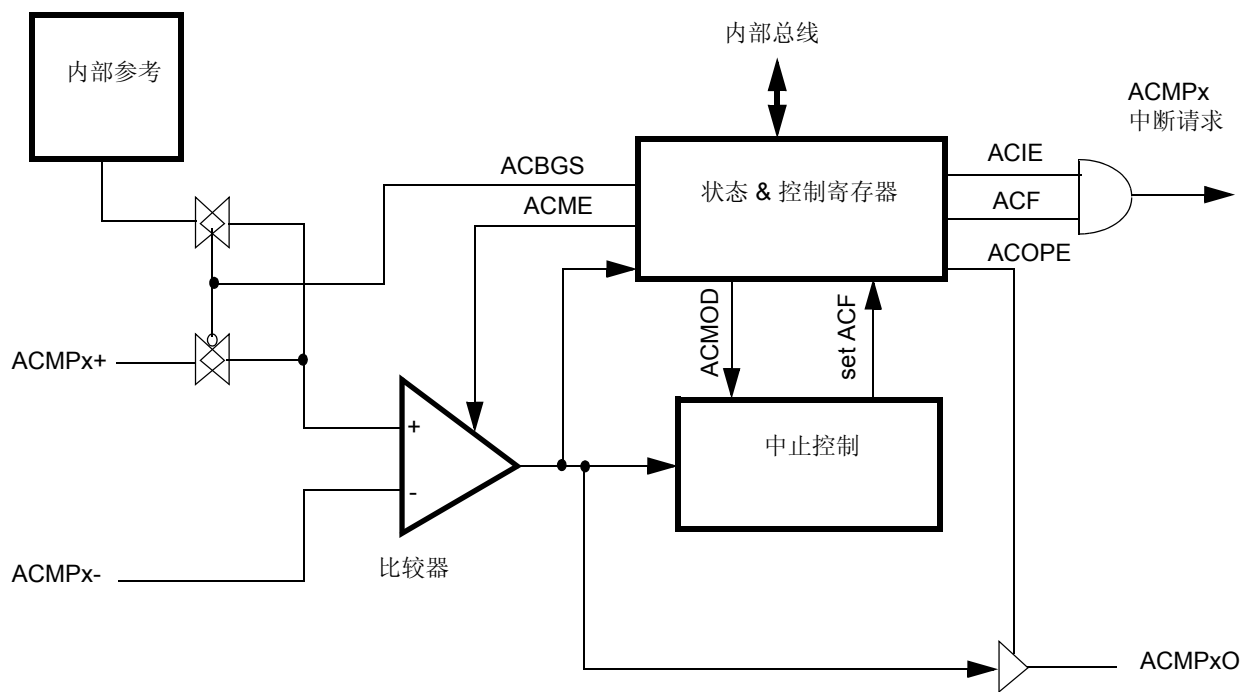
Figure 10-2. 模拟比较器（ACMP）结构图
