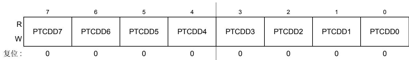
Figure 0-46. C 端口数据方向寄存器 (PTCDD)
