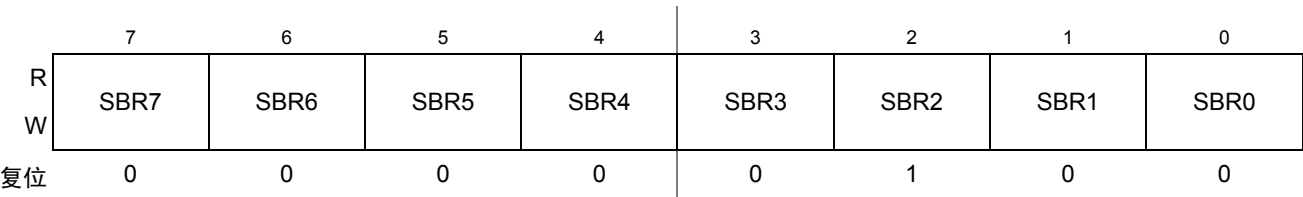
Figure 15-5. 波特率寄存器 (SCIxBDL)
