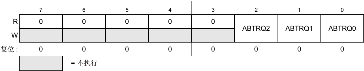
Figure 13-12. MSCAN 发送器报文中止请求寄存器 (CANTARQ)
