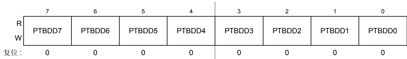
Figure 0-38. B 端口数据方向寄存器 (PTBDD)
