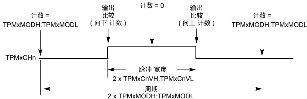
Figure 17-16. CPWM 周期和脉冲宽度（ELSnA=0）
