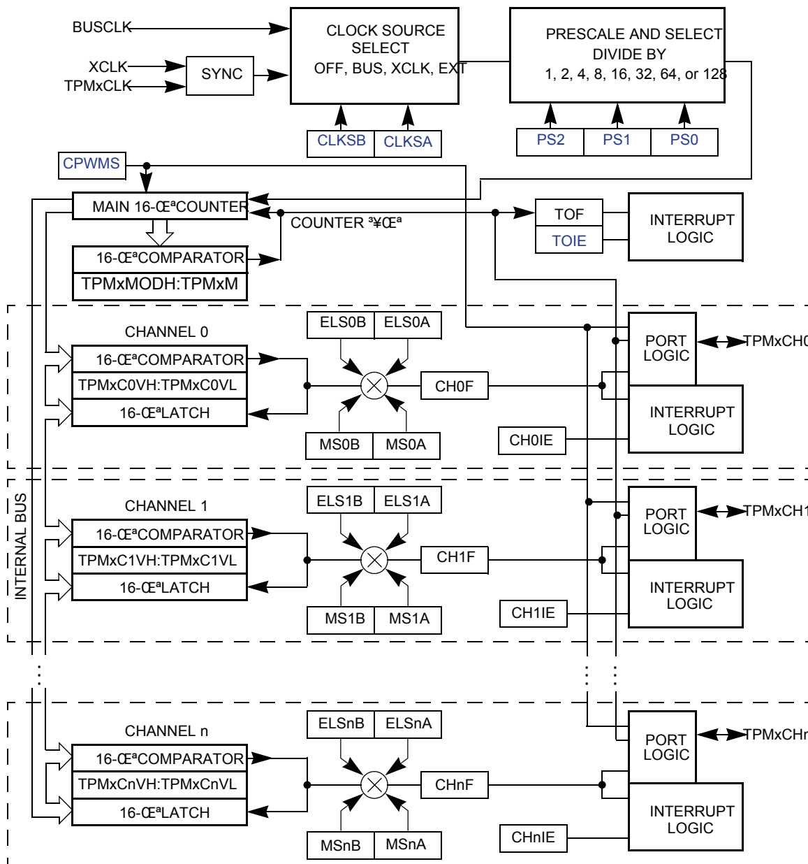
Figure 18-10. TPM 结构图
