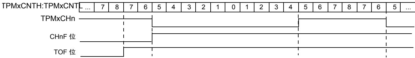
Figure 17-6. 中央对齐 PWM 的 Low-True 脉冲
