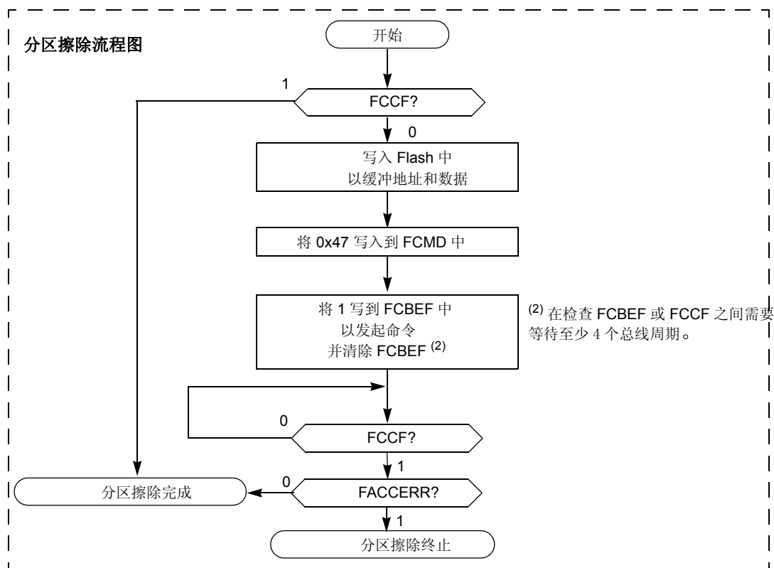
Figure 0-10. 分区擦除终止流程图
