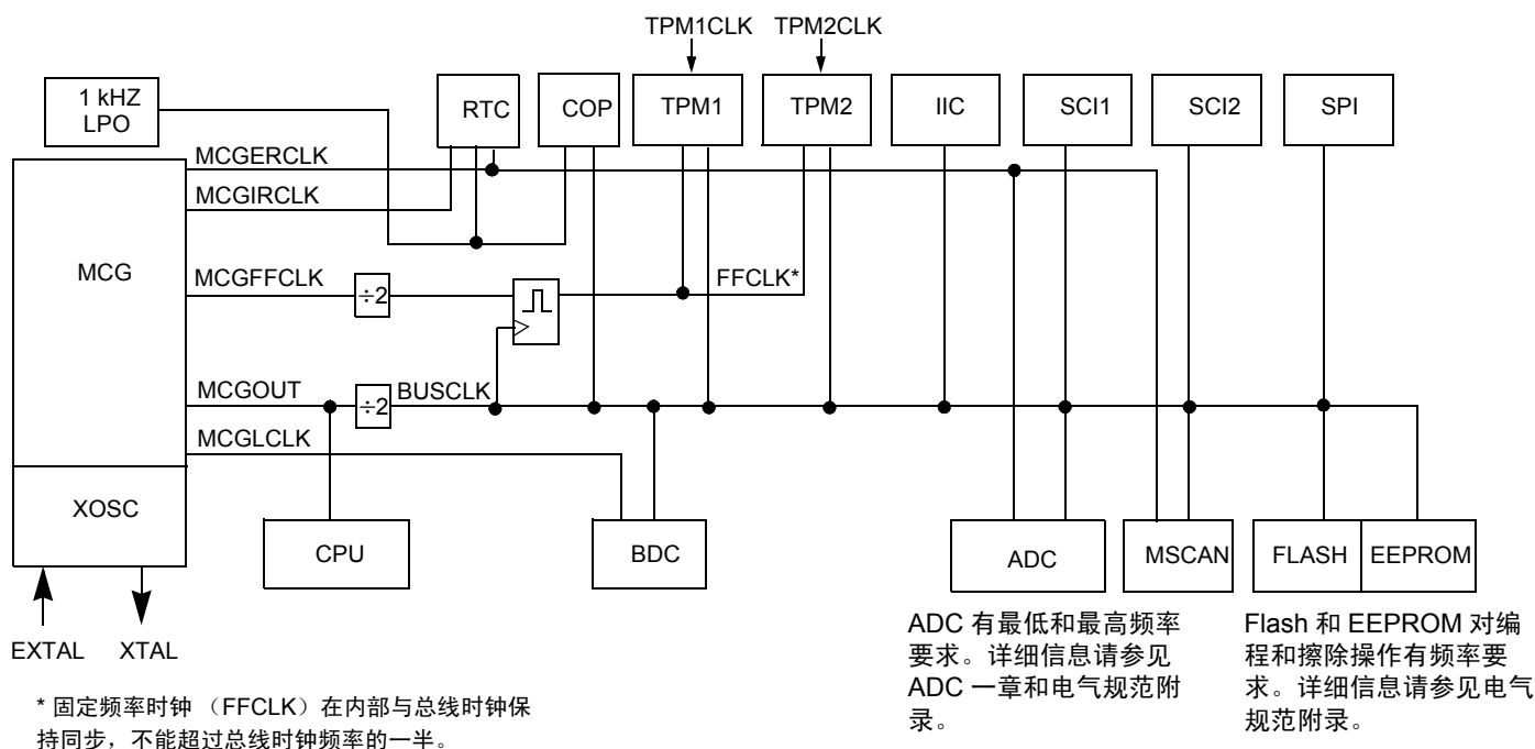
Figure 0-2. MC9S08DZ60 系统时钟分配图
