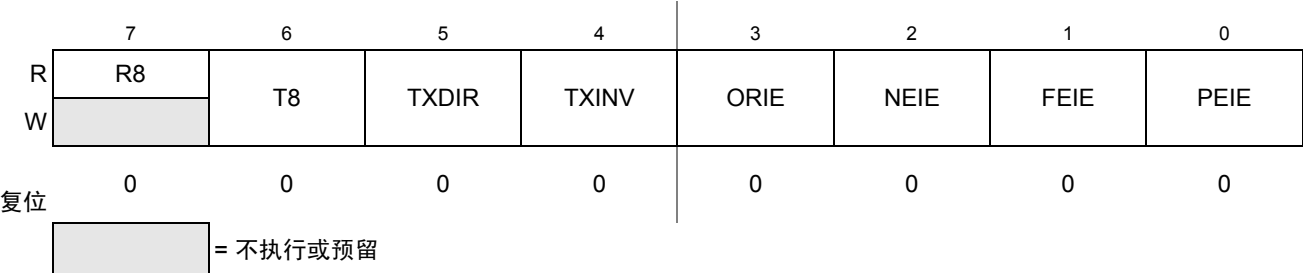
Figure 15-10. SCI 控制寄存器 3 (SCIxC3)
