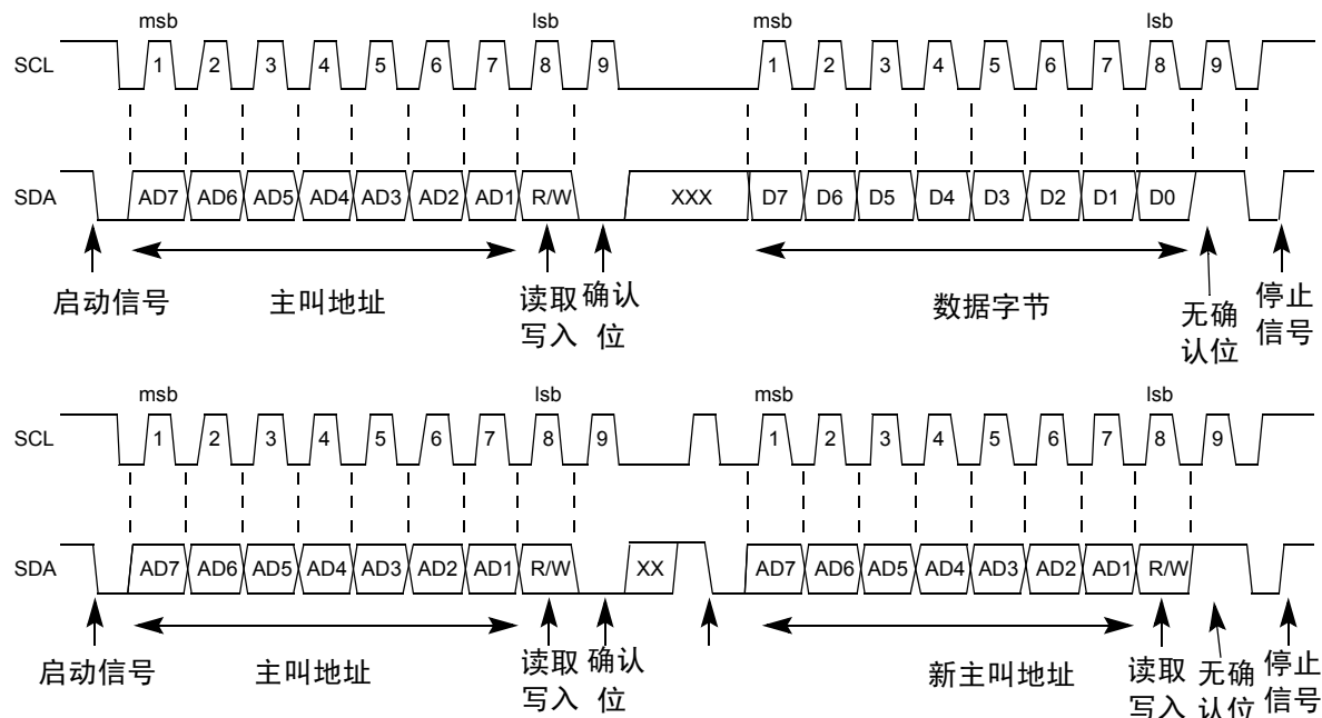
Figure 12-9. IIC 总线传输信号
