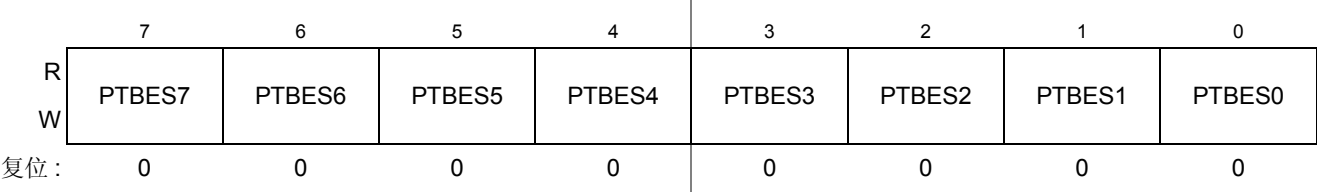
Figure 0-44. B 端口边沿选择寄存器 (PTBES)
