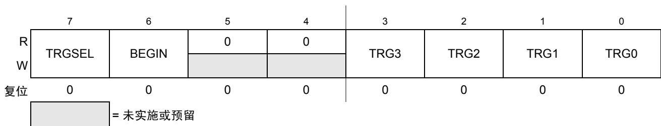
Figure 18-8. 调试触发寄存器 (DBGT)
