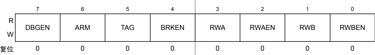
Figure 18-7. 调试控制寄存器 (DBGC)
