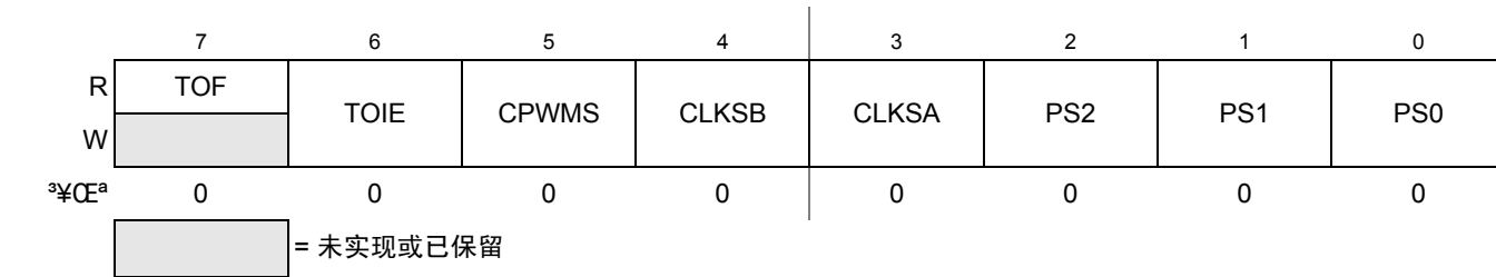
Figure 18-11. 定时器状态和控制寄存器 (TPMxSC)
