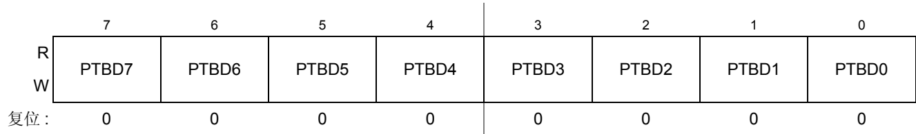
Figure 0-37. B 端口数据寄存器 (PTBD)
