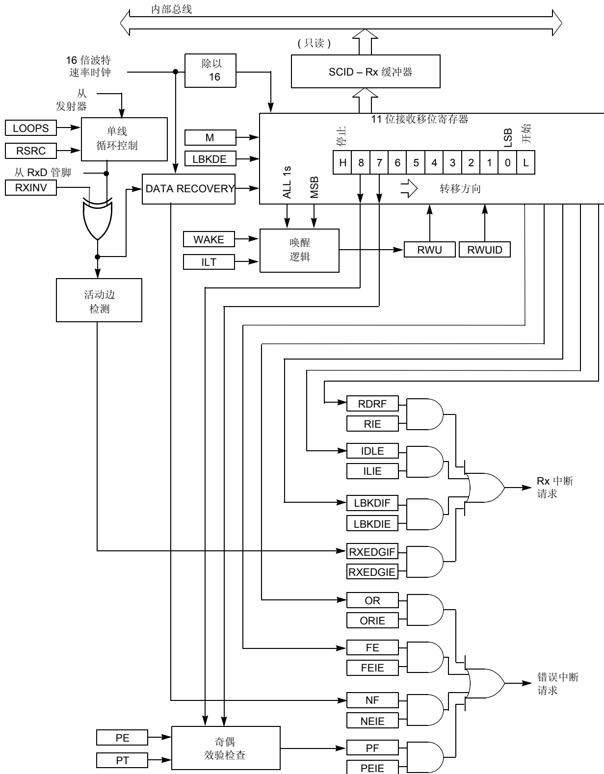
Figure 15-3. SCI 接收器结构图
