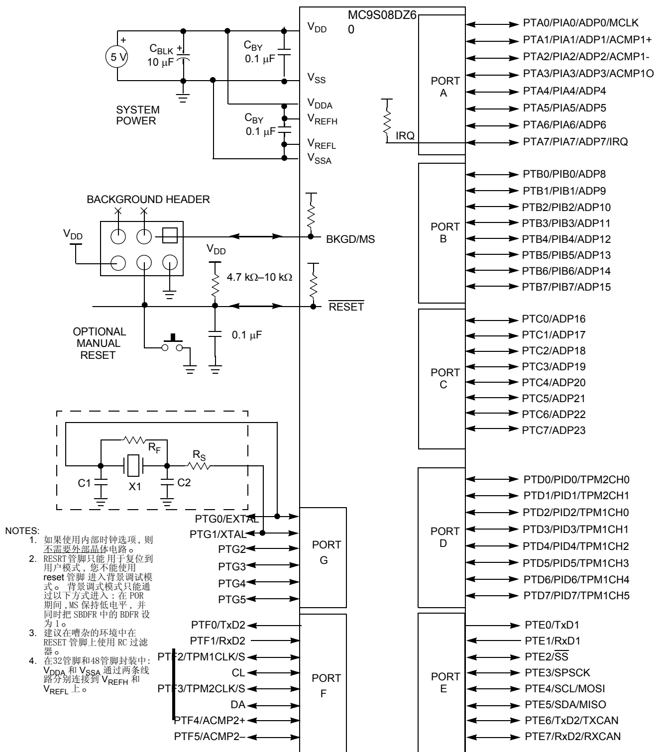
Figure 0-6. 基本系统连接 (显示的为 64 管脚封装)
