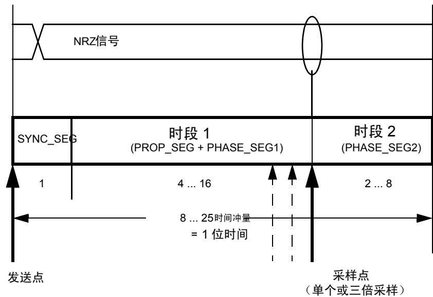
Figure 13-46. 位时间内的段
