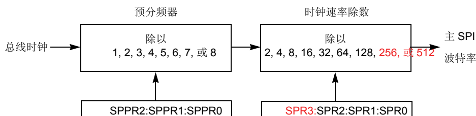
Figure 14-4. SPI 波特率生成
