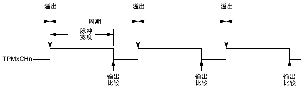
Figure 17-15. PWM 周期和脉冲宽度 (ELSnA=0)
