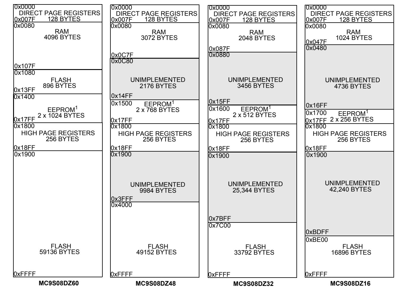
Figure 0-7. MC9S08DZ60 存储器图
