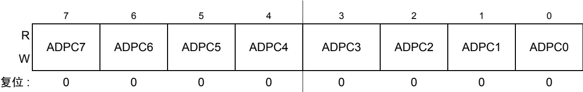
Figure 11-10. 管脚控制寄存器 1（APCTL1）
