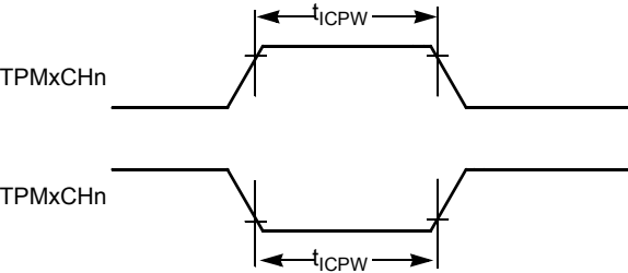
Figure B-6. 定时器输入捕捉脉冲
