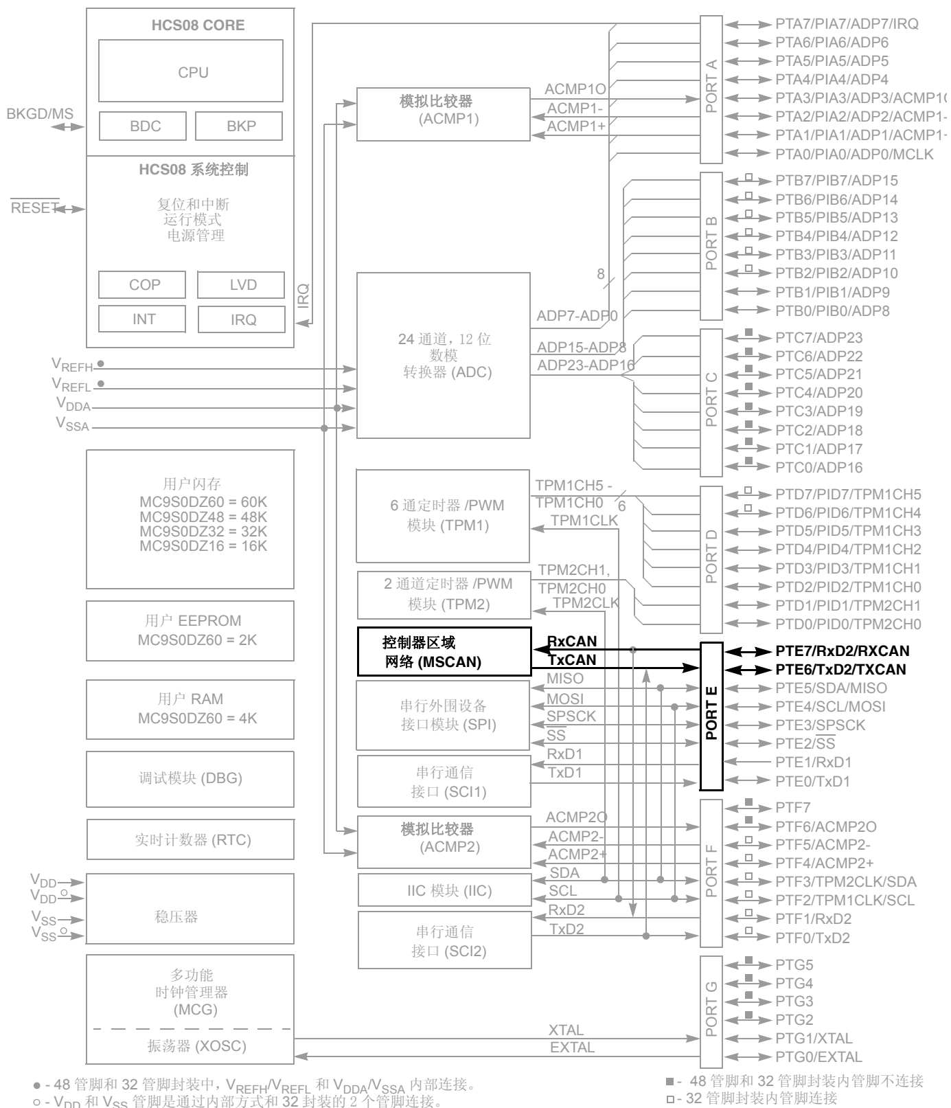
Figure 13-1. MC9S08DZ60 结构图
