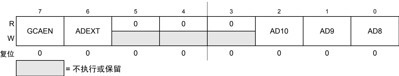
Figure 12-8. IIC 控制寄存器（IICC2）
