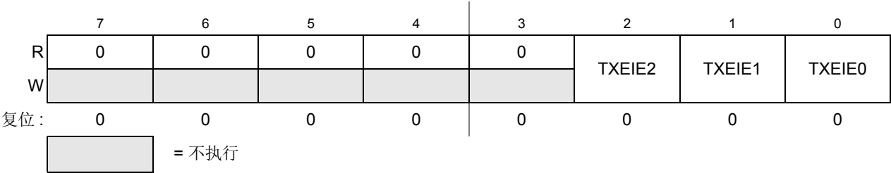
Figure 13-11. MSCAN 发送器中断使能寄存器 (CANTIER)
