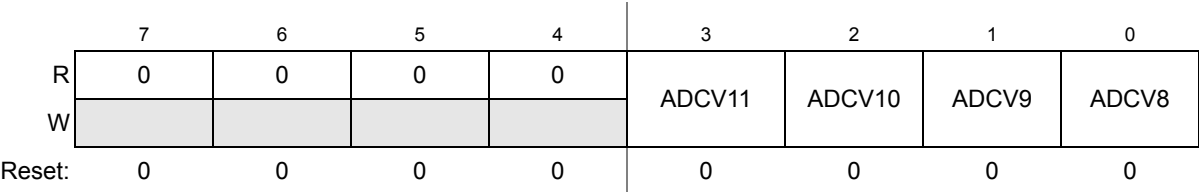
Figure 11-7. 比较值高态寄存器（ADCCVH）
