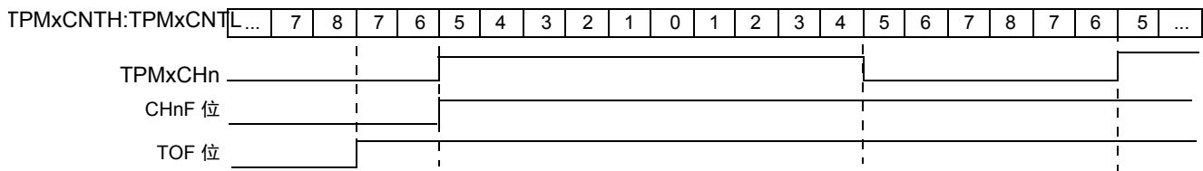
Figure 17-5. 中央对齐 PWM 的 High-True 脉冲
