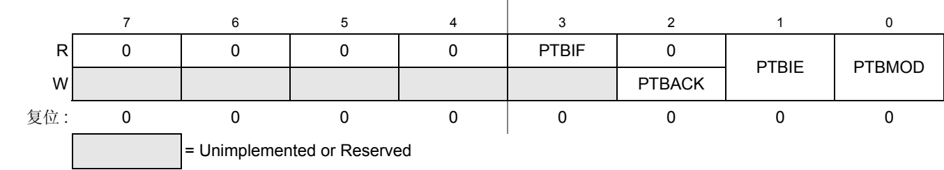
Figure 0-42. B 端口中断状态和控制寄存器 (PTBSC)
