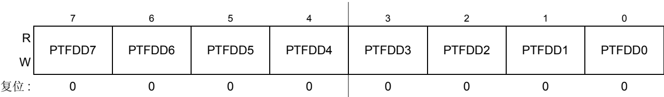
Figure 0-64. F 端口数据方向寄存器 (PTFDD)
