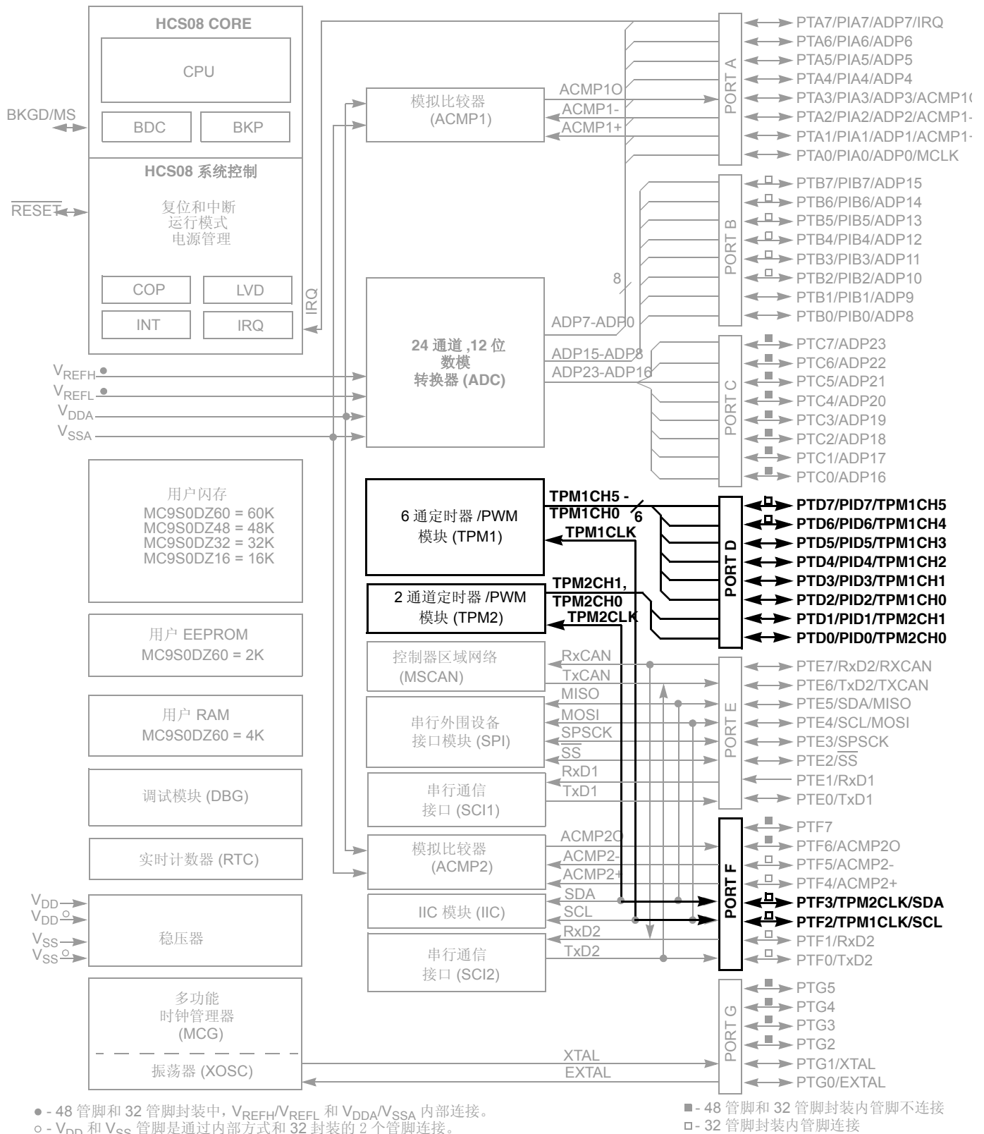
Figure 16-7. MC9S08DZ60 结构图
