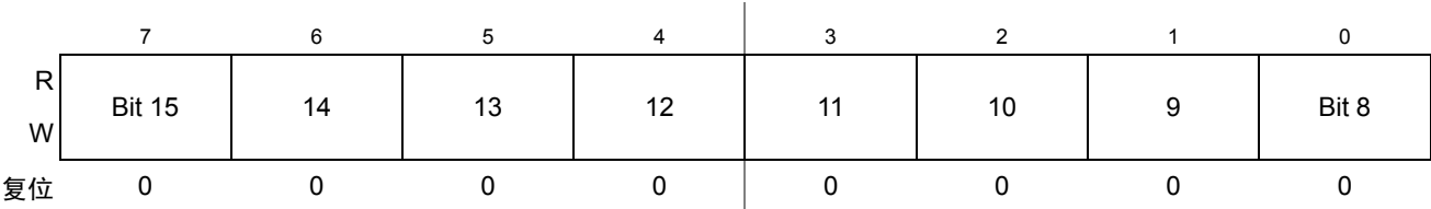
Figure 18-17. 定时器通道值寄存器高 (TPMxCnVH)
