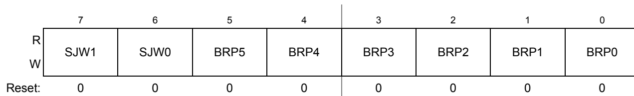
Figure 13-6. MSCAN 总线计时寄存器 0(CANBTR0)
