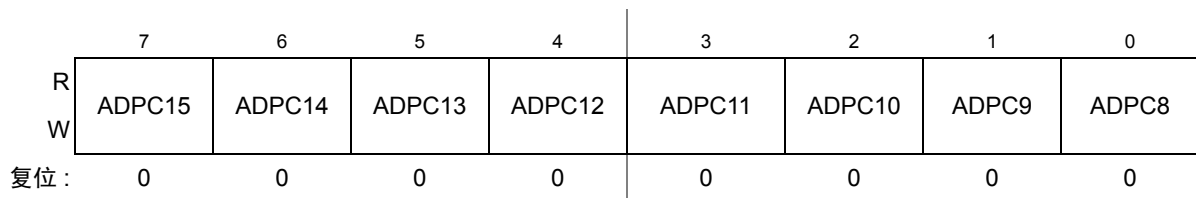
Figure 11-11. 管脚控制寄存器 2 (APCTL2)
