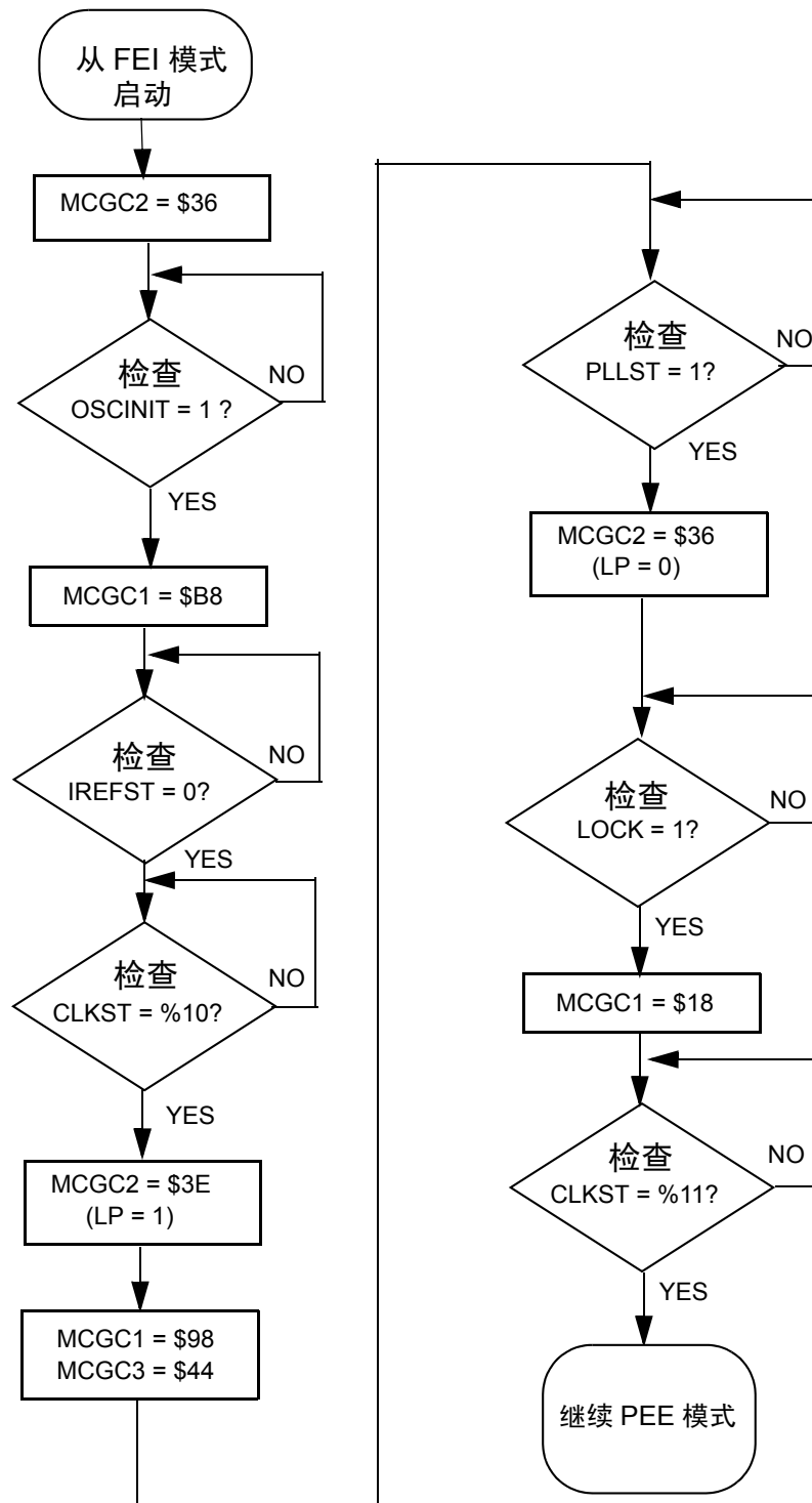
Figure 9-12. 使用 8 MHz 晶体从 FEI 转换到 PEE 模式的流程图
