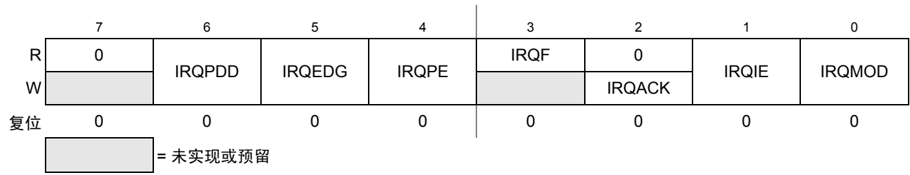
Figure 0-18. 中断请求状态和控制寄存器 (IRQSC)
