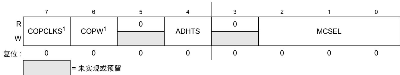
Figure 0-22. 系统选项寄存器 2 (SOPT2)
