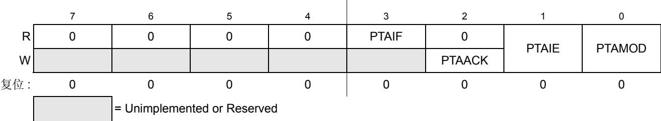
Figure 0-34. A 端口中断状态和控制寄存器 (PTASC)
