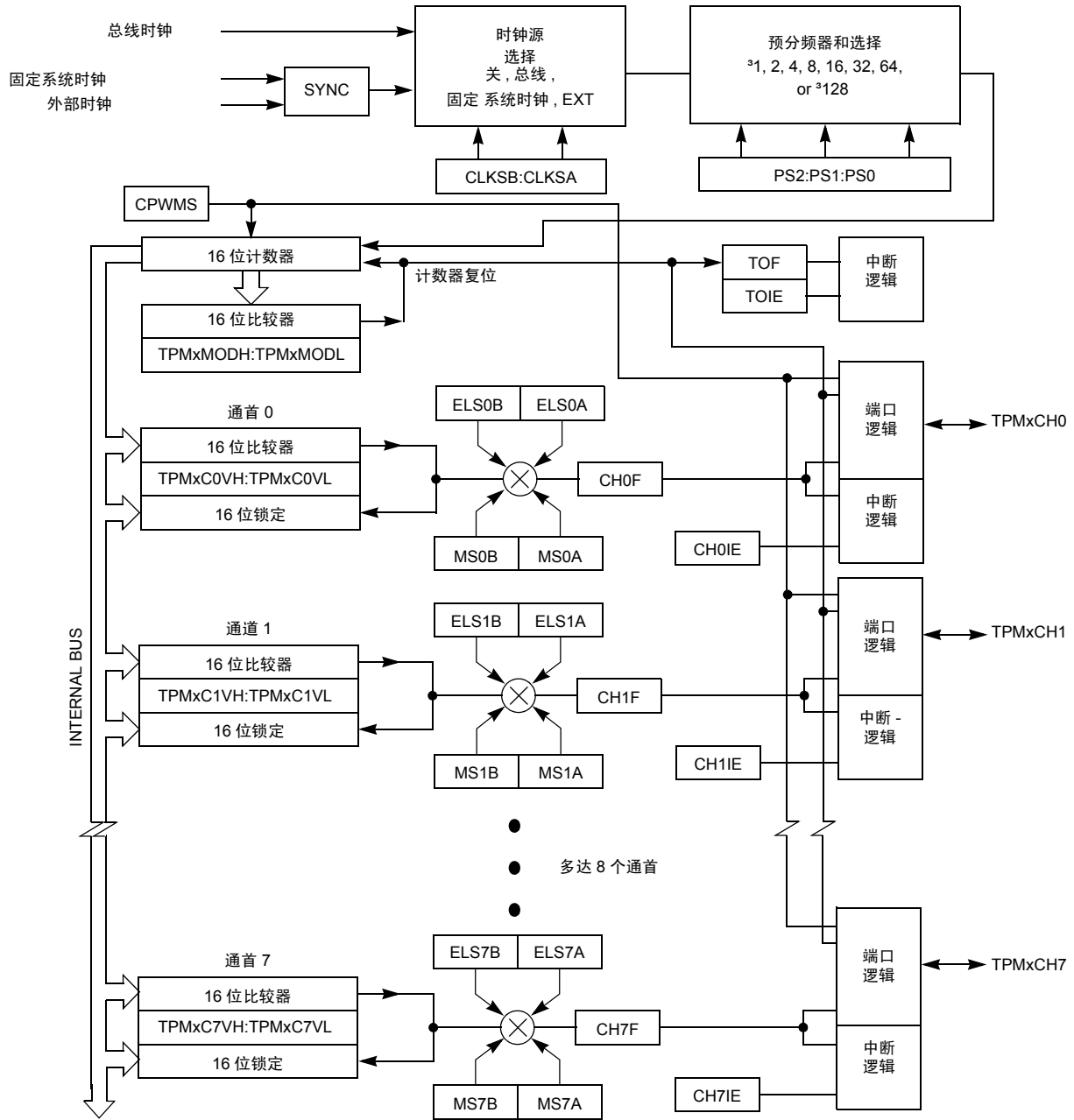
Figure 17-2. TPM 结构图
