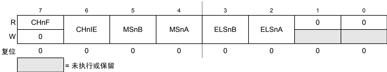
Figure 17-12. TPM 通道 n 状态和控制寄存器（TPMxCnSC）
