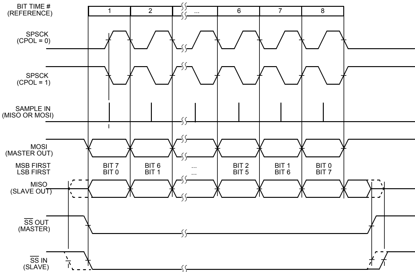
Figure 14-11. SPI 时钟格式 (CPHA = 0)
