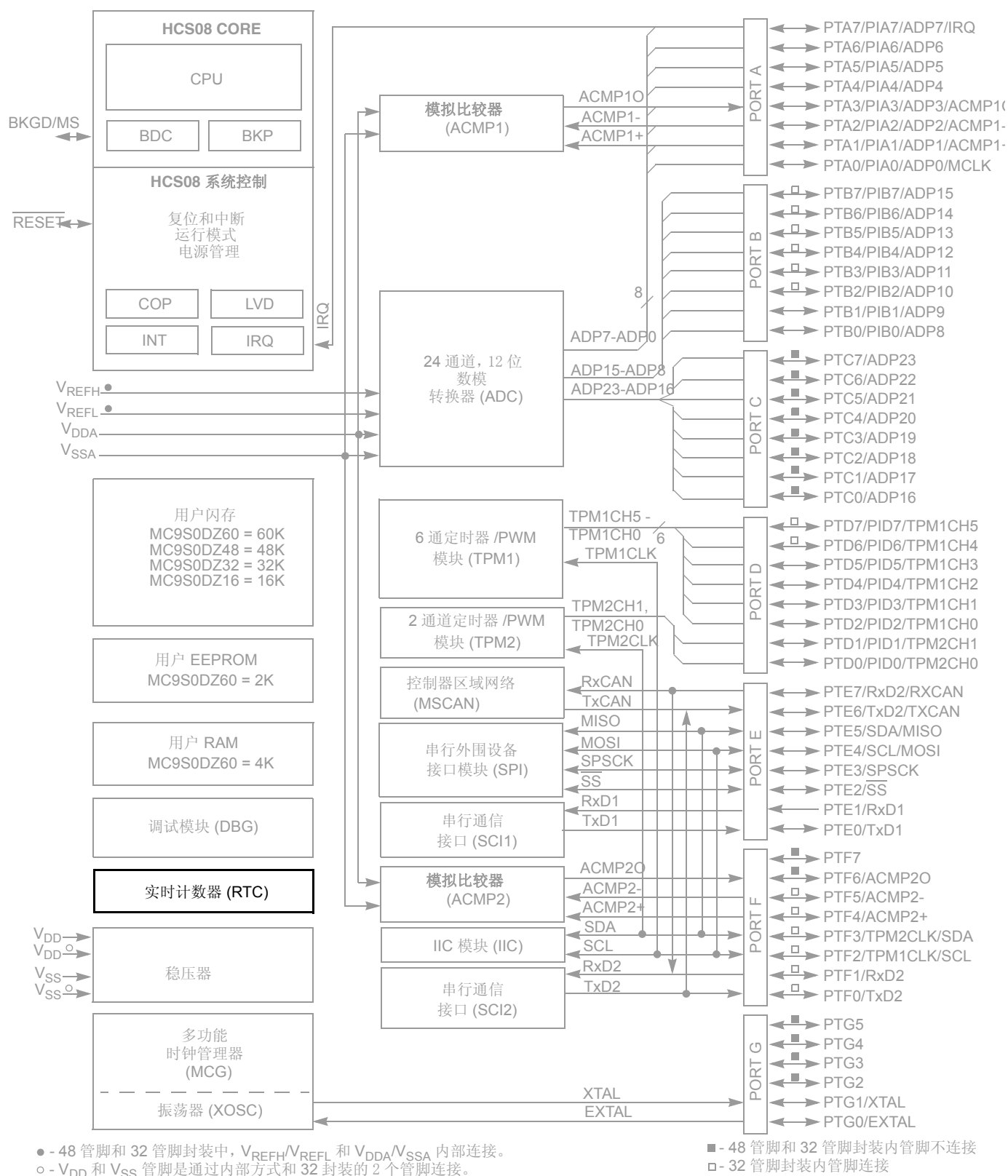
Figure 16-1. MC9S08DZ60 结构图
