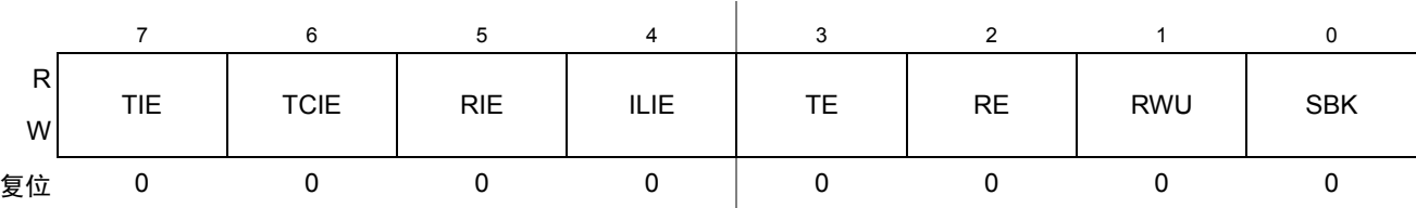
Figure 15-7. SCI 控制寄存器 2 (SCIxC2)
