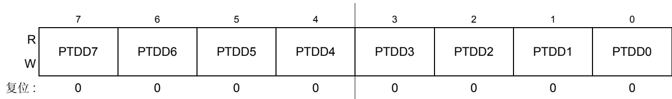
Figure 0-50. D 端口数据寄存器 (PTDD)
