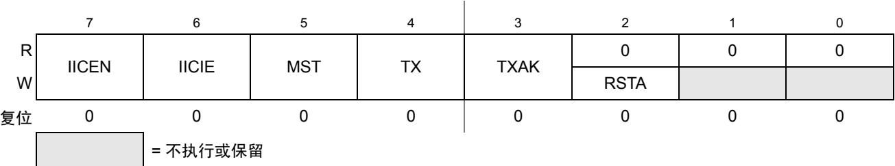
Figure 12-5. IIC 控制寄存器（IICC1）
