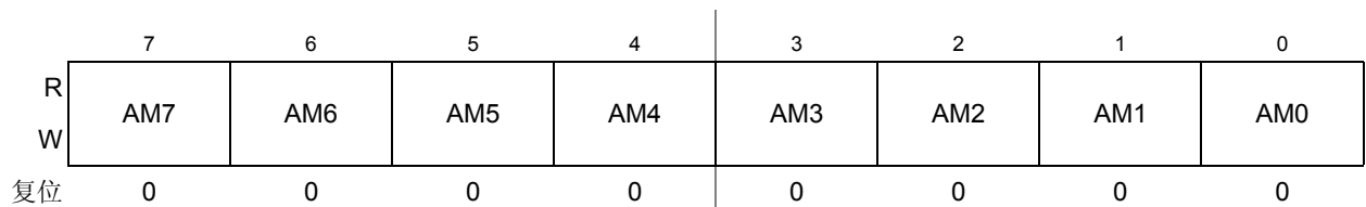
Figure 13-21. MSCAN 标识符掩码寄存器（第一页）— CANIDMR0–CANIDMR3
