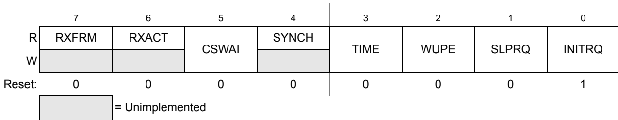
Figure 13-4. 控制寄存器 0 (CANCTL0)
