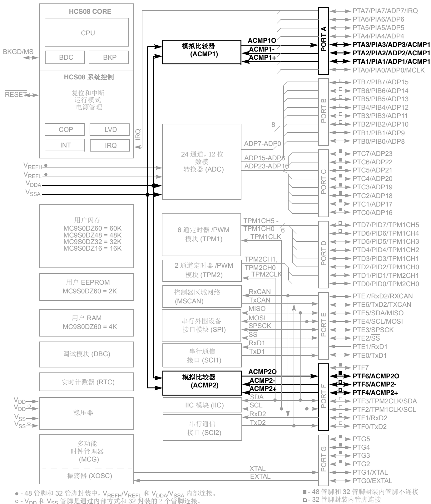
Figure 10-1. MC9S08DZ60 结构图
