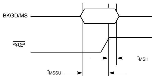
Figure B-3. 激活背景调试模式锁定时序
