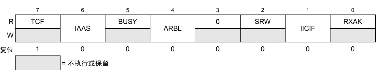
Figure 12-6. IIC 状态寄存器（IICS）
