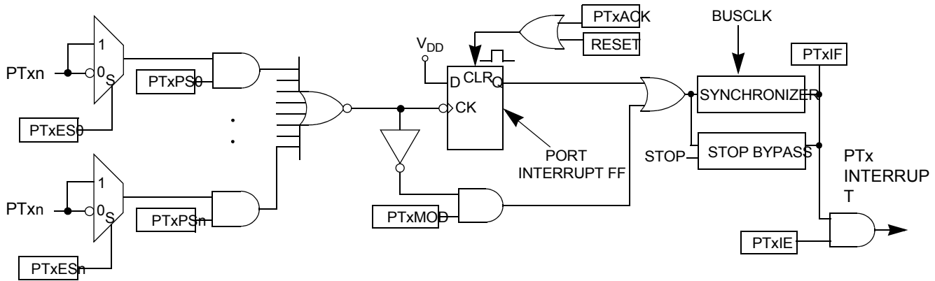
Figure 0-28. 端口中断示意图
