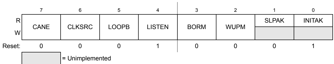
Figure 13-5. 控制寄存器 1(CANCTL1)
