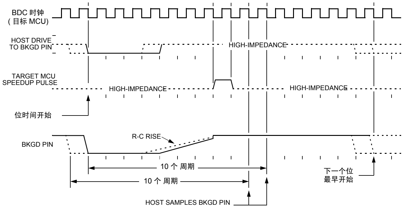
Figure 18-3. BDC 目标 - 到 - 主机串行位时序 (逻辑 1)
