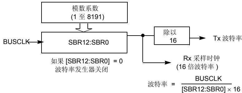
Figure 15-12. SCI 波特率生成
