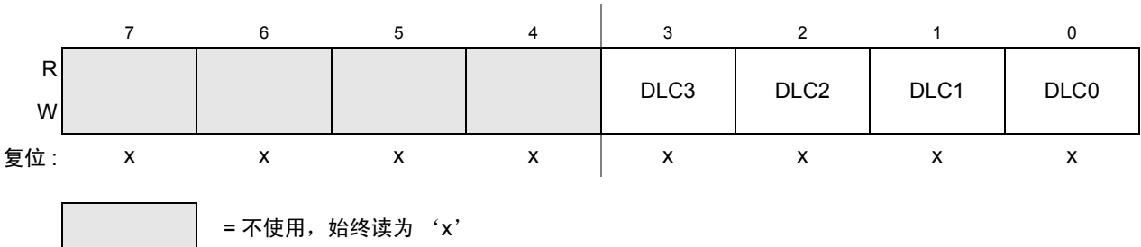
Figure 13-37. 数据长度寄存器（DLR）— 扩展标识符映射
