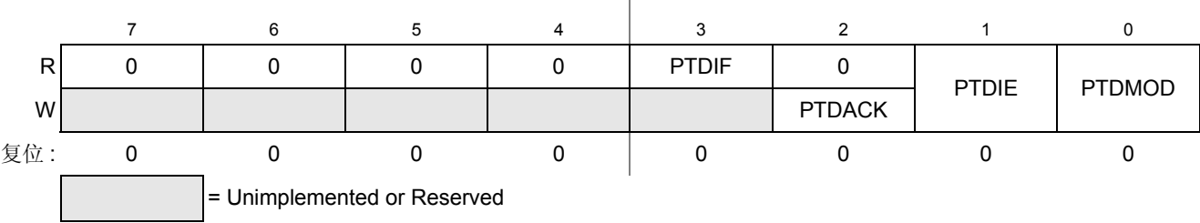
Figure 0-55. D 端口中断状态和控制寄存器 (PTDSC)
