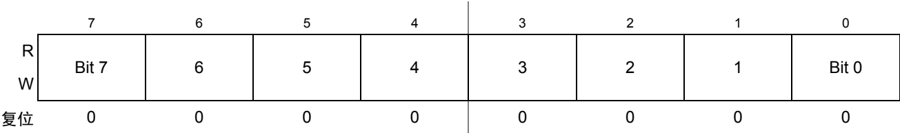
Figure 14-9. SPI 数据寄存器 (SPID)
