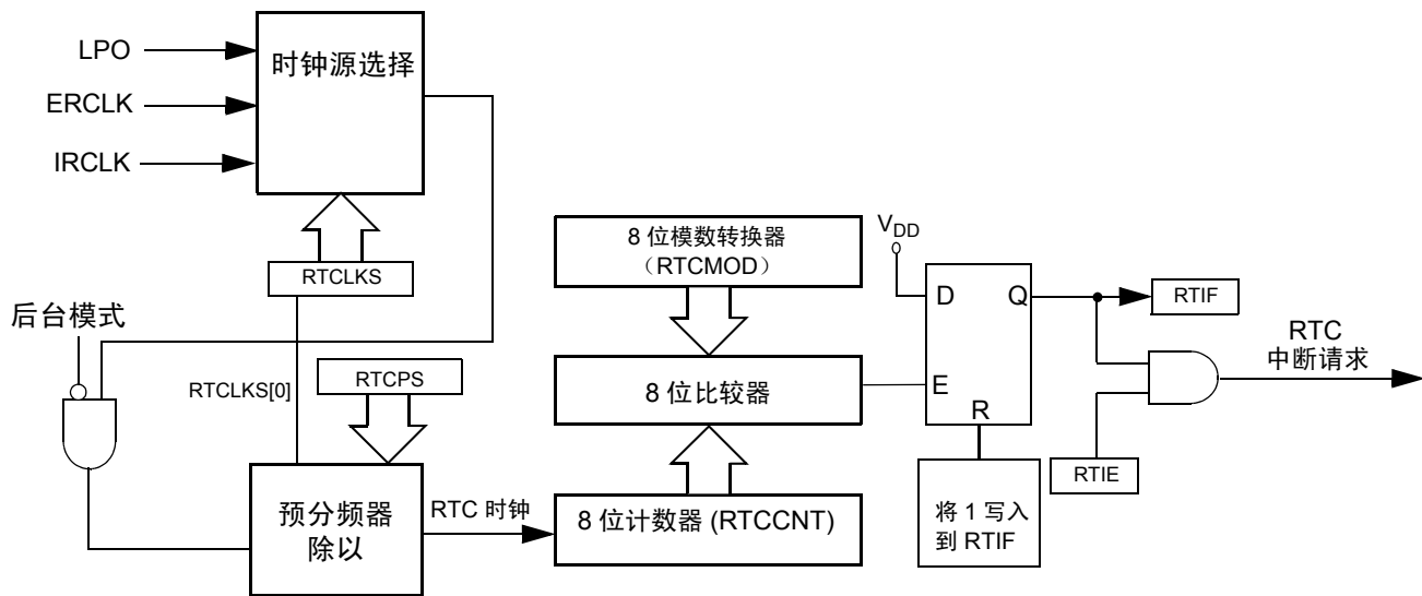
Figure 16-2. 实时计数器（RTC）结构图
