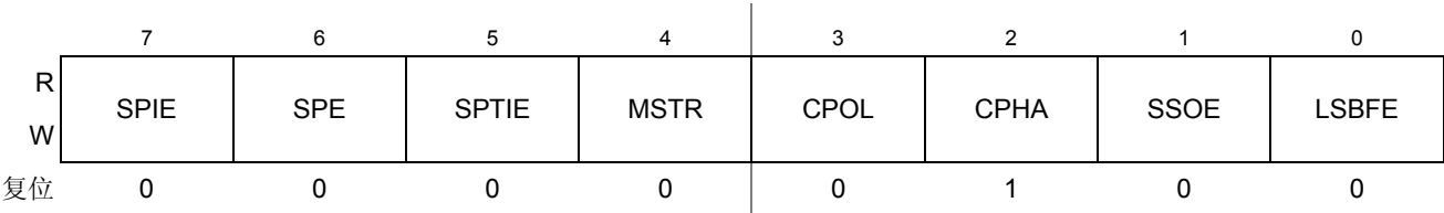
Figure 14-5. SPI 控制寄存器 1 (SPIC1)
