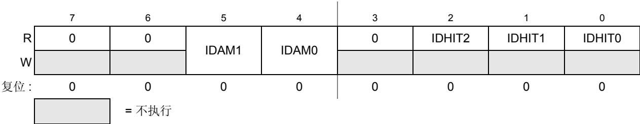
Figure 13-15. MSCAN 标识符验收控制寄存器 r (CANIDAC)
