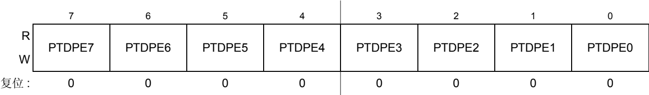
Figure 0-52. D 端口寄存器内部上拉使能 (PTDPE)
