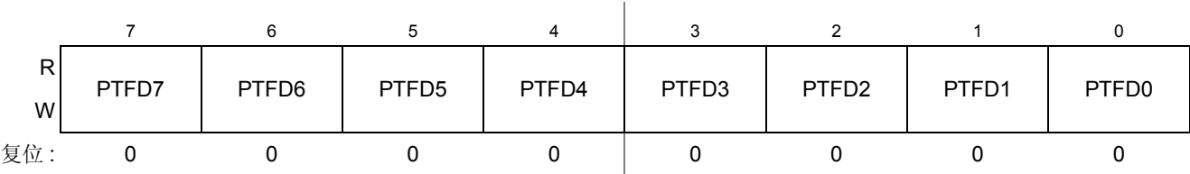
Figure 0-63. F 端口数据寄存器 (PTFD)
