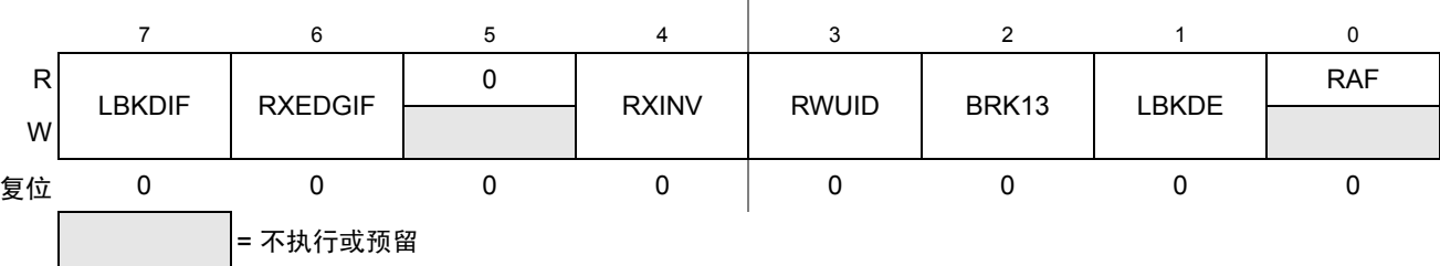
Figure 15-9. SCI 状态寄存器 2 (SCIS2)
