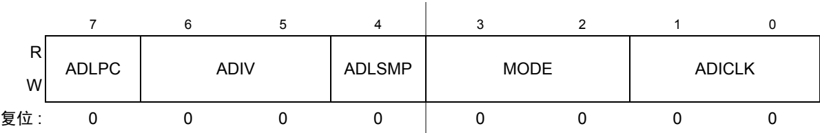
Figure 11-9. 配置寄存器（ADCCFG）
