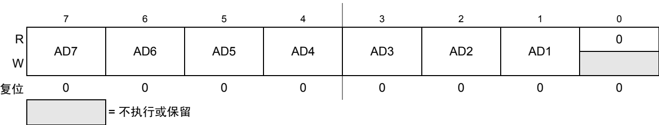
Figure 12-3. IIC 地址寄存器 (IICA)
