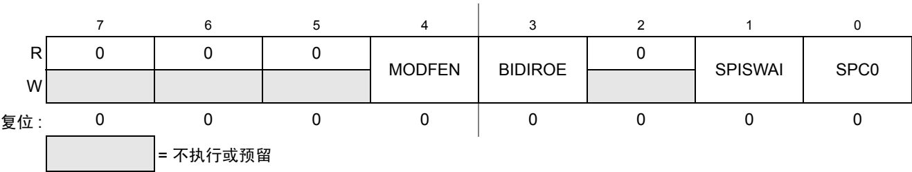
Figure 14-6. SPI 控制寄存器 2 (SPIC2)
