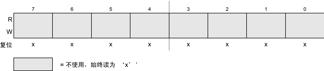
Figure 13-34. 标识符寄存器 2 —标准映射
