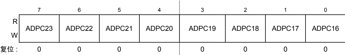
Figure 11-12. 管脚控制寄存器 3（APCTL3）
