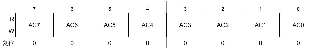
Figure 13-19. MSCAN 标识符接收寄存器 (第一页) — CANIDAR0-CANIDAR3
