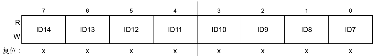
Figure 13-30. 标识符寄存器 2 (IDR2) — 扩展标识符映射
