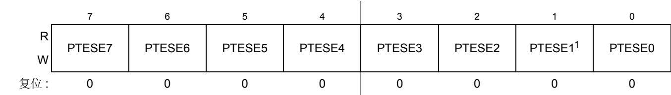
Figure 0-61. E 端口寄存器斜率使能 (PTESE)
