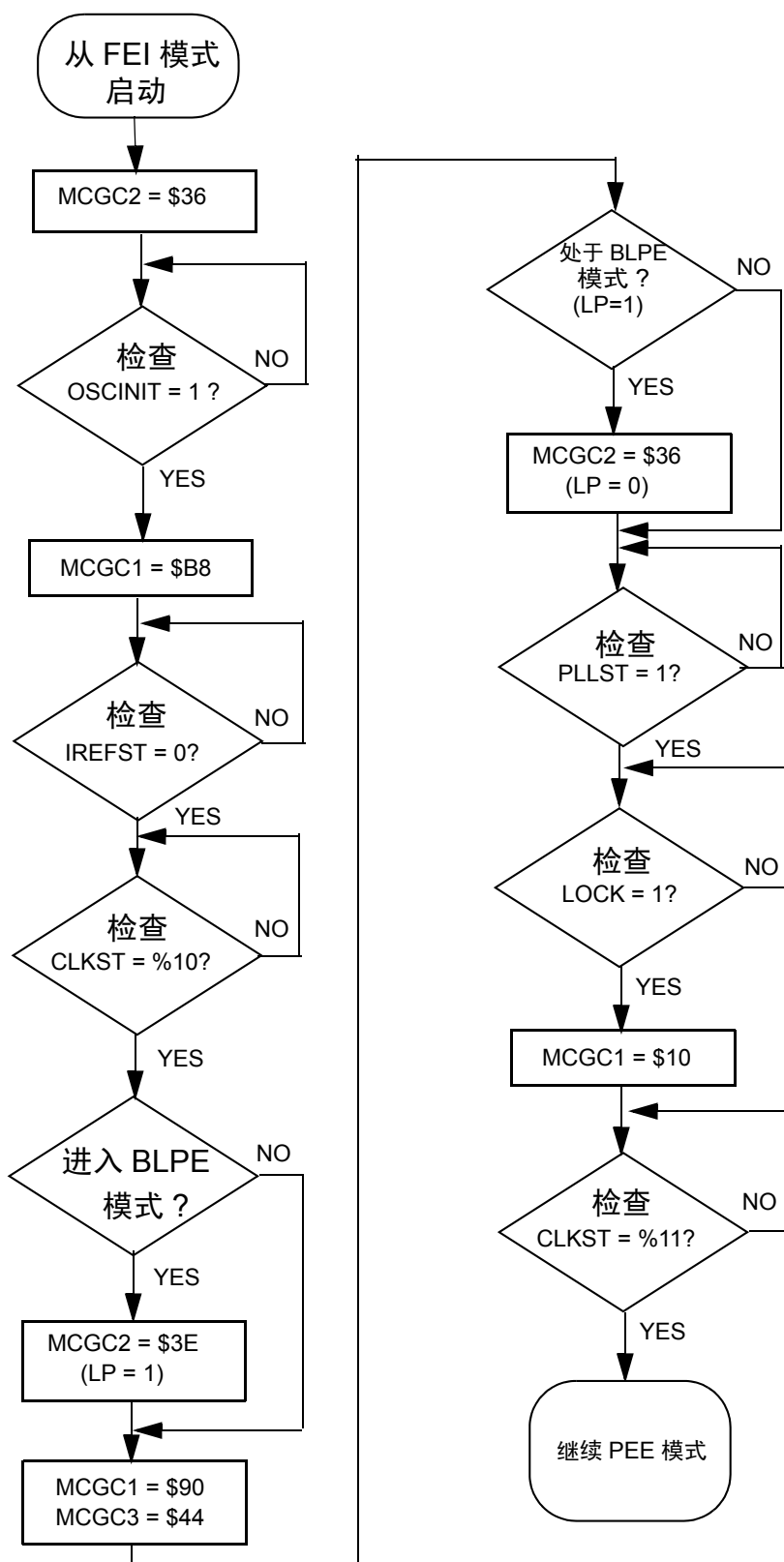
Figure 9-9. 使用 4 MHz 晶体从 FEI 转换到 PEE 模式的流程图
