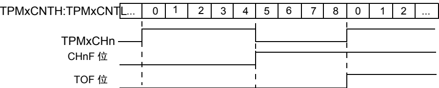
Figure 17-3. 边缘对齐 PWM 的 High-True 脉冲
