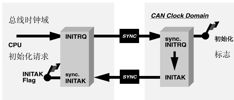
Figure 13-49. 初始化请求 / 确认周期
