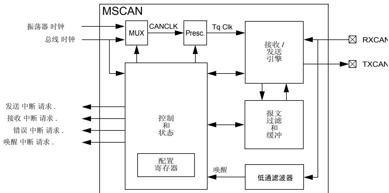
Figure 13-2. MSCAN 结构图
