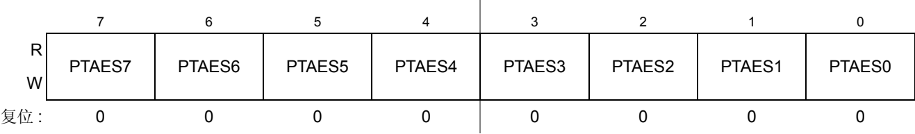
Figure 0-36. A 端口边沿选择寄存器 (PTAES)
