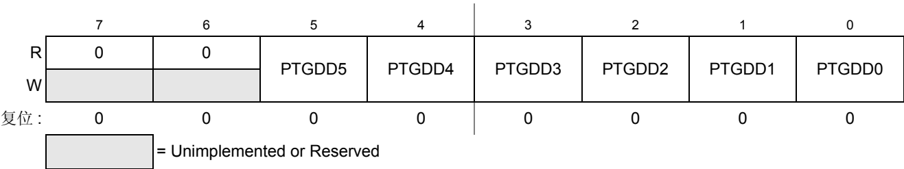
Figure 0-69. G 端口数据方向寄存器 (PTGDD)
