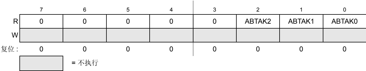
Figure 13-13. MSCAN 发送器报文中止确认寄存器 (CANTAANK)
