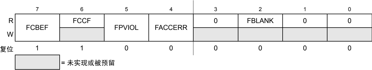
Figure 0-15. Flash 和 EEPROM 状态寄存器 (FSTAT)
