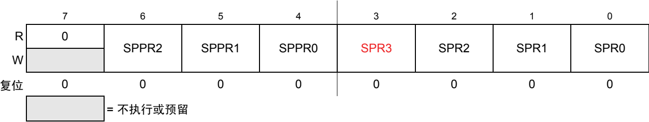
Figure 14-7. SPI 波特率寄存器 (SPIBR)
