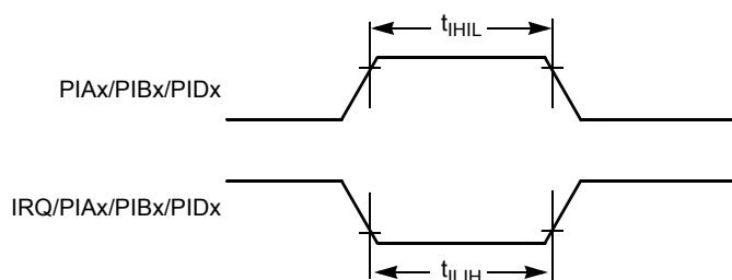
Figure B-4. 管脚中断时序
