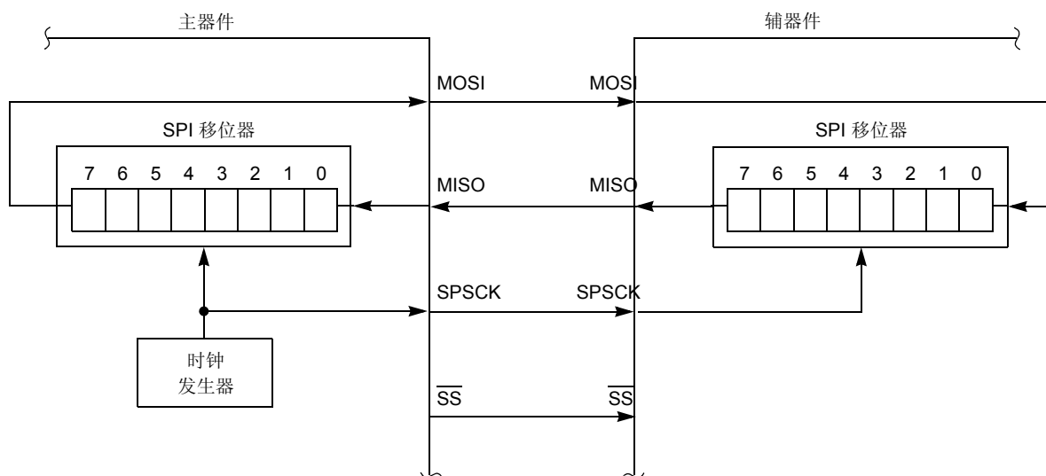
Figure 14-2. SPI 系统连接
