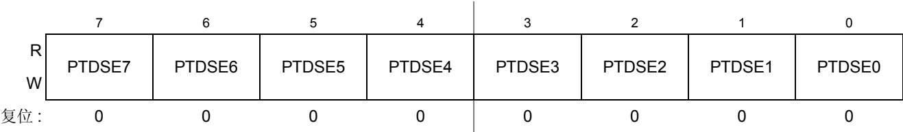
Figure 0-53. D 端口寄存器斜率使能 (PTDSE)
