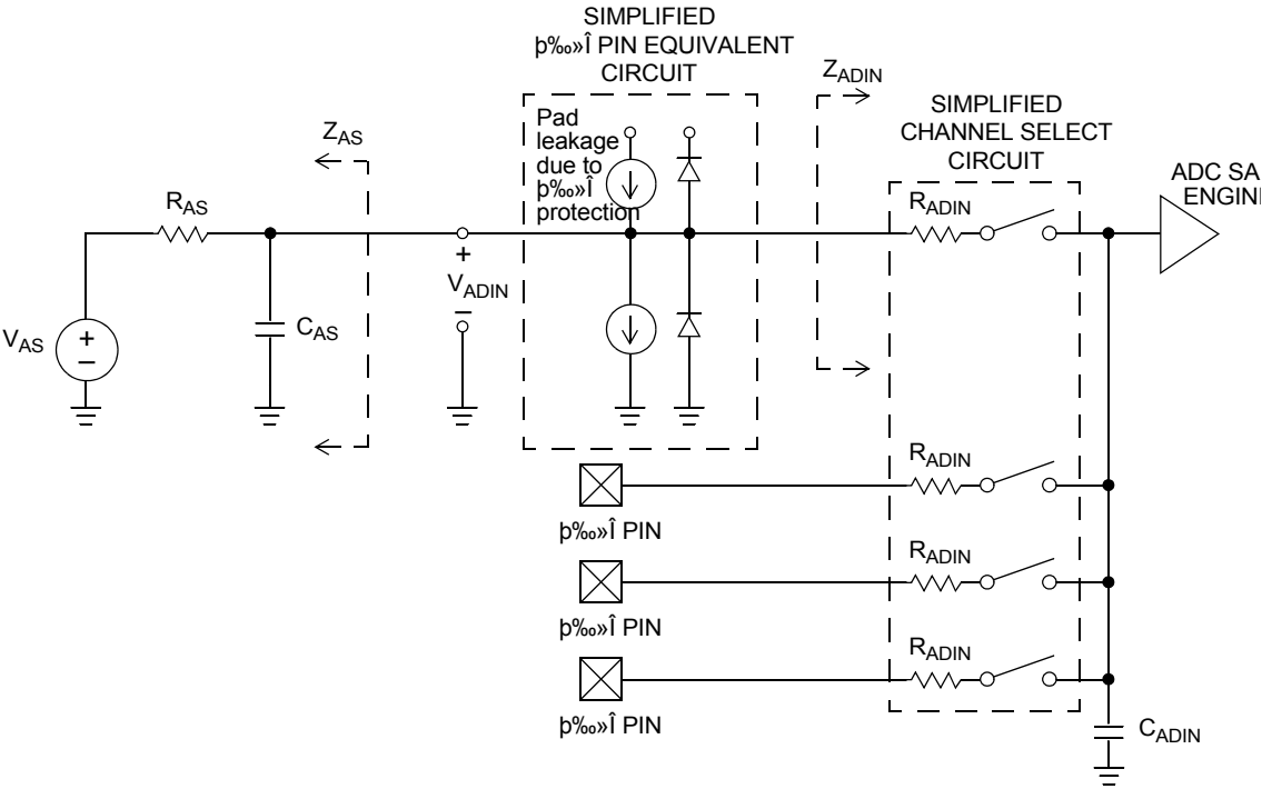
Figure B-1. ADC 输入抗阻等效示意图
