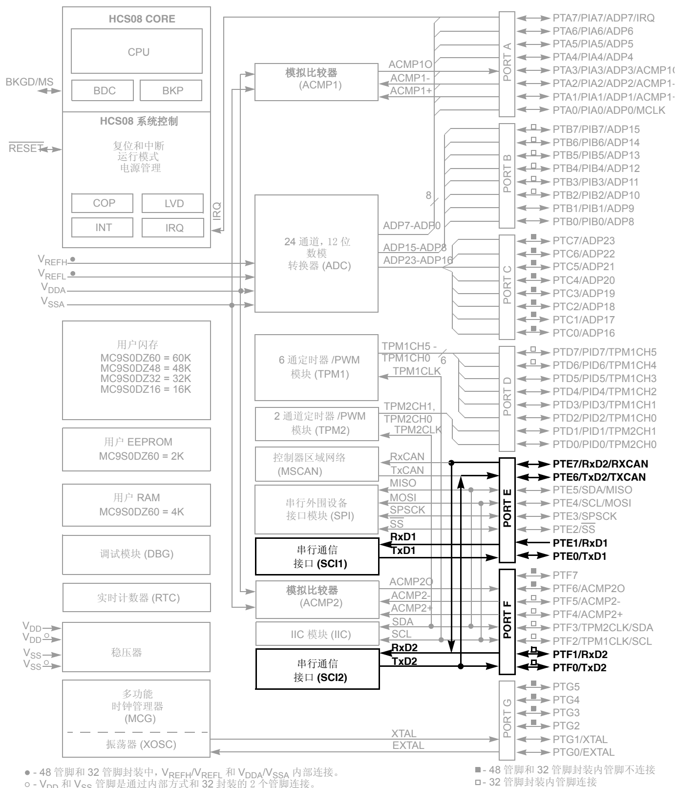
Figure 15-1. MC9S08DZ60 结构图
