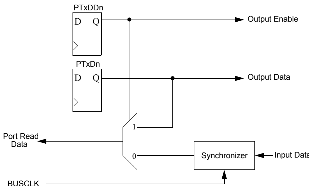
Figure 0-27. 并行输入 / 输出示意图
