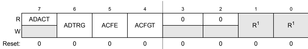
Figure 11-4. 状态和控制寄存器 2 (ADCSC2)
