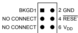
Figure 18-1. 工具接口
