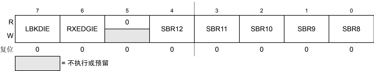
Figure 15-4. SCI 波特率寄存器 (SCIxBDH)
