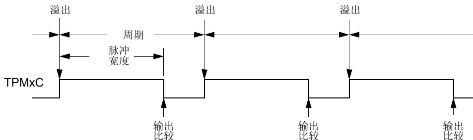
Figure 18-19. PWM 周期和脉冲宽度 (ELSnA = 0)
