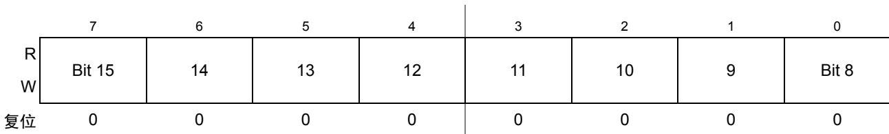
Figure 17-10. TPM 计数器模数寄存器高字节（TPMxMODH）
