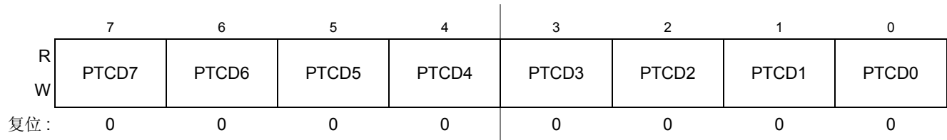
Figure 0-45. C 端口数据寄存器 (PTCD)
