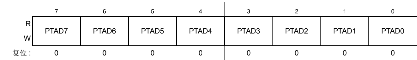
Figure 0-29. A 端口数据寄存器 (PTAD)
