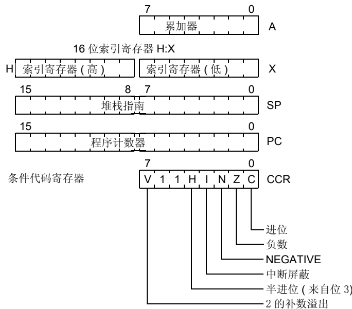
Figure 8-1. CPU 寄存器
