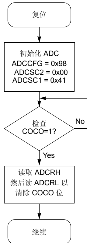
Figure 11-13. 初始化流程图示例
