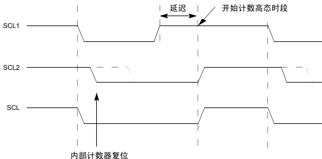
Figure 12-10. IIC 时钟同步
