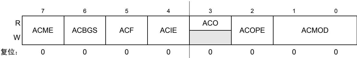
Figure 10-3. ACMPx 状态和控制寄存器 (ACMPxSC)
