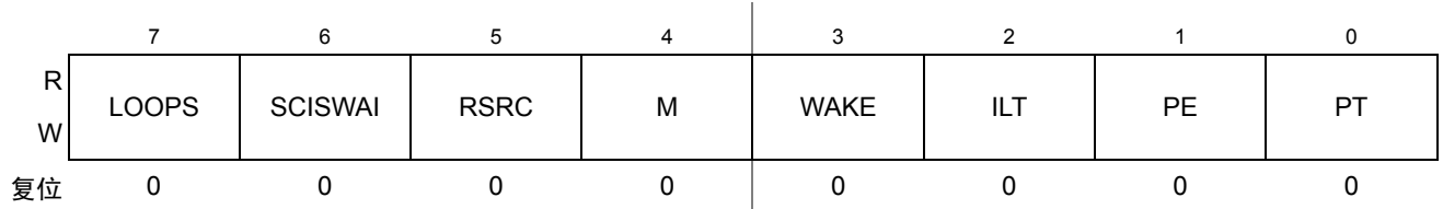
Figure 15-6. SCI 控制寄存器 1 (SCIxC1)
