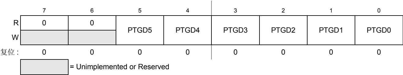
Figure 0-68. G 端口数据寄存器 (PTGD)
