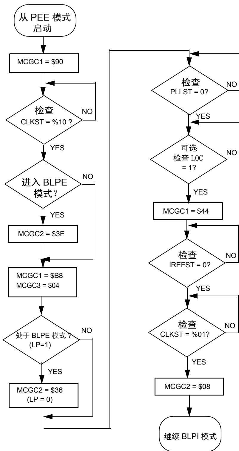
Figure 9-10. 使用 4 MHz 晶体从 PEE 转换到 BLPI 模式的流程图
