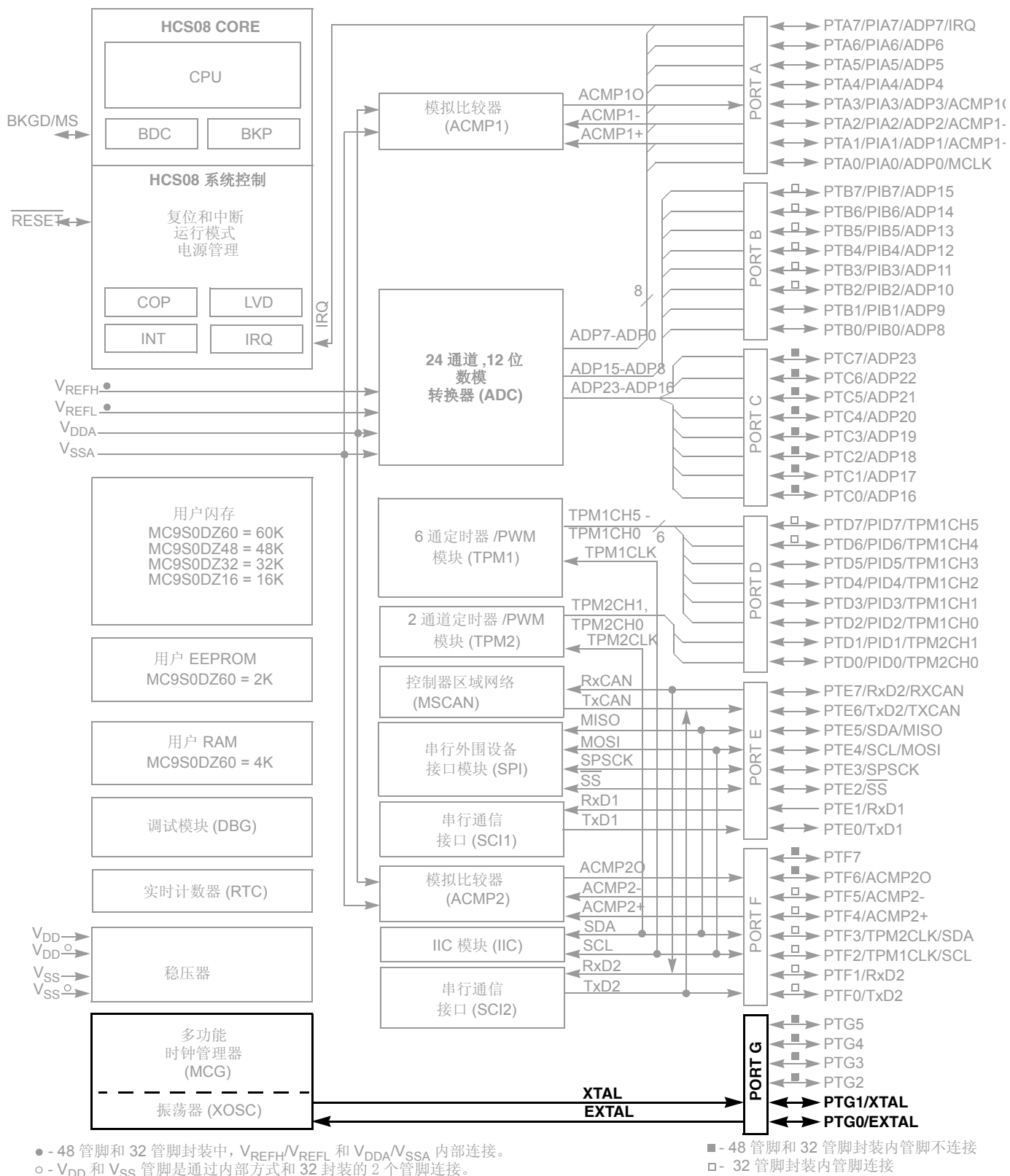
Figure 8-3. MC9S08DZ60 结构图
