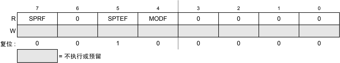
Figure 14-8. SPI 状态寄存器 (SPIS)
