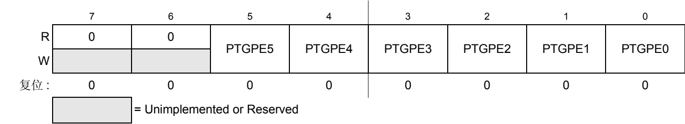
Figure 0-70. G 端口寄存器内部上拉使能 (PTGPE)
