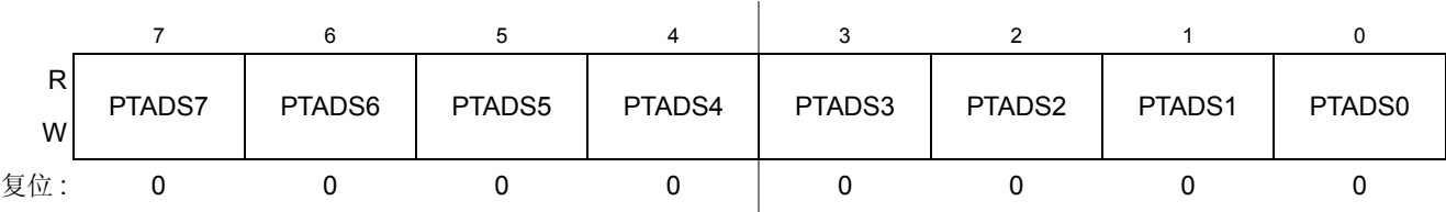
Figure 0-33. A 端口寄存器的驱动强度选择 (PTADS)
