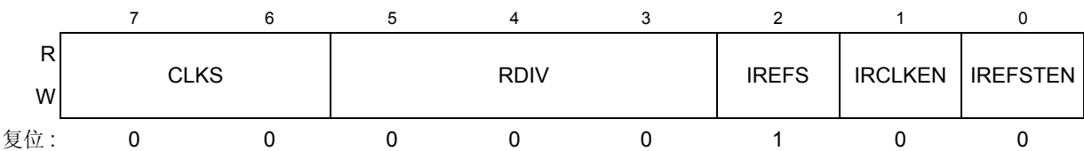
Figure 9-3. MCG 控制寄存器 1 (MCGC1)
