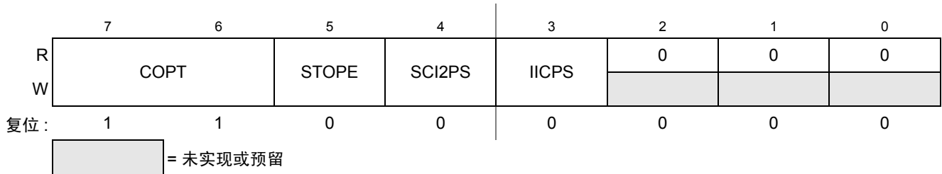
Figure 0-21. 系统选项寄存器 1 (SOPT1)
