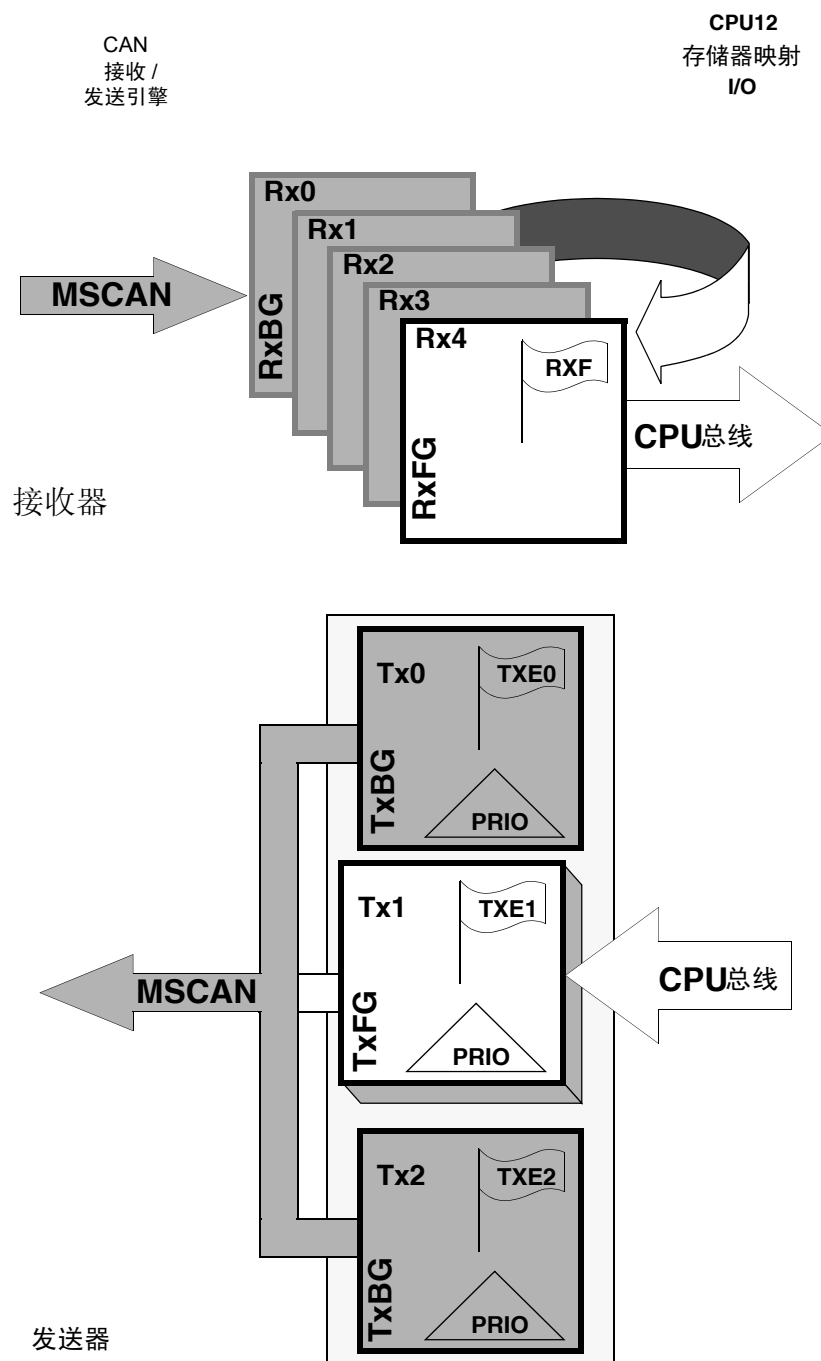
Figure 13-41. 报文缓冲器结构的用户模型
