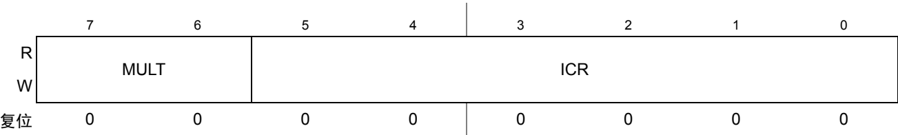
Figure 12-4. IIC 分频器寄存器 (IICF)
