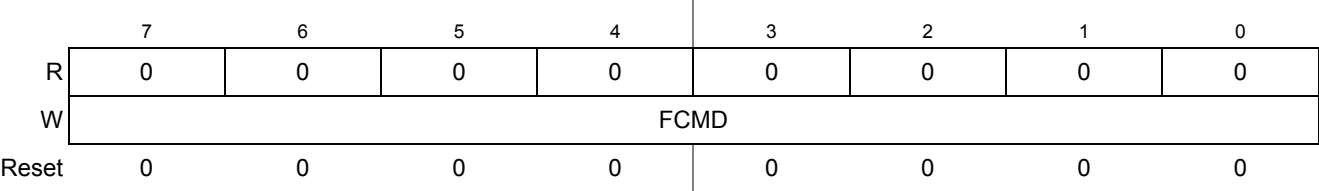
Figure 0-16. Flash 和 EEPROM 命令寄存器 (FCMD)
