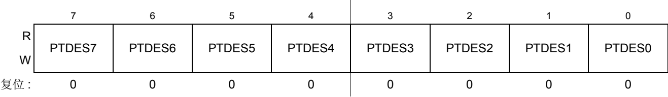
Figure 0-57. D 端口边沿选择寄存器 (PTDES)
