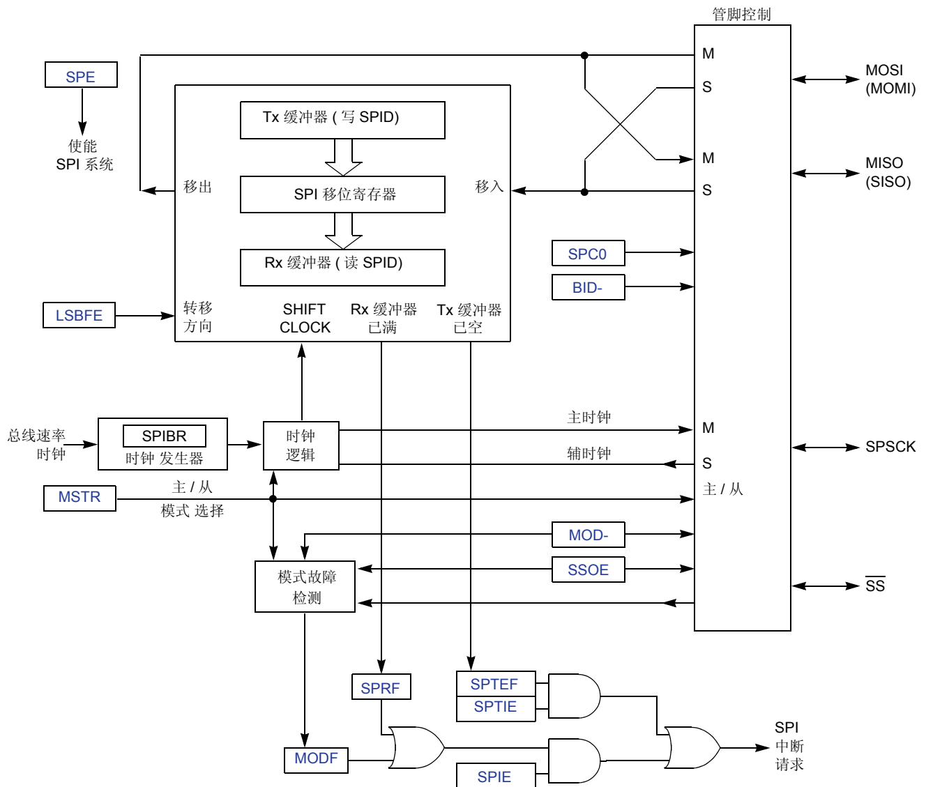
Figure 14-3. SPI 模块结构图
