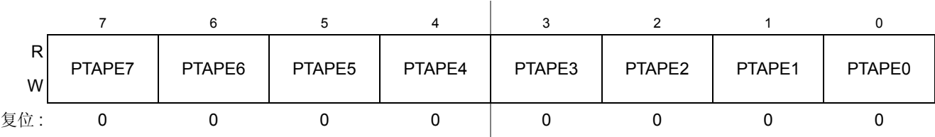
Figure 0-31. A 端口寄存器的内部上拉使能 (PTAPE)
