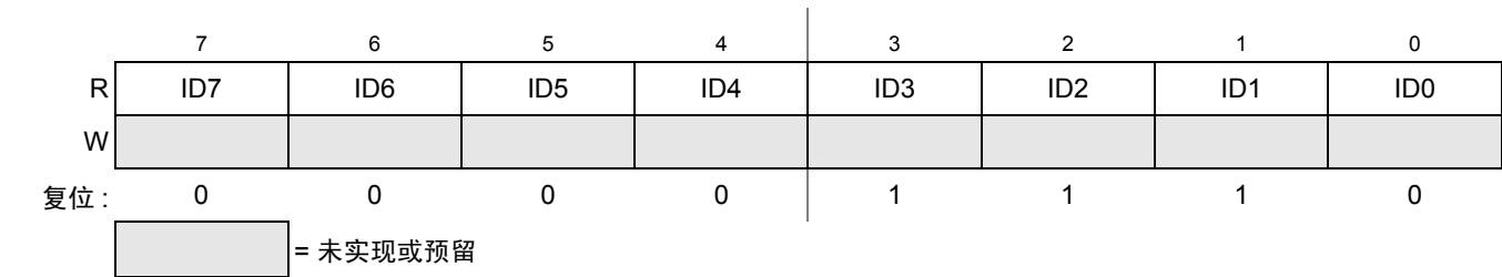
Figure 0-24. 系统器件识别寄存器 — 低 (SDIDL)
