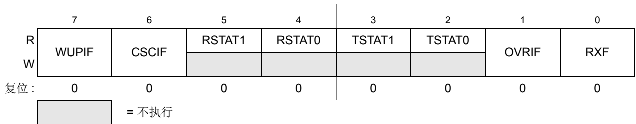
Figure 13-8. MSCAN 接收器标志寄存器 (CANRFLG)
