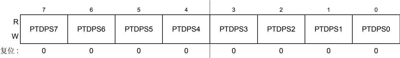
Figure 0-56. D 端口中断管脚选择寄存器 (PTDPS)
