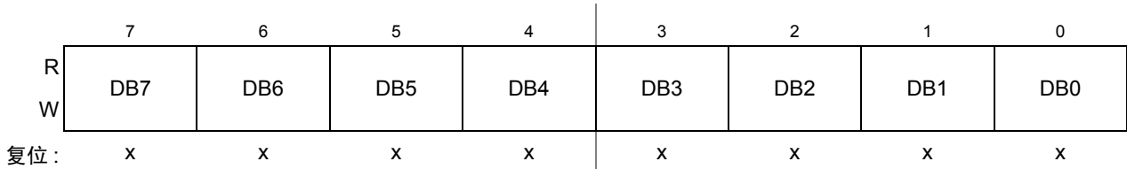
Figure 13-36. 数据段寄存器（DSR0 - DSR7）— 扩展标识符映射
