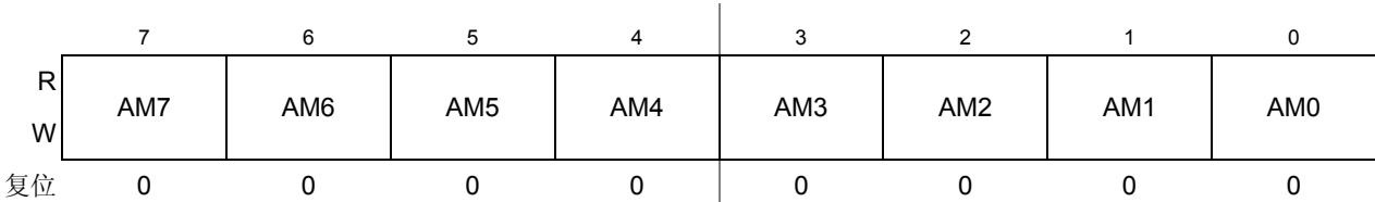
Figure 13-22. MSCAN I 标识符掩码寄存器（第二页） — CANIDMR4–CANIDMR7
