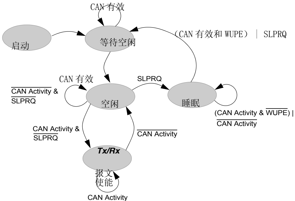
Figure 13-48. 进入 / 退出睡眠模式的简单状态 转换
