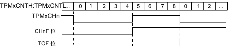
Figure 17-4. 边缘对齐 PWM 的 Low-True 脉冲
