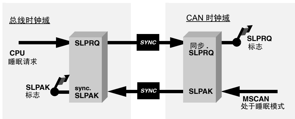
Figure 13-47. 睡眠请求 / 确认周期
