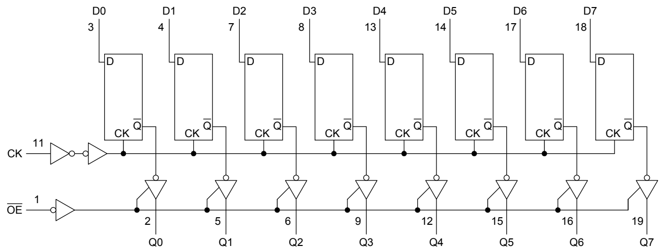
システム図
