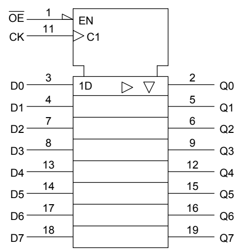
論理図
