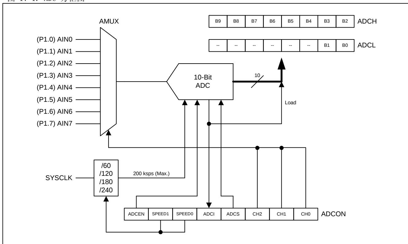
图 17-1. ADC 方框图
