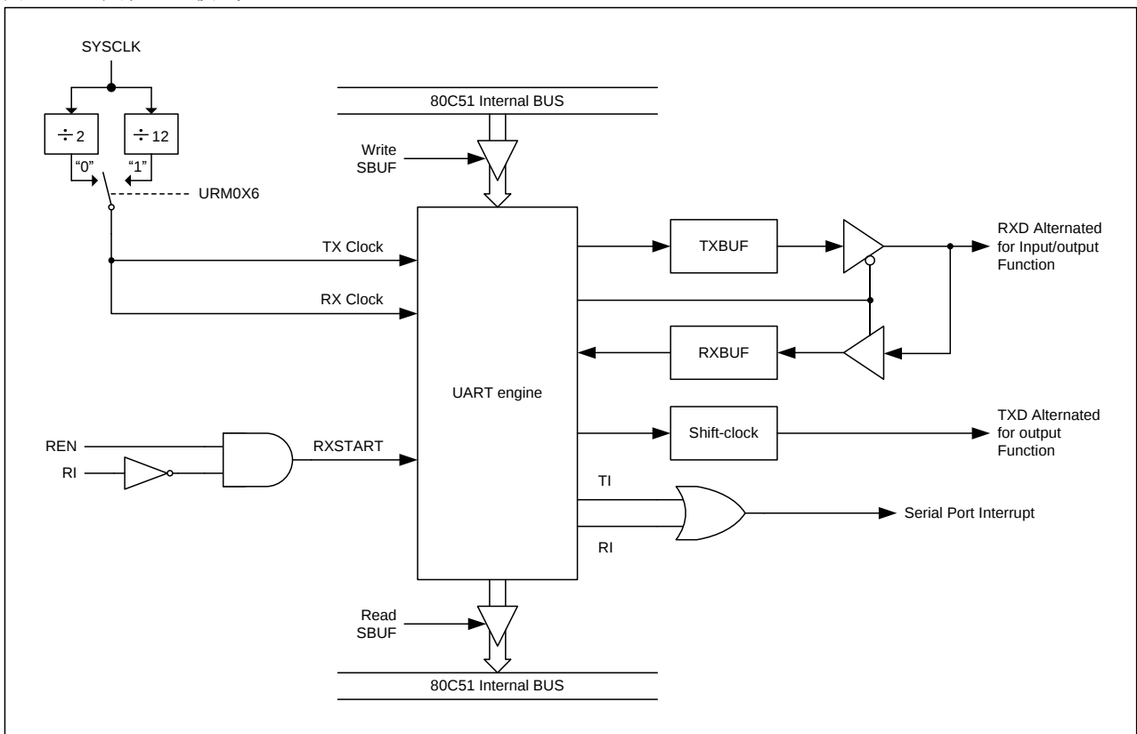
图 12-3 串行口 0 模式 0
