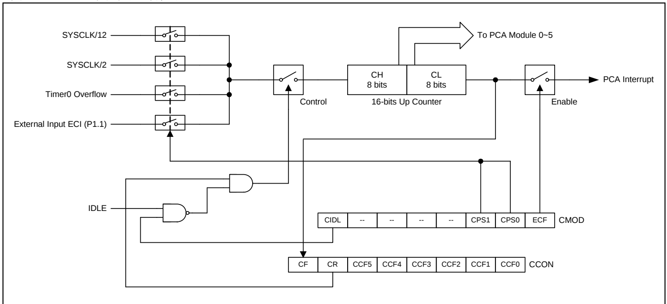
图 14-2. PCA 定时器/计数器
