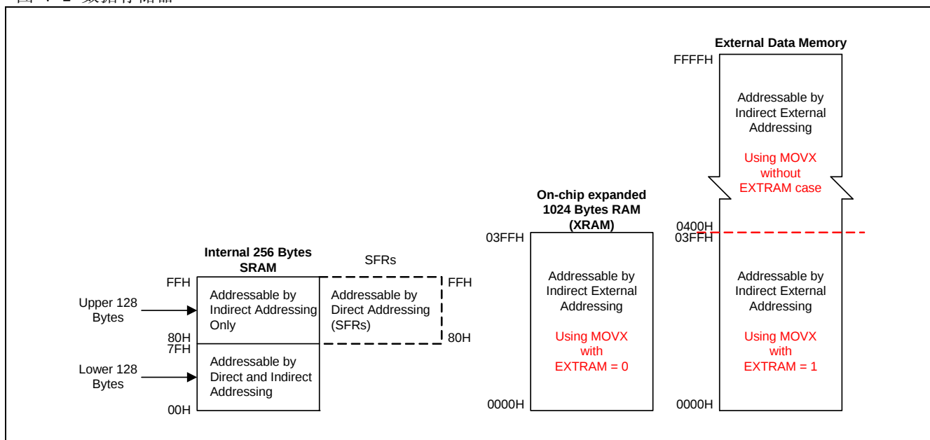
图 7-2 数据存储器
