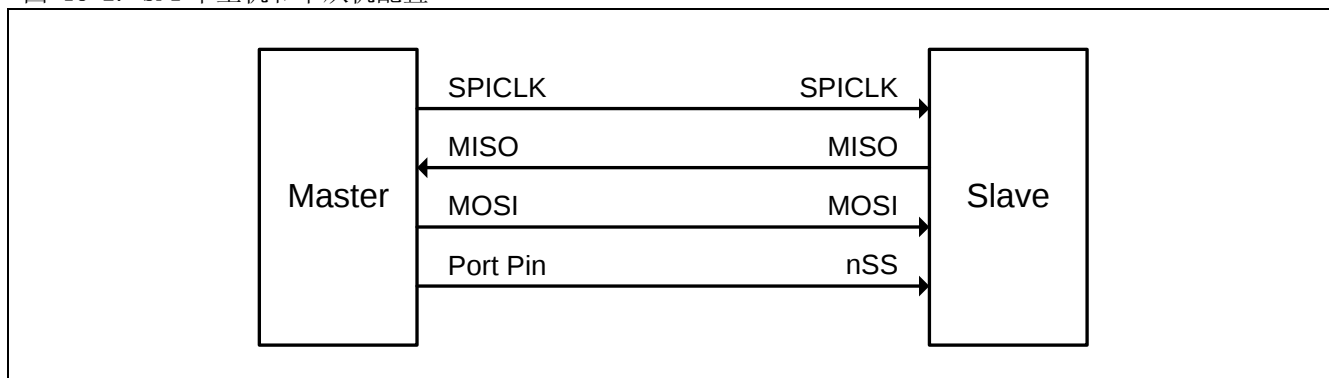
图 15-2. SPI 单主机和单从机配置
