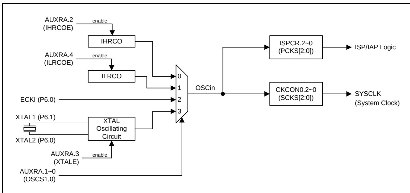
图 21-1. 系统时钟方框图
