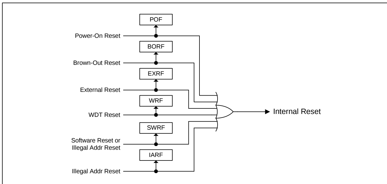
图 19-1. 复位源图示
