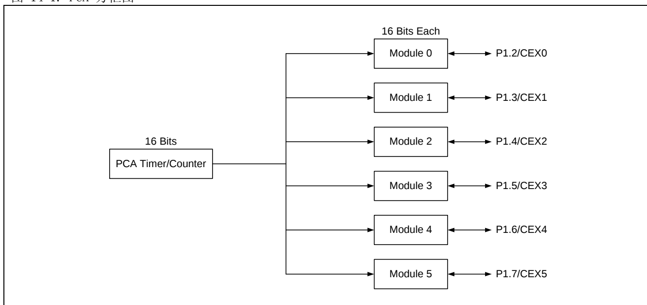
图 14-1. PCA 方框图
