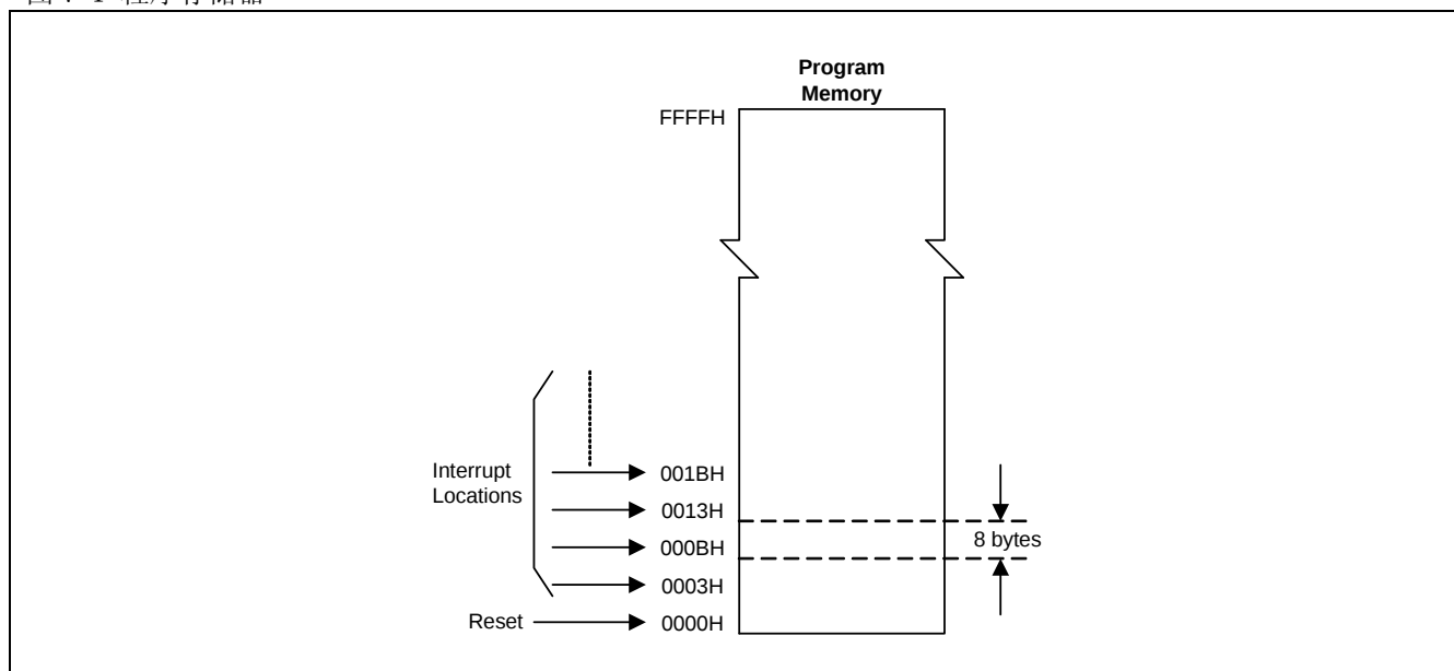
图 7-1 程序存储器
