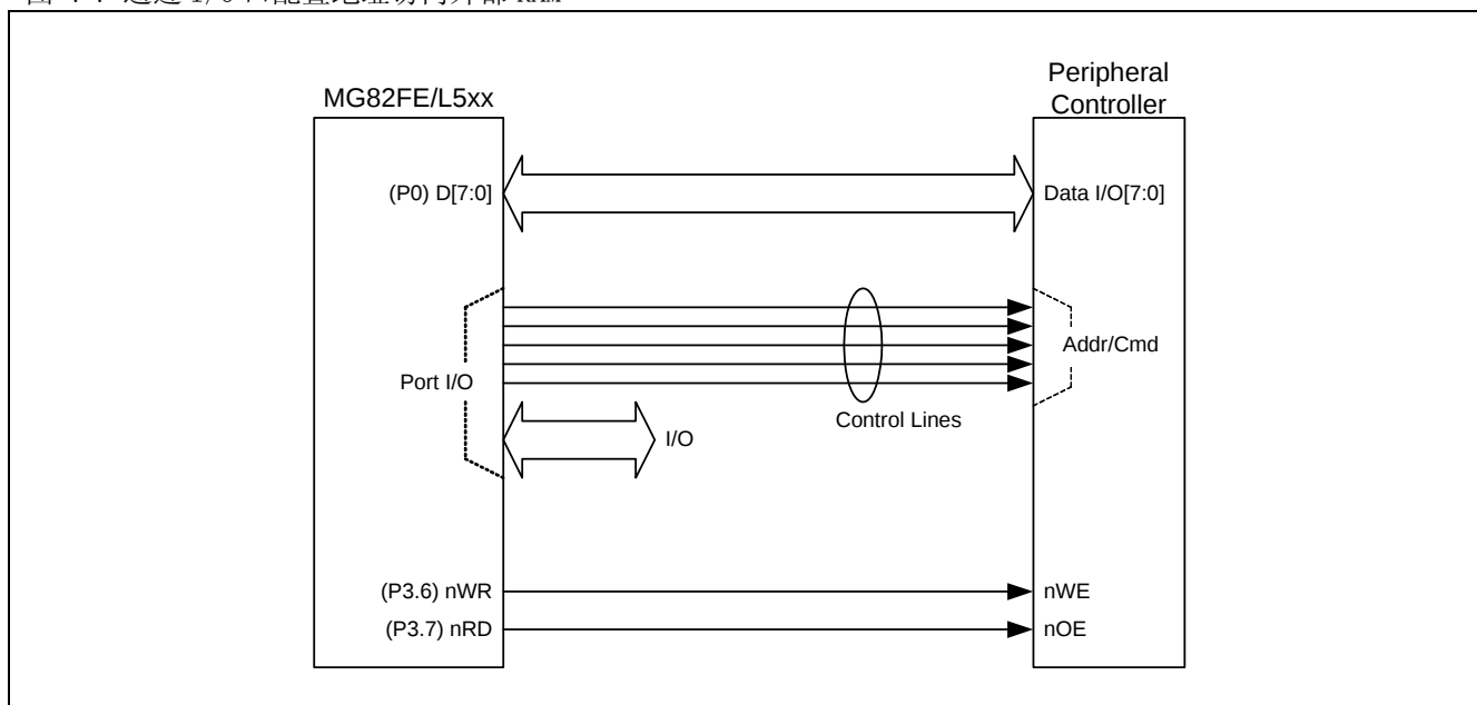
图 7-7 通过 I/O 口配置地址访问外部 RAM
