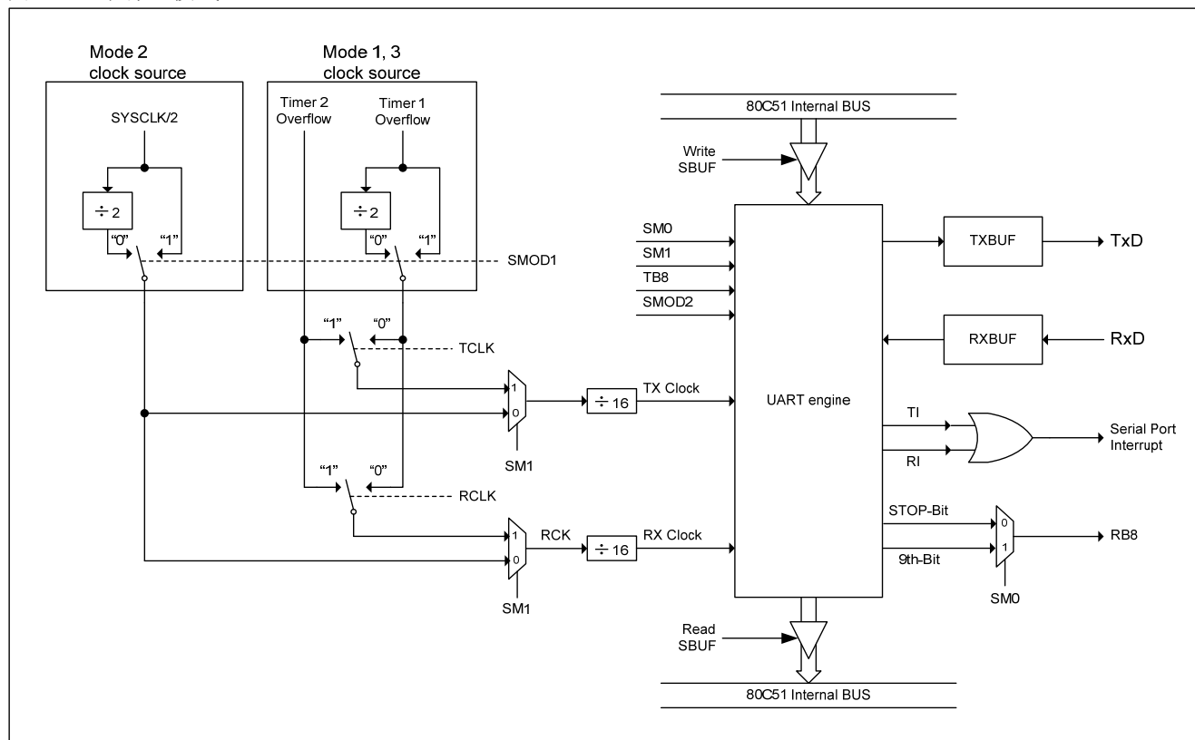
图 12-6 串行 0 模式 1、2、3
