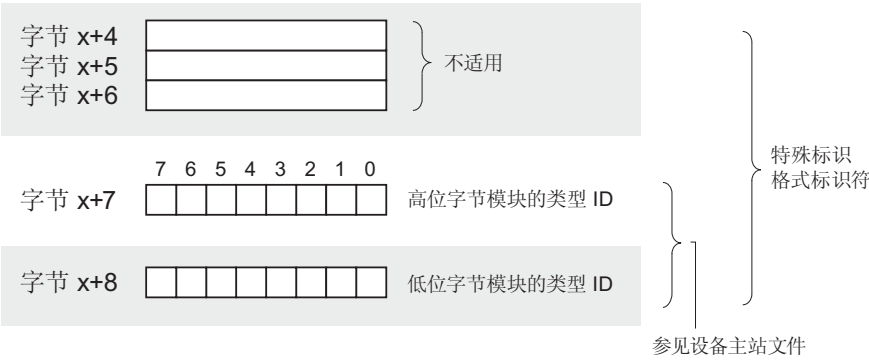
图 9-17 卸下/插入中断自字节 x+4 开始的结构
