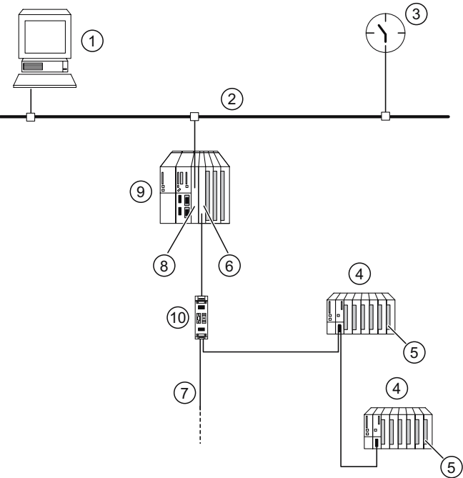
图 8-1 用 IM 153-2 实现时间标记信号更改的实例结构
