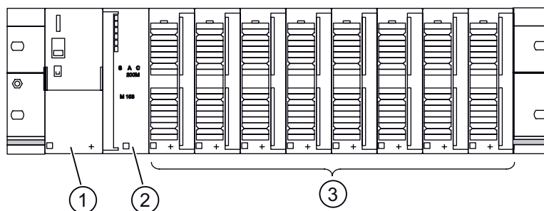
图 1-2 ET 200M 分布式 I/O 设备的组态（实例）
