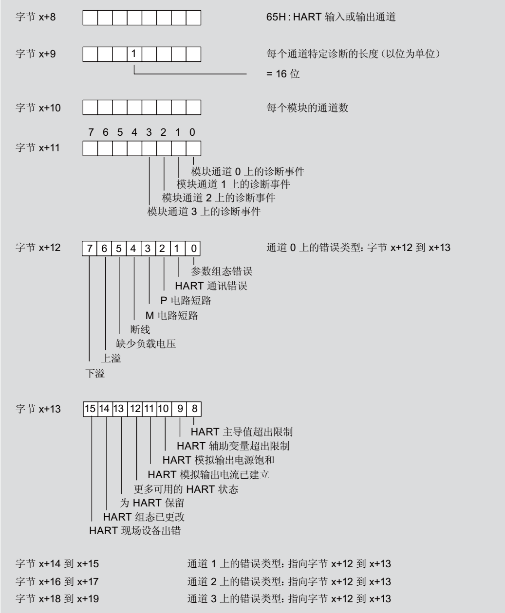
图 9-13 诊断中断自字节 x+8 开始的结构 (带有 HART 的输入或输出模块)
