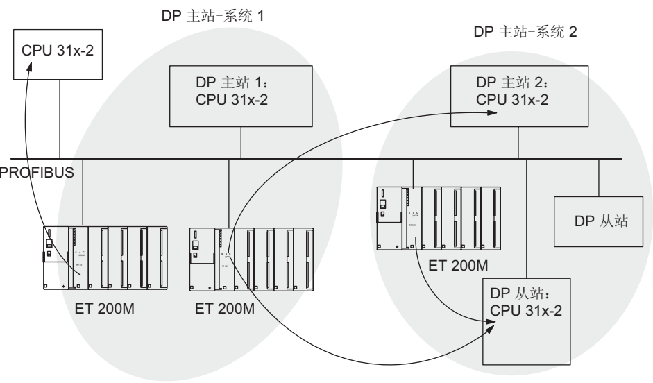
图 8-23 与 IM 153-x 的直接数据交换
