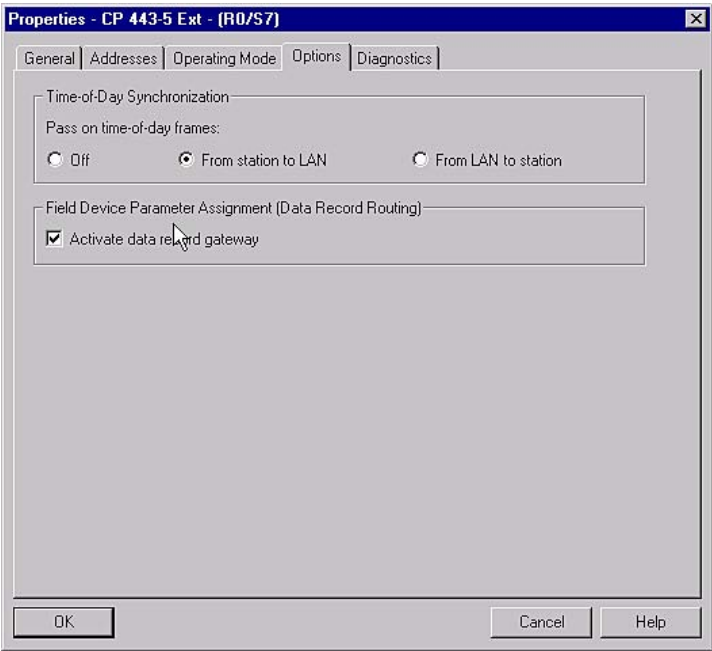
图 8-4 CP 443-5 扩展属性
