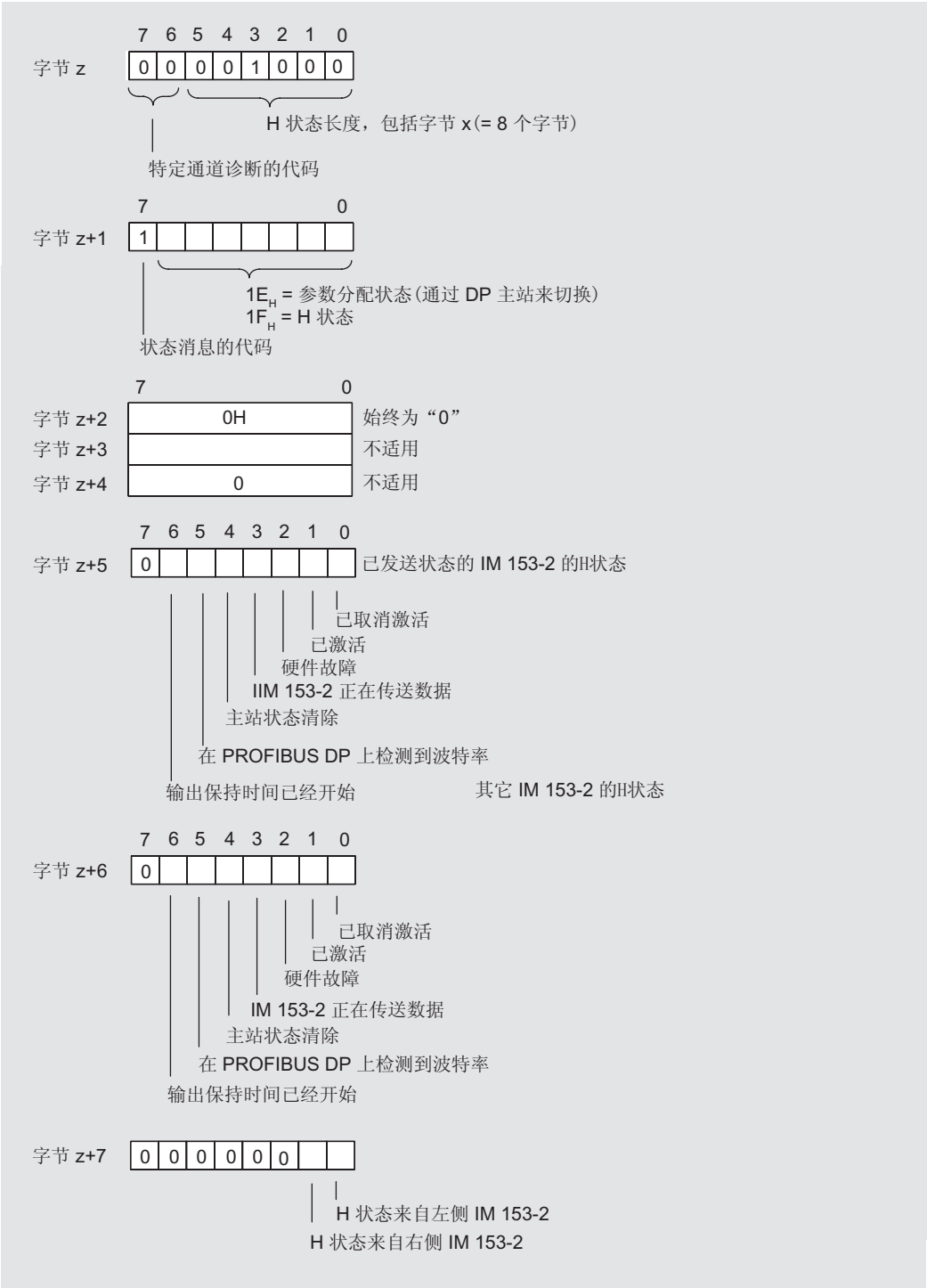
图 9-6 H 状态的结构
