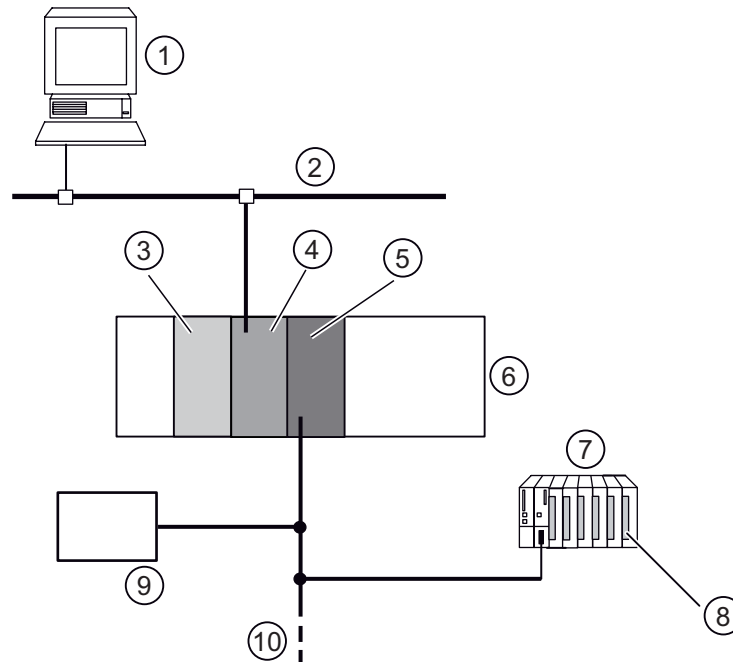
图 8-12 示例组态：作为 DP 主站和独立时间主站的通讯处理器
