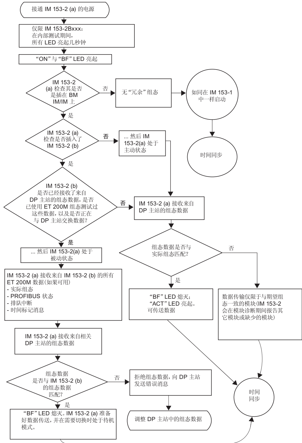
图 6-3 IM 153-2 的启动
