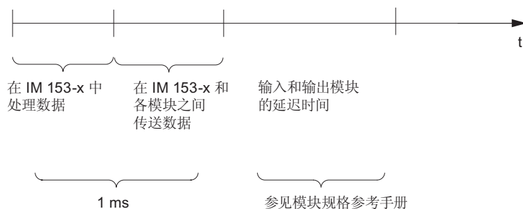
图 10-4 ET 200M 的响应时间
