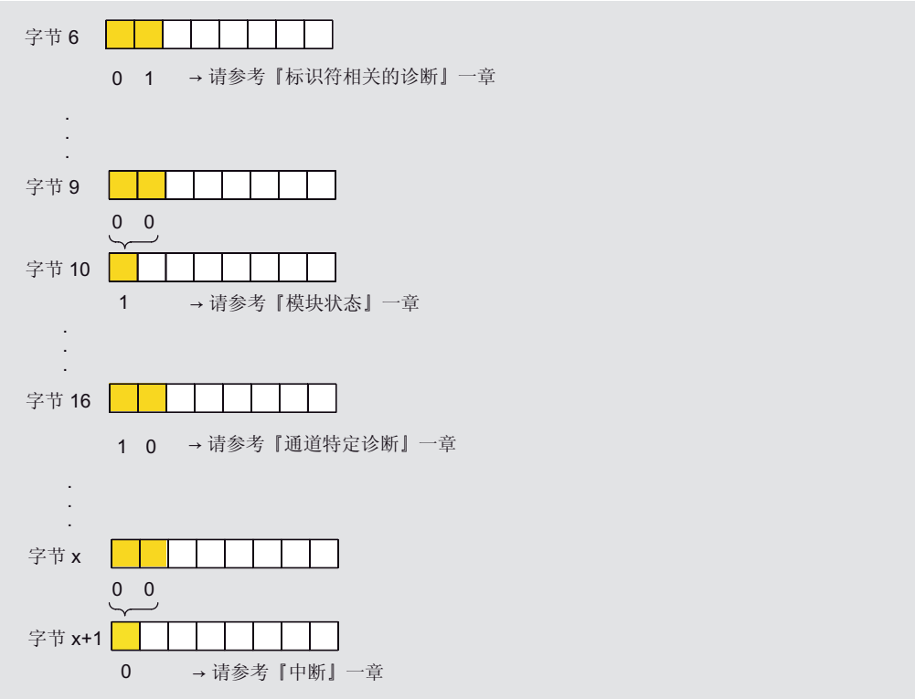
图 9-2 评估从站诊断
