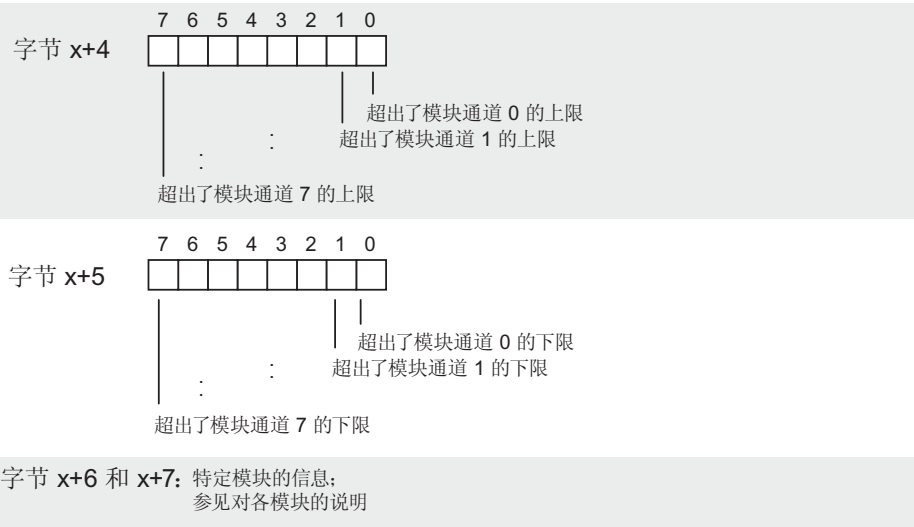
图 9-15 过程中断自字节 x+4 开始的结构（模拟输入）
