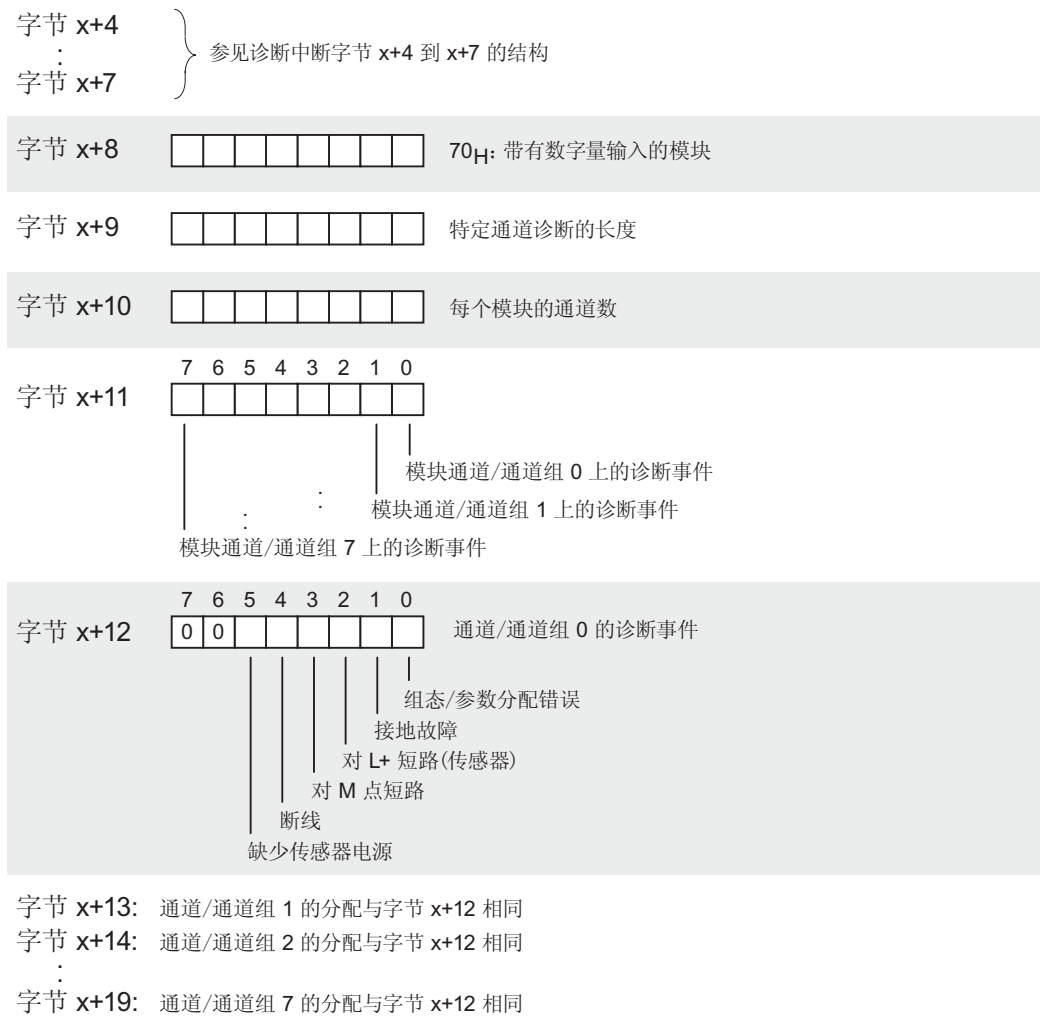
图 9-9 诊断中断自字节 x+8 开始的结构（数字输入）
