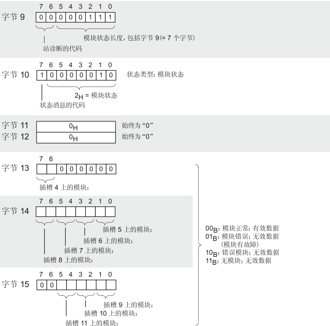
图 9-4 ET 200M 的模块状态的组态
