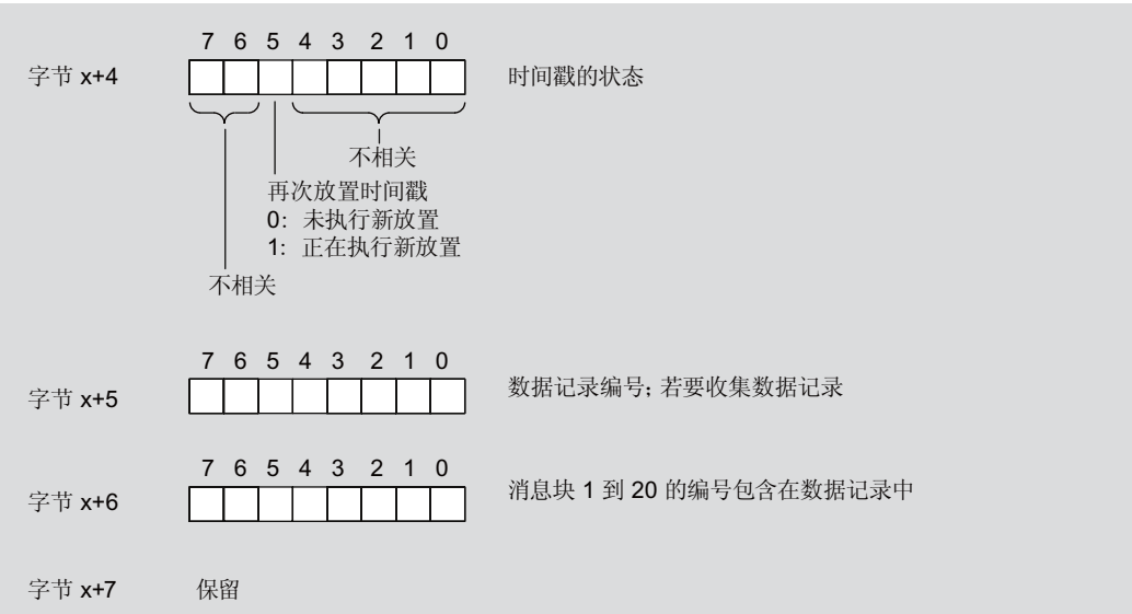
图 9-14 过程中断自字节 x+4 开始的结构（时间戳）
