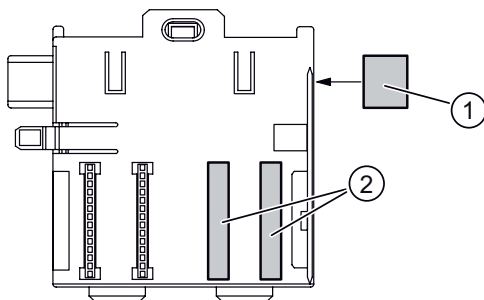
图 3-8 实例：总线模块 2 x 40 (...-7HB00-)
