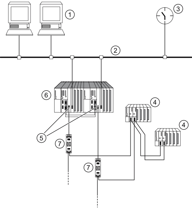
图 8-7 在 H 系统中将 2 个 IM 153-2 用作冗余的实例结构
