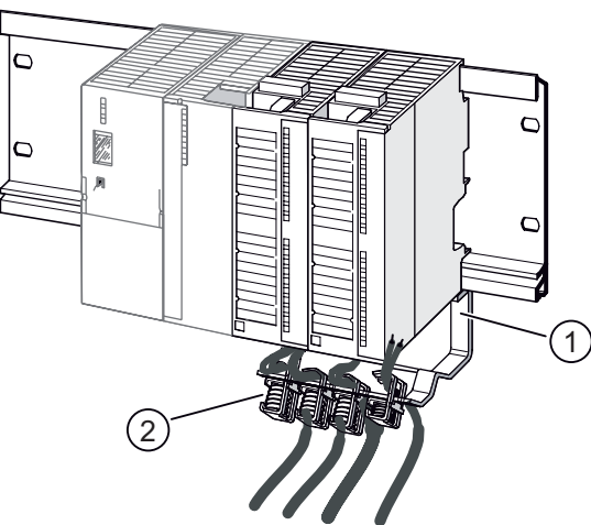
图 5-4 将带屏蔽的 2 线电缆放置在屏蔽接触元件上
