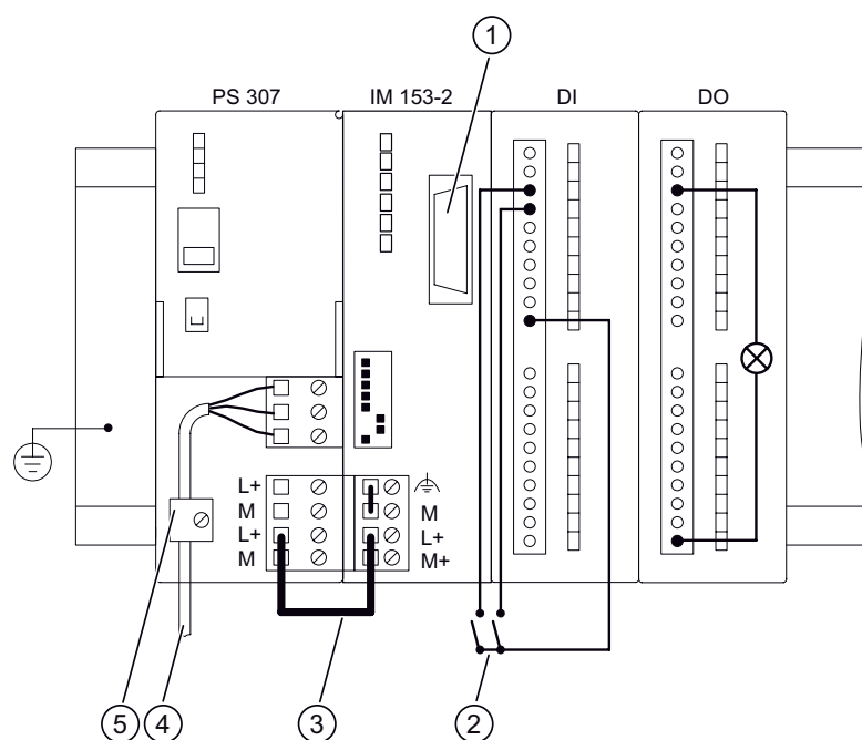
图 2-3 ET 200M 接线
