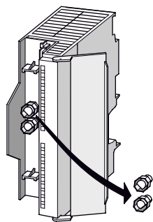
图 7-2 卸下前连接器编码设备
