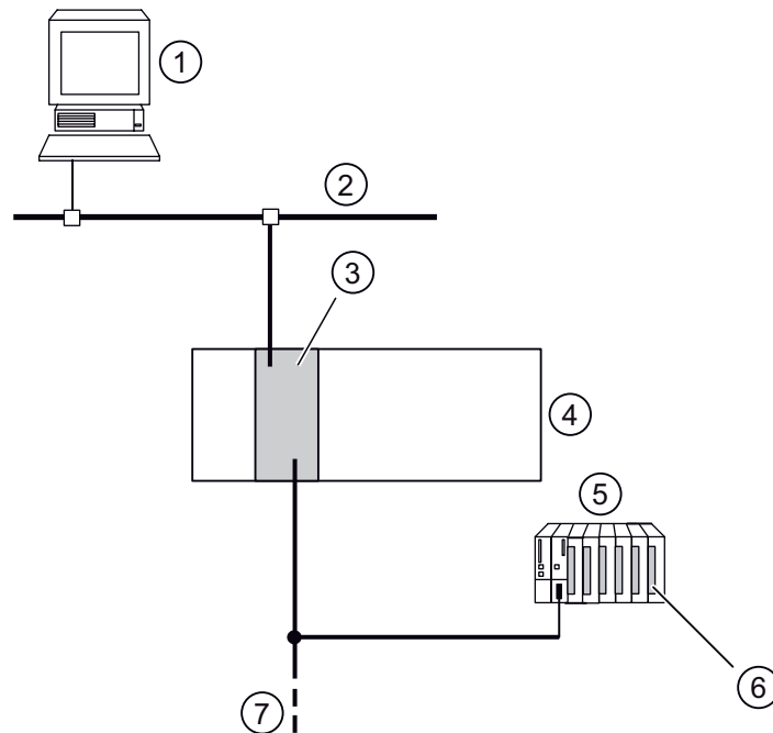
图 8-10 示例组态：集成 DP 主站转发从 CPU（时钟主站）中接收的时间
