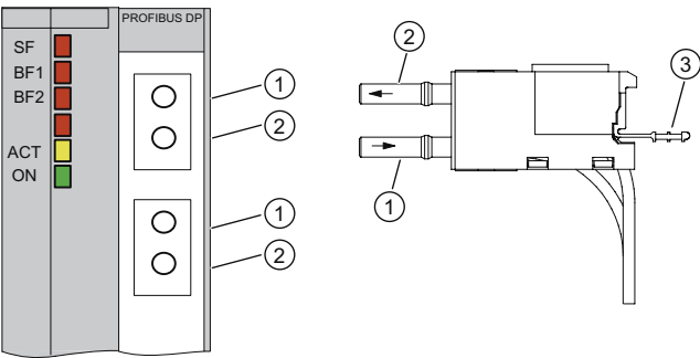
图 5-1 将 FOC 连接至 IM 153-2 FO
