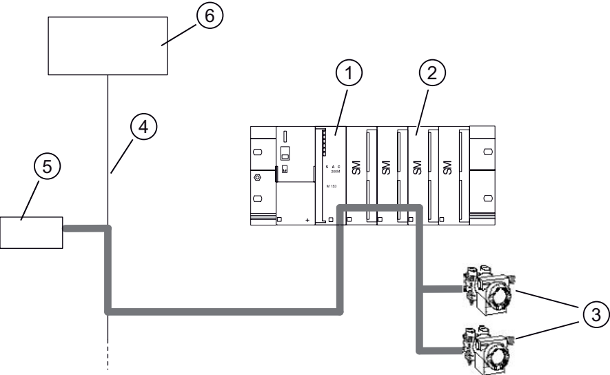
图 3-2 使用 IM 153-2 和 HART 模块传递参数分配数据
