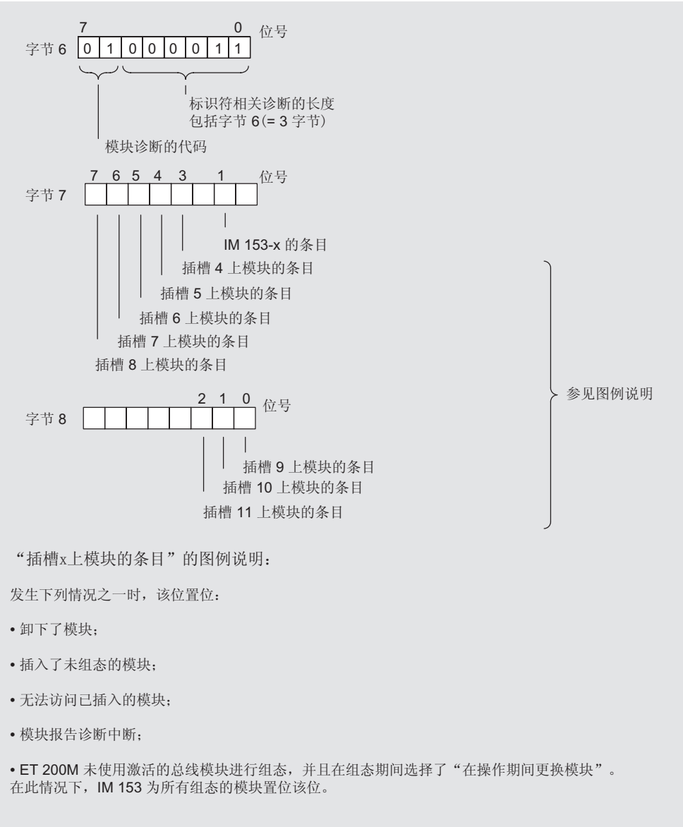
图 9-3 标识符相关的诊断的结构
