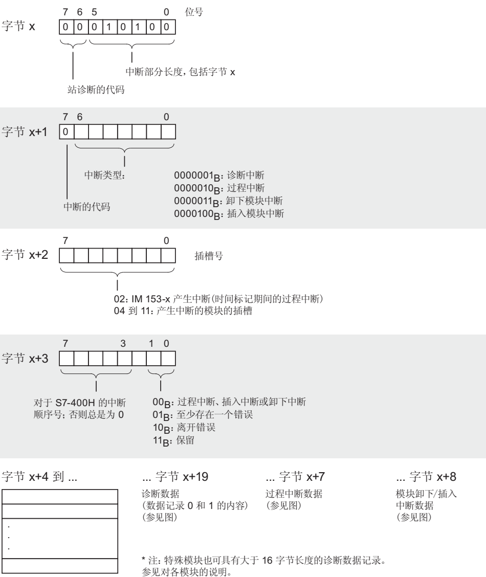
图 9-7 中断部分的中断状态的结构
