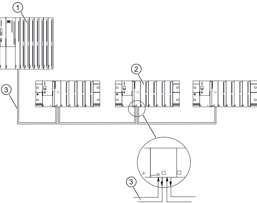
图 3-4 使用 IM 153-2 FO 的 FOC 网络
