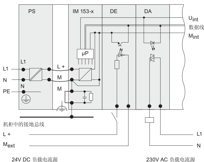
图 3-13 具有隔离模块的组态的简单表示
