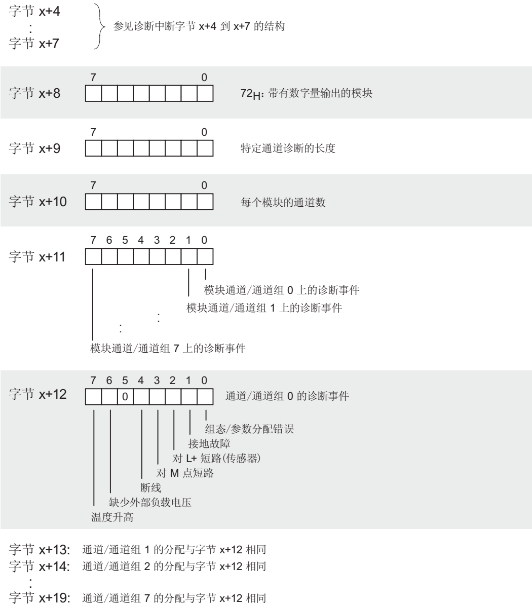
图 9-10 诊断中断自字节 x+8 开始的结构（数字输出）
