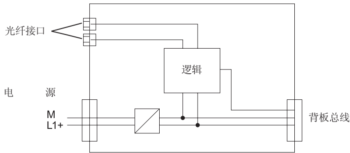
图 10-3 IM 153-2 FO 的方框图
