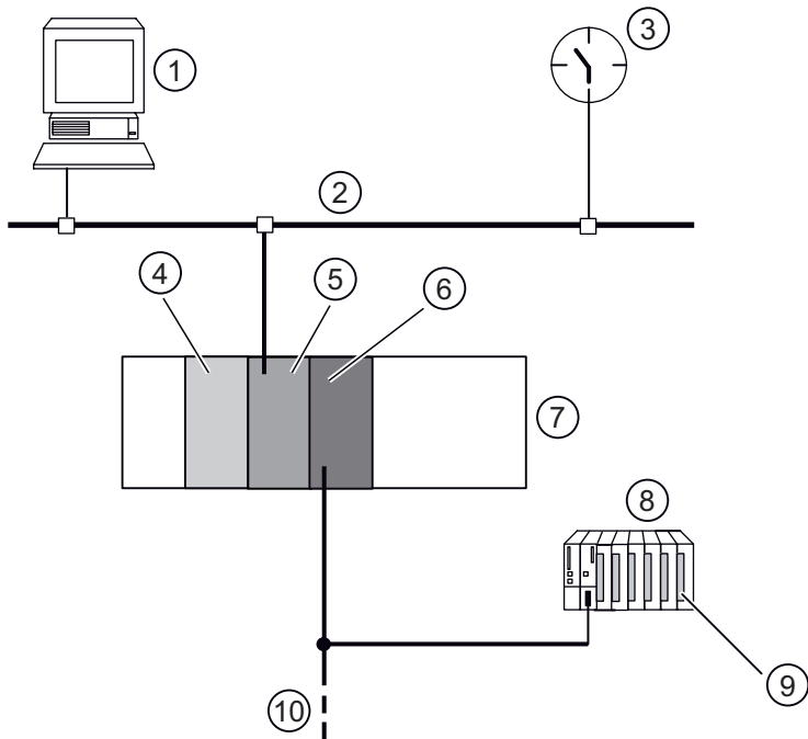
图 8-11 示例组态：作为 DP 主站和 DP 时钟主站的通讯处理器
