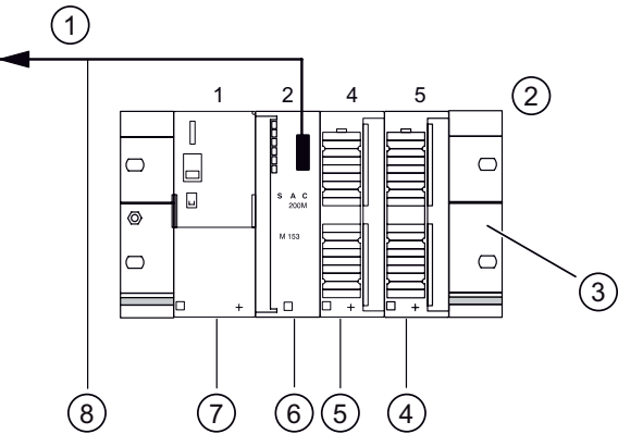
图 2-1 用于实例组态的 ET 200M 组件
