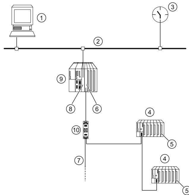
图 8-9 用 IM 153-2 实现时间标记信号更改的实例结构
