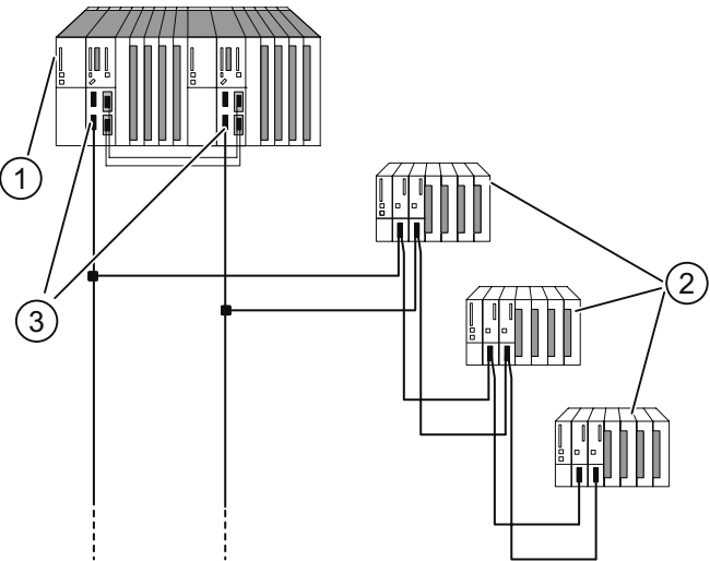
图 8-19 在 H 系统中 2 x IM 153-2 的冗余
