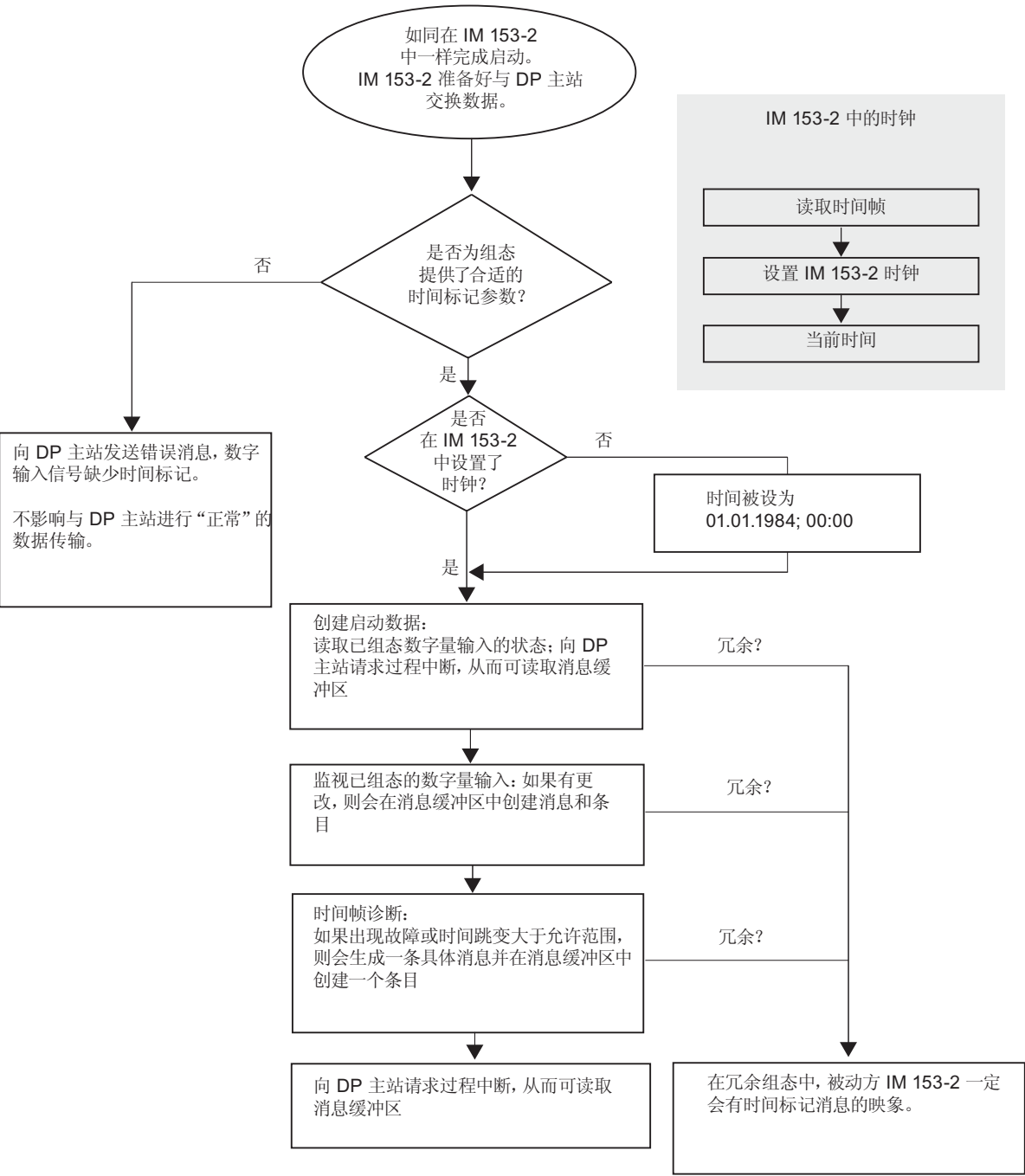
图 6-4 时间同步/时间标记的启动
