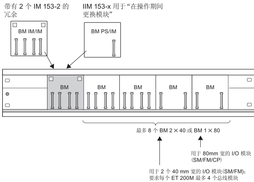
图 3-9 具有有源总线模块的组态
