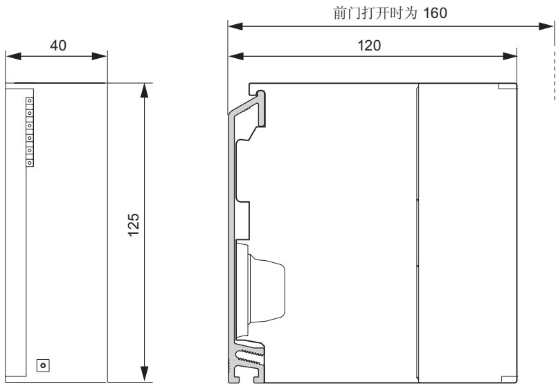
图 10-1 接口模块 IM 153-1、IM 153-2 和 IM 153-2 FO 的尺寸图
