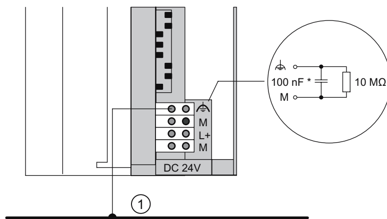
图 3-12 具有未接地参考电位的 ET 200M 的组态
