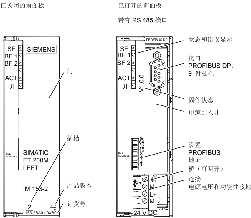
图 1-5 IM 153-2Bxx1 的正视图
