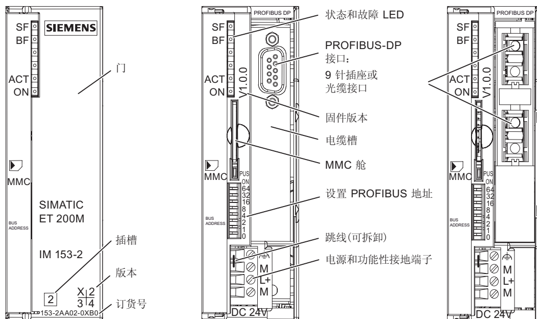
图 1-4 IM 153-2Bx00 的正视图
