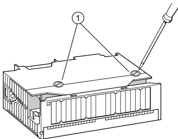
图 7-3 数字输出模块上保险丝的位置
