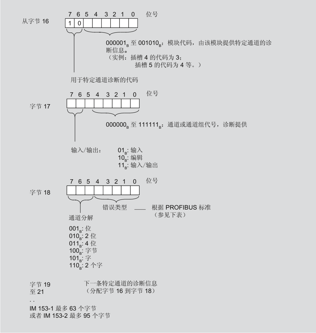
图 9-5 特定于通道的诊断结构
