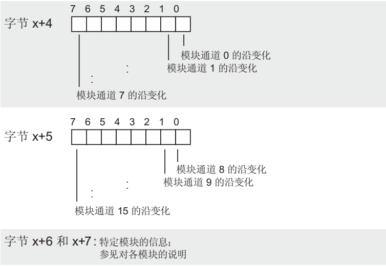
图 9-16 过程中断自字节 x+4 开始的结构（数字输入）
