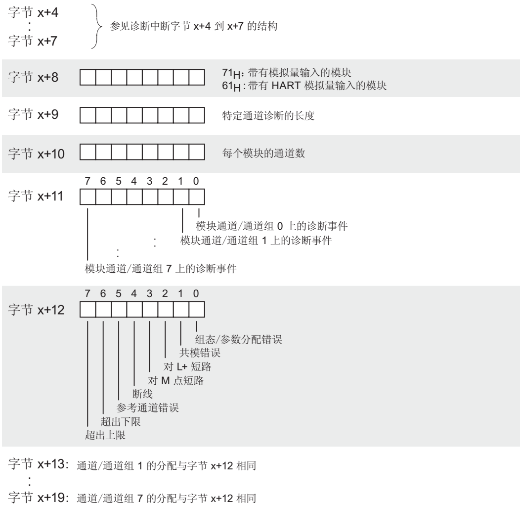
图 9-11 诊断中断自字节 x+8 开始的结构（模拟输入）
