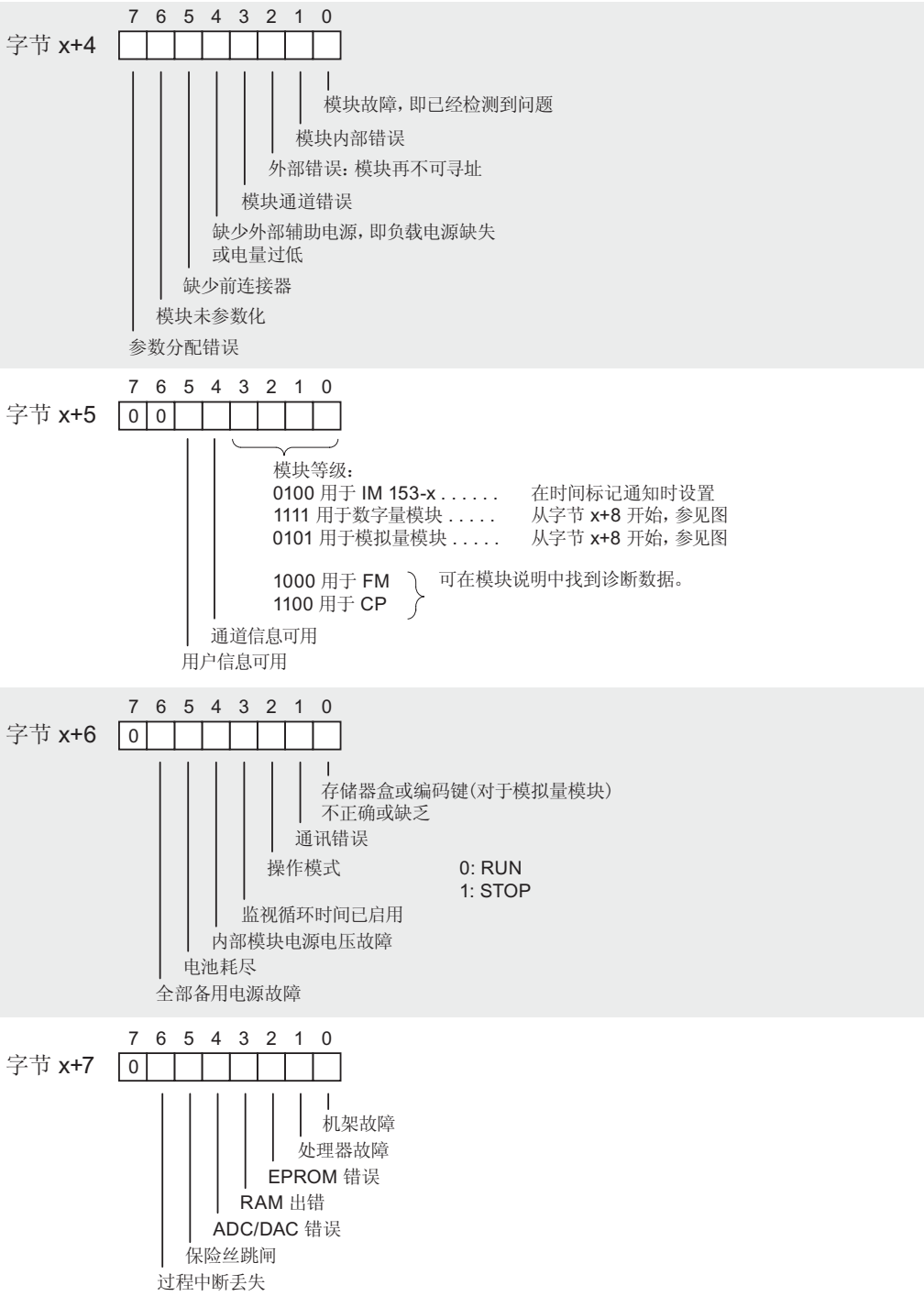
图 9-8 有关数字和模拟模块的诊断中断的附加中断信息
