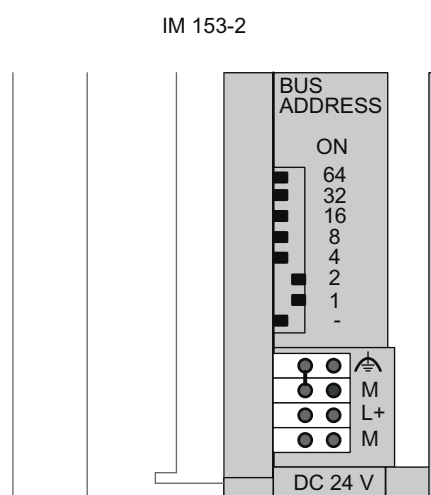
图 2-2 将 PROFIBUS 地址设置为 3
