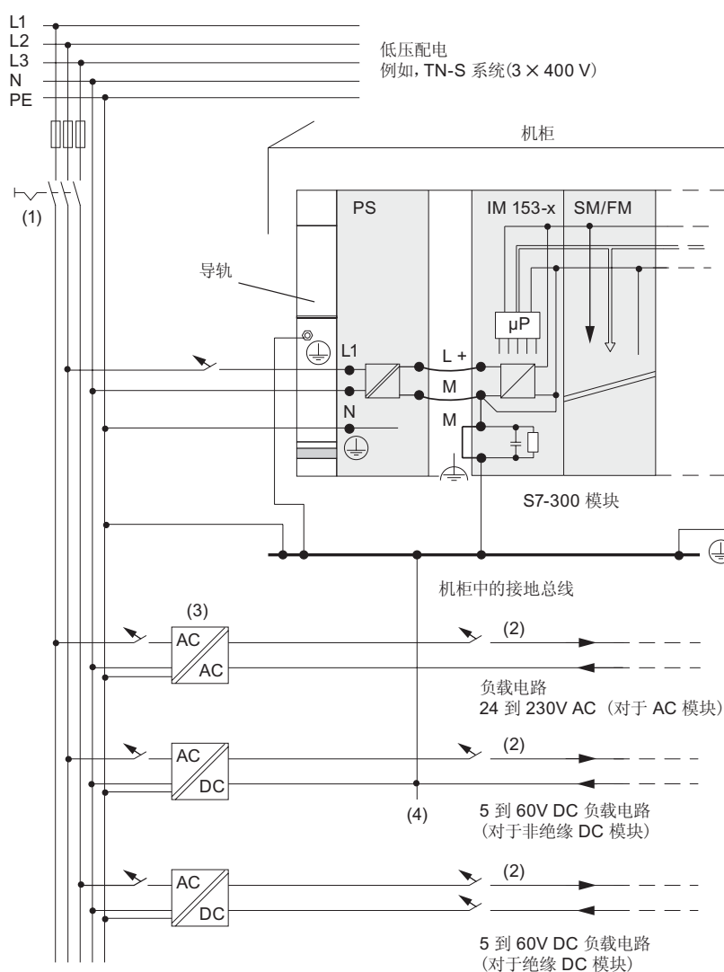
图 3-10 以接地电源运行 S7-300 模块
