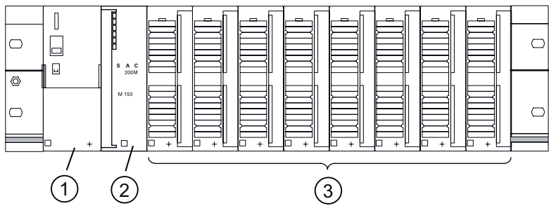
图 3-7 ET 200M 模块的排列
