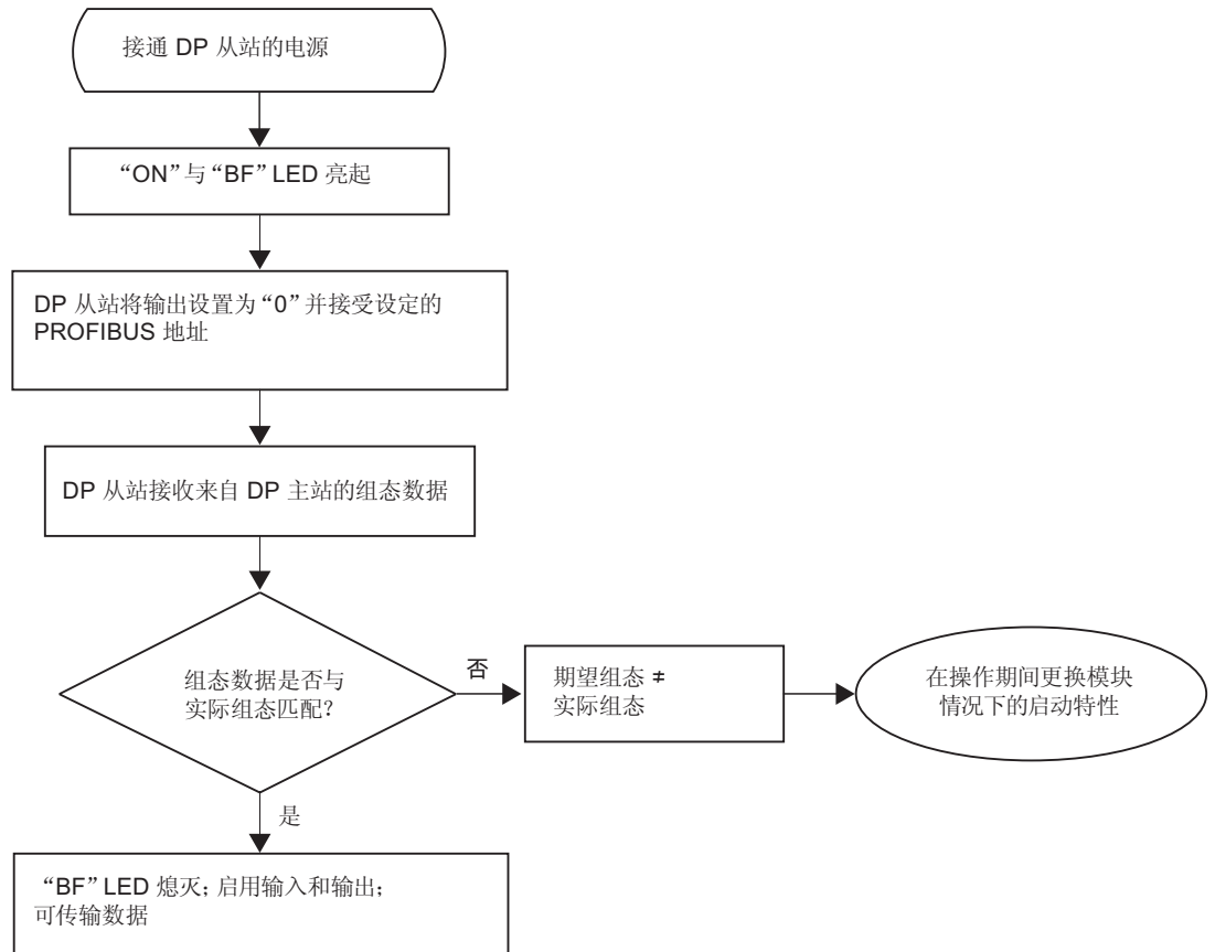
图 6-1 IM 153-1 的启动
