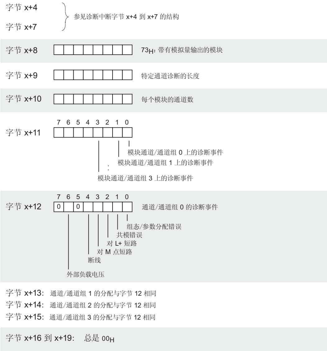
图 9-12 诊断中断自字节 x+8 开始的结构（模拟输出）
