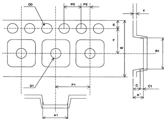
Fig. 3 Tape dimensions
