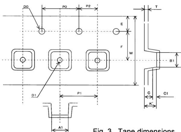
Fig. 3 Tape dimensions
